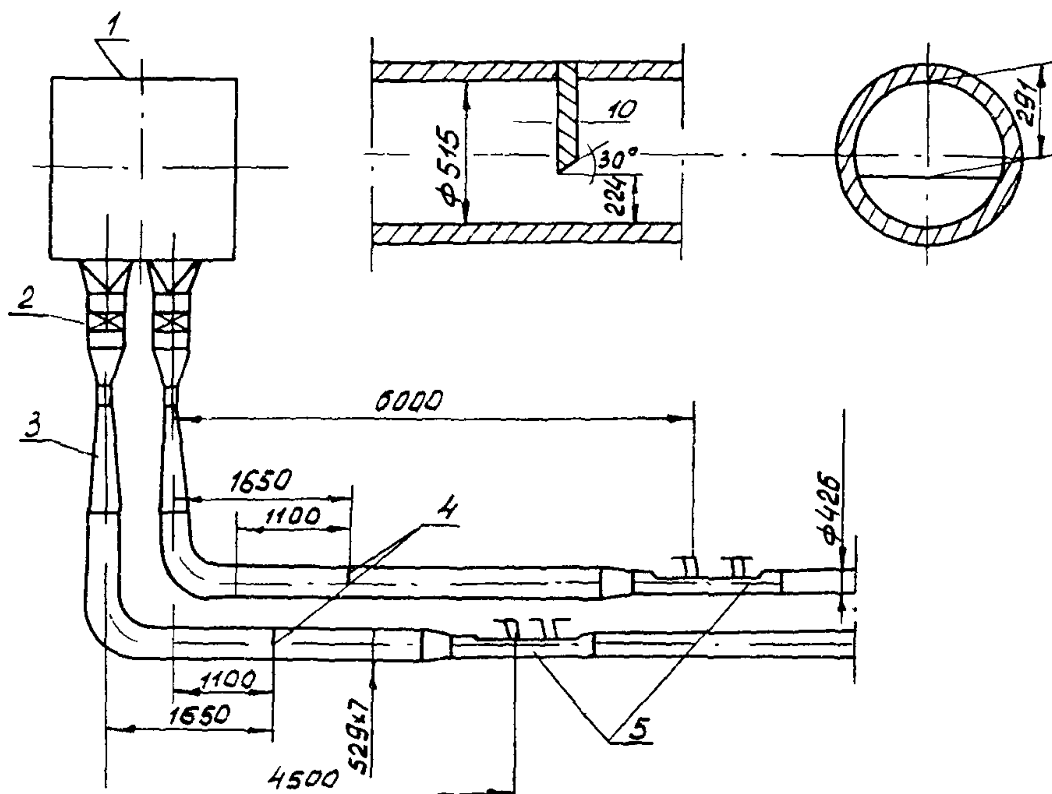
Рис. 5. Схема установки сегментных диафрагм на коротких пылепроводах котла ТПП-200:
