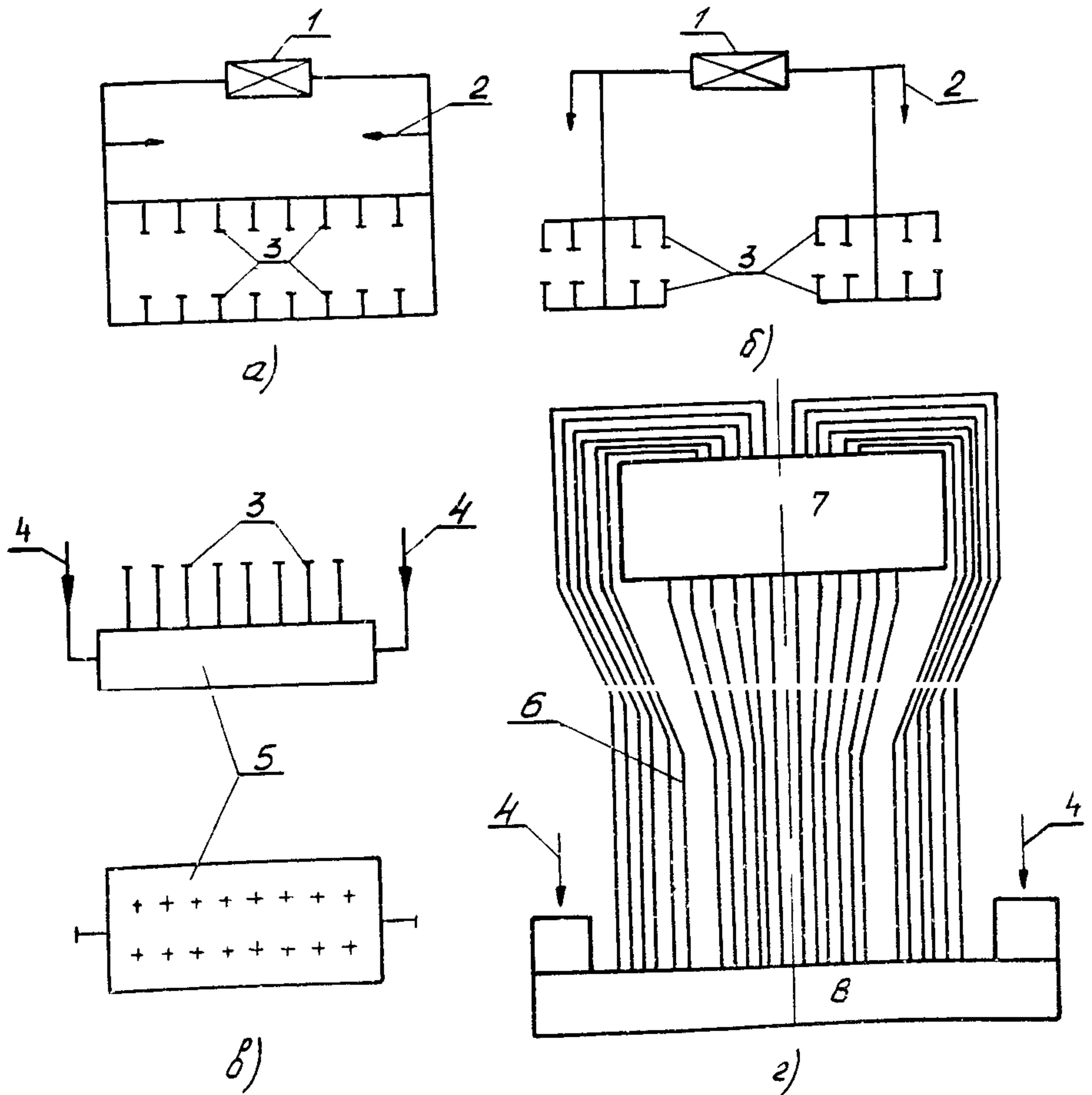
Рис. I. Схемы распределения вторичного (а, б, в) и первичного (г) воздуха по горелкам:
