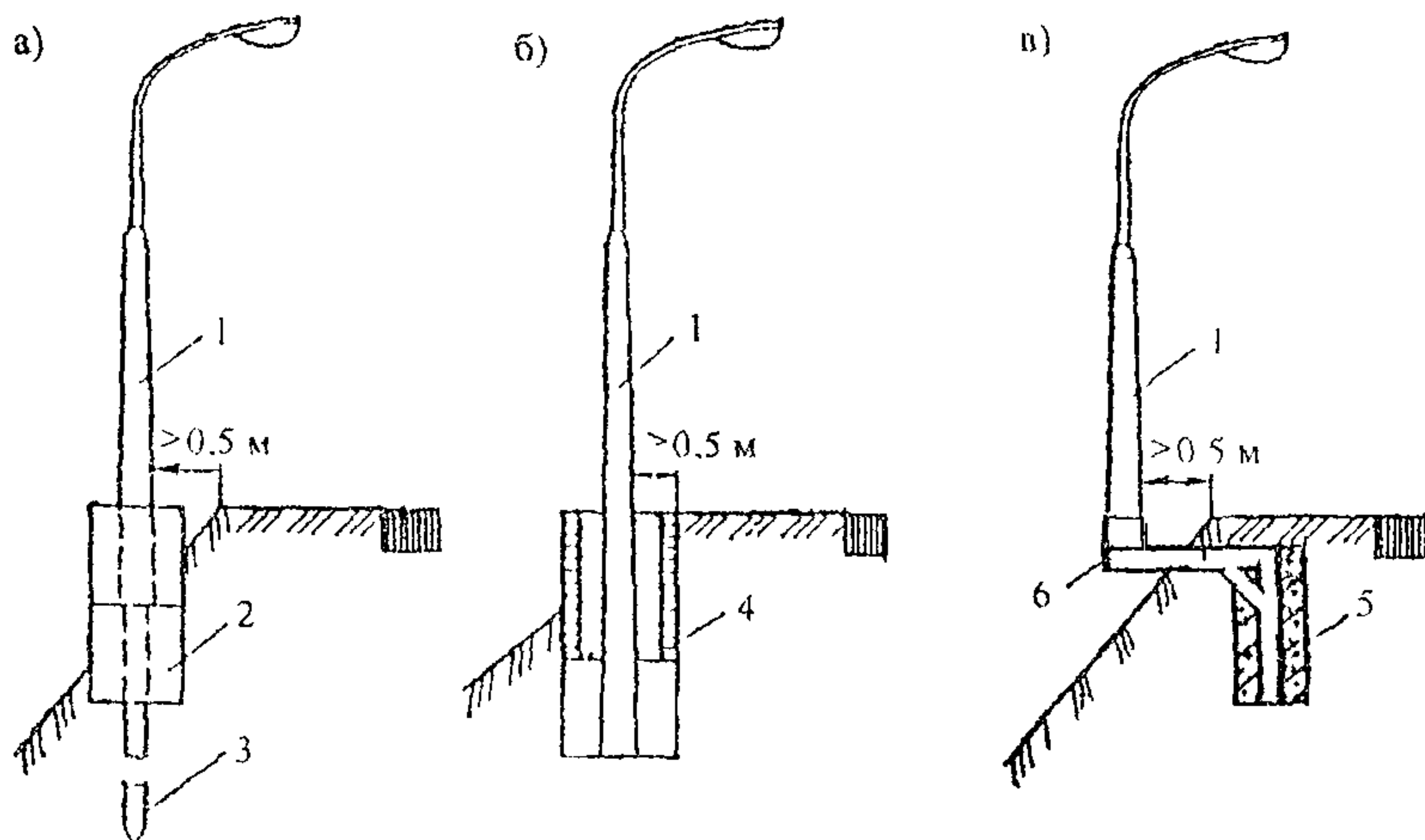
Рис. 15.1. Схема заделки в грунт опор освещения: а – при благоприятных условиях; б – в пучинистых грунтах; в – при наличии подземных коммуникаций; 1 – опора; 2 – оголовок; 3 – свая; 4 – деревянный короб; 5 – бетонный фундамент; 6 – металлический Г-образный фундамент
