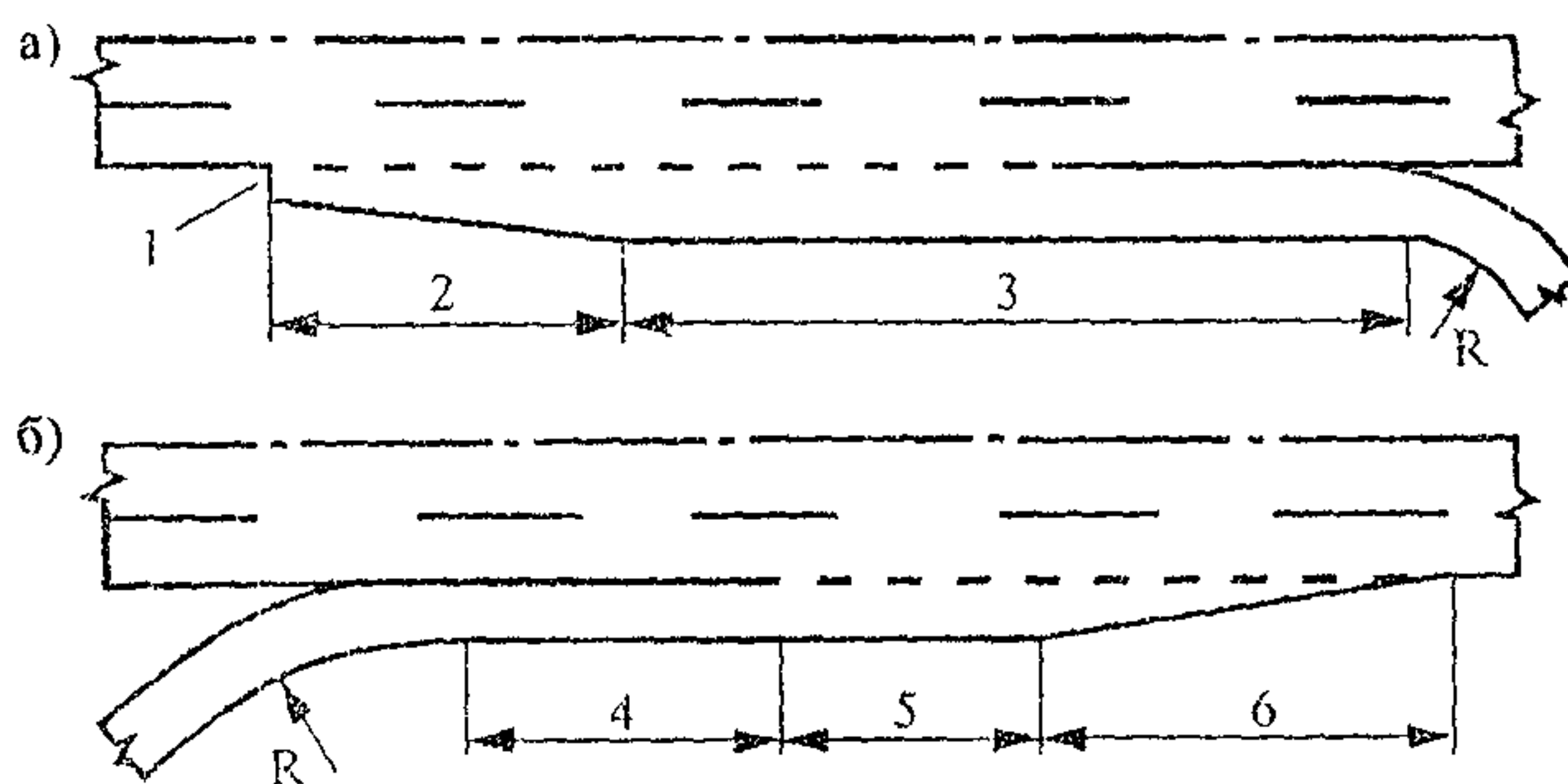
Рис. 9.1. Элементы полос торможения (а) и разгона (б): 1 – уступ шириной 0,5 м; 2 – участок смены полосы движения (отгон ширины полосы); 3 – участок снижения скорости; 4 – участок ускорения; 5 – участок маневрирования
