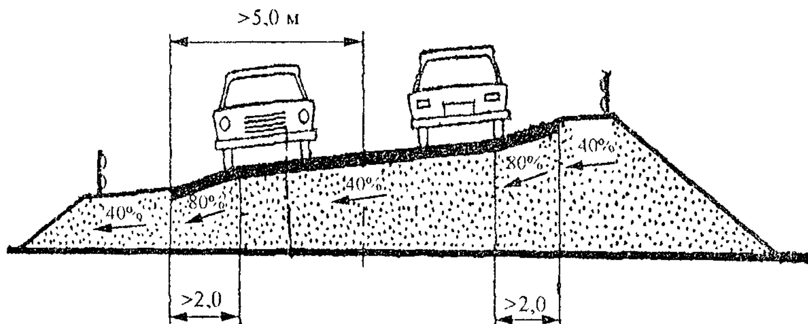
Рис. 4.1. Схема устройства ступенчатого виража на кривых малого радиуса
