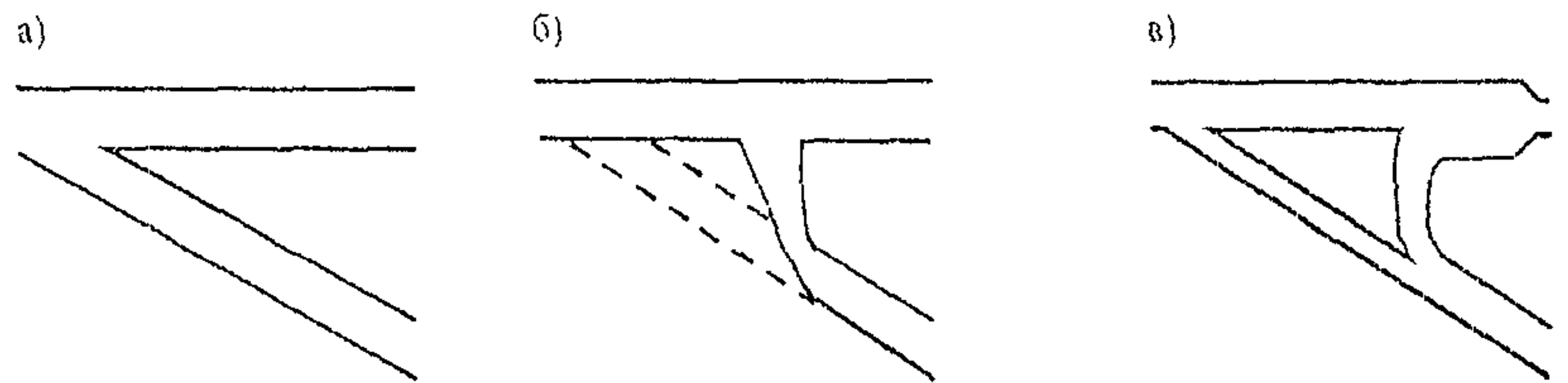
Рис. 8.4. Способы реконструкции примыканий дорог: а – неправильная планировка примыкания; б – улучшение условий движения путем смещения места примыкания; в – устройство дополнительной полосы
