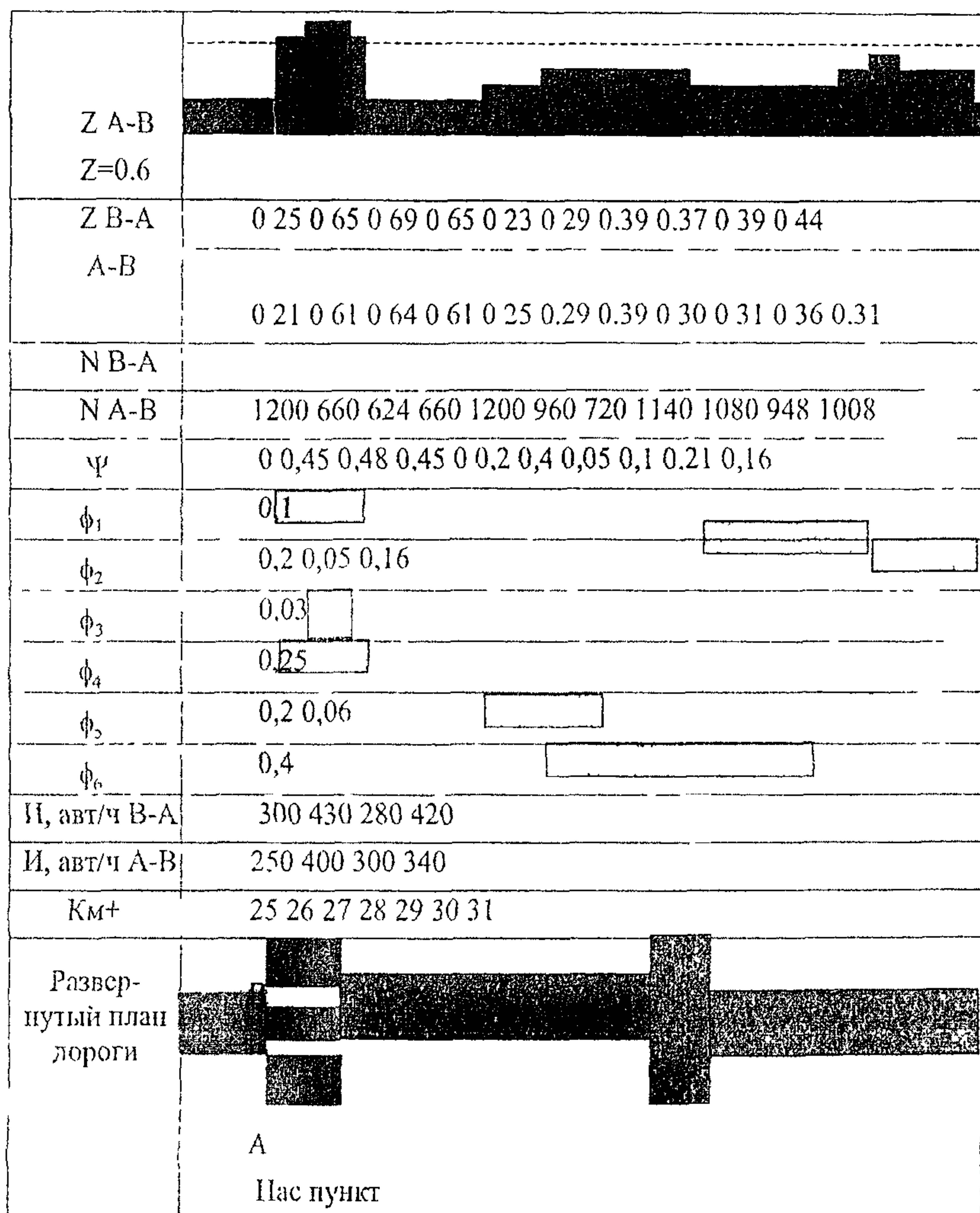
Рис. П-4.1. Линейный график пропускной способности и уровня загрузки дороги
