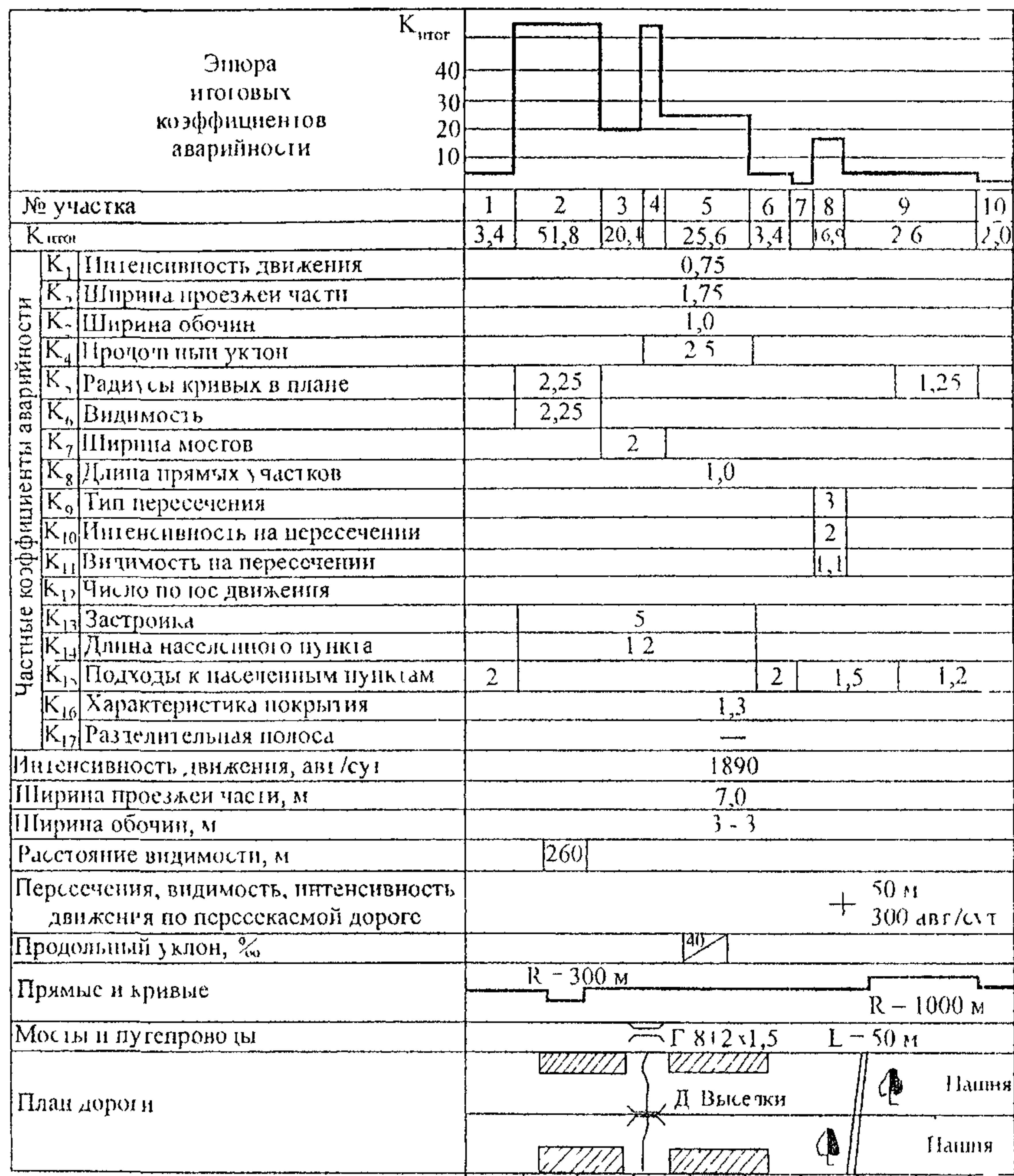
Рис. 1.2. Пример графика итогового коэффициента аварийности 1.4.8.
