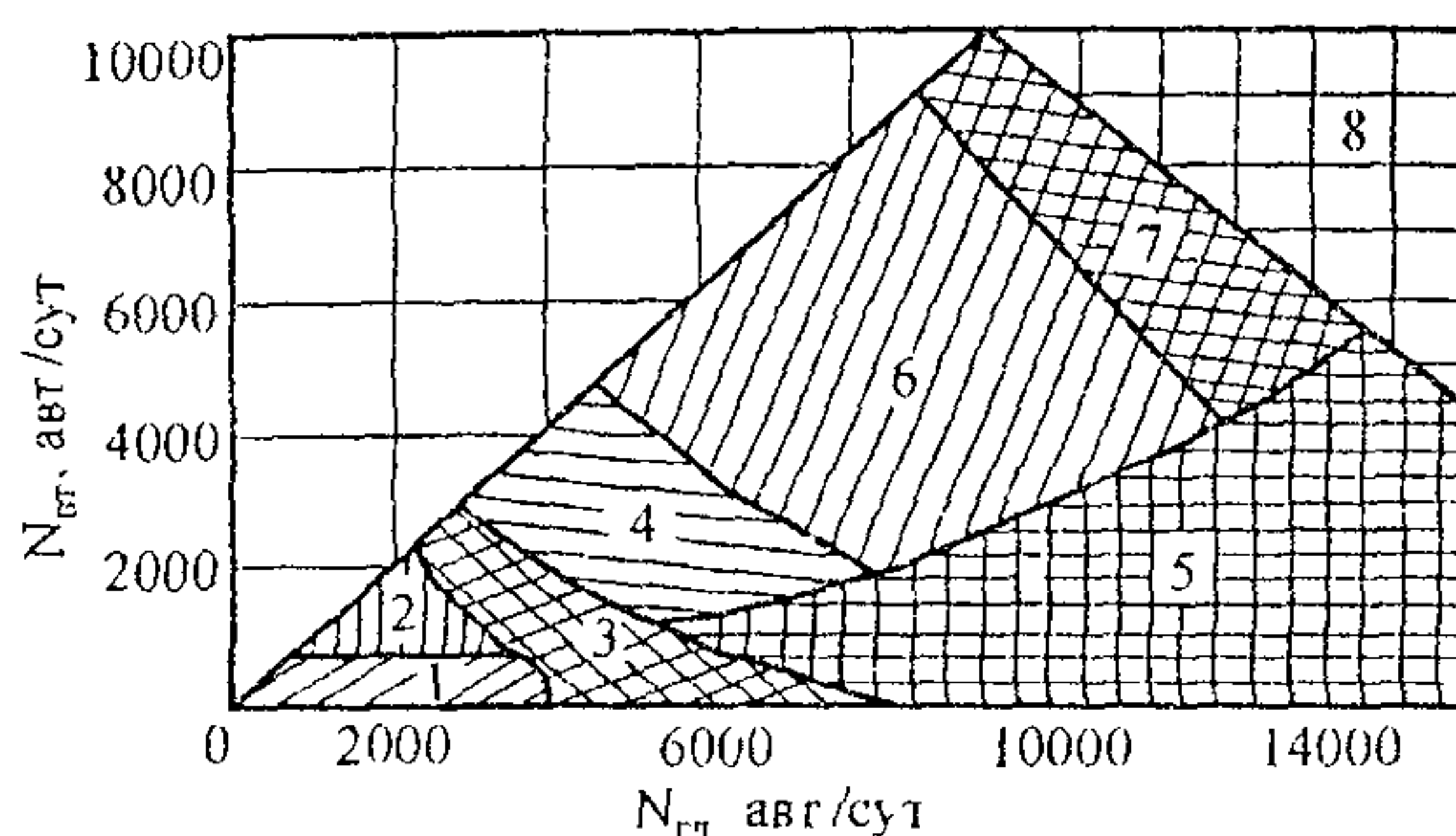
Рис. 8.1. Номограмма для выбора типа планировочных решений пересечений:
