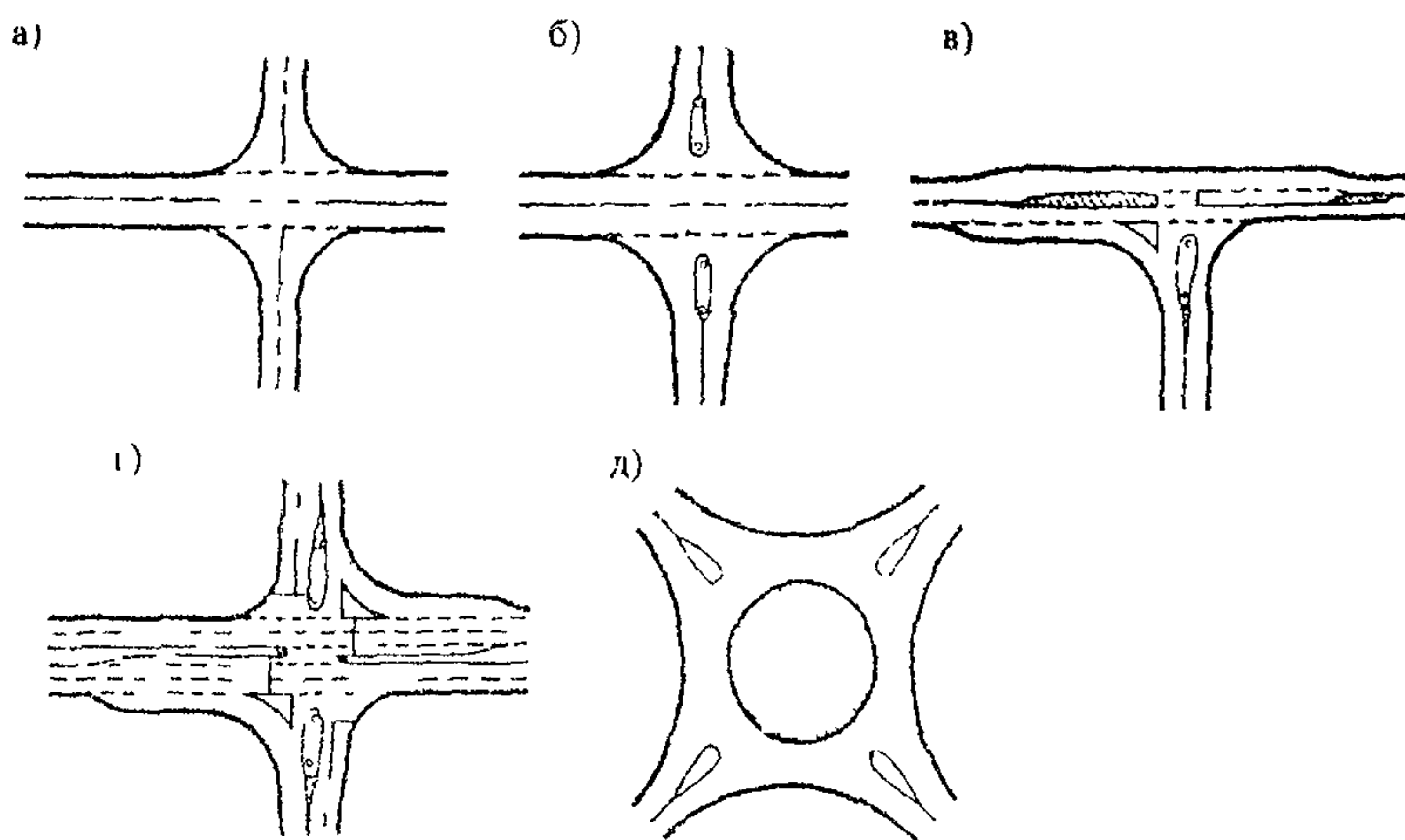
Рис. 8.2. Схемы планировочных решений пересечений: а – простое необорудованное пересечение; б – частично канализированное пересечение с направляющими островками на второстепенной дороге; в, г – полностью канализированное примыкание и пересечение с направляющими островками на обеих дорогах, с переходно-скоростными полосами; д – кольцевые саморегулируемые пересечения
