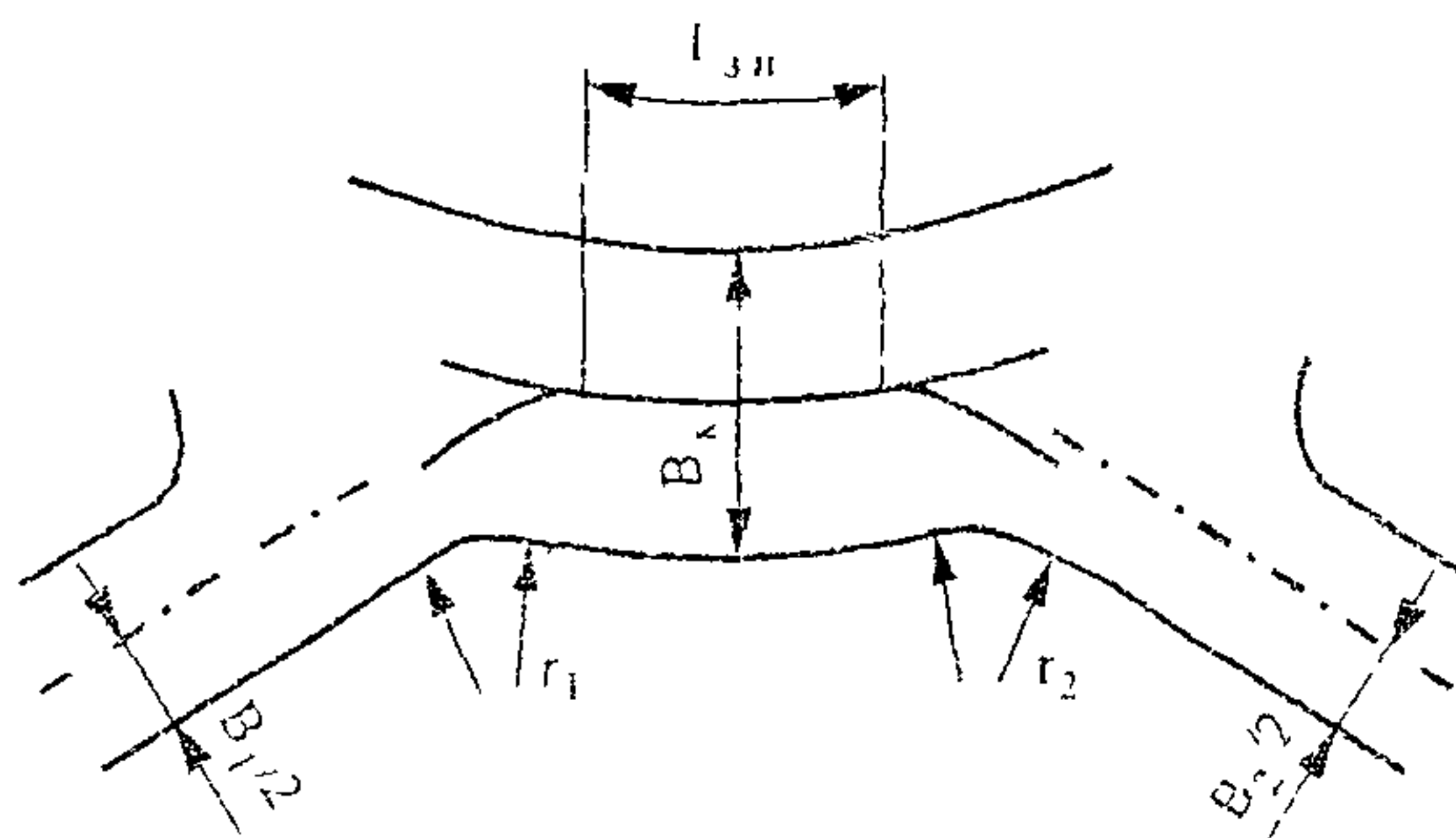
Рис. 8.16. Схема к расчету диаметра центрального островка на кольцевом пересечении:
