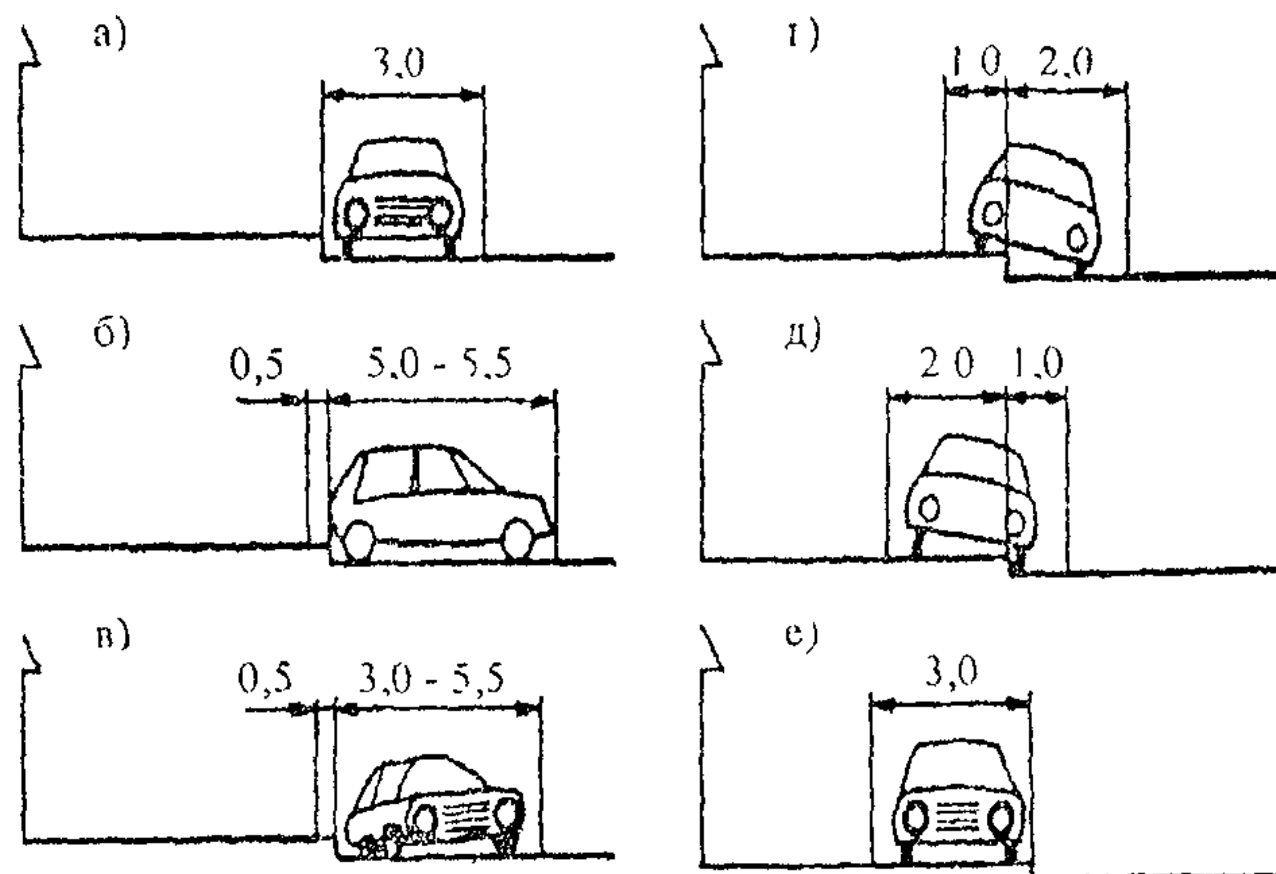
Рис. 11.6. Размещение стоянок в пределах улиц: а - расстановка автомобилей вдоль улицы; б - поперечная расстановка; в - расстановка под углом; г-д - частичное использование тротуара; е - расстановка на тротуаре
