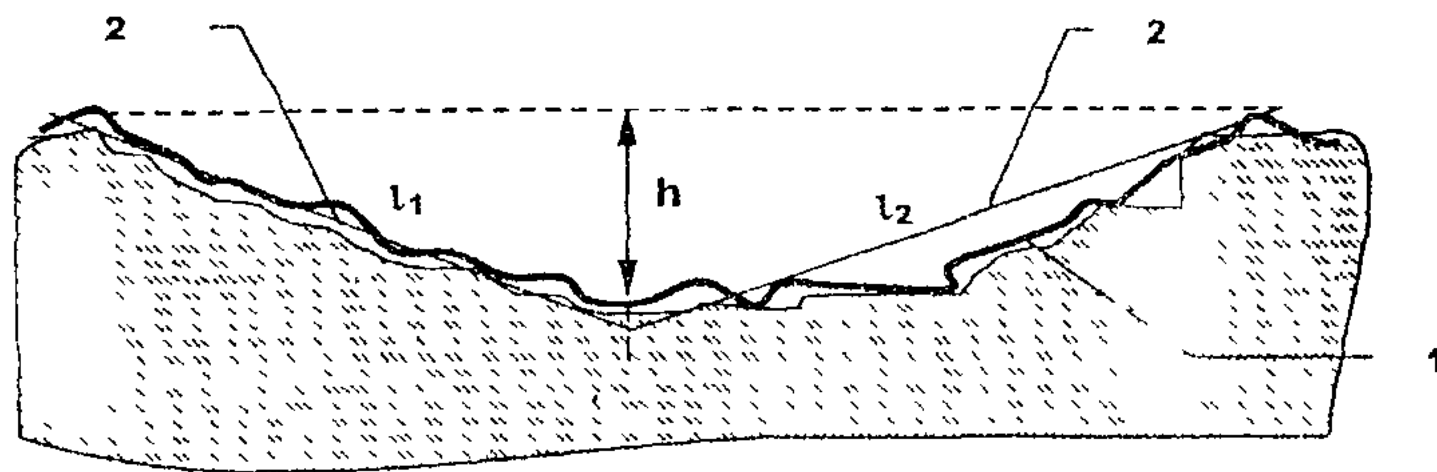
Рис. П-7.2. Схема к расположению опорной рамки для оценки колеи:
