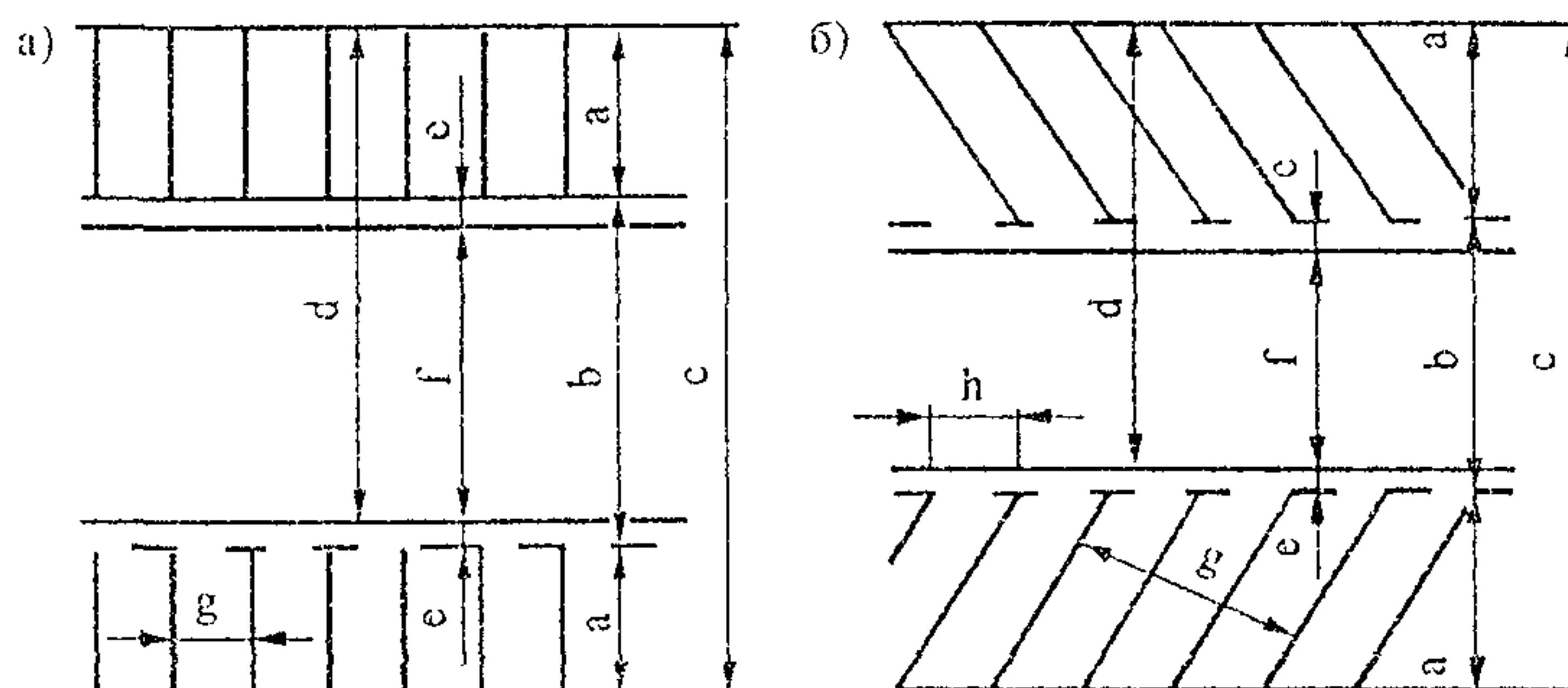
Рис. 11.7. Схемы расстановки автомобилей на стоянках: а - прямоугольная; б - косоугольная
