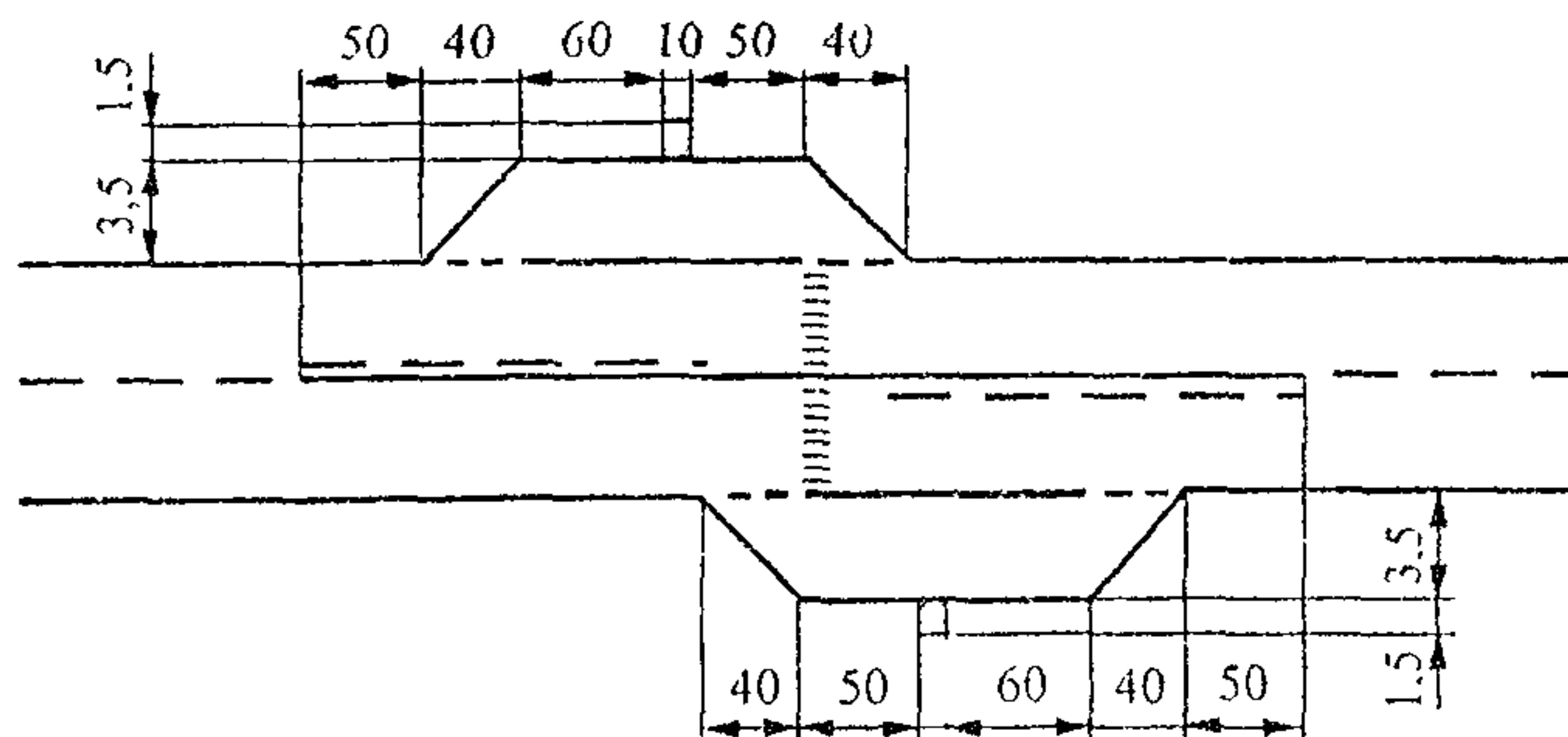
Рис. 11.9. Планировка автобусных остановок в населенных пунктах
