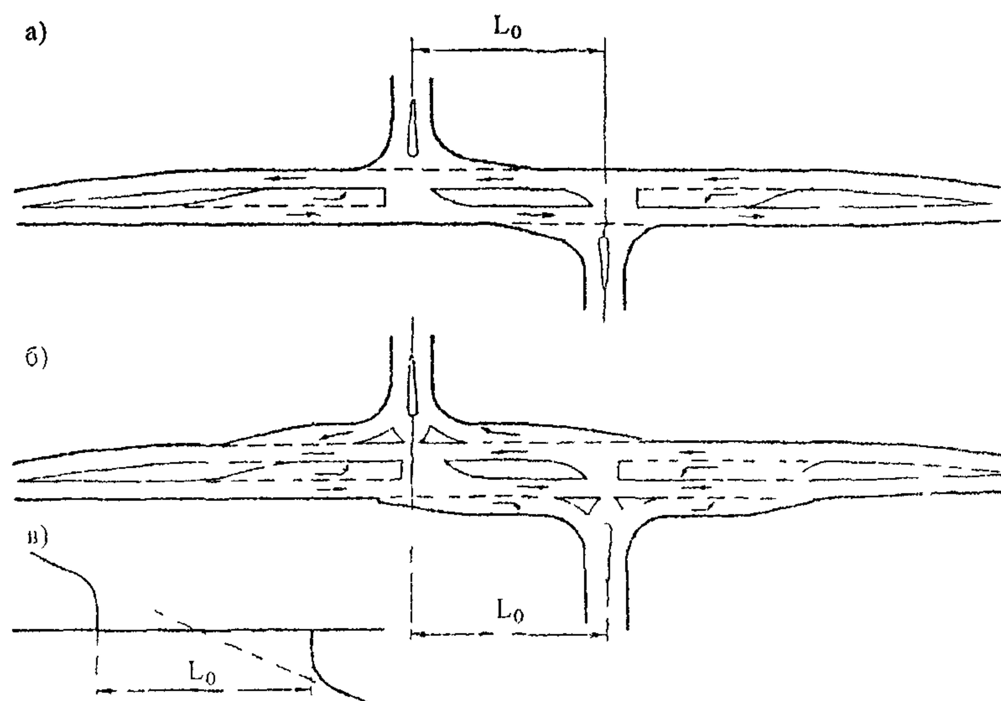
Рис. 8.6. Перестройка пересечения на два смещенных примыкания: а – без переходно-скоростных полос; б – с переходно-скоростными полосами; в – схема изменения пересечения
