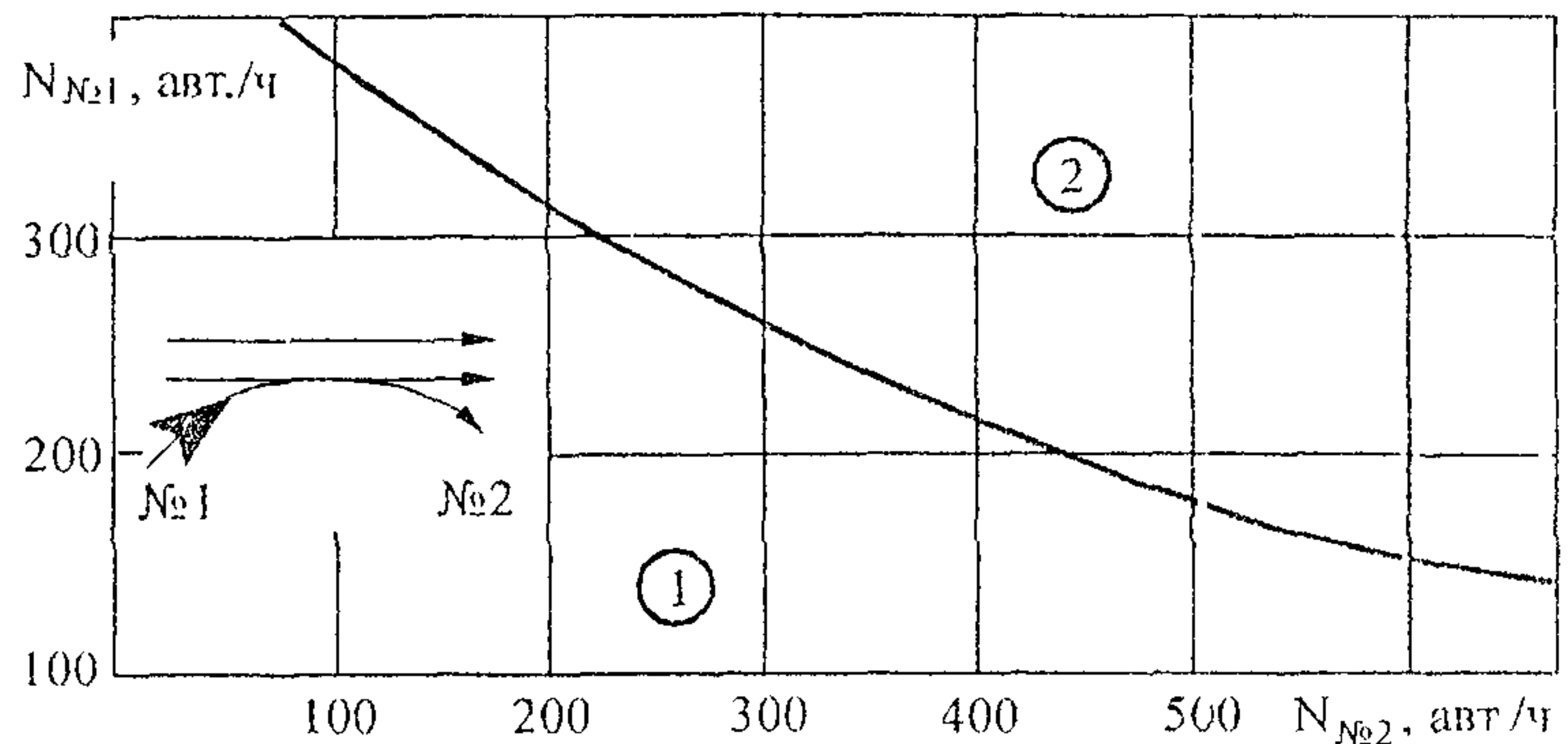
Рис. 9.3. Диаграмма применимости различных типов левоповоротных съездов:
