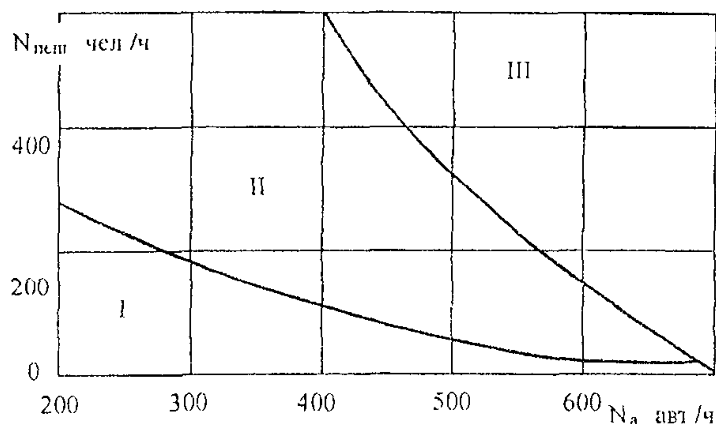
Рис. 11.2. Области применения пешеходных переходов различных типов:
