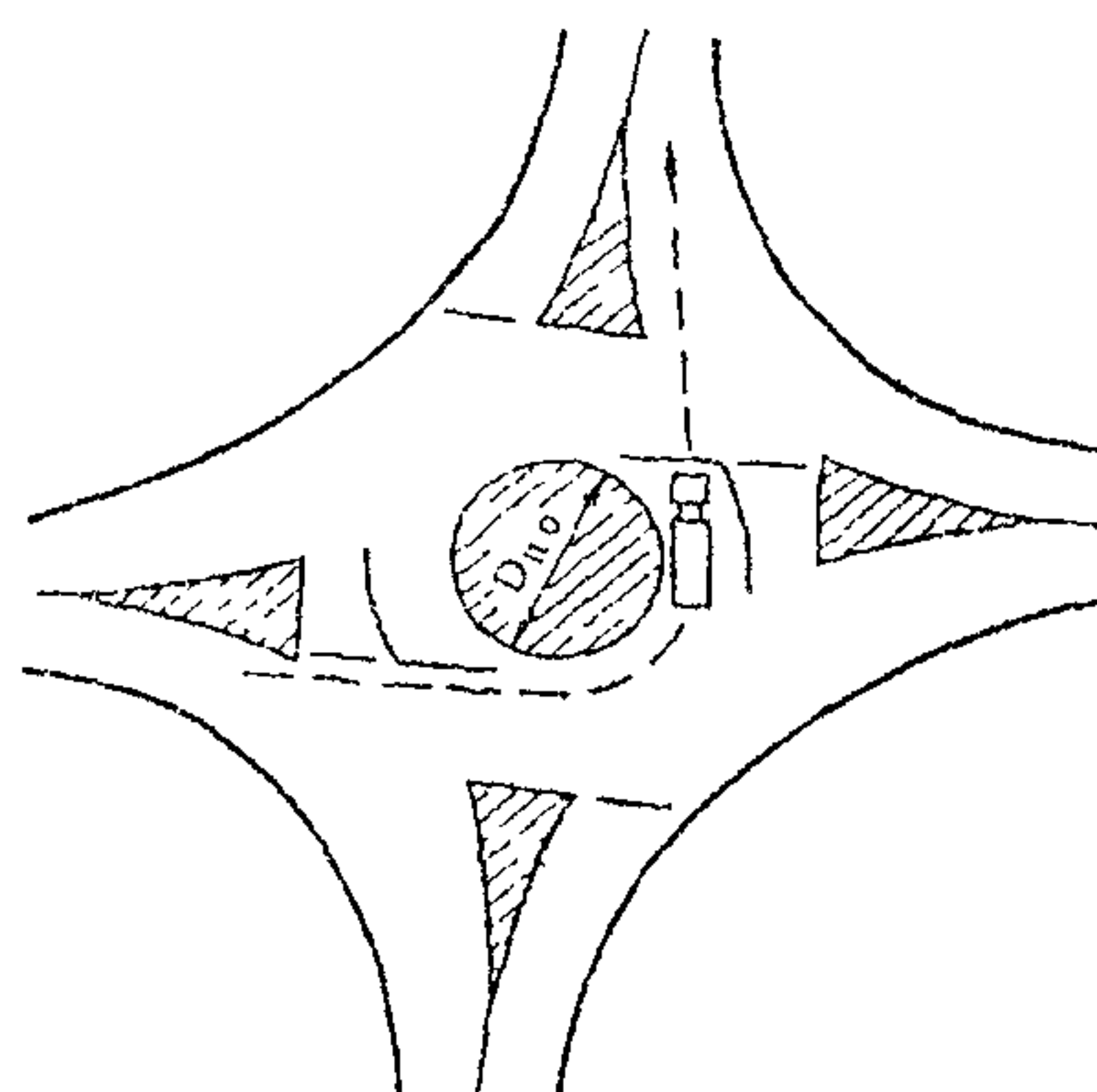
Рис. 8.17. Схема расположения автомобиля в зоне ожидания на кольцевой проезжей части
