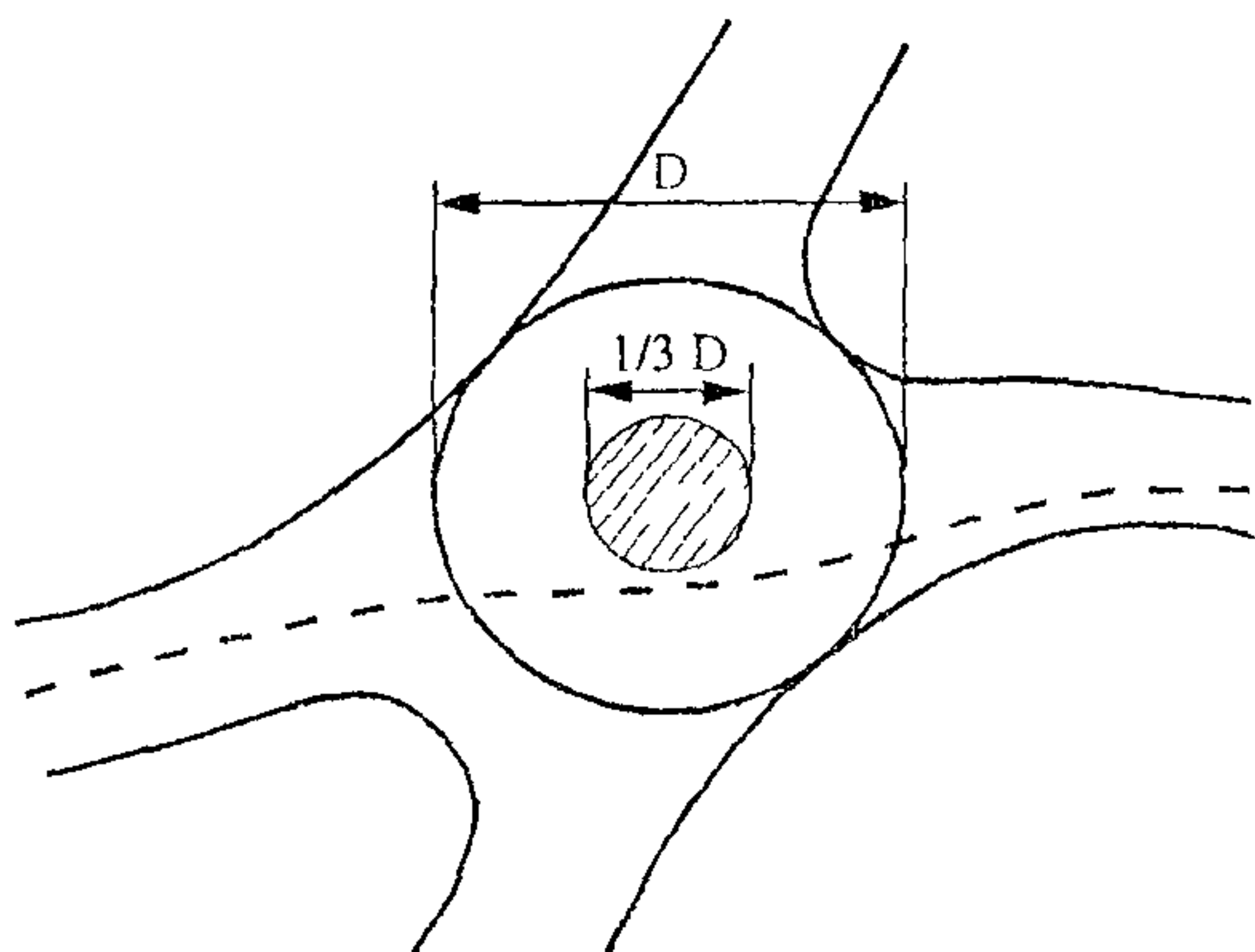
Рис. 8.15. Улучшение условий движения на пересечении путем устройства островков небольшого диаметра
