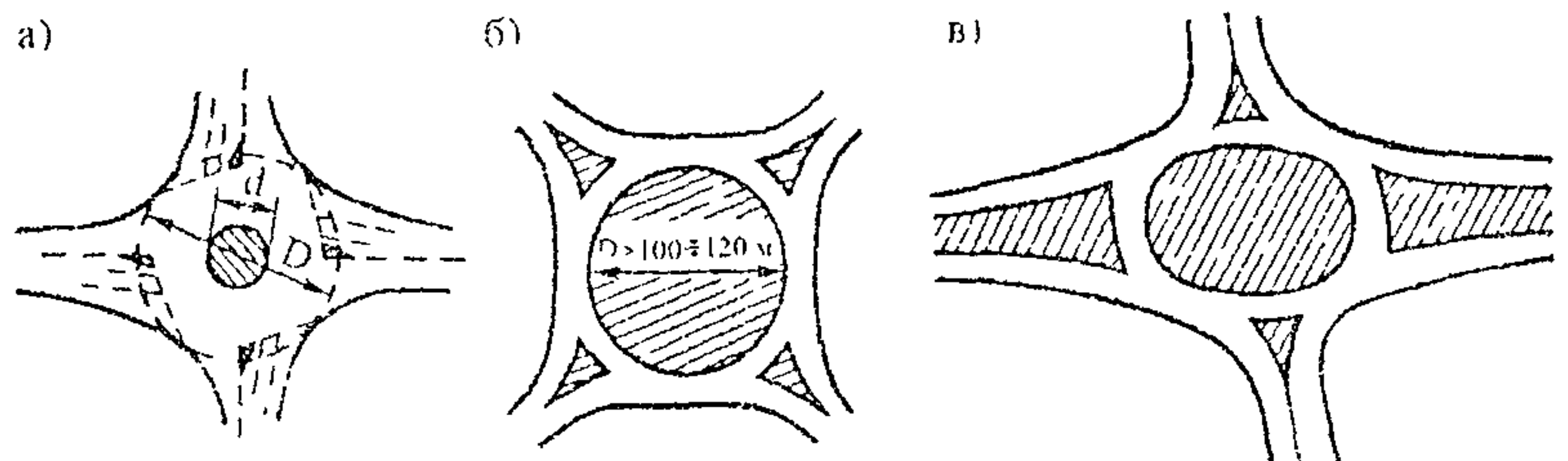
Рис. 8.14. Планировочные схемы кольцевых пересечений: а – с малым островком; б – с большим островком; в – с эллиптическим
