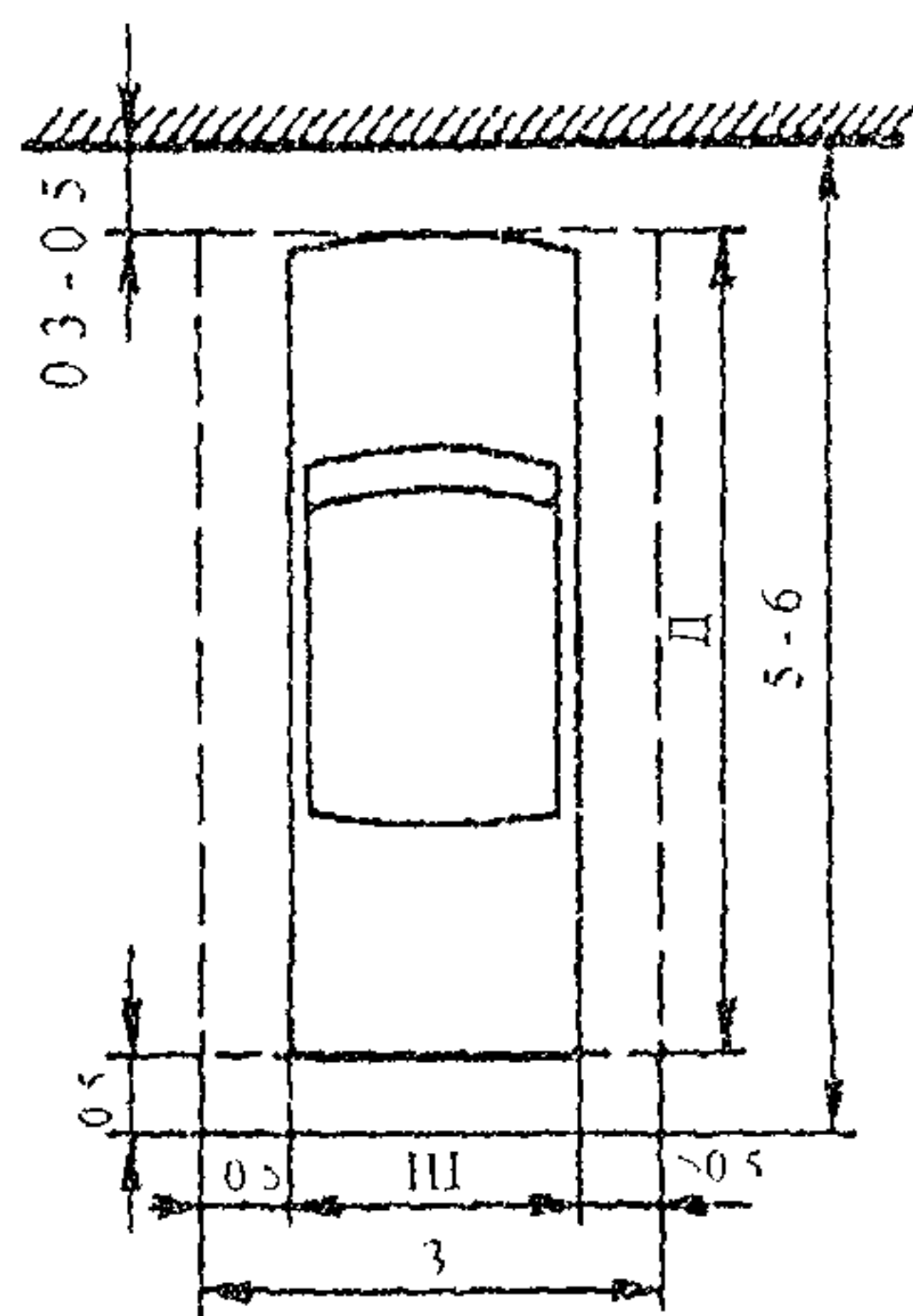
Рис. 11.4. Размеры (м) ячейки для хранения автомобиля на стоянках: Д и Ш - габаритные длина и ширина расчетного автомобиля, соответственно
