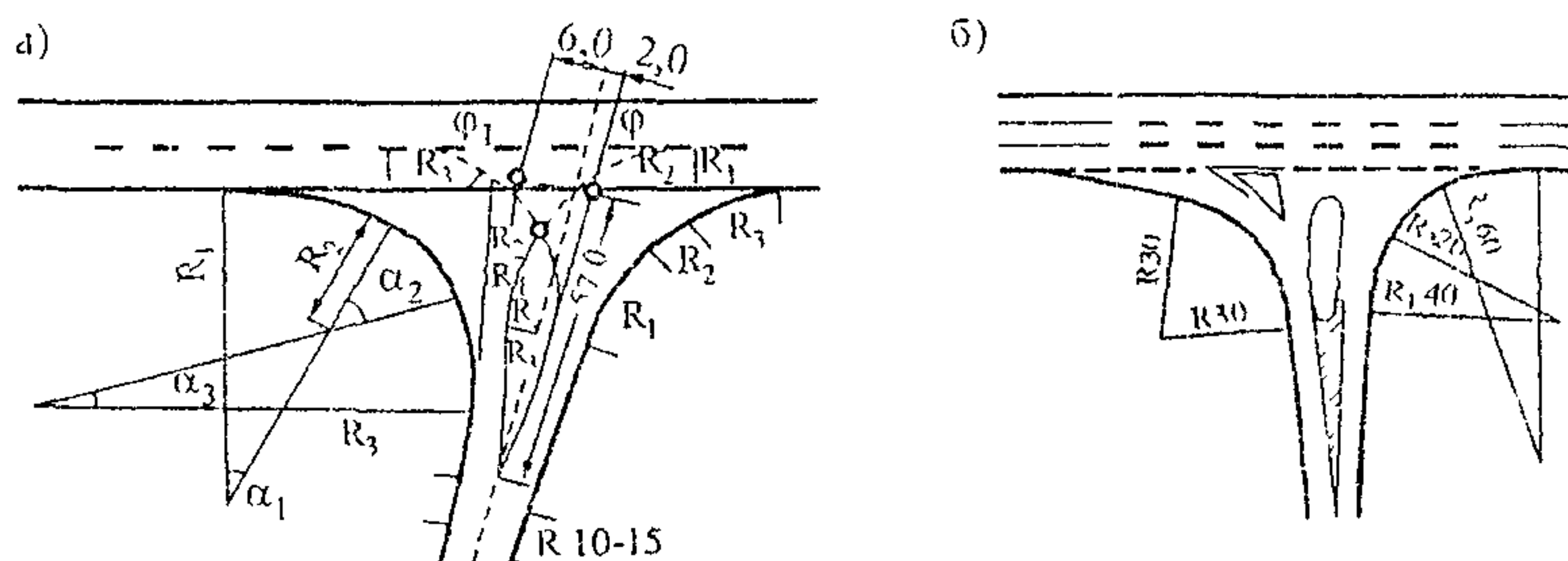
Рис. 8.10. Расположение островков на второстепенной дороге: а – схема размещения островка; б – выделение островка разметкой
