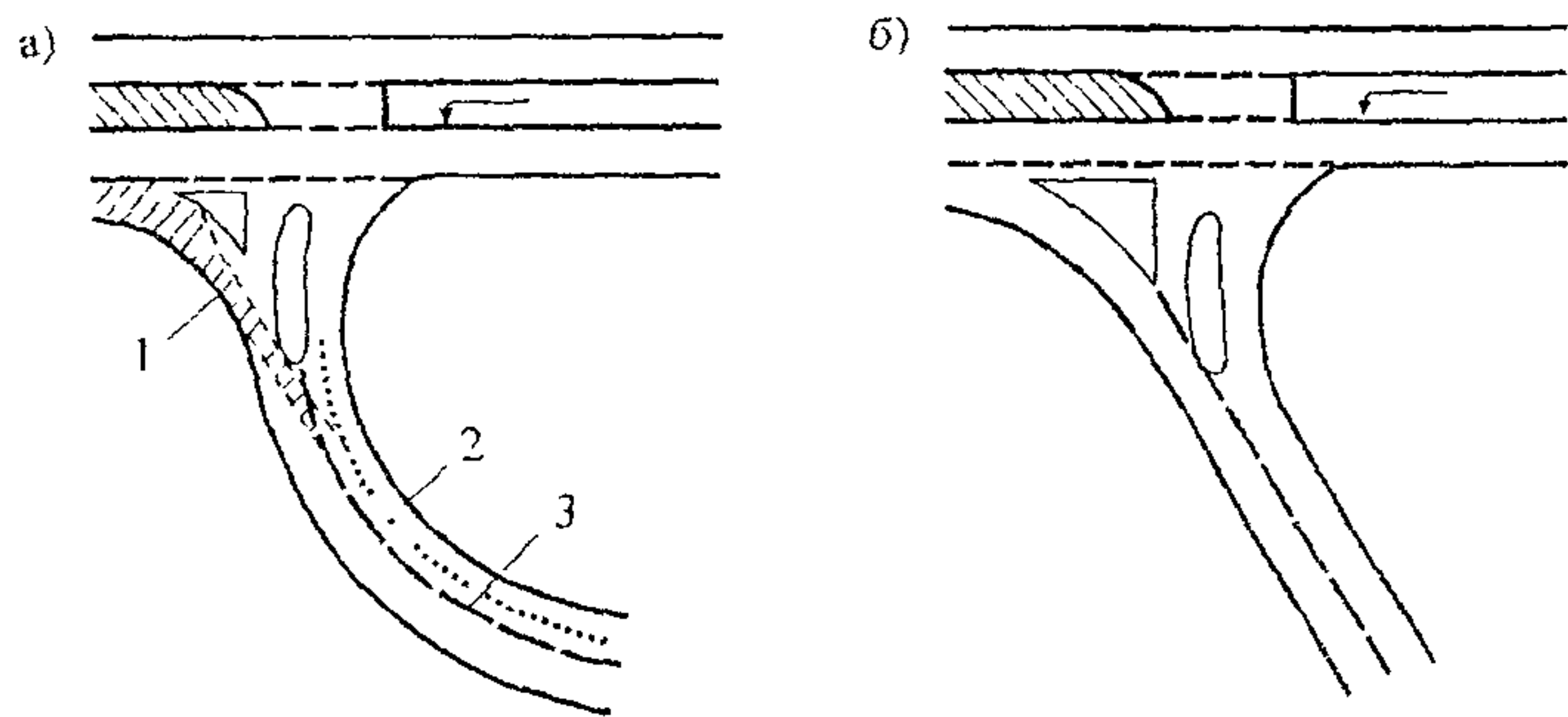
Рис. 8.7. Зрительное перекрытие островками неправильного направления движения:
