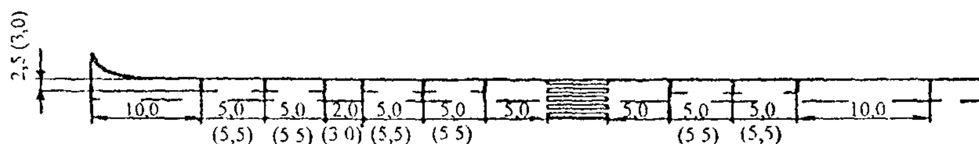
Рис. 11.5. Размещение стоянок вдоль тротуара на проезжей части улицы (размеры, м)
