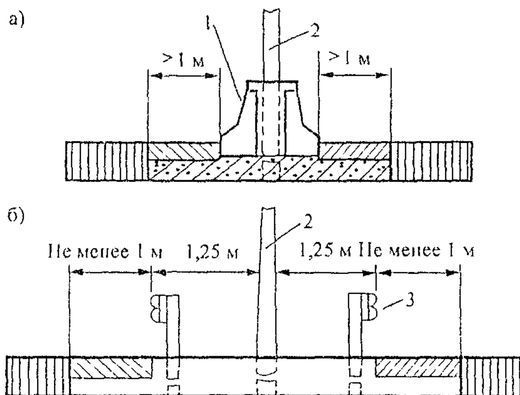
Рис. 15.1. Схема заделки в грунт опор освещения: а – при благоприятных условиях; б – в пучинистых грунтах; в – при наличии подземных коммуникаций; 1 – опора; 2 – оголовок; 3 – свая; 4 – деревянный короб; 5 – бетонный фундамент; 6 – металлический Г-образный фундамент
