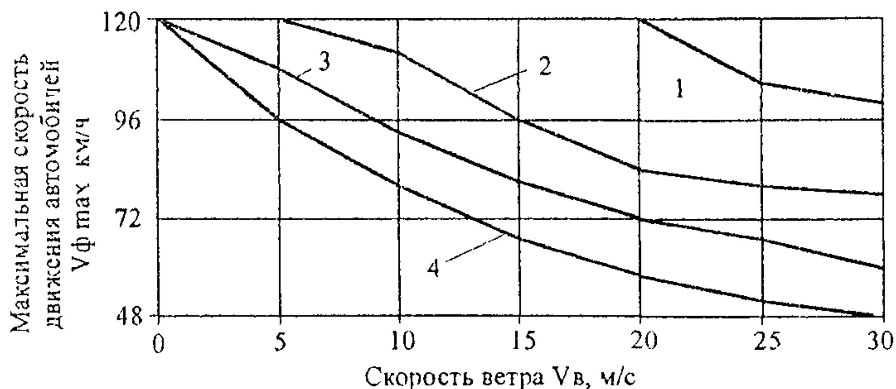
Рис. 1.3. Зависимости максимальной безопасной скорости движения автомобилей от скорости ветра:
