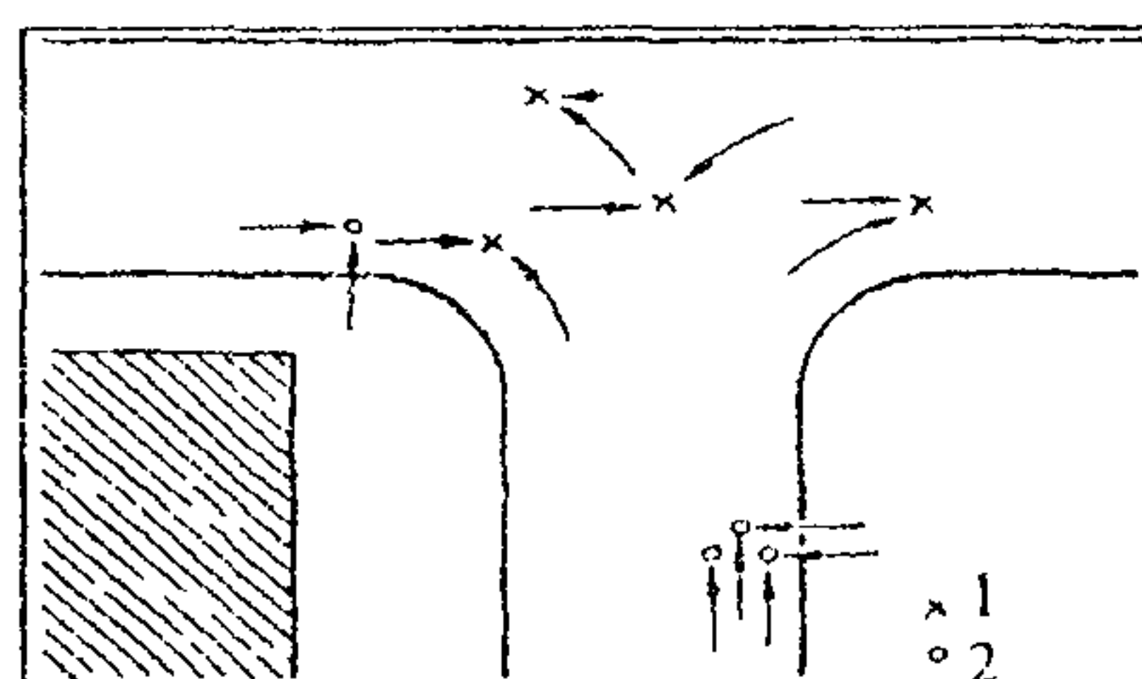
Рис. 8.9. План пересечения с нанесенными на него схемами дорожно-транспортных происшествий: 1 – столкновение транспортных средств; 2 – наезд на пешеходов
