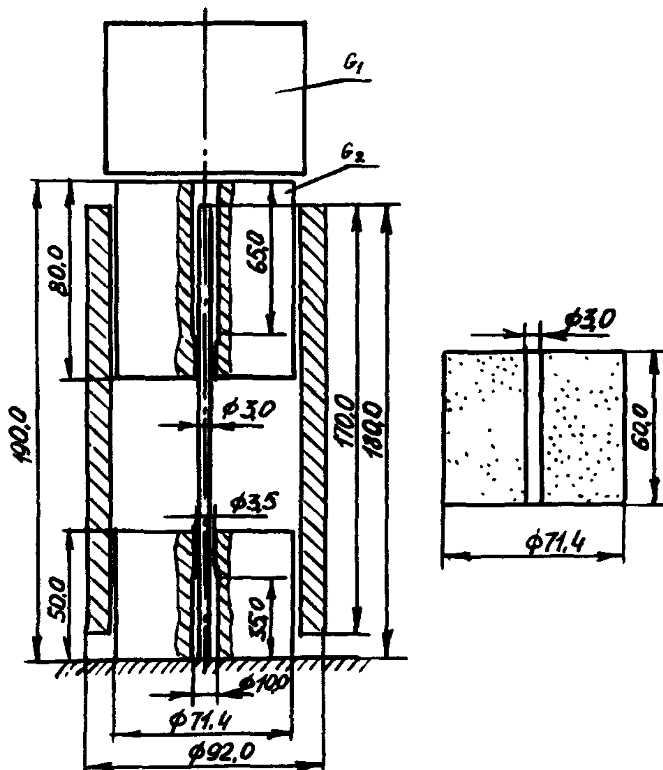
Рис.1. Приспособление для уплотнения образцов
