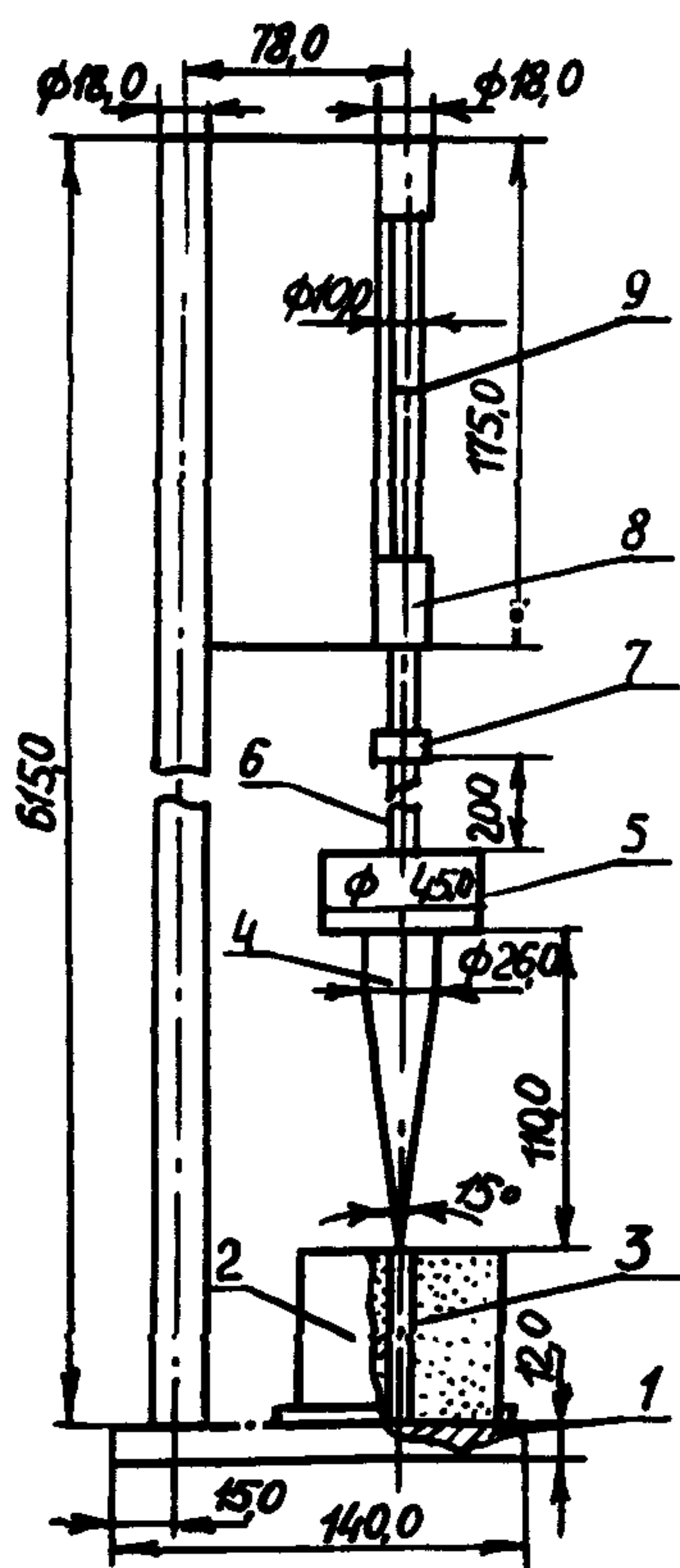
Рис.2. Прибор для определения показателя условной когезии:
