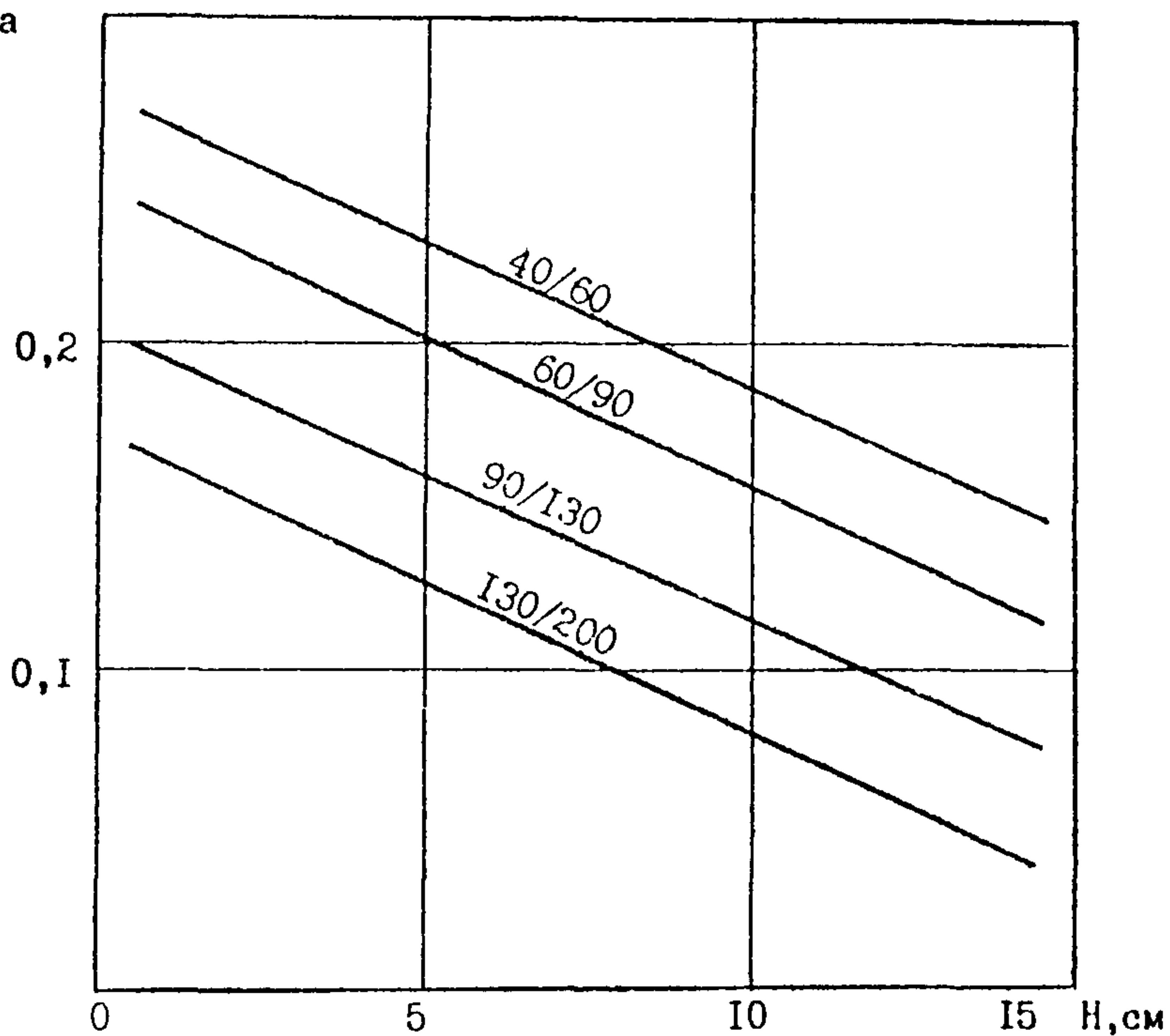
Рис. 2.2. Номограмма для определения напряжений в асфальтобетонных покрытиях на рези-нобитумных вяжущих от перемещения блока основания
