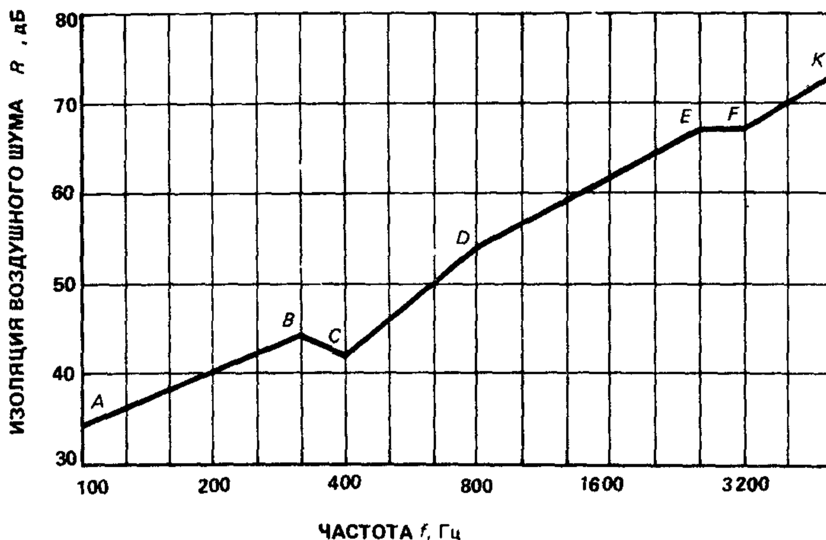
Рис. 2. Расчетная частотная характеристика
