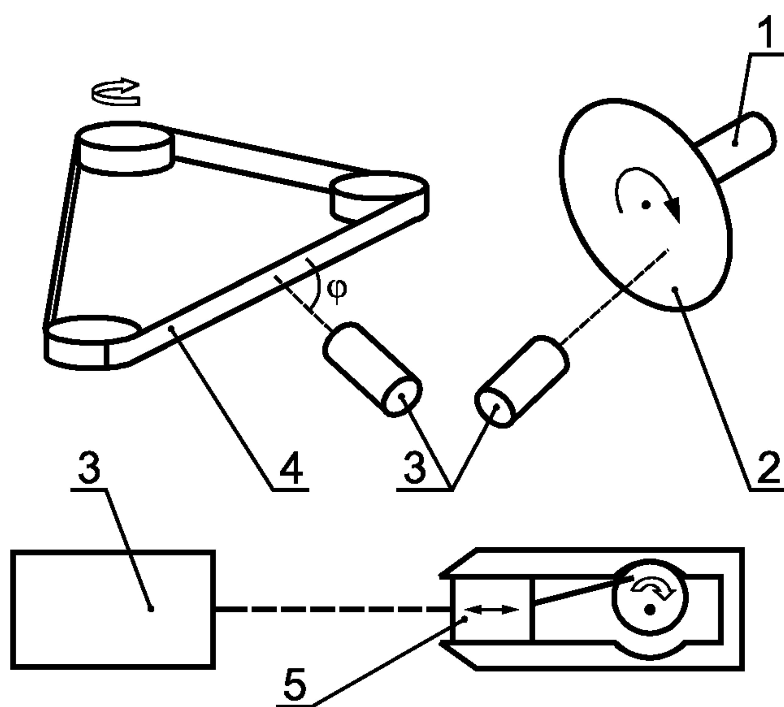
1 — двигатель; 2 — диск; 3 — датчики; 4 — лента; 5 — поршень
