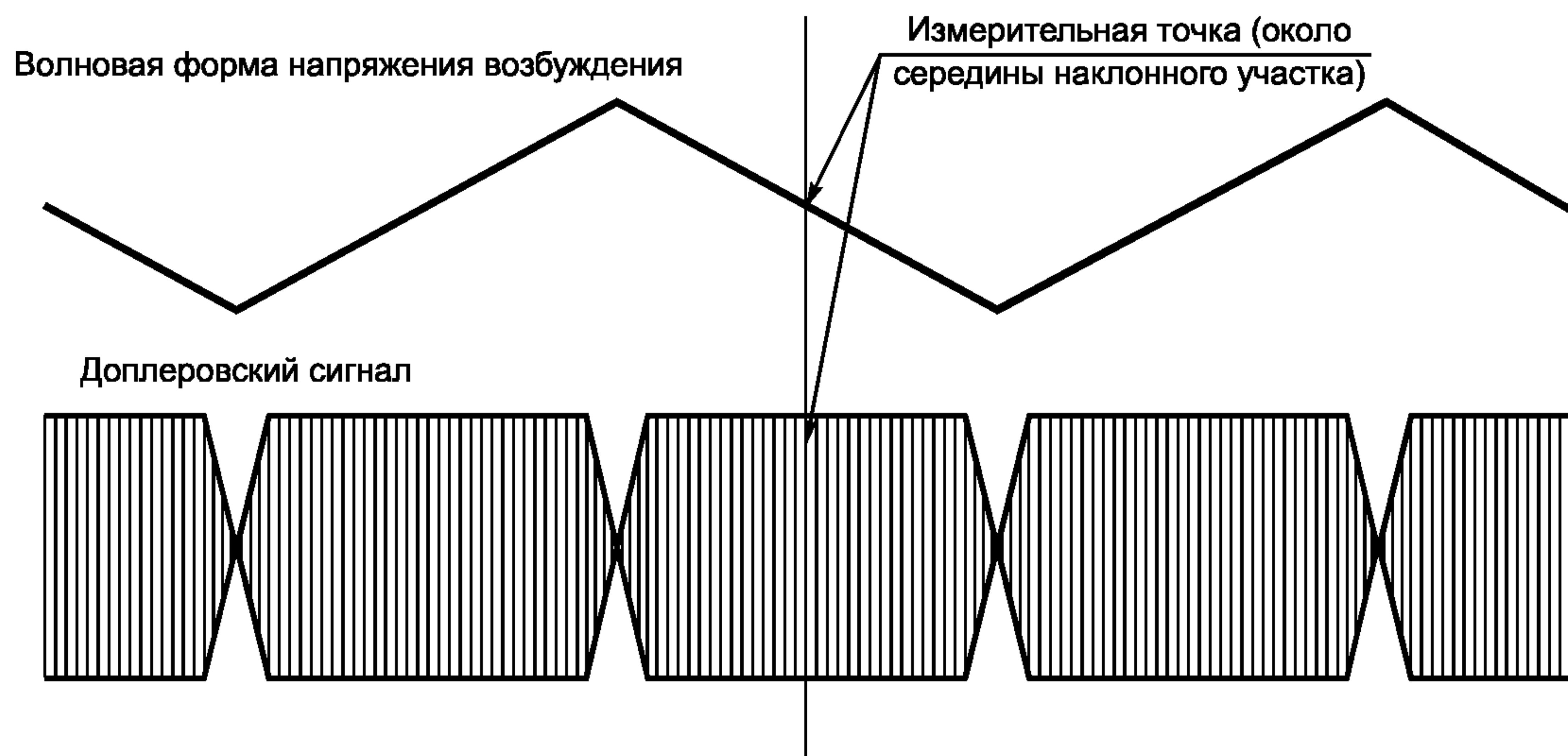
Рисунок 4 — Точка отсчета для определения уровня сигнала при пилообразной форме напряжения на генераторе привода мишени
