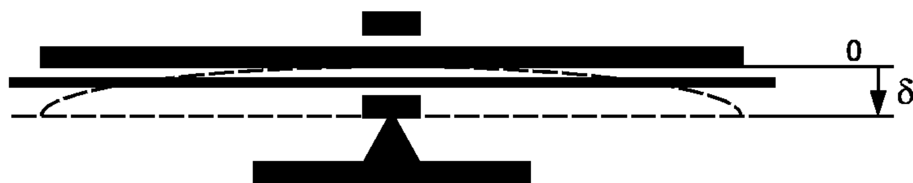
Рисунок 1 — Схема испытания модельных образцов гипсовых повязок прямоугольной формы по консольному бесконтактному методу
