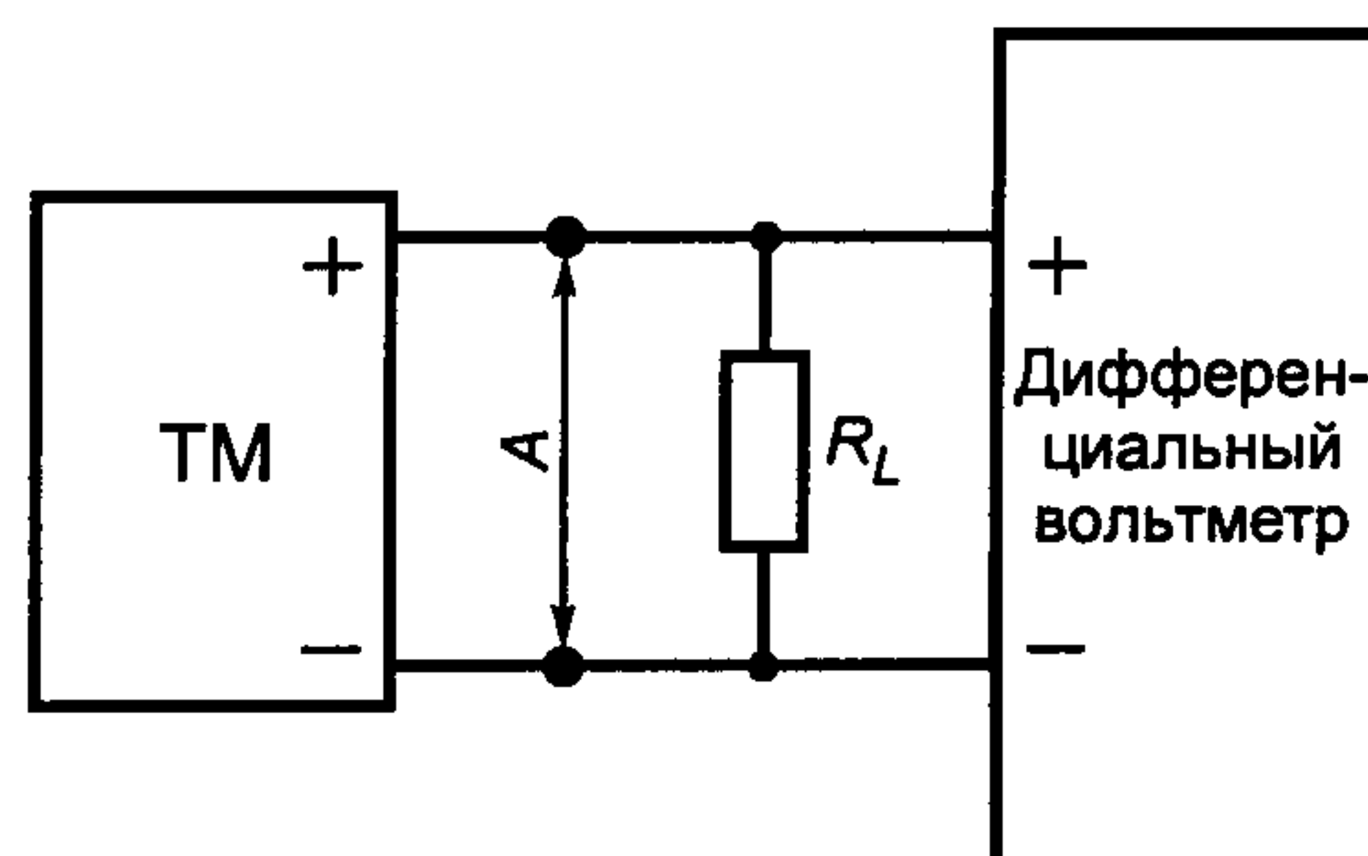
Рисунок 5 — Схема измерения выходного шума ТМ
