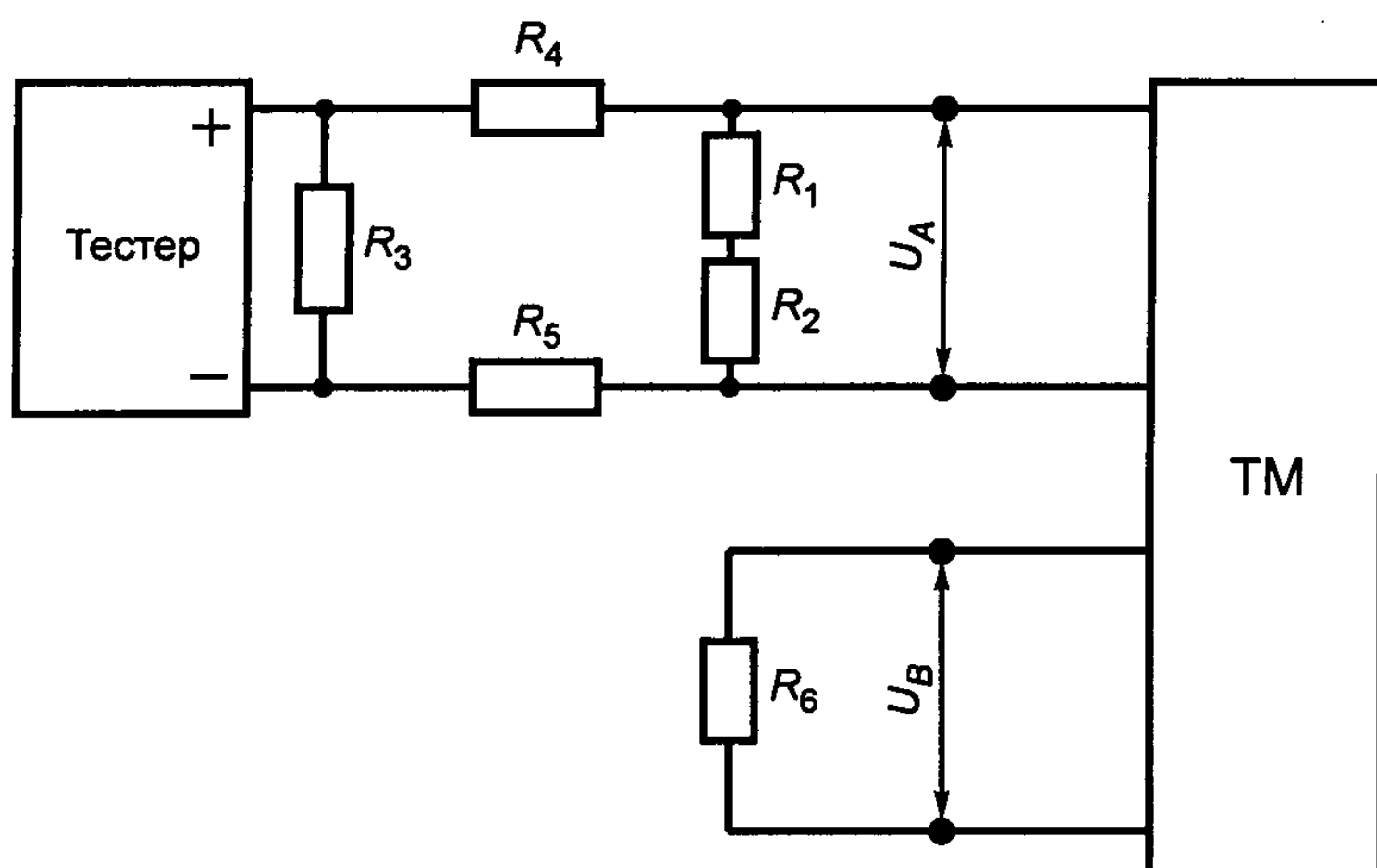
Рисунок 6 — Схема измерения взаимного влияния магистральных шин
