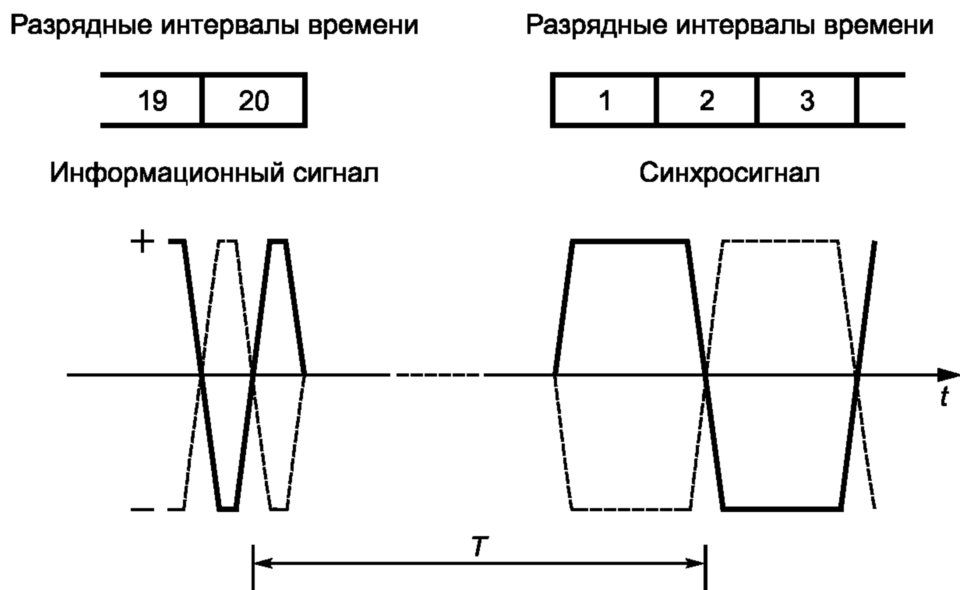
Рисунок 9 — Измерение временных пауз при передаче информации
