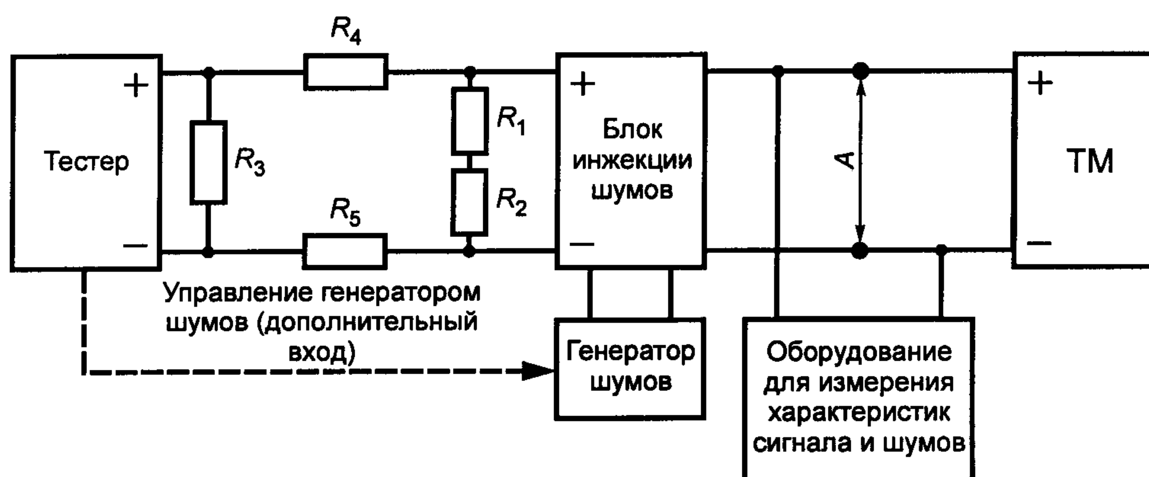
Рисунок 11 — Схема тестирования устойчивости к помехам ТМ
