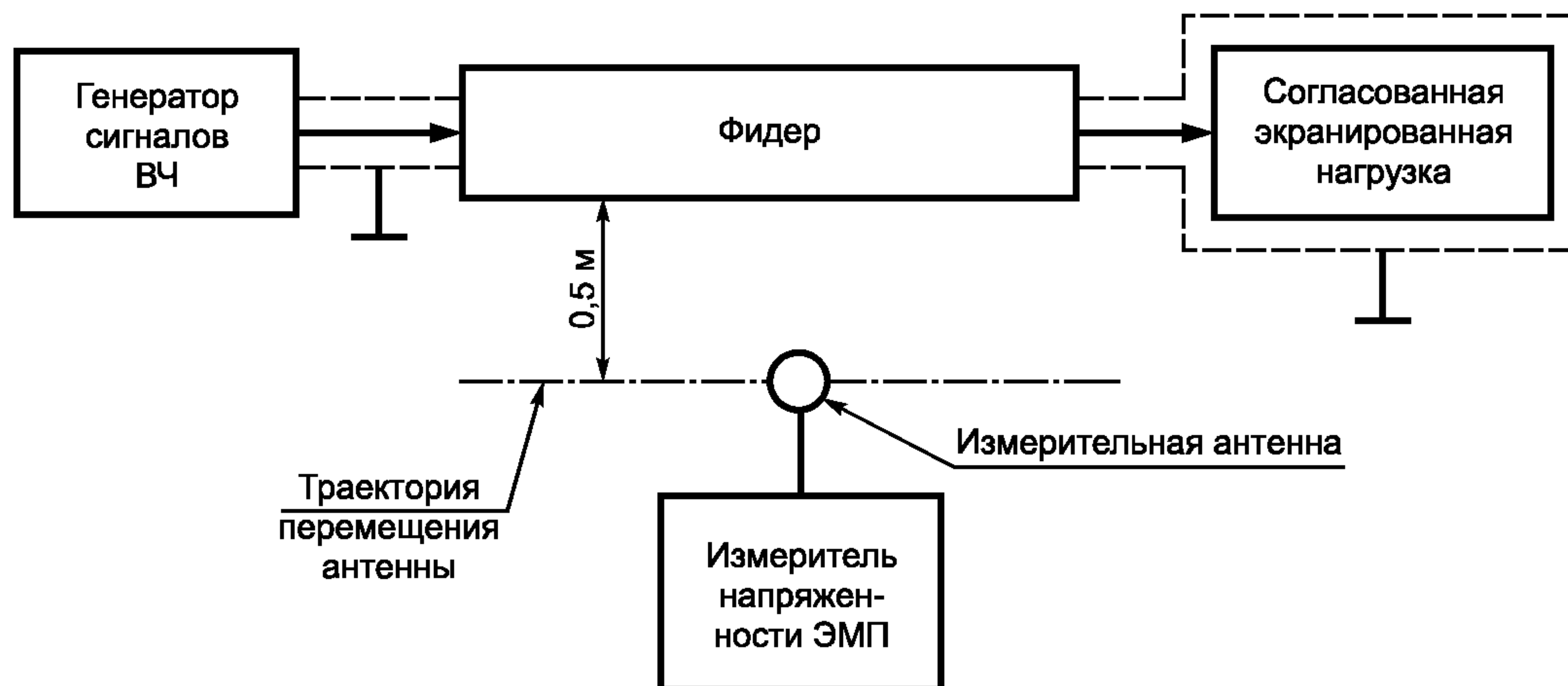
Рисунок 2 — Схема расположения оборудования при измерении напряженности ЭМП
