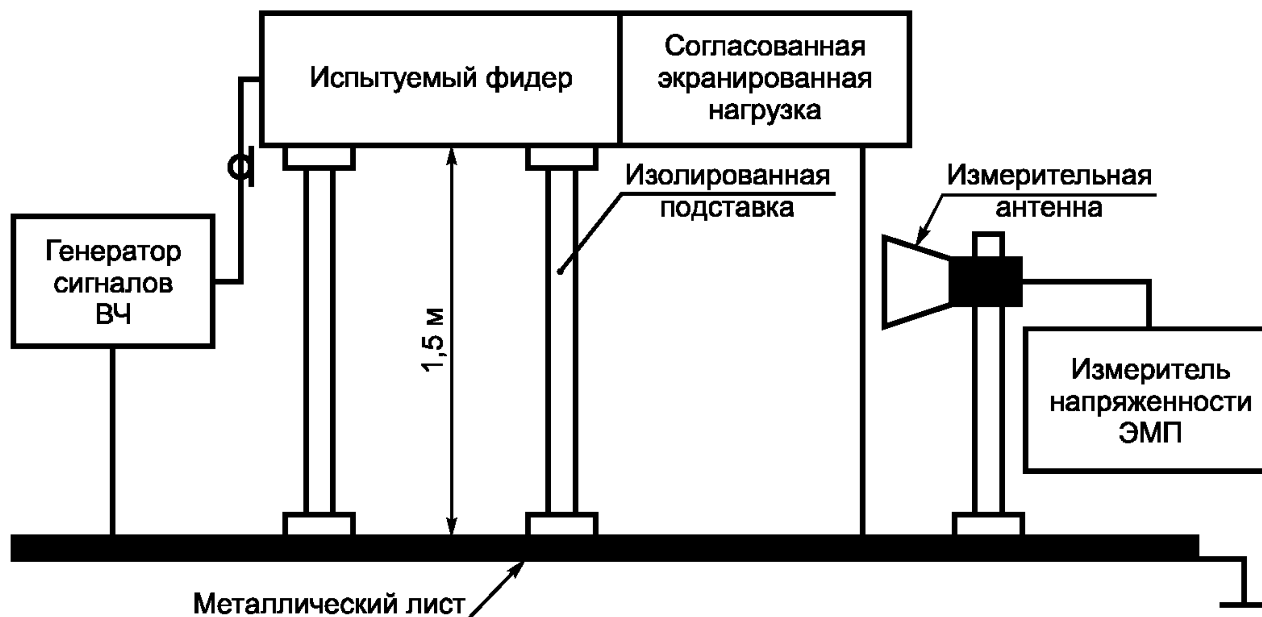
Рисунок Г.1 — Расположение оборудования на испытательной площадке
