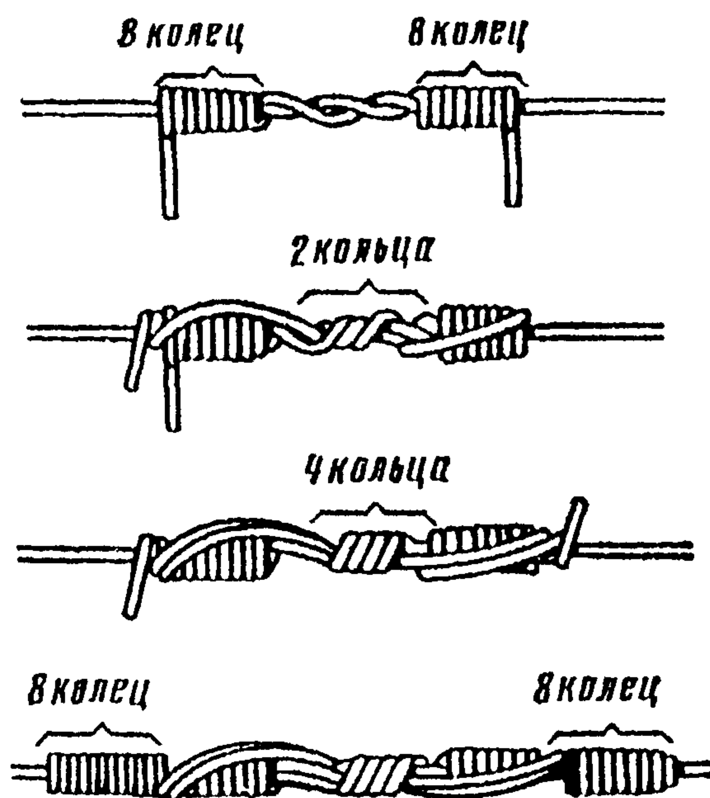
Рис. 3.7. . Скрутка проводов
