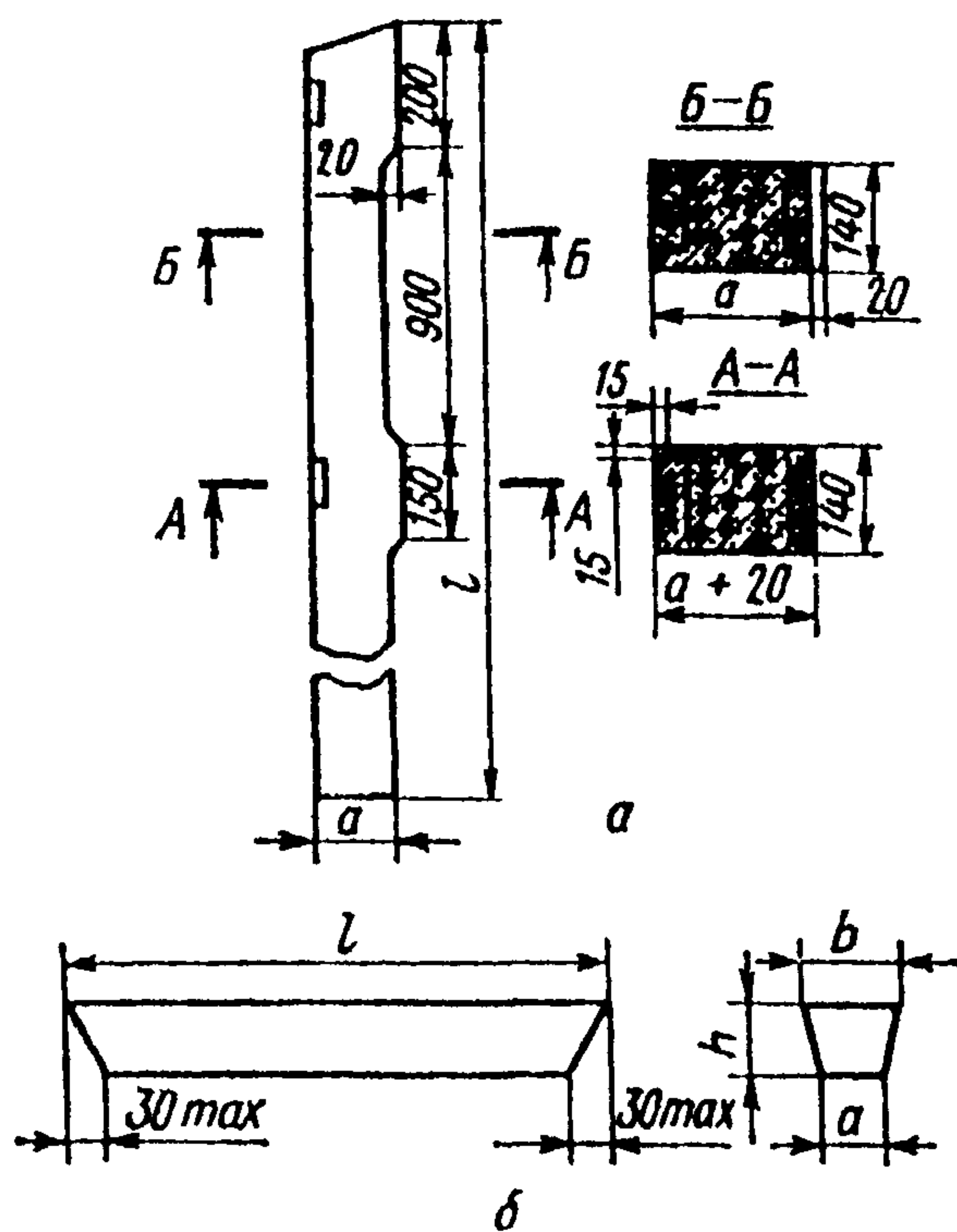
Рис. 2.2. Приставки железобетонные: a — типа ПР; б — типа ПТ
