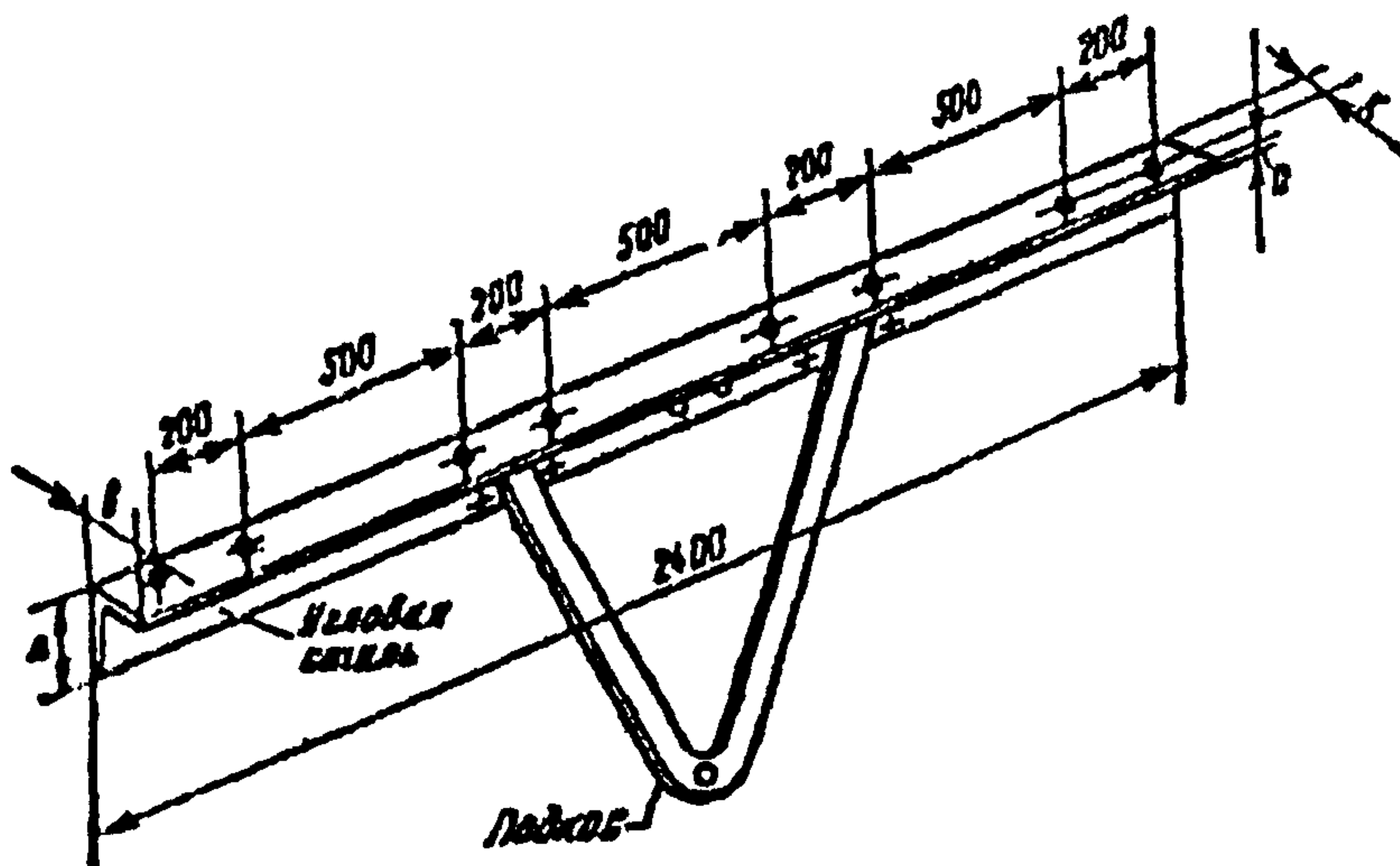
Рис. 2.9. Стальная телефонная усиленная траверса СТС
