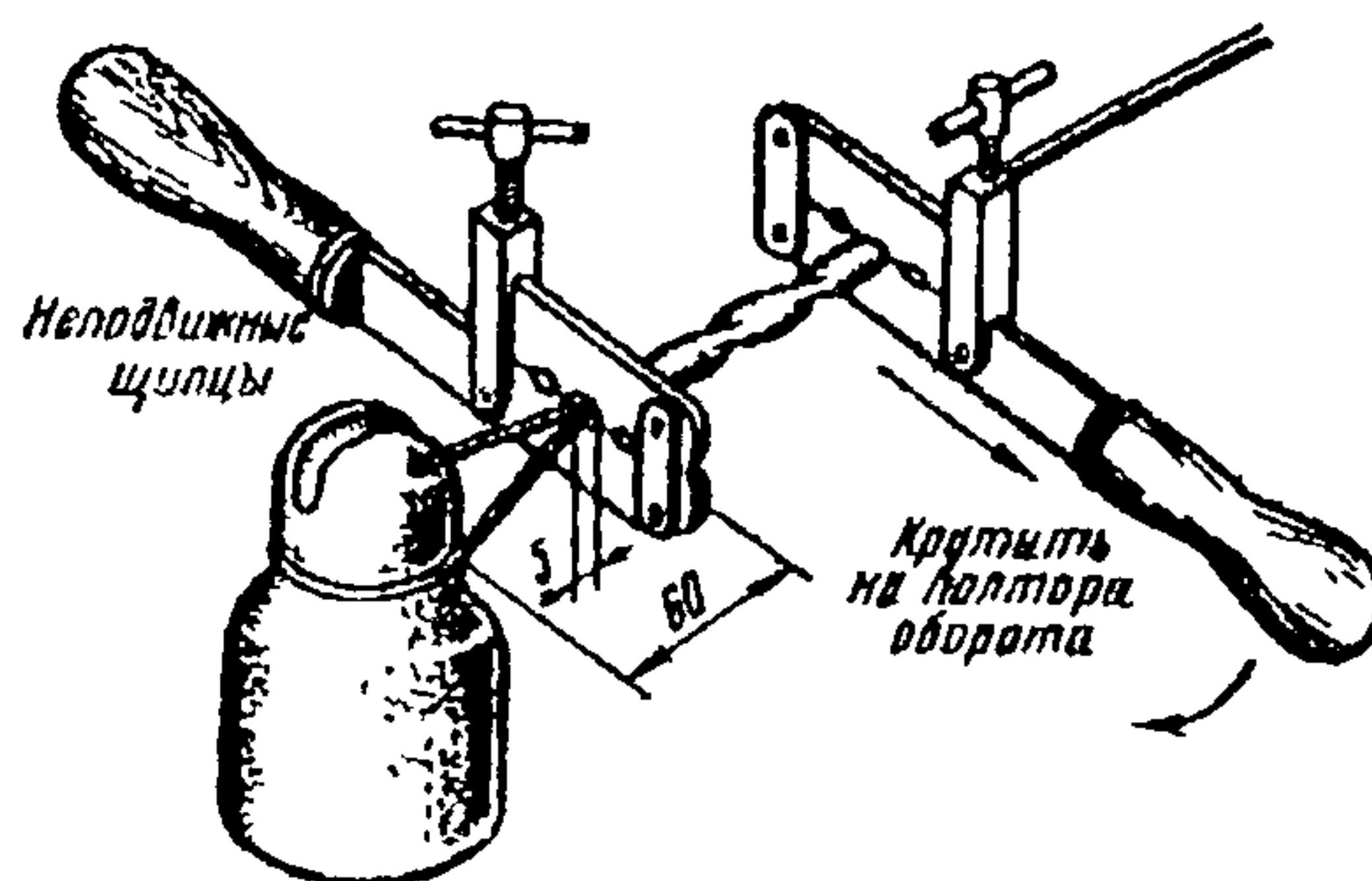
Рис. 3.14. Оконечная заделка провода из цветного металла
