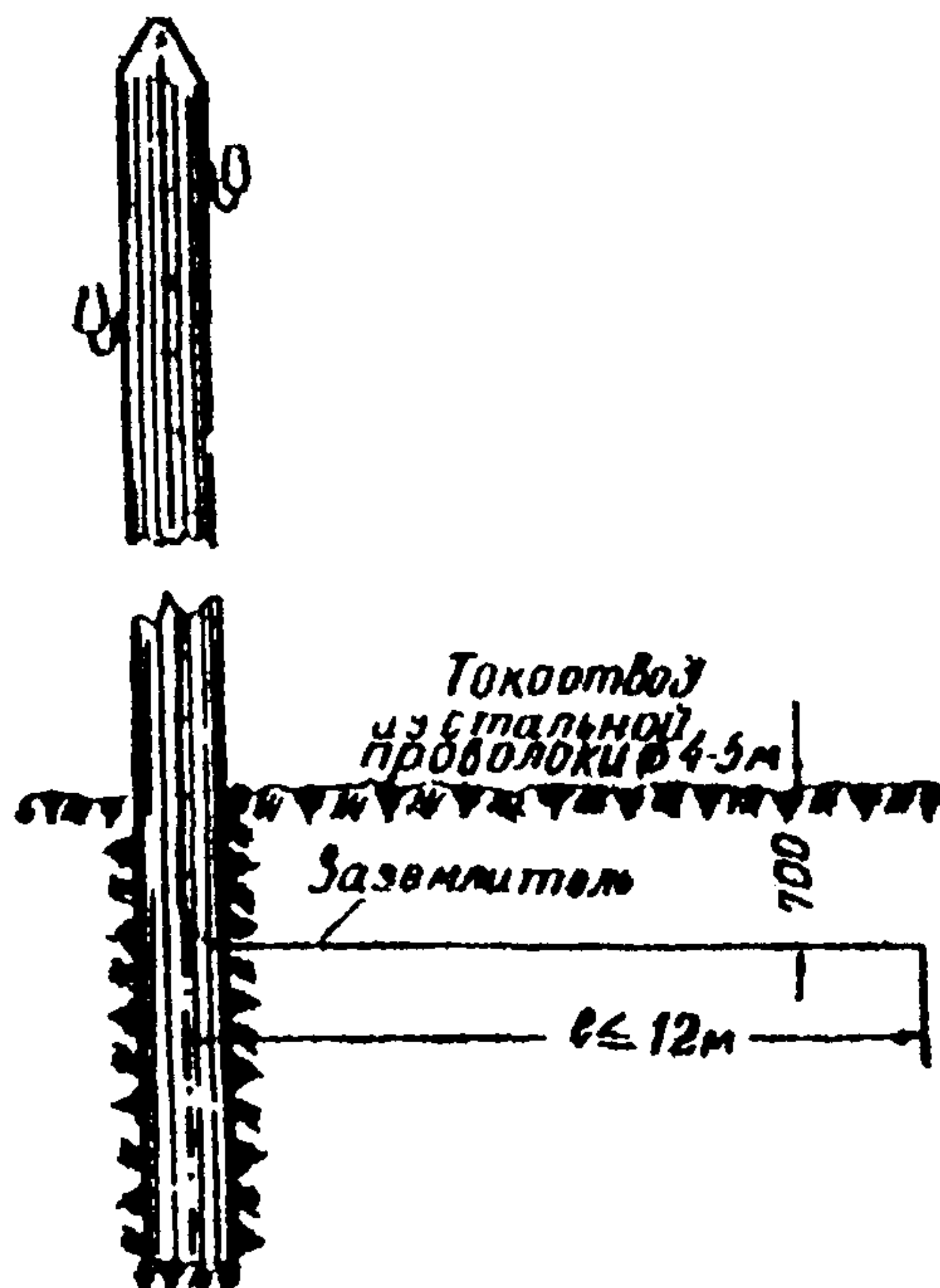
Рис. 3.20. Протяженный винтовой заземнитель
