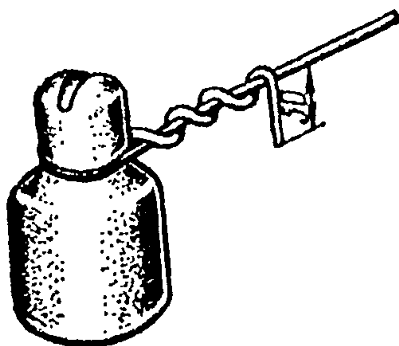
Рис. 3.13. Оконечная заделка провода малого диаметра скруткой
