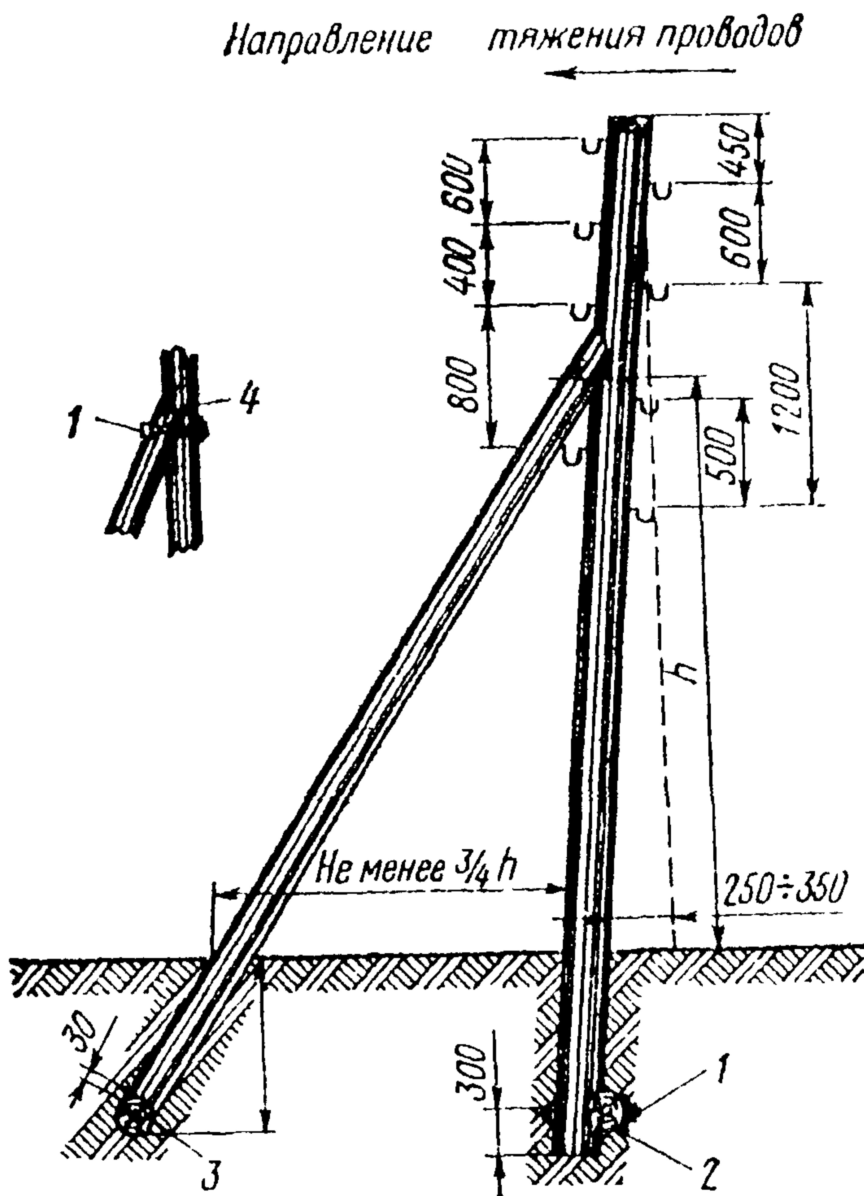
Рис. 3.5. Угловая опора, укрепленная подпорой:
