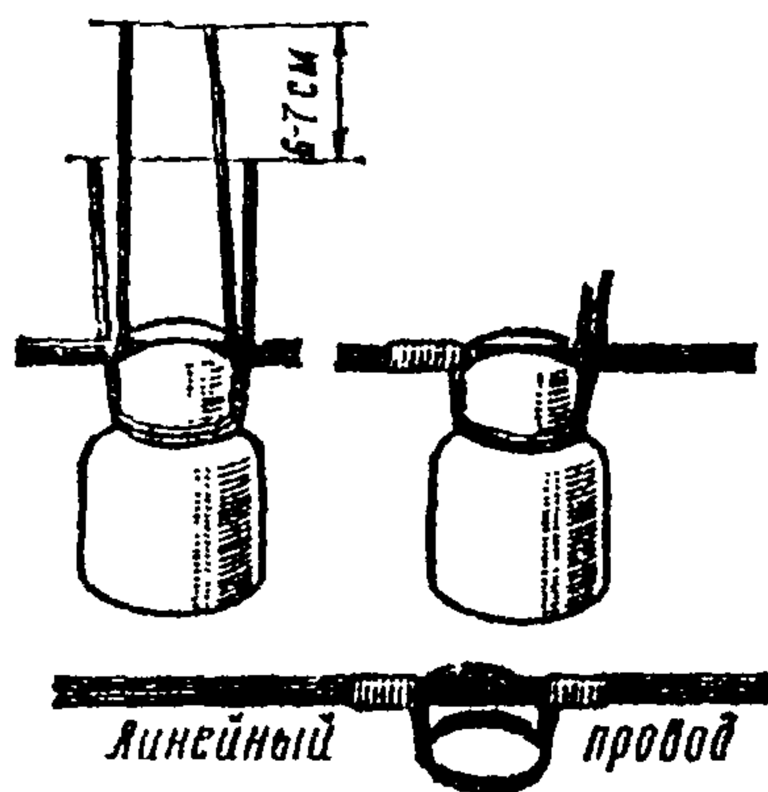
Рис. 3.10. Крепление провода к изолятору на прямой линии
