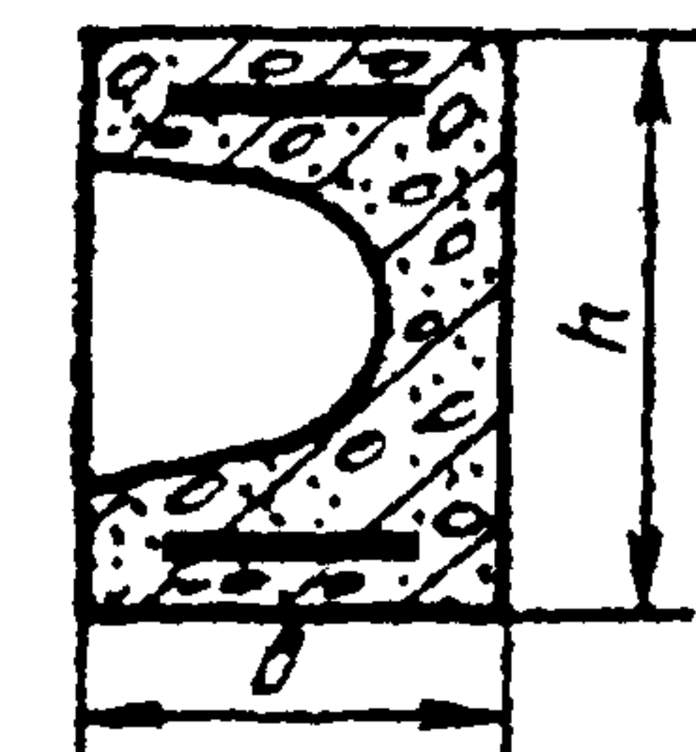
Сечение по 1-1
