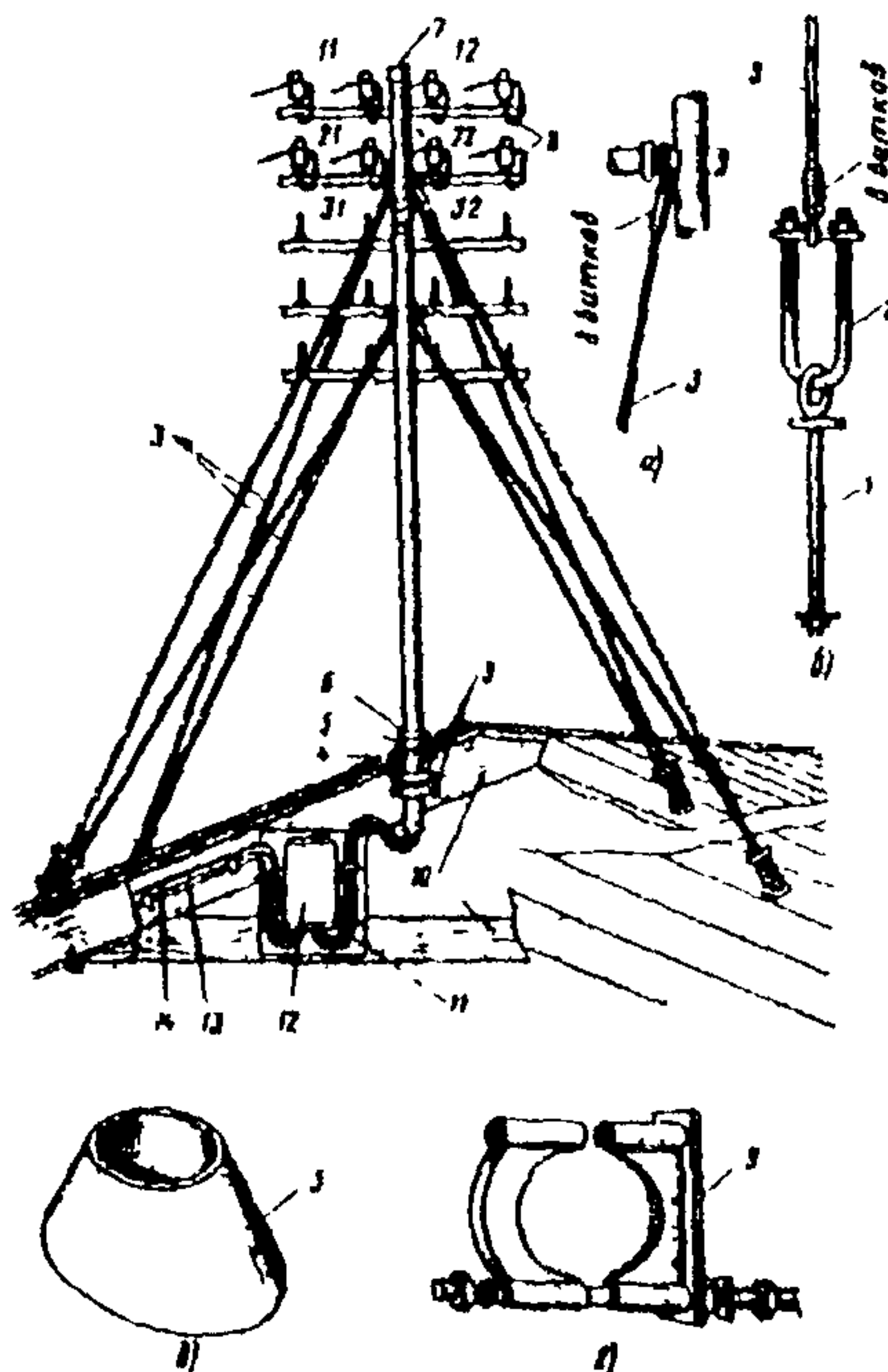
Рис. 2.10. Установка стойки 10×2 и детали ее крепления:
