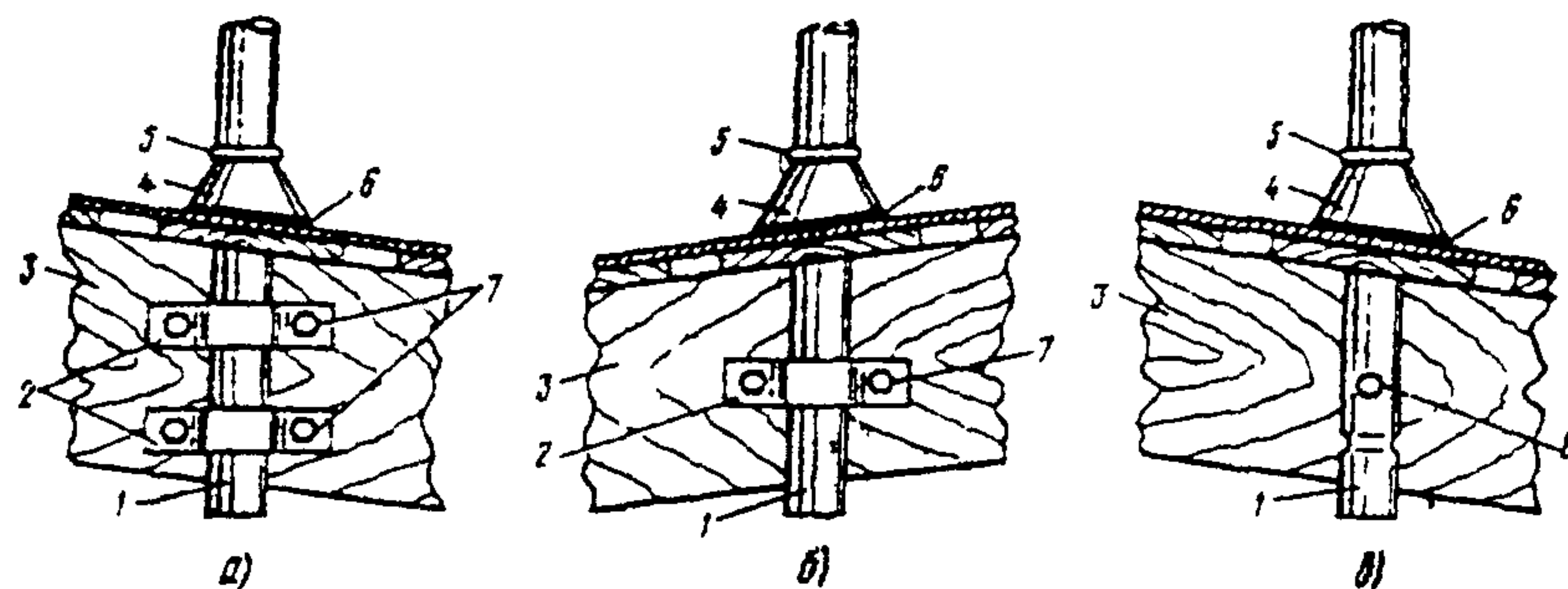
Рис.3.22. Крепление стоек
