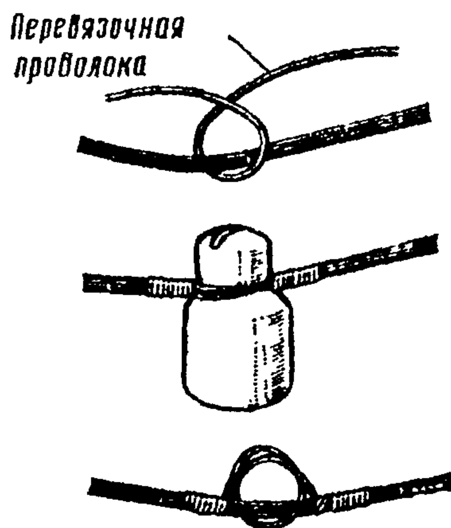
Рис. 3.11. Крепление провода к изолятору на угловой опоре
