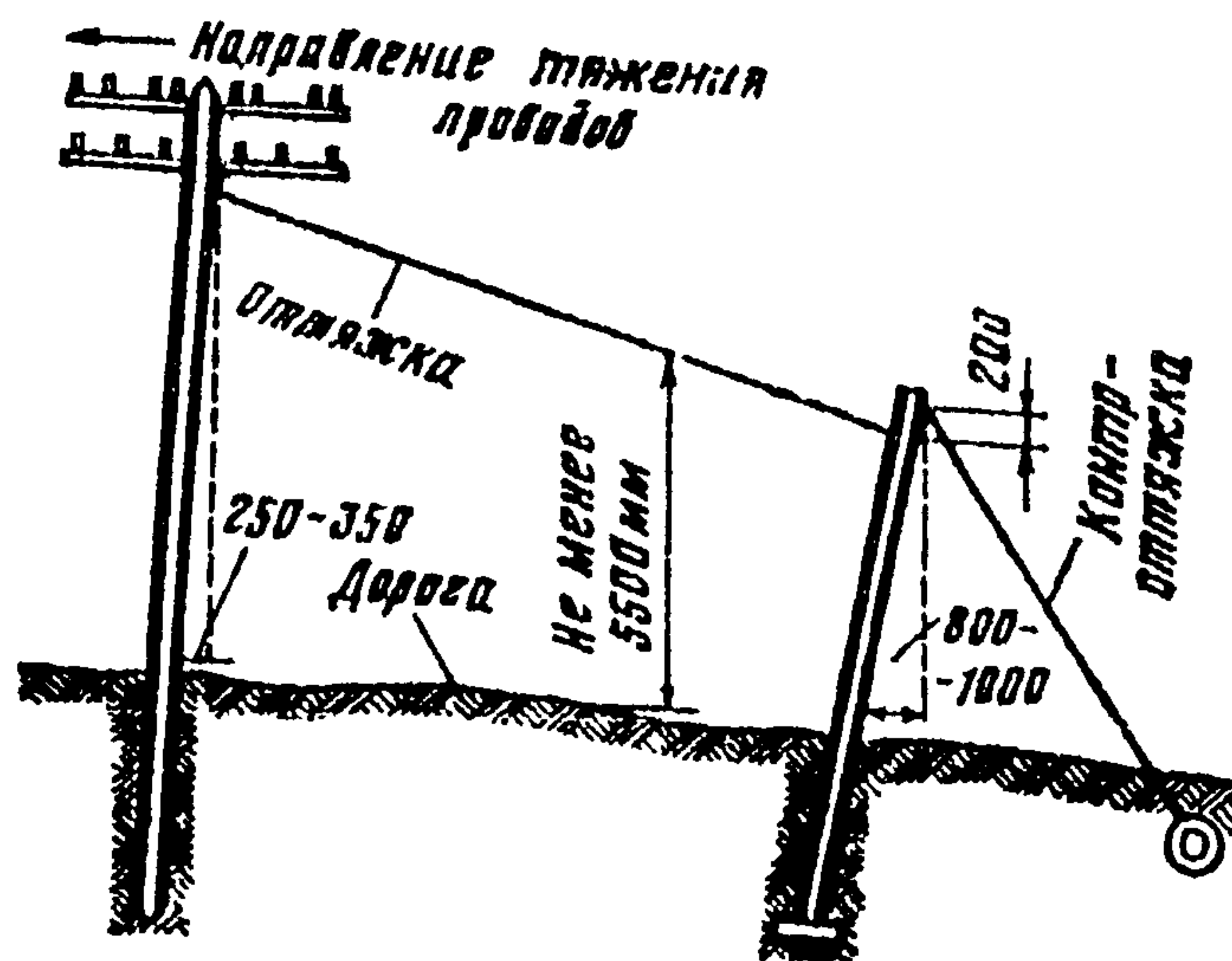
Рис. 3.6. Устройство оттяжного столба
