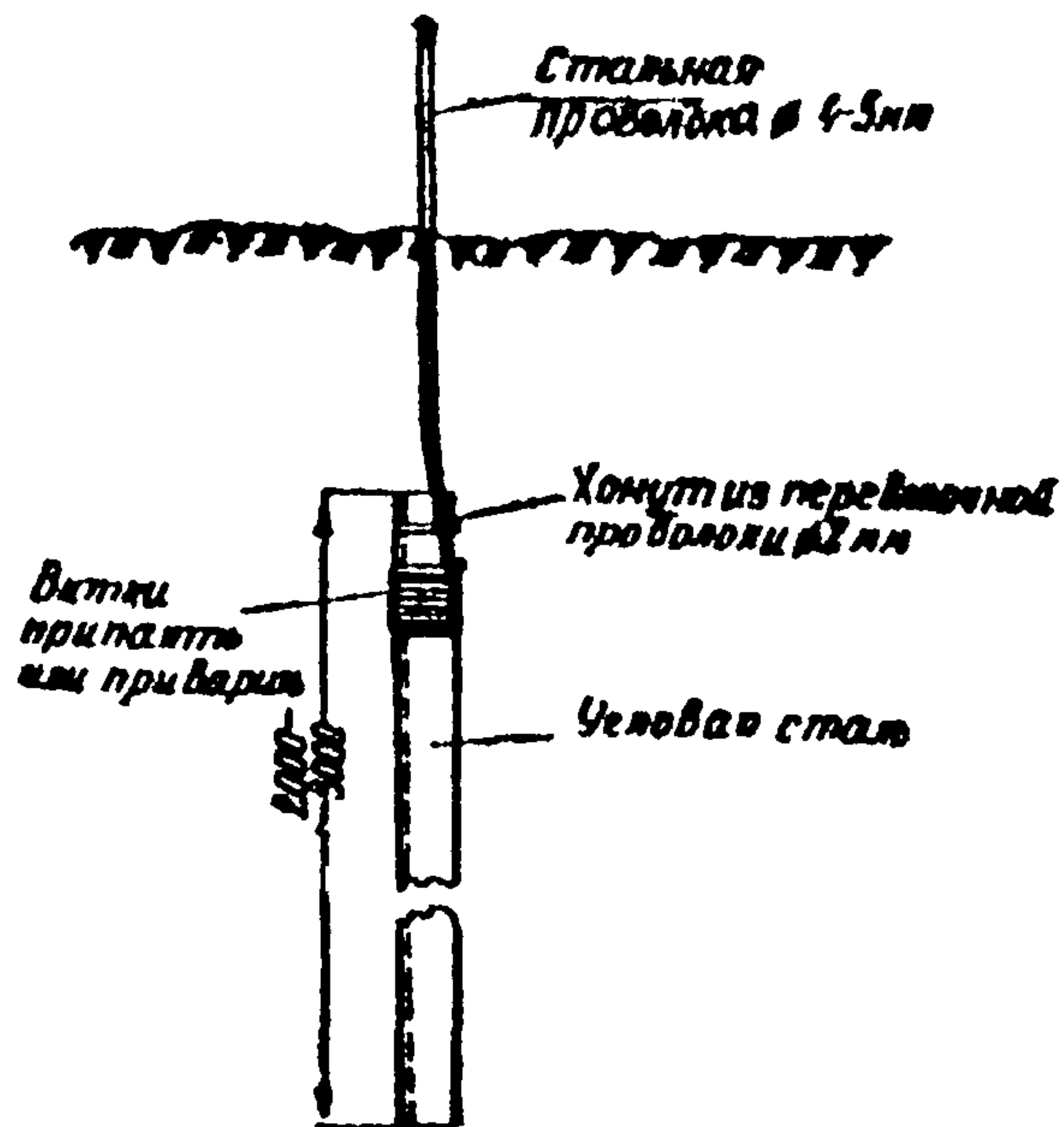
Рис. 3.21. Заземнитель из угловой стали
