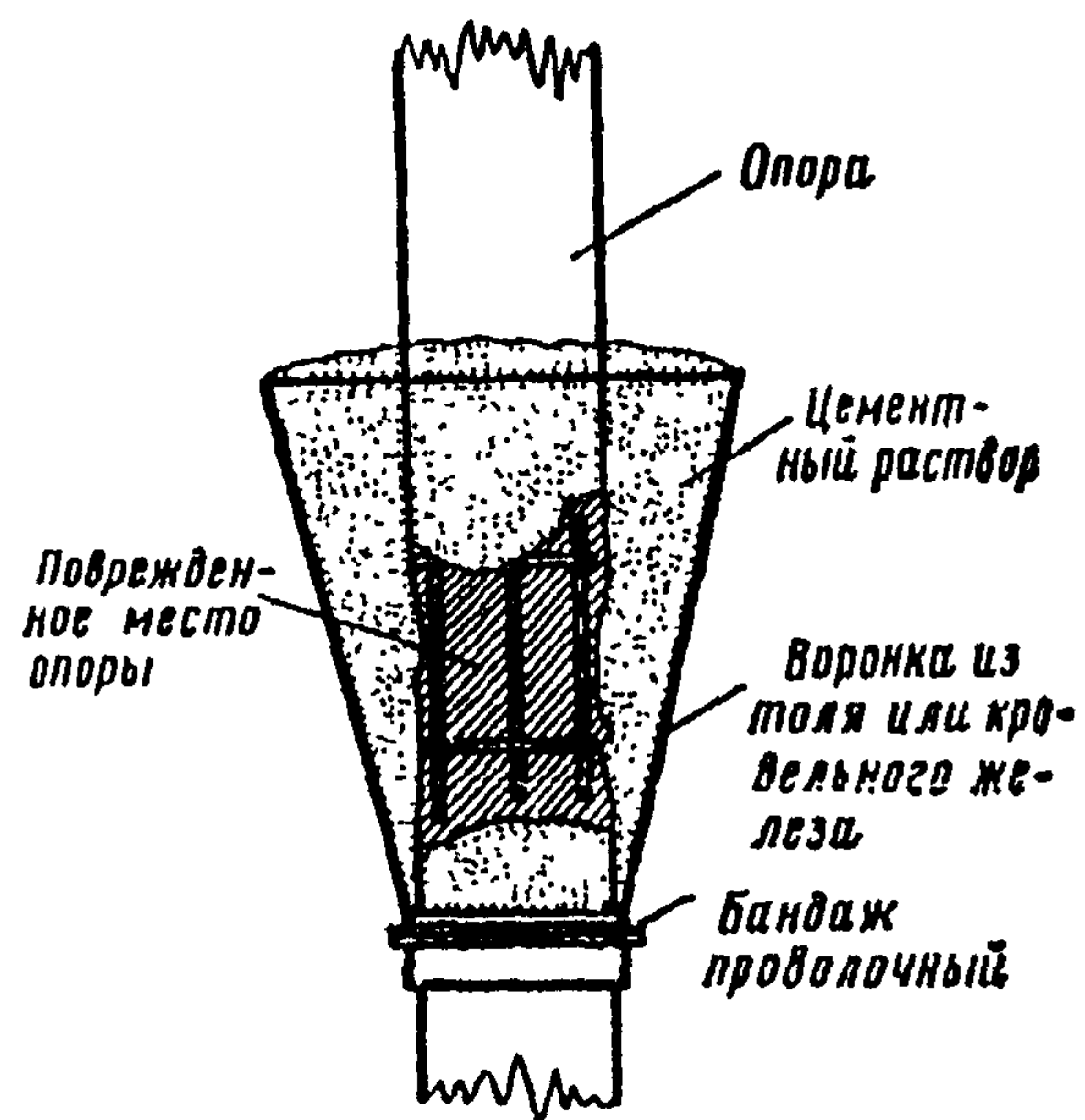
Рис. 6.1. Ремонт железобетонной опоры
