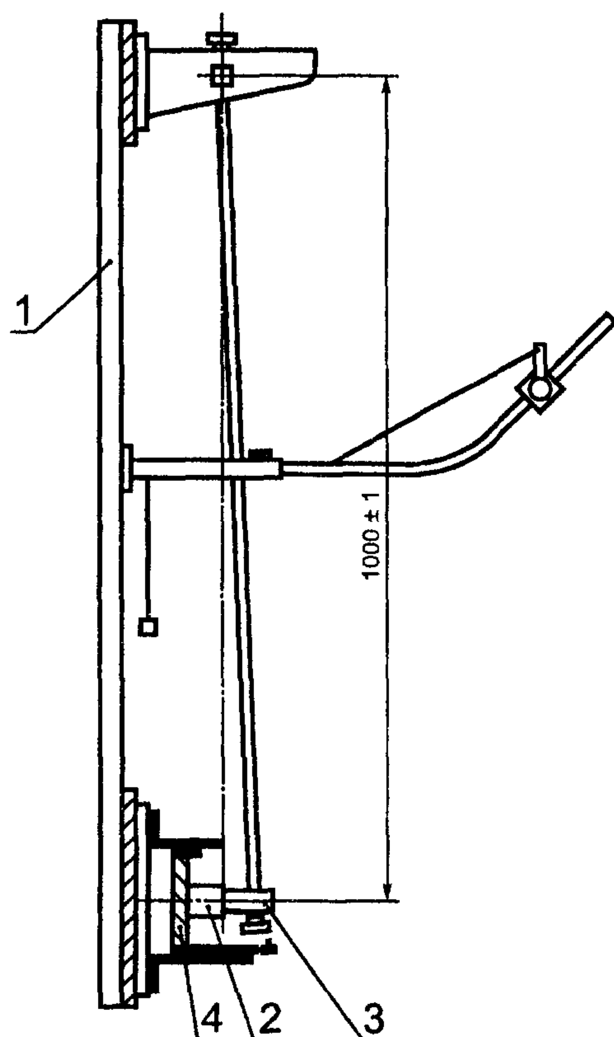
1 — плита (рама); 2 — образец; 3 — боек; 4 — монтажная опора
