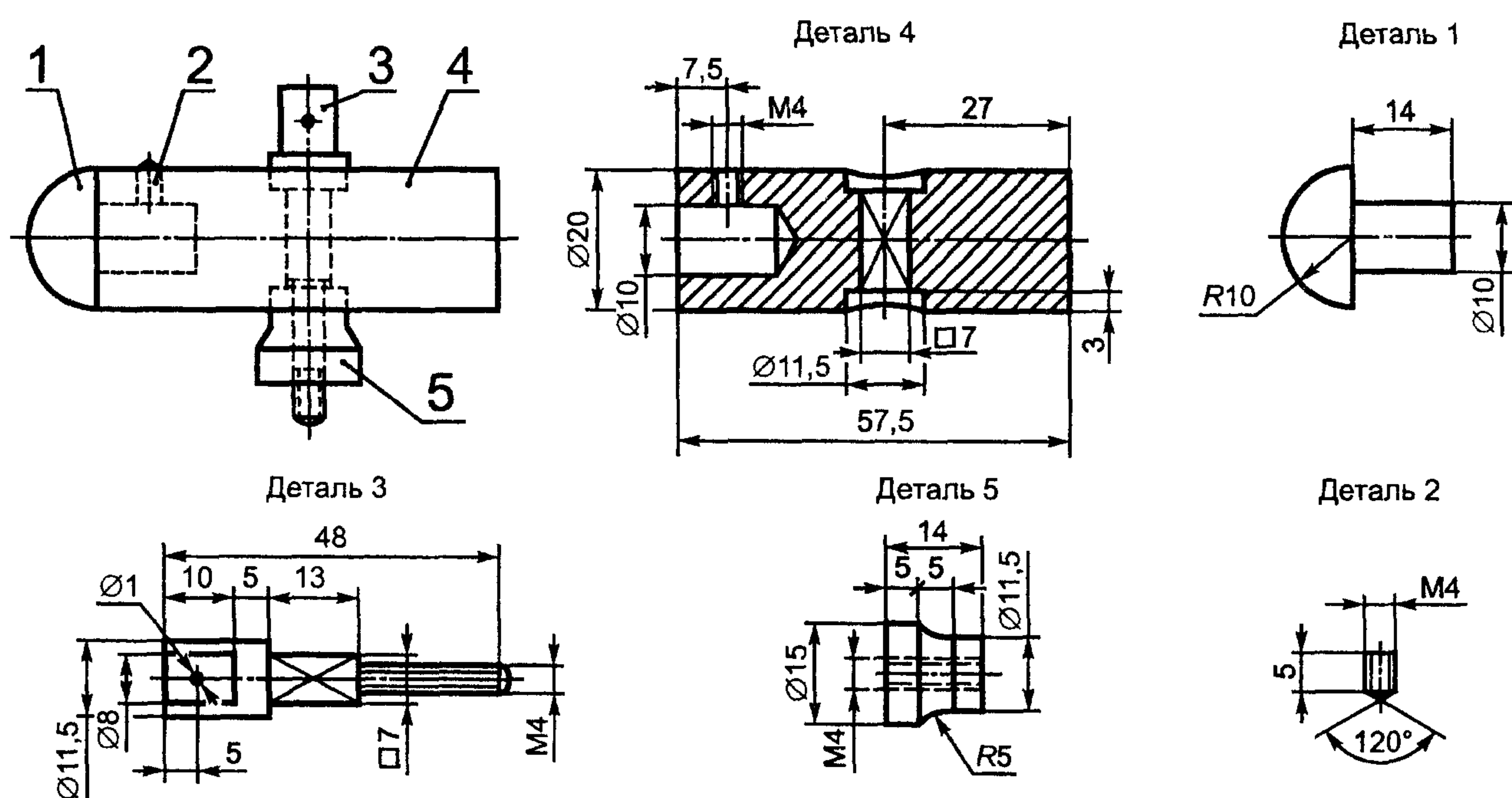
Материал: 1 — полиамид; 2 — 5 — сталь
