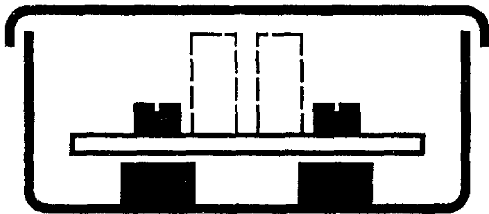
Рисунок В.3 — Коробка, обеспечивающая встроенность зажима или соединительного устройства
