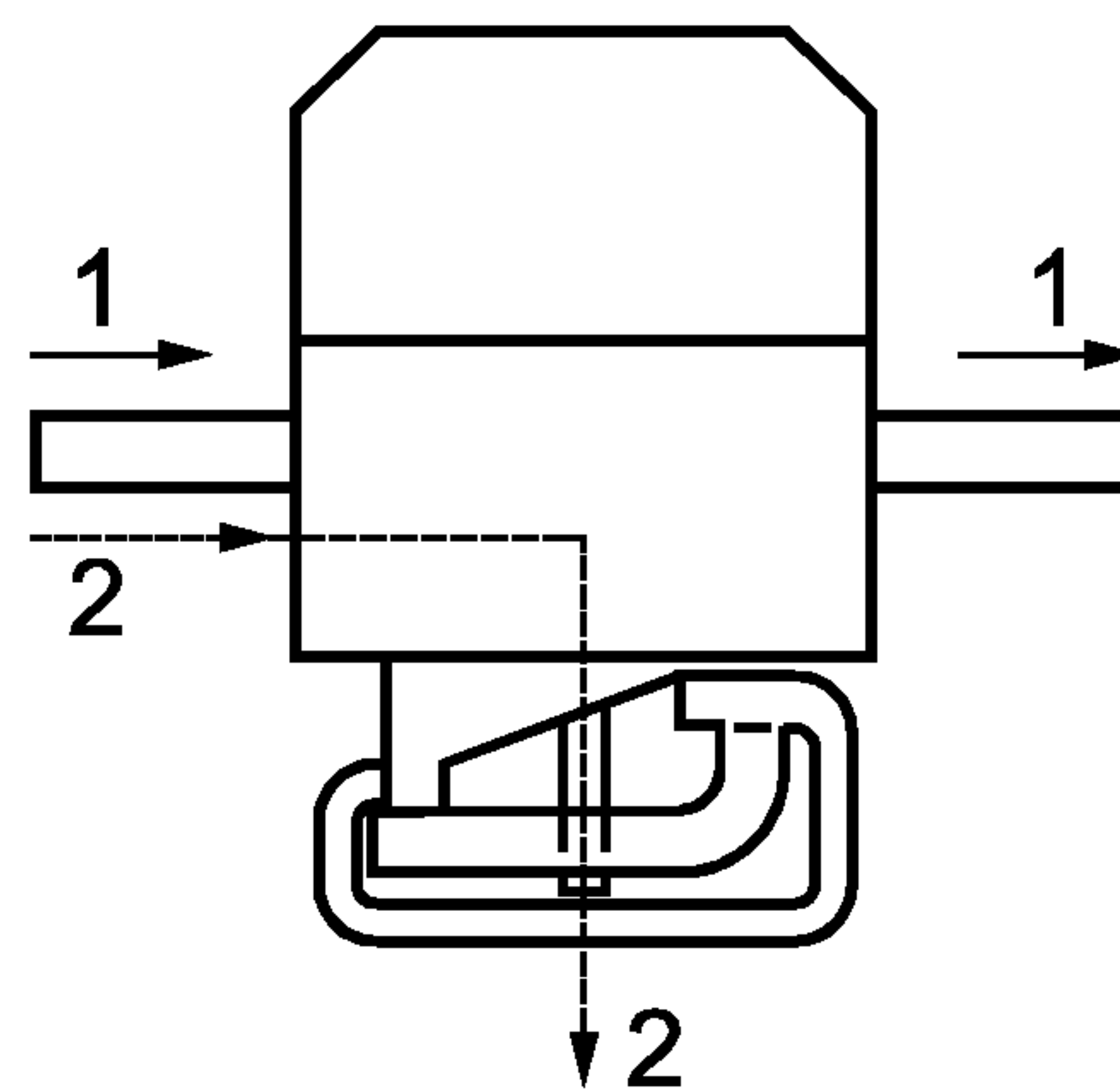
Рисунок 4 — Испытание на тепловой ток короткого замыкания
