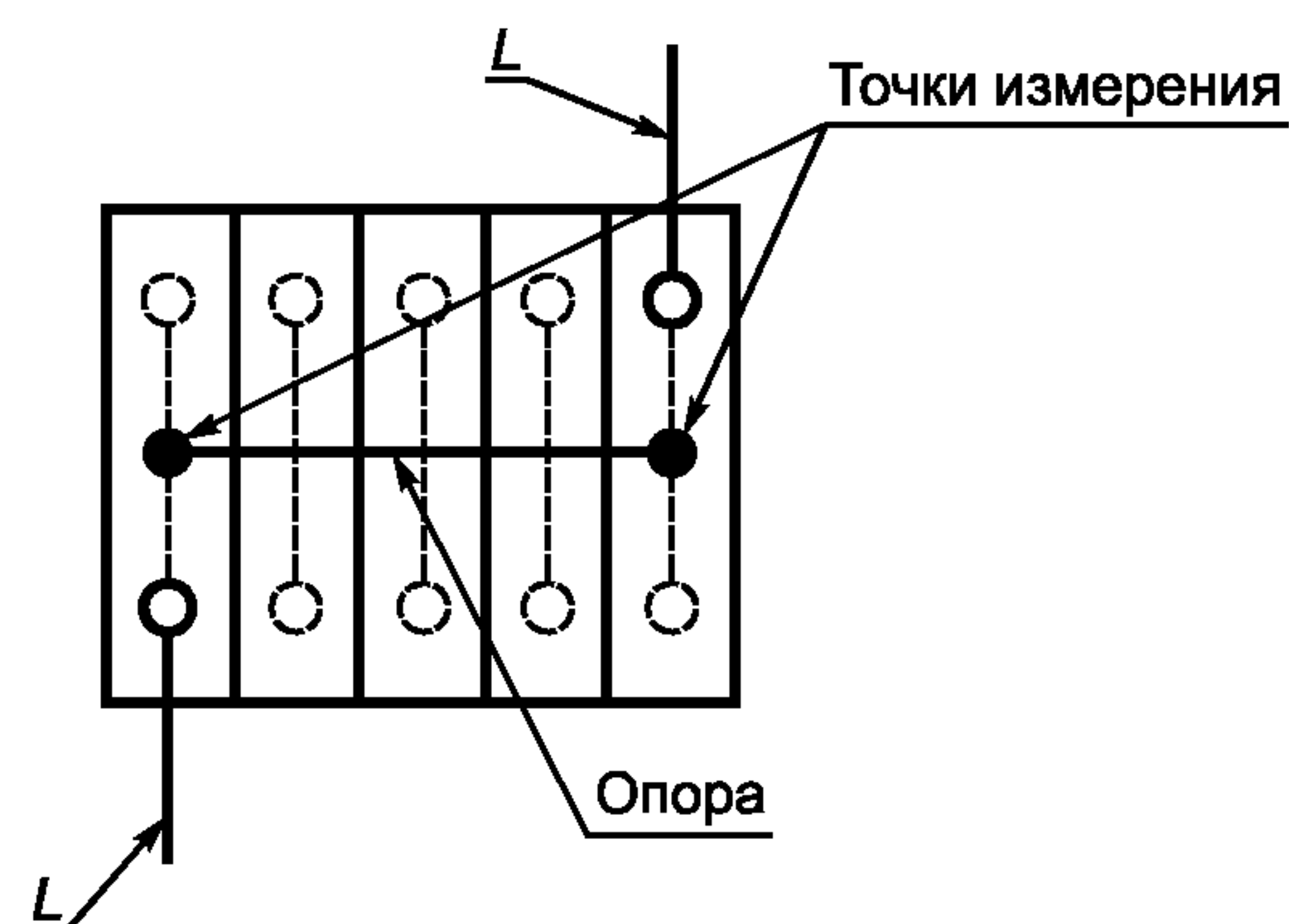
Рисунок 3 — Установка для испытания на превышение температуры для второй группы испытаний
