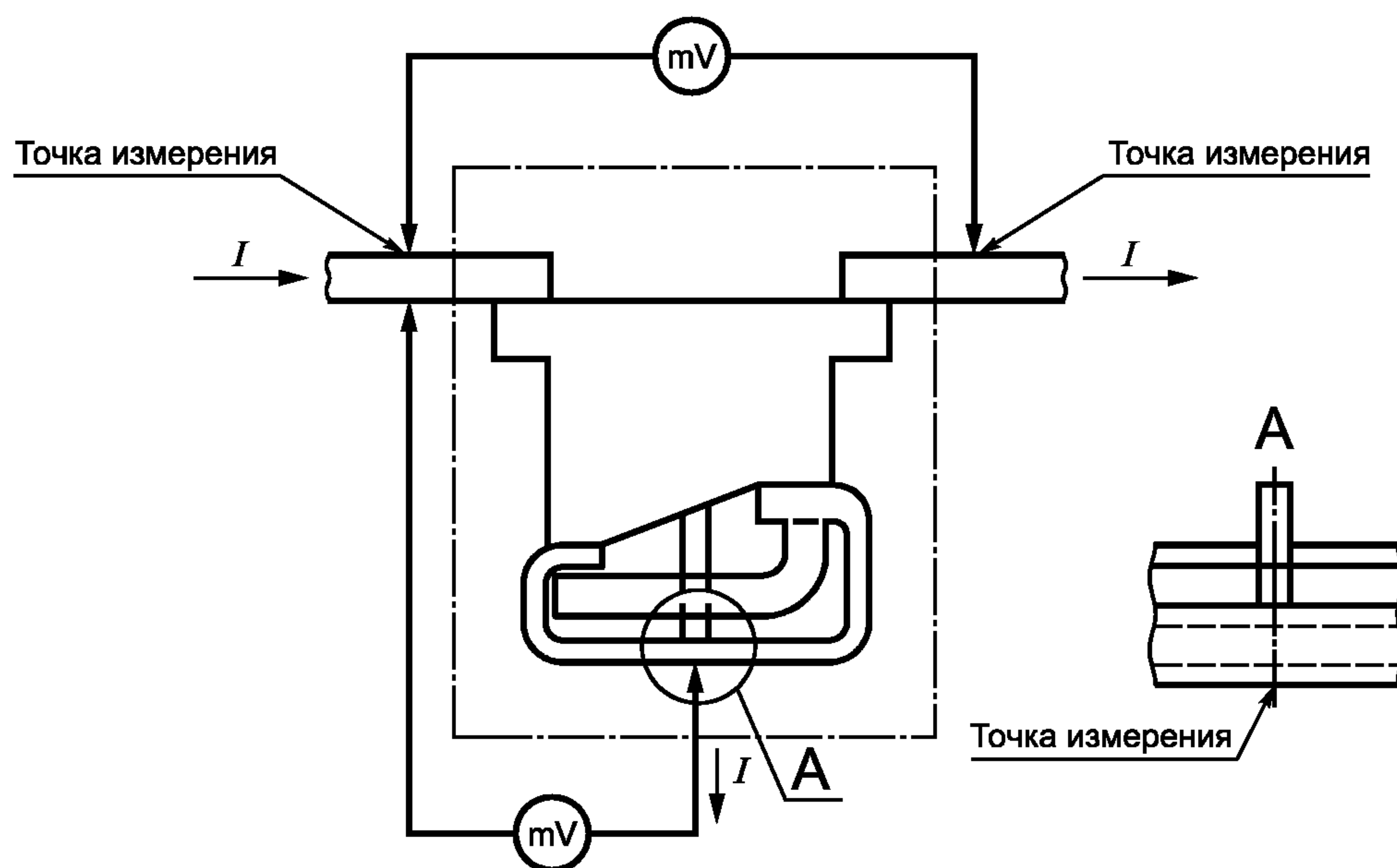
Рисунок 1 — Установка для испытания на падение напряжения
