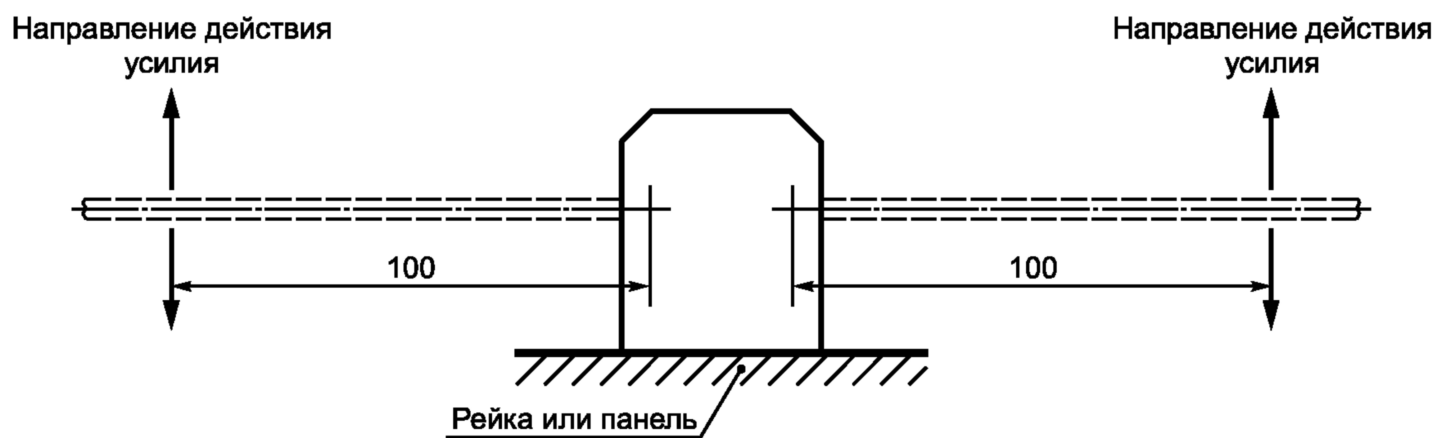
Рисунок 1 — Установка для испытания
