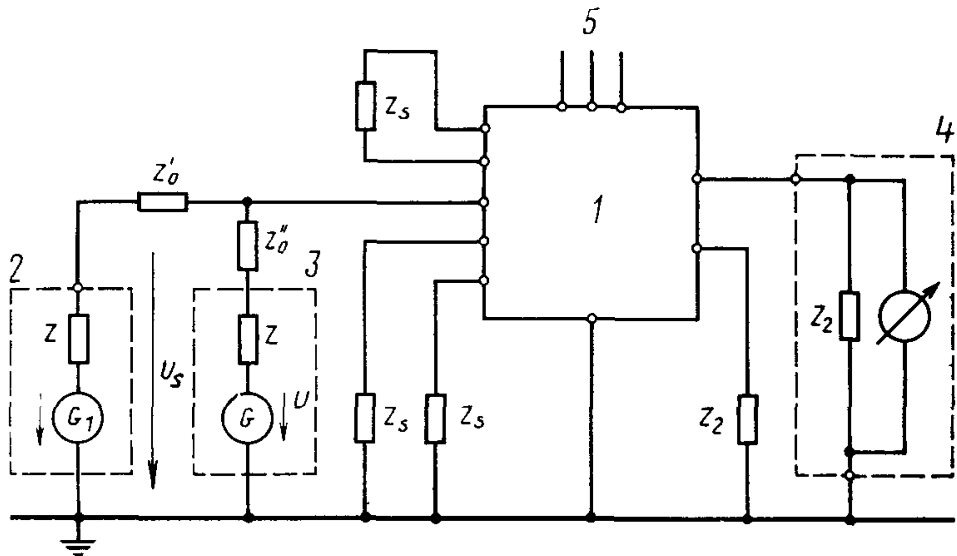
1—испытуемое изделие; 2—генератор входного сигнала; 3—генератор стандартных помех; 4—испытательное устройство на выходе изделия; 5—источник питания
