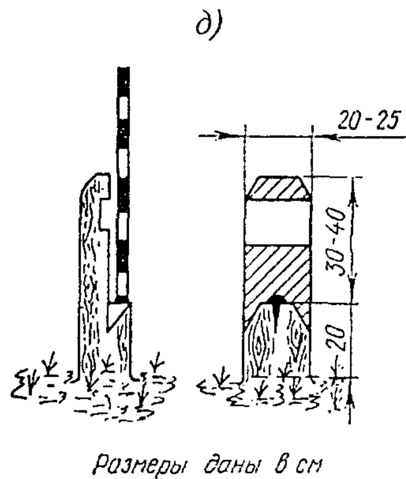
Рис. 4.1. Типы знаков долговременного закрепления пунктов съёмочного обоснования
