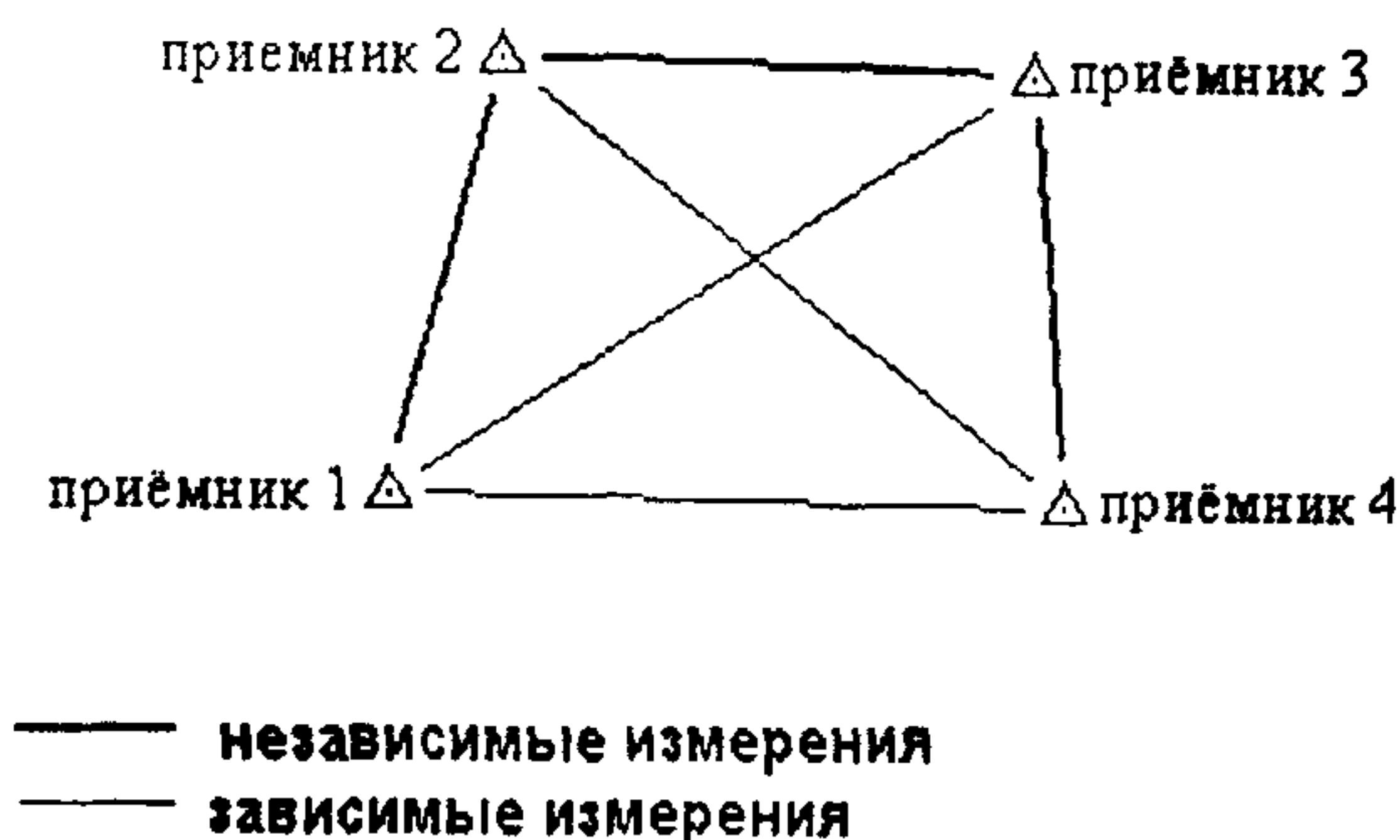
Рис. 2. Схема, иллюстрирующая проект независимого определения 3-х линий из сеанса, выполняемого на 4-х пунктах
