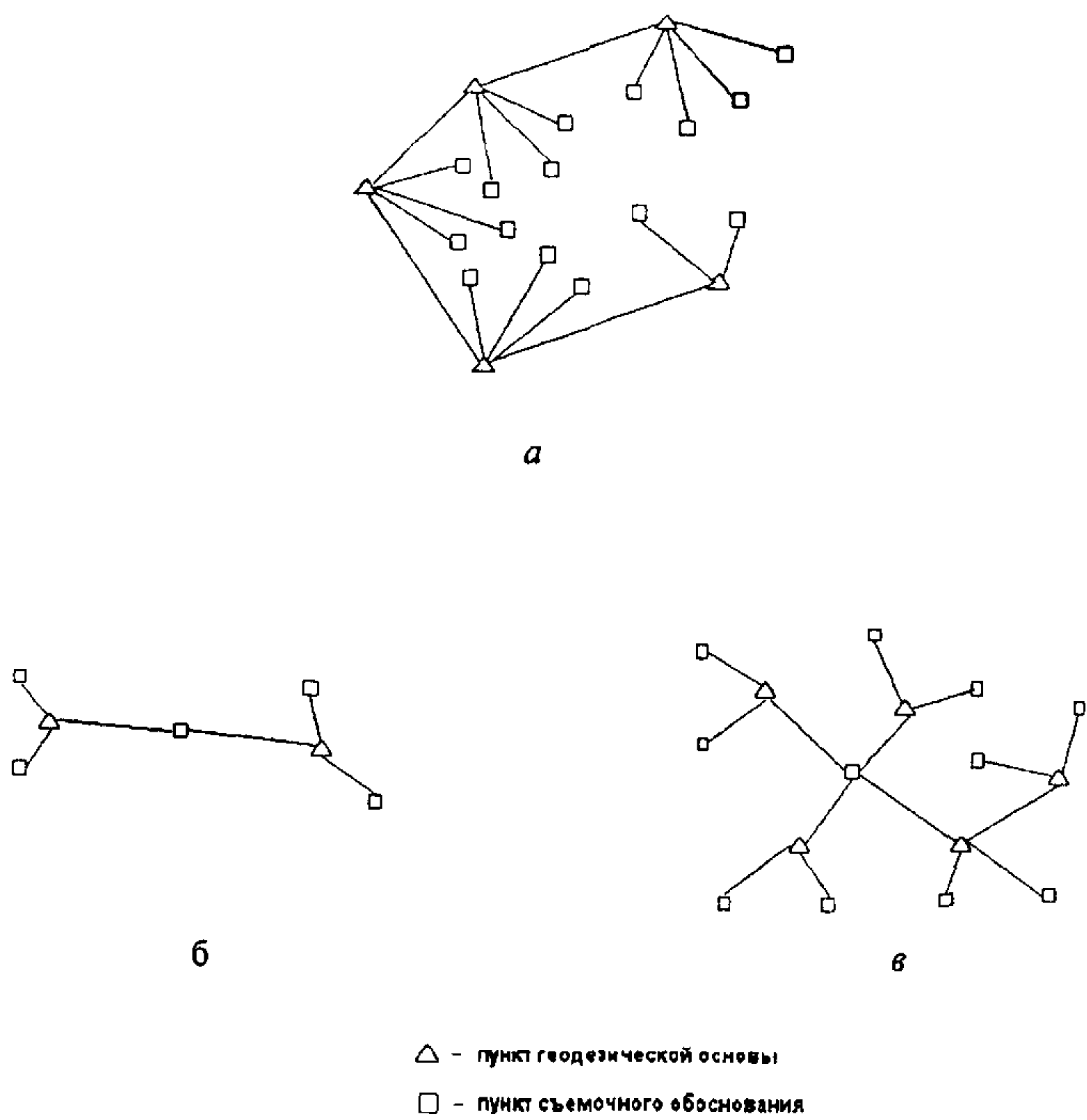
Рис. 3. Схемы, иллюстрирующие проект развития съёмочного обоснования методом определения висячих пунктов
