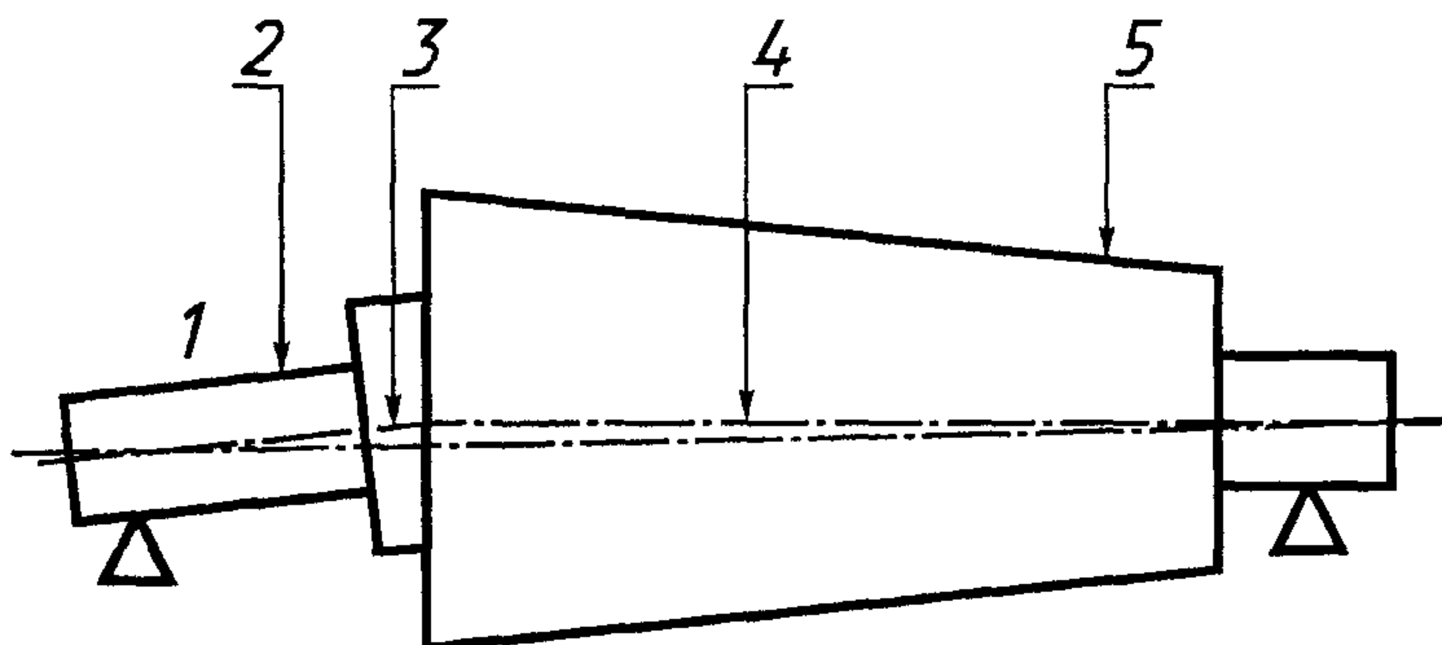
1 — цапфа; 2 — оправка; 3 — ось оправки; 4 — ось ротора; 5 — ротор
