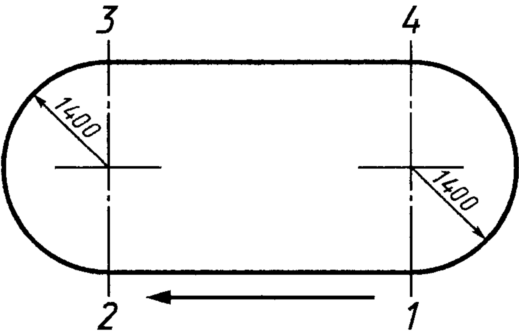
Рисунок А.1 — Испытательный полигон
