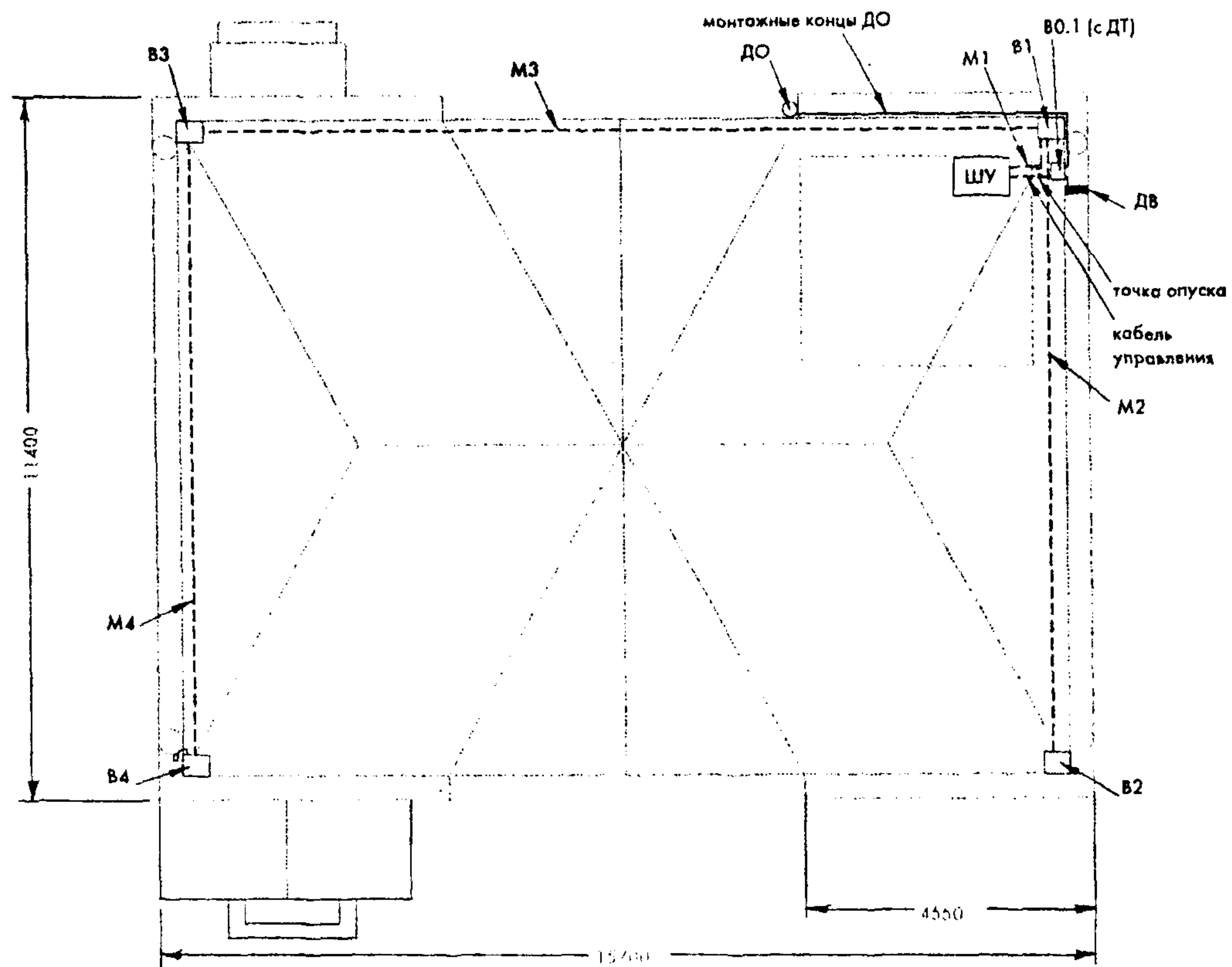
Рис. 4.5. Схема разводки силовых кабелей и кабелей управления.
