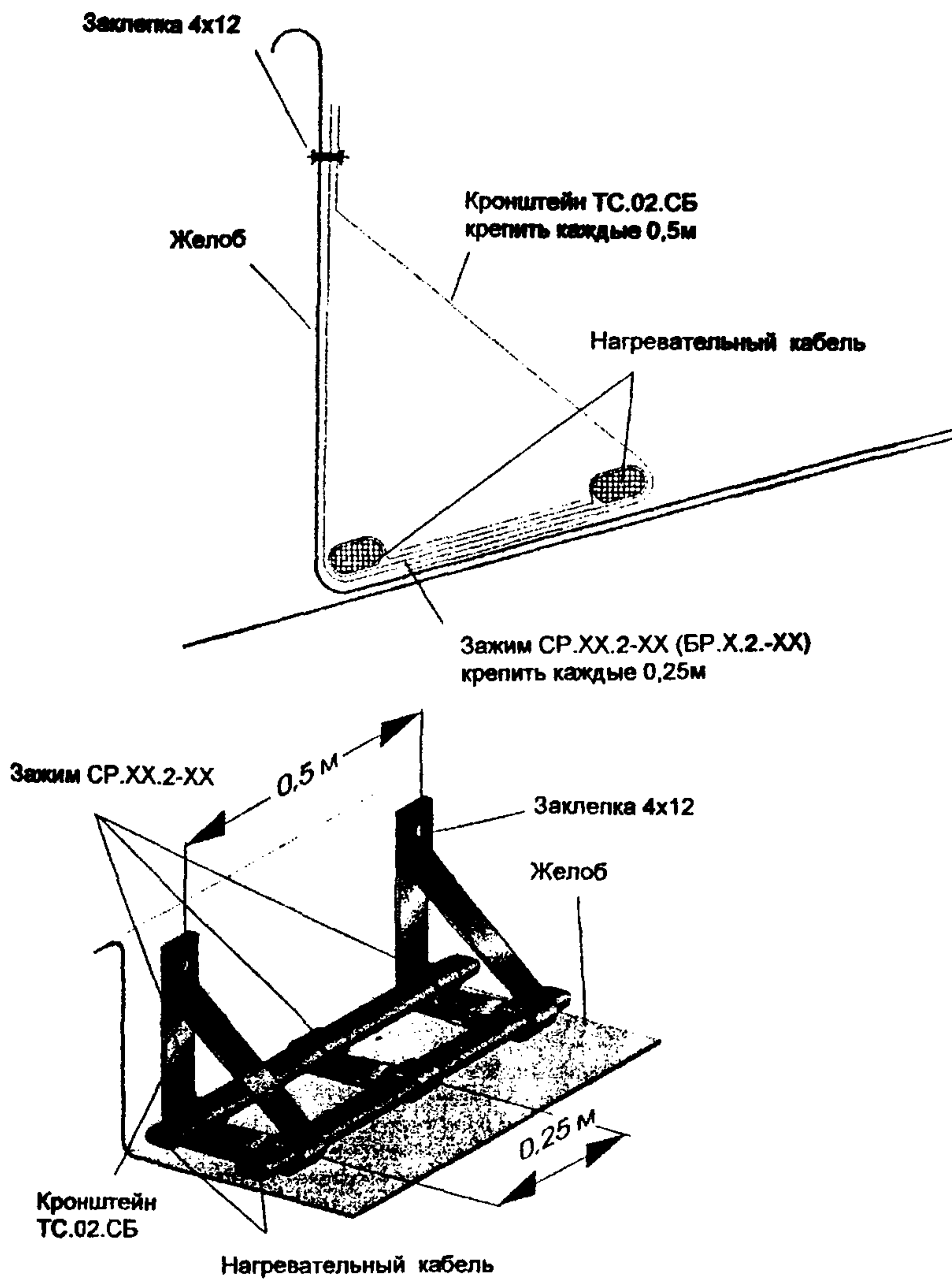
Рис. 5.5. Крепление двух ниток греющего кабеля в желобе.
