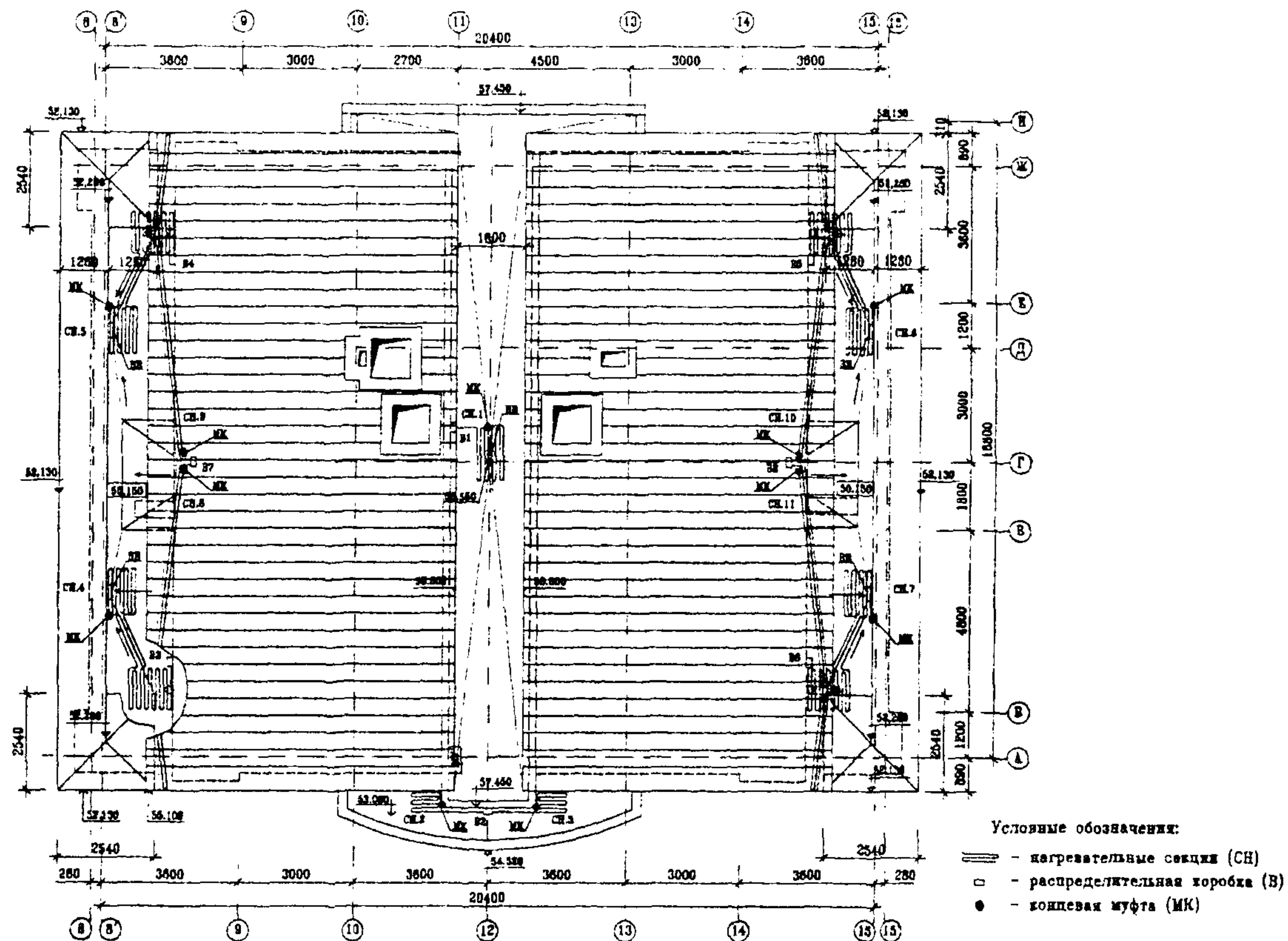
Рис. 4.8. Схема установки нагревательных секций на кровле секции № 2.
