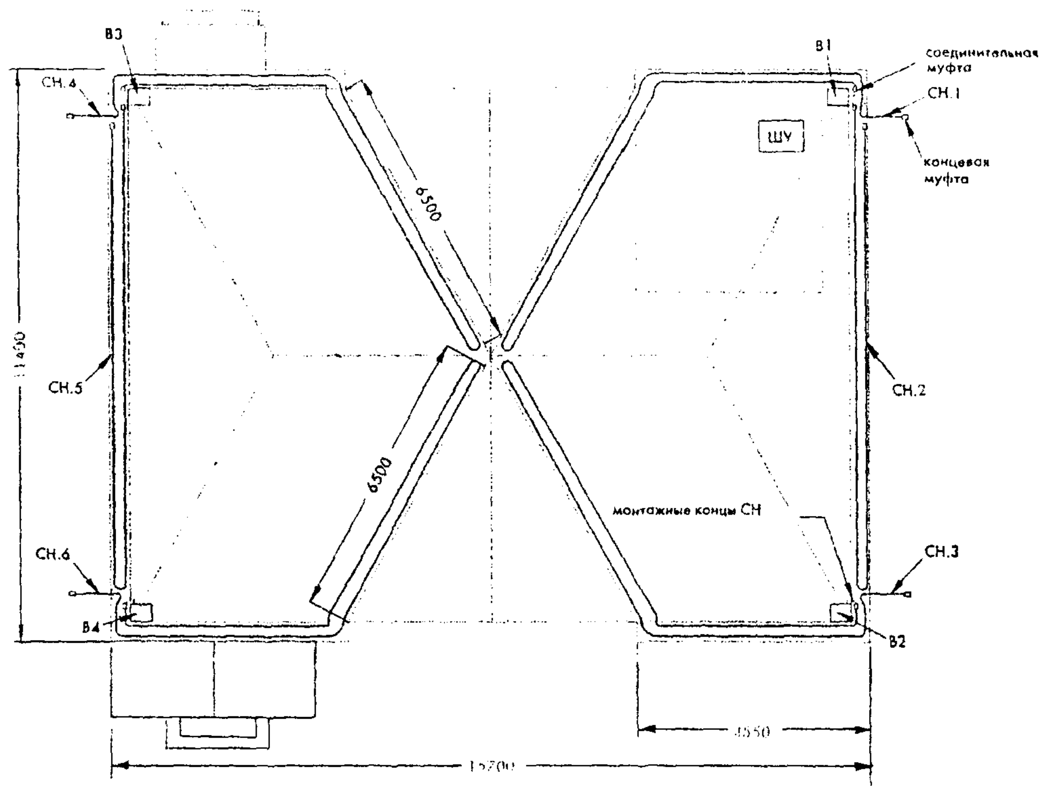
Рис. 4.4. Схема укладки нагревательных секций.
