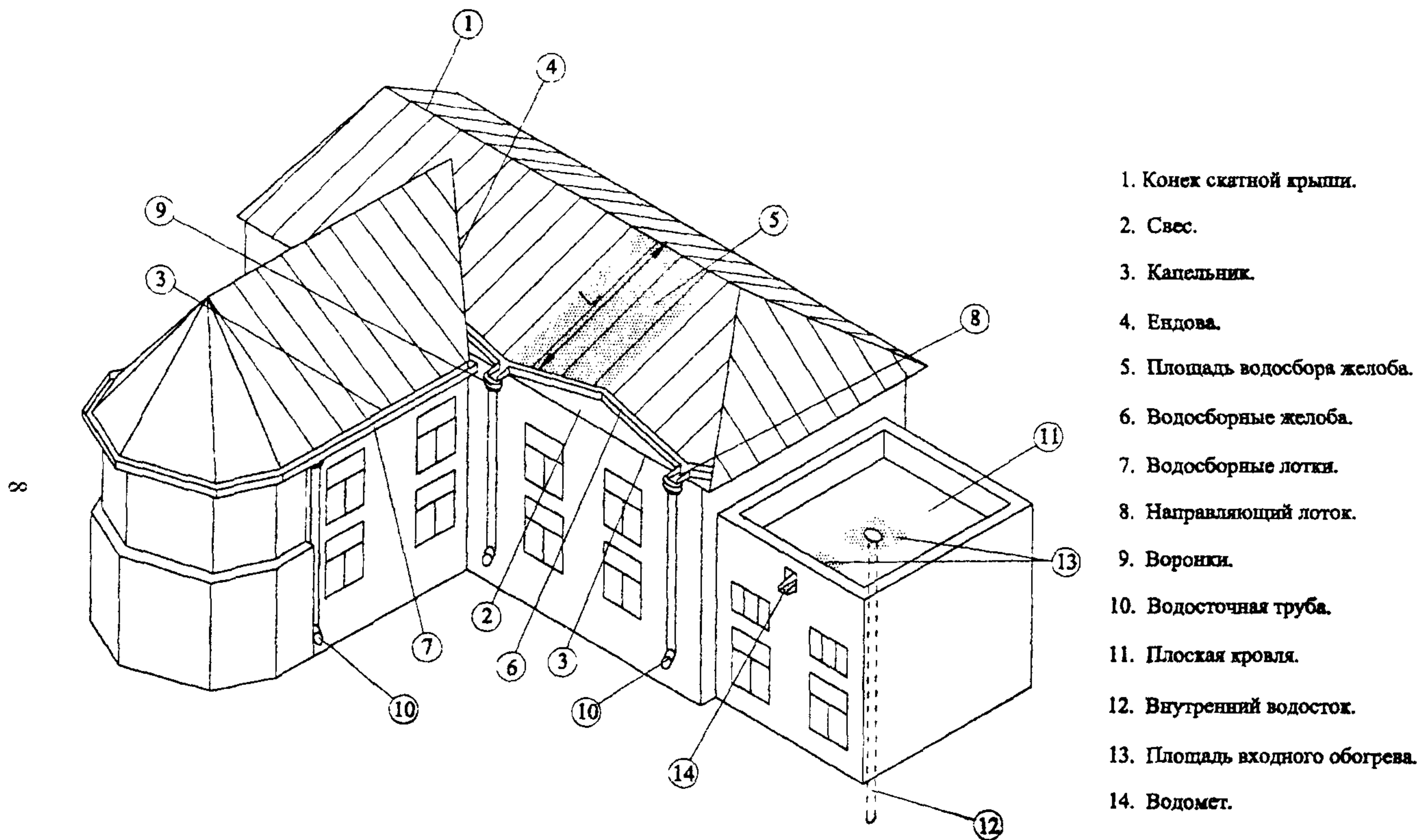
Рис. 2. 1. Схема скатной и плоской крыш с элементами организованного водостока.
