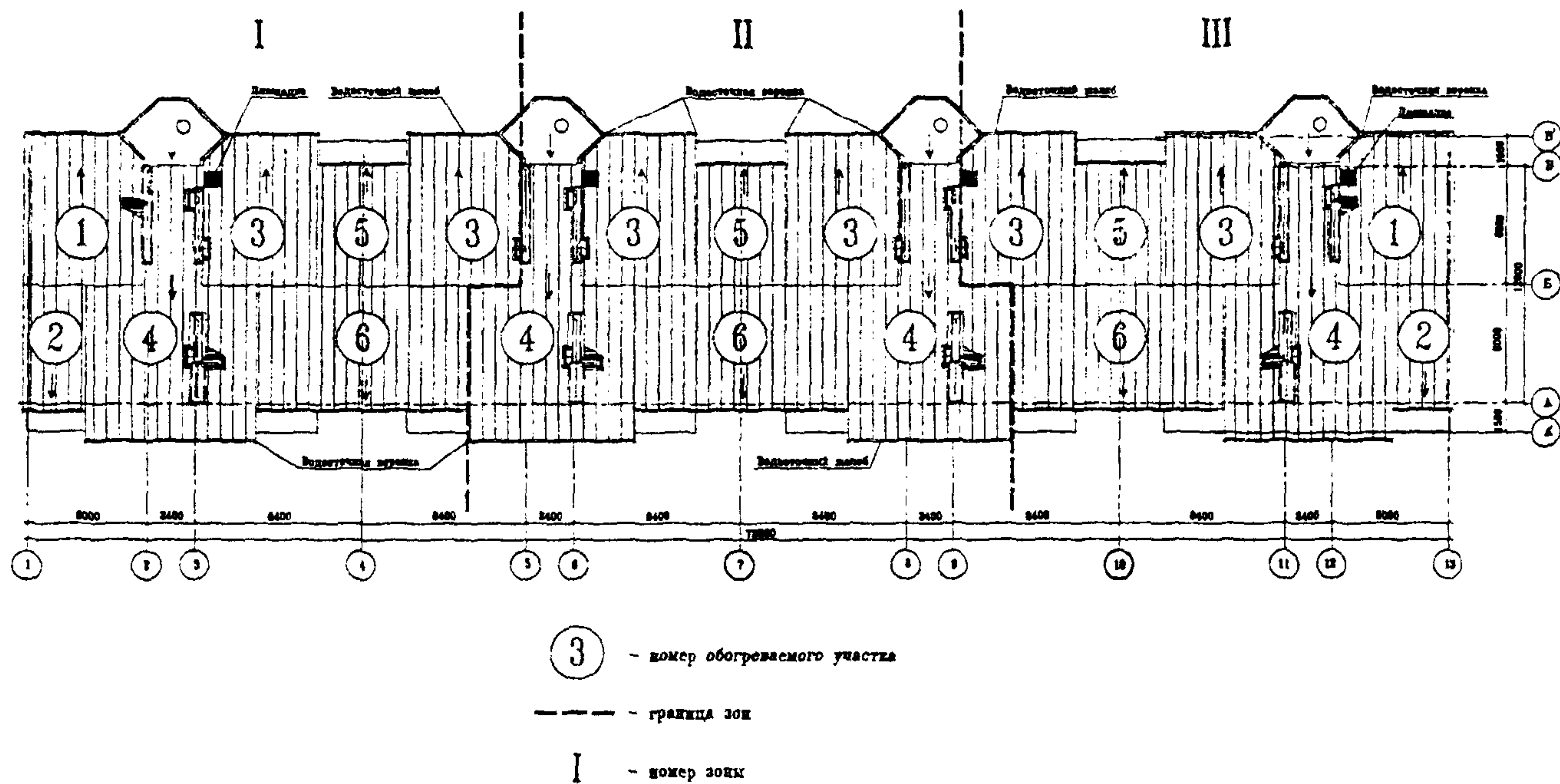
Рис. 4.10. Схема деления кровли на участки и зоны.
