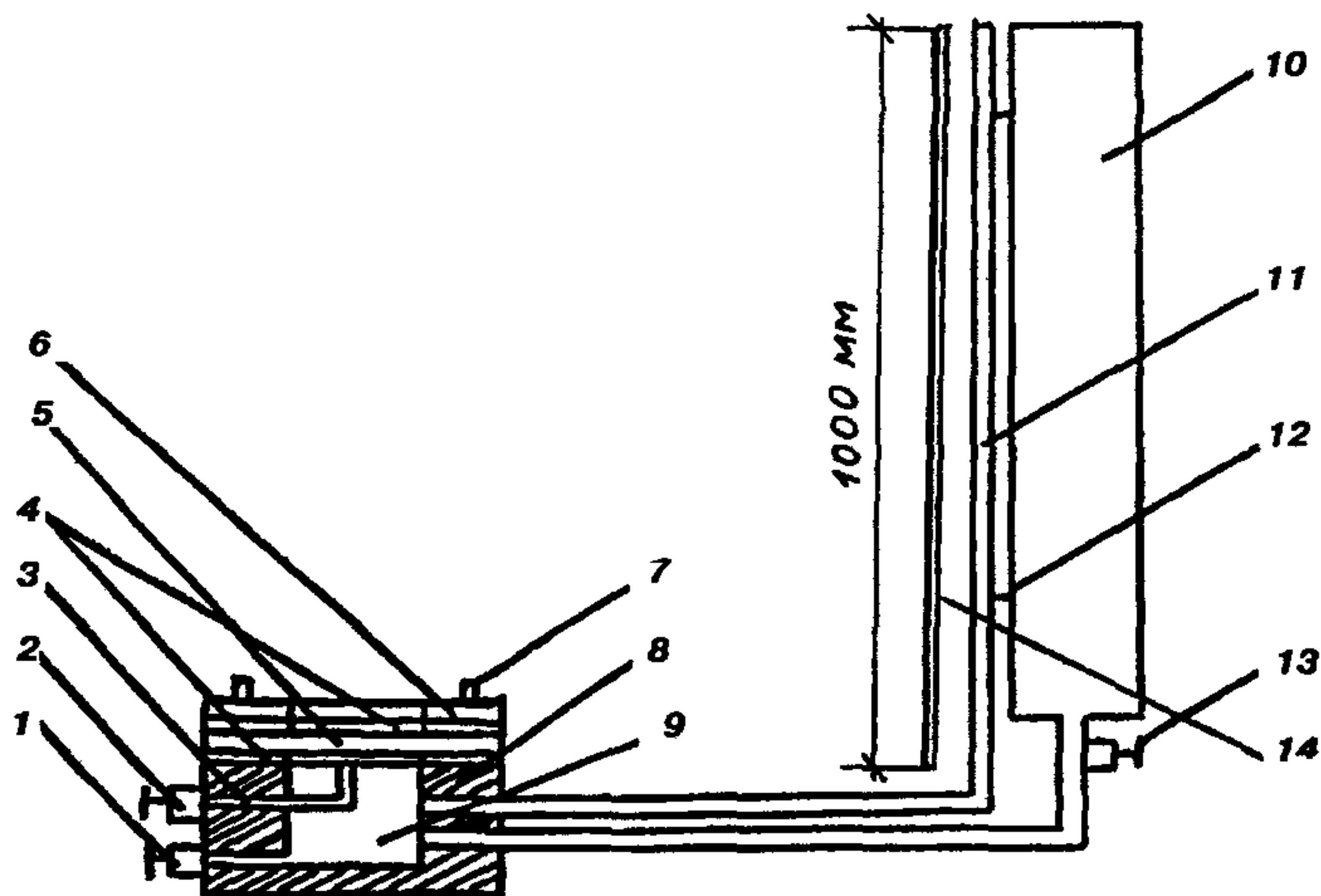
Рис. 2. Принципиальная схема установки для определения водонепроницаемости материалов:
