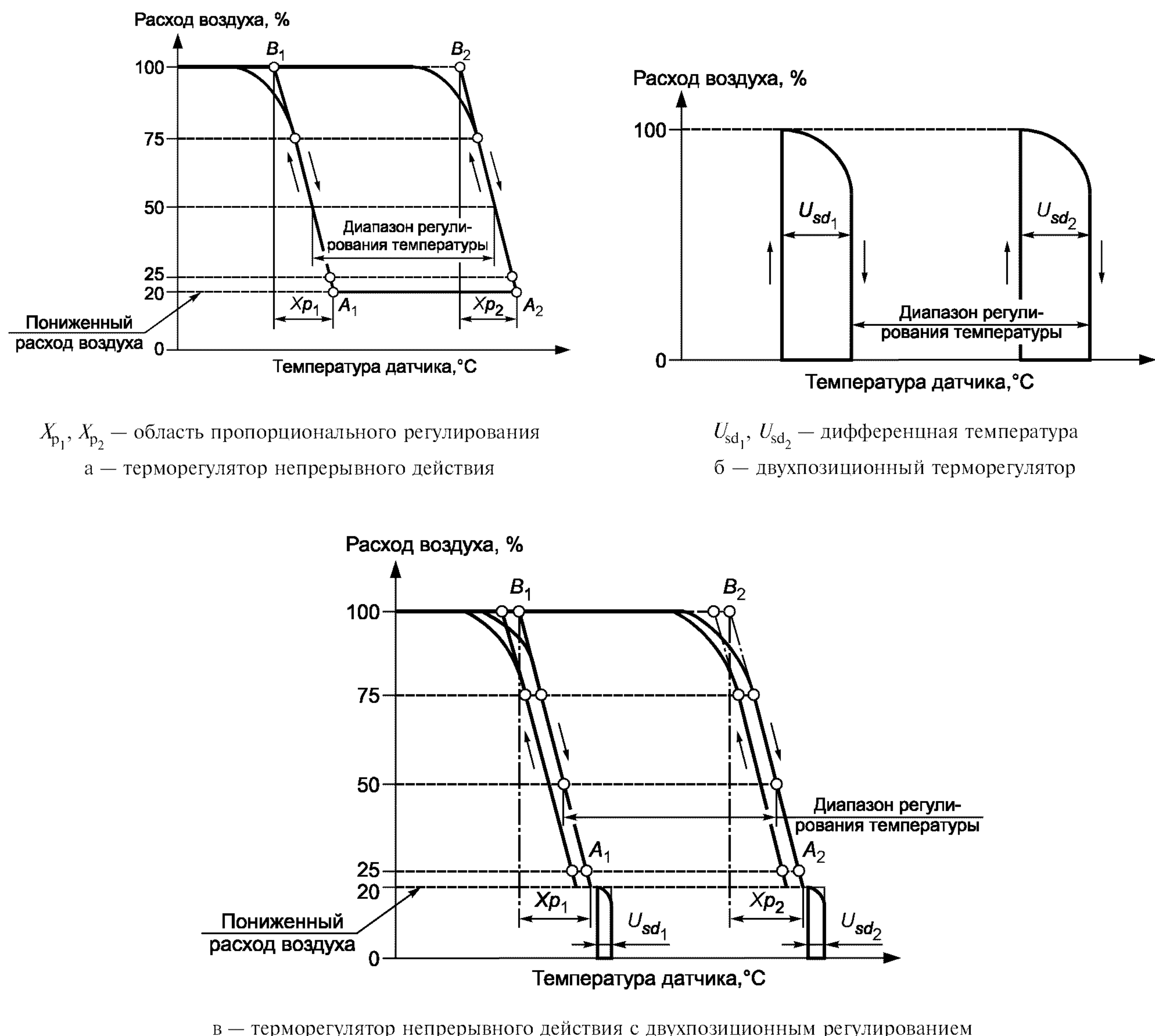
Рисунок 2 — Типовые характеристики терморегуляторов
