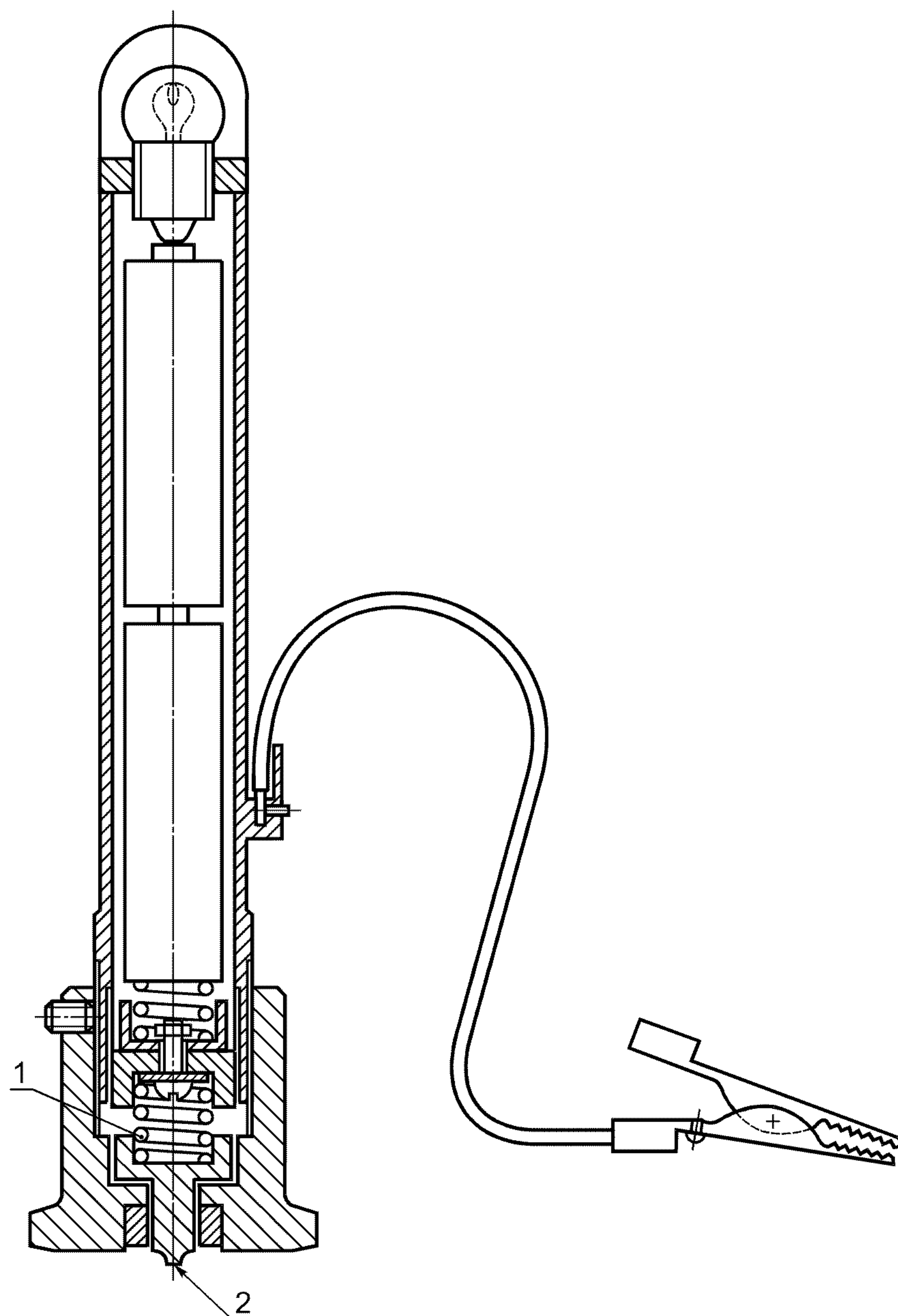
1 — пружина; 2 — рабочая точка (стальной шарик диаметром 1 мм)
