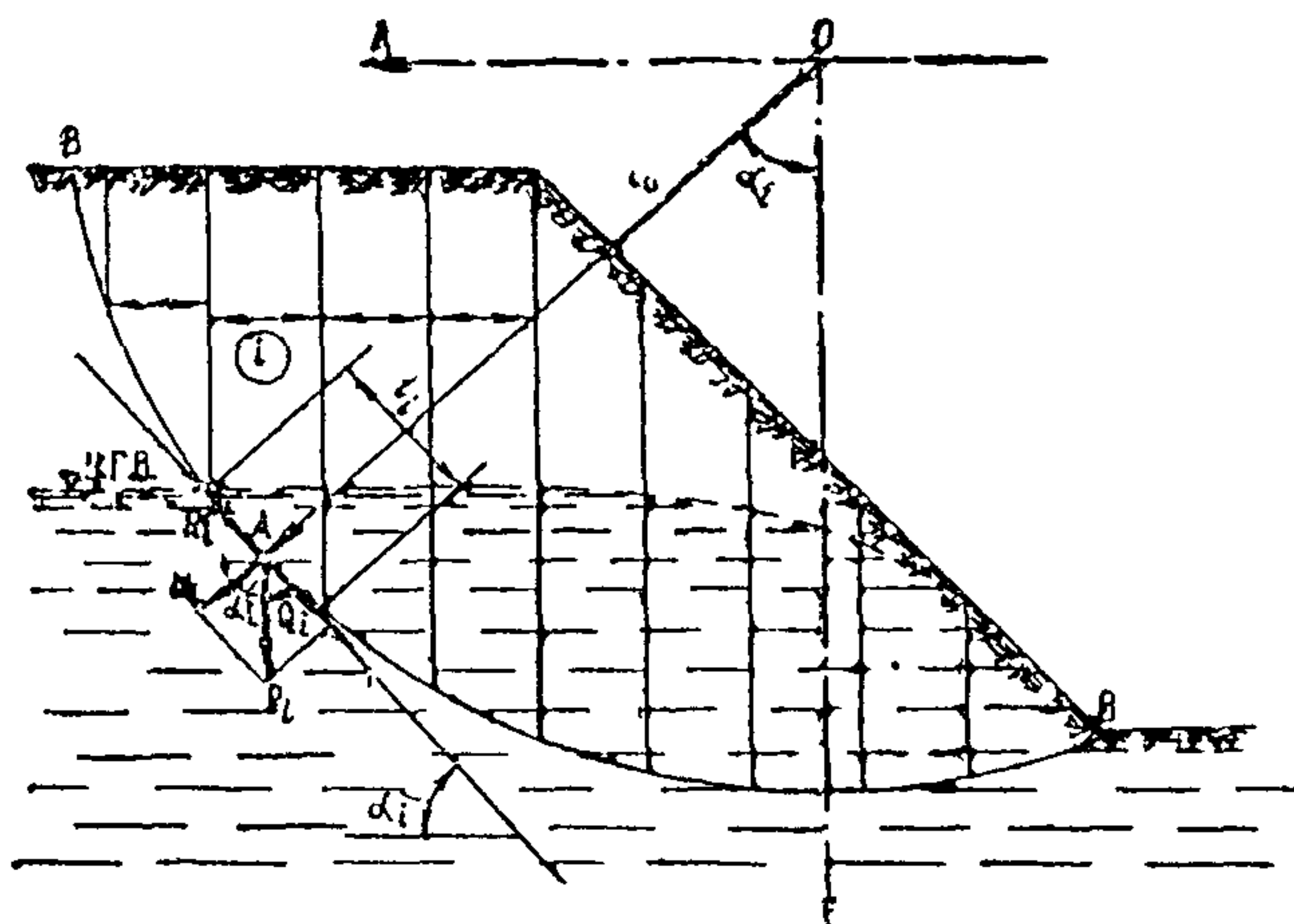
Рис. 2. Метод круглоцилиндрической поверхности скольжения
