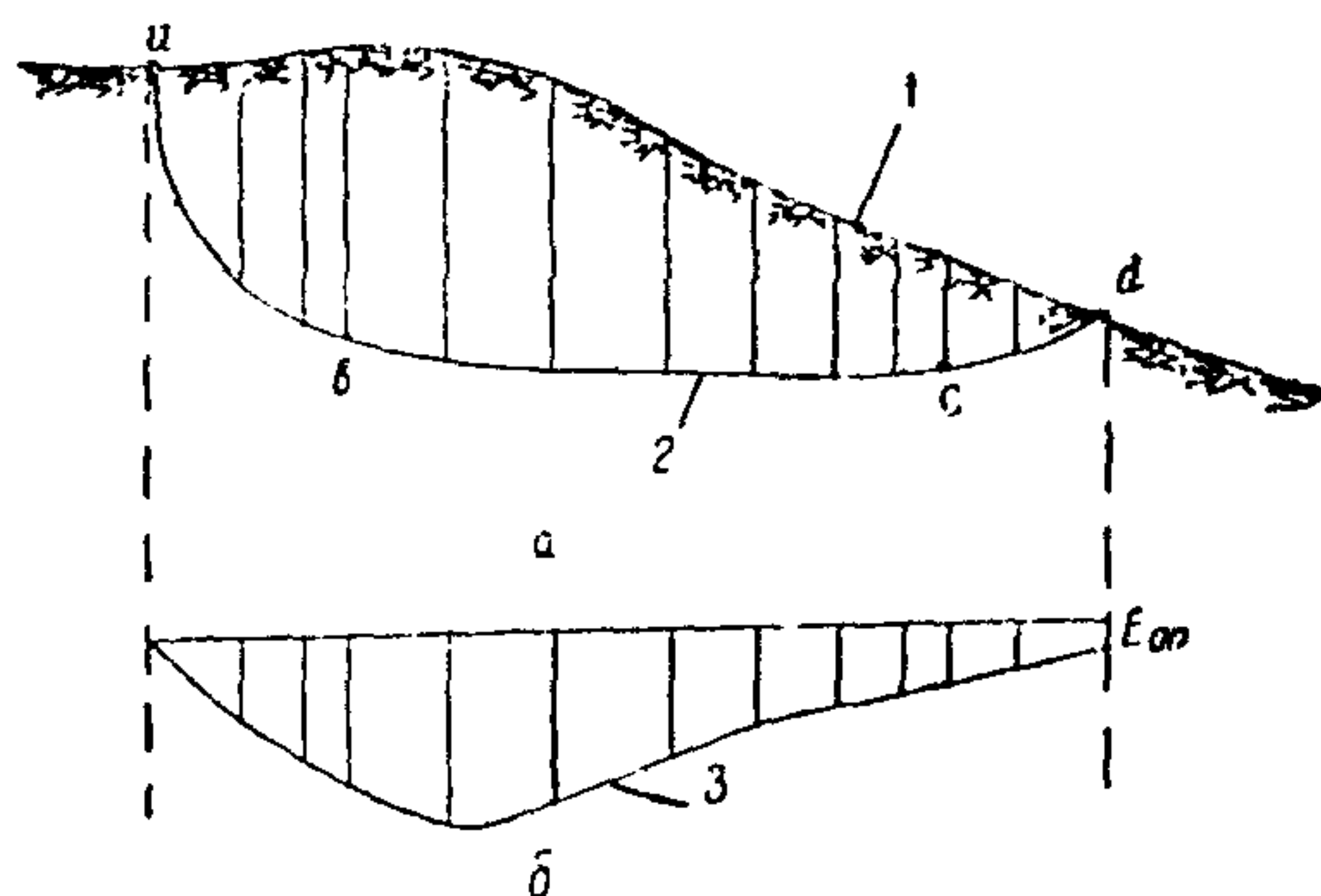
Рис. 29. Расчетный поперечник (а) с эпюрой оползневое давления (б): 1 — поверхность склона; 2 — поверхность скольжения; 3 — контур эпюры оползневое давления
