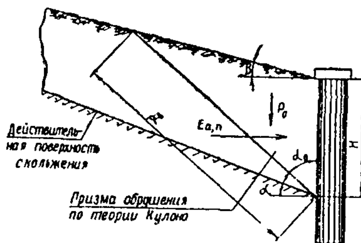
Рис. 23. Методы, основанные на теории Кулона
