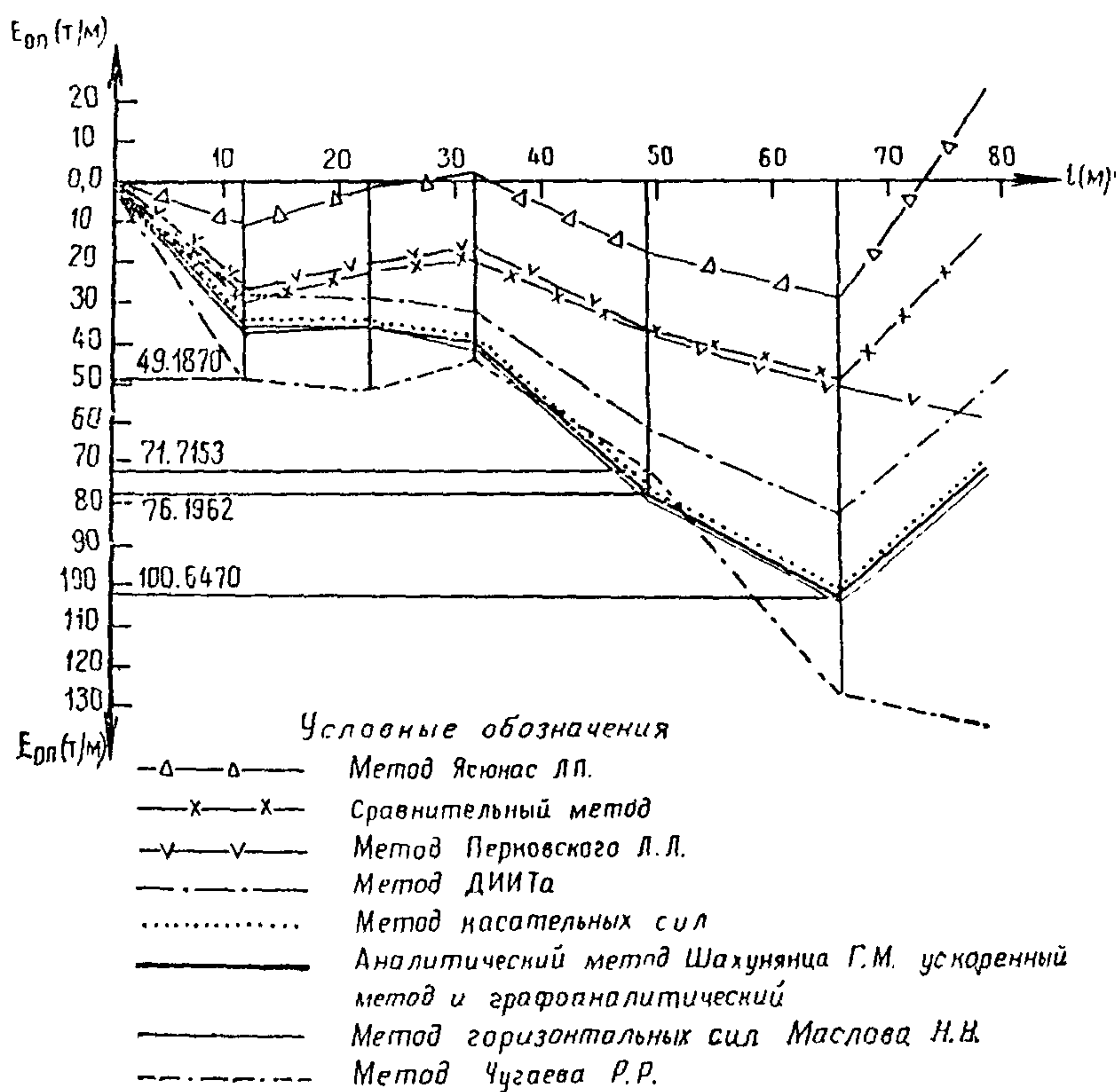
Рис. 24. Сравнение эпюр оползневое давления, рассчитанного различными методами
