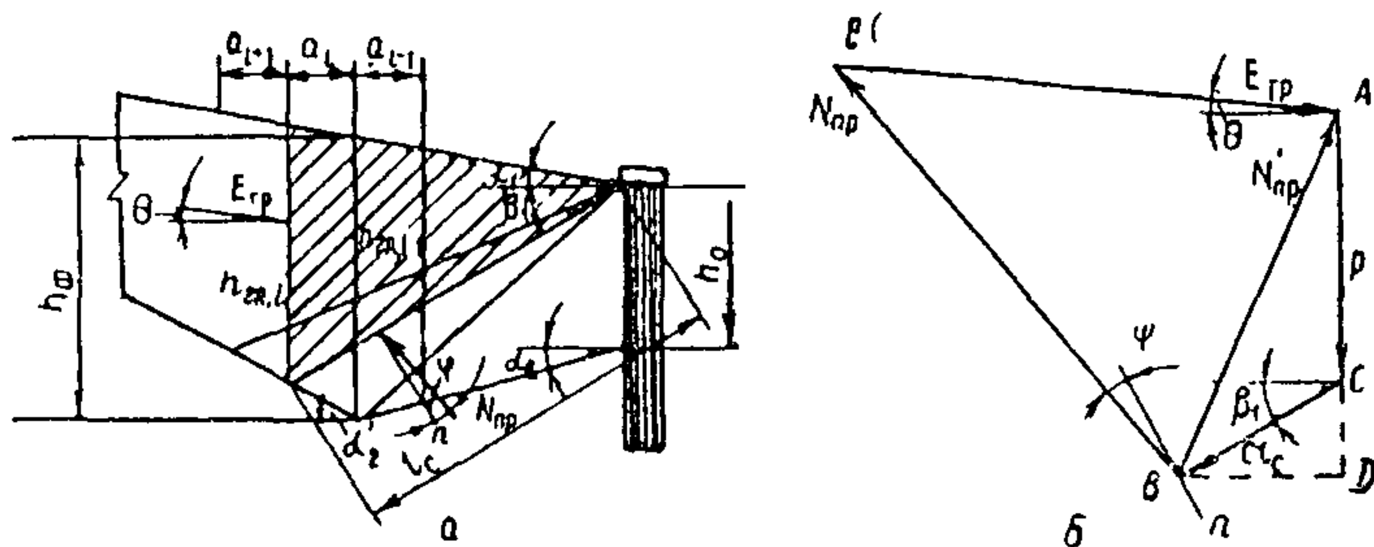
Рис. 22. Определение силы выпора: а — схема клина выпирания; б — силовой многоугольник
