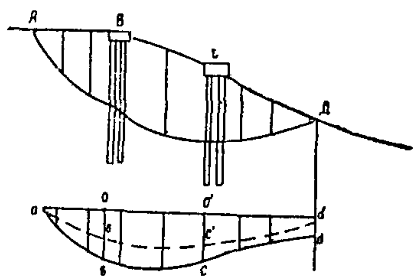
Рис. 32. Учет отпора нижележащего грунта
