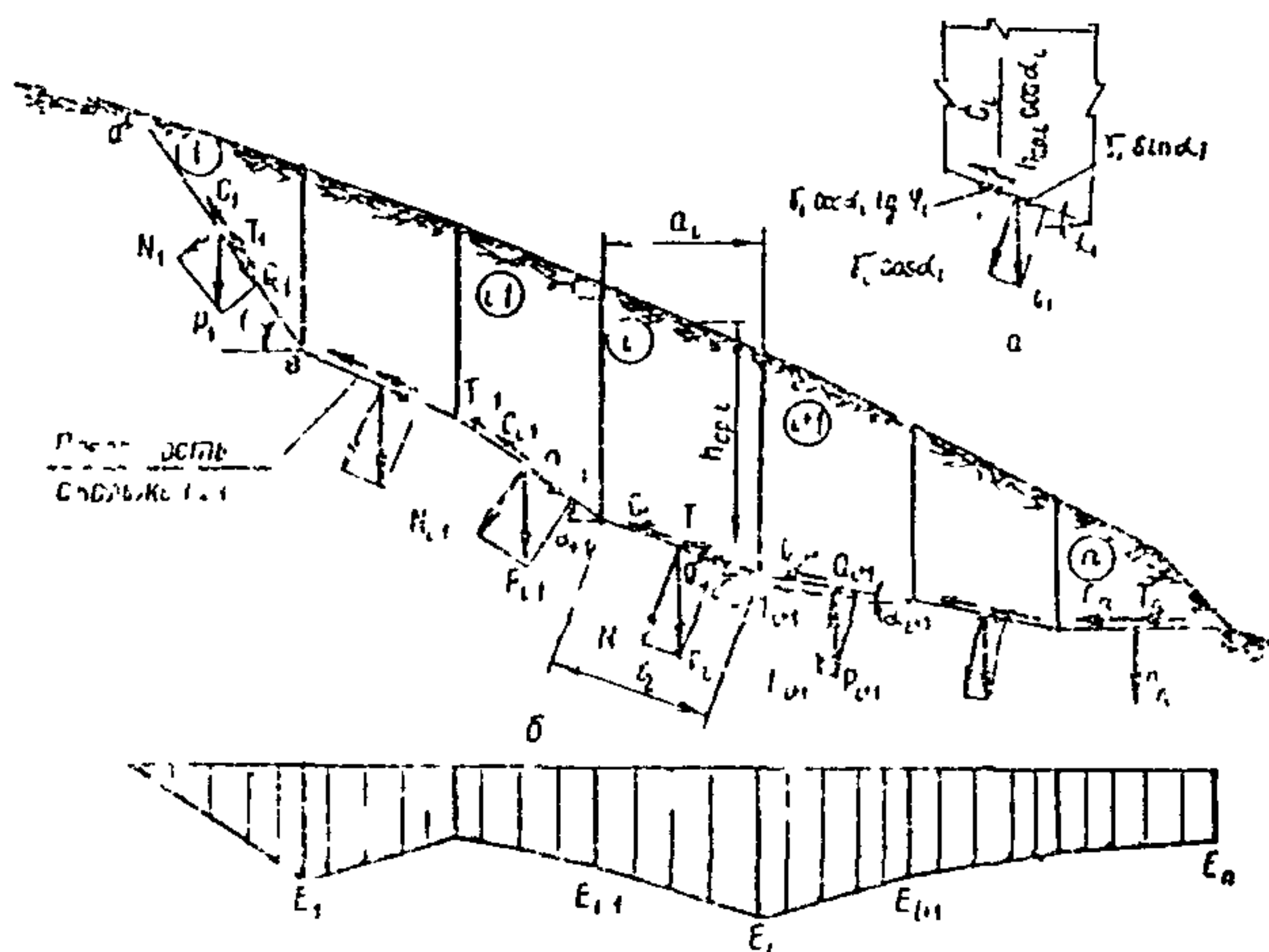
Рис 18 Метод Л. П. Ясюнас.
