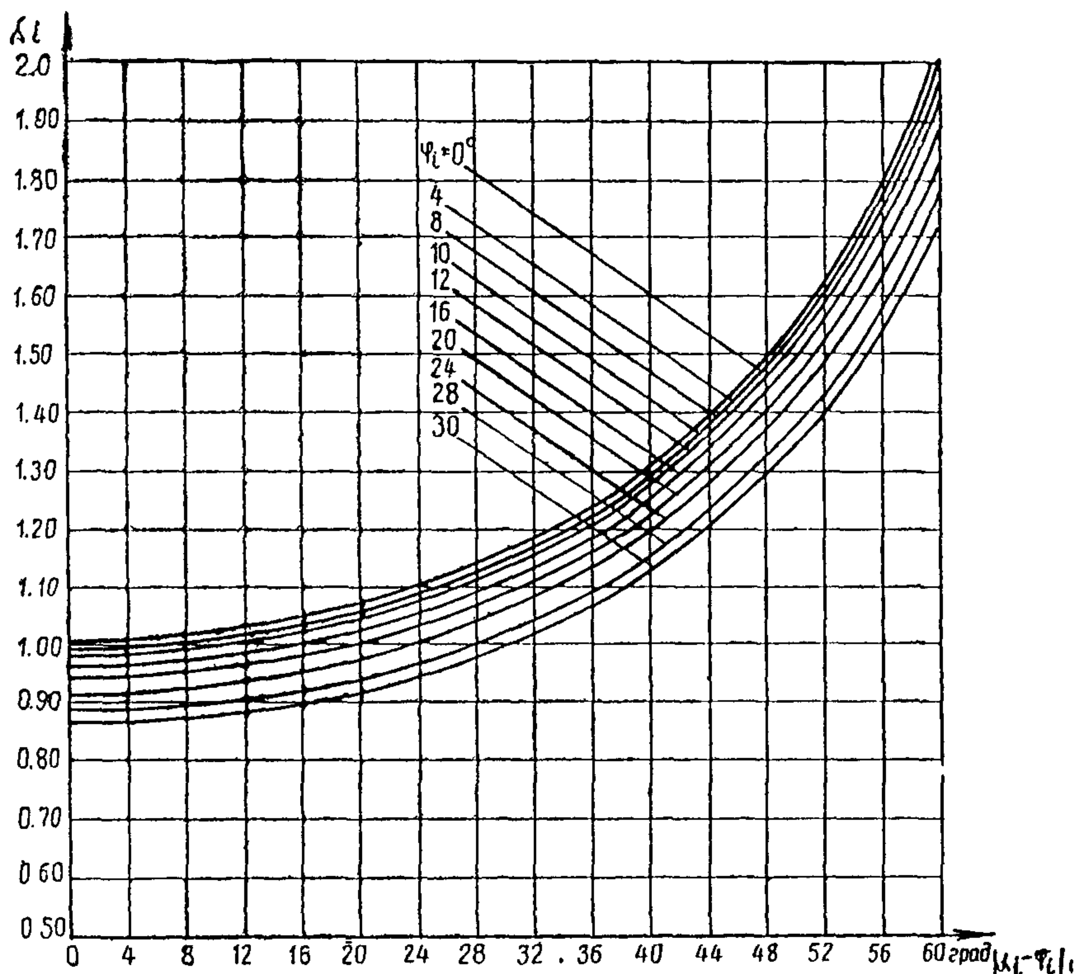
Рис. 15. Графики зависимости \lambda_i = \frac{\cos \varphi_i}{\cos (\alpha_i - \varphi_i)}
