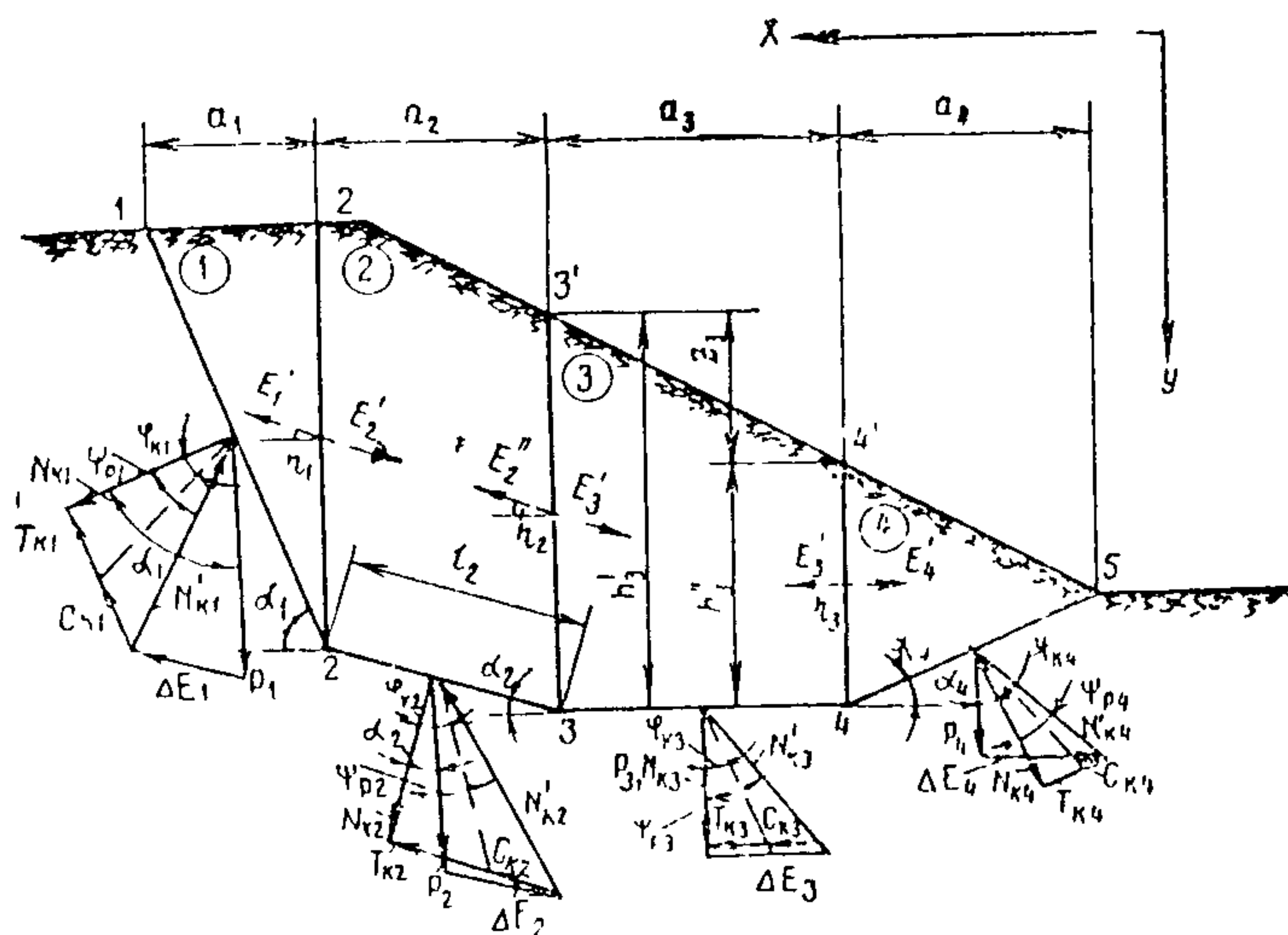
Рис. 6. Метод Р. Р. Чугаева
