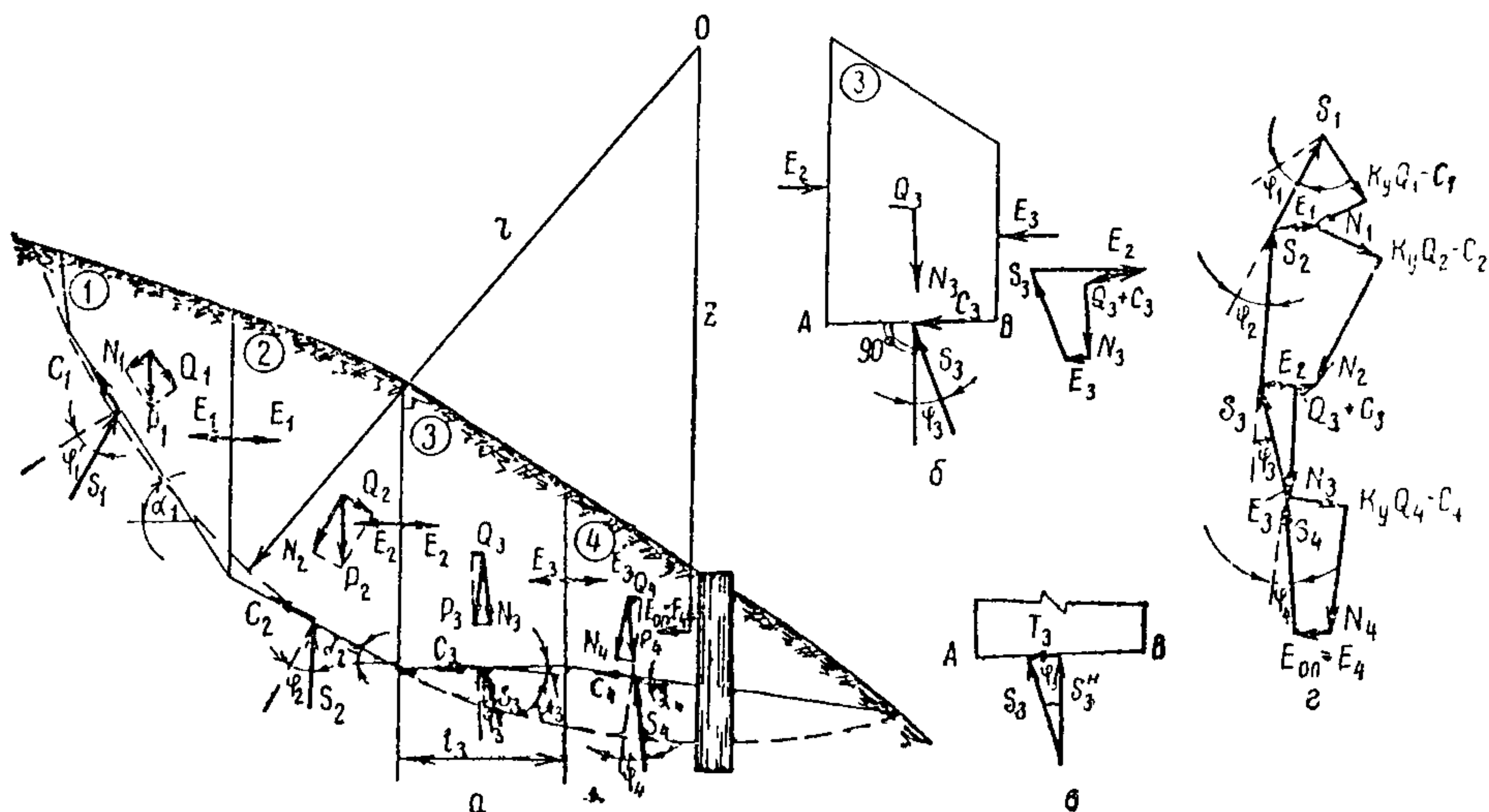
Рис. 11. Метод многоугольников сил:
