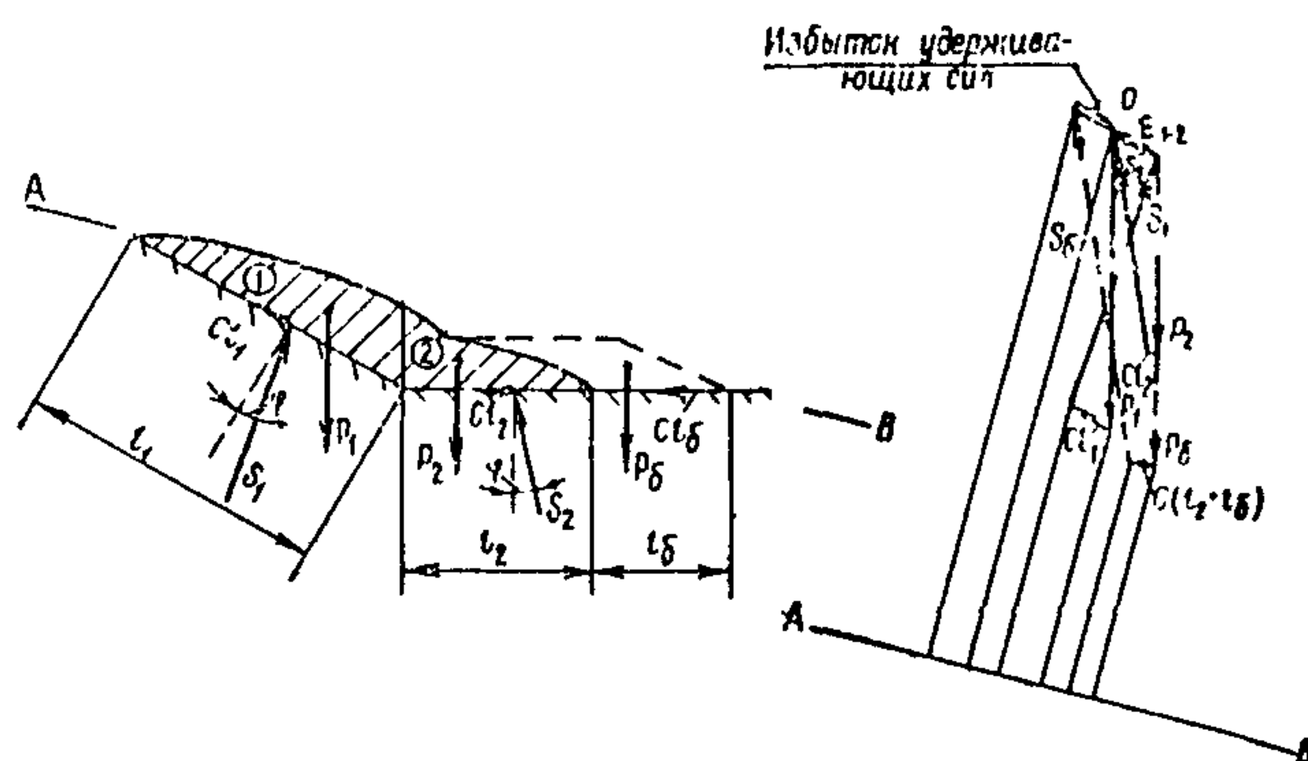
Рис. 16. Графостатический метод Л. Л. Перковского
