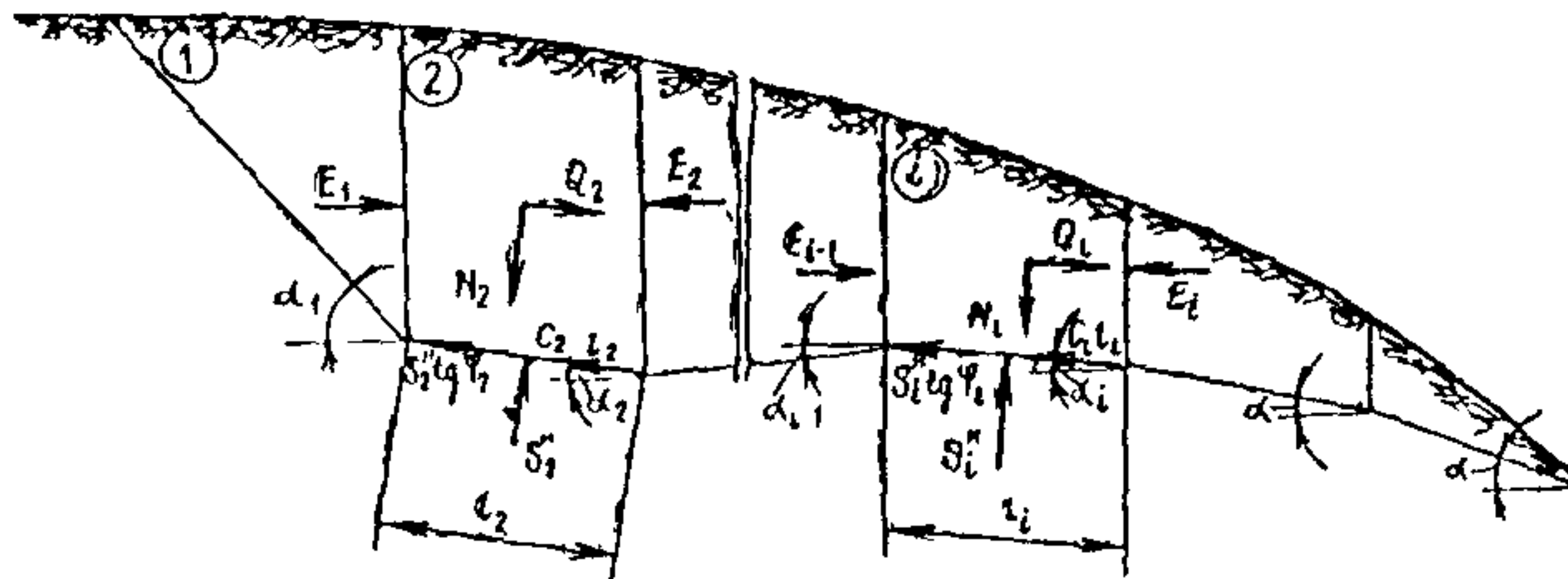
Рис. 10. Аналитический метод Г. М. Шахунянца
