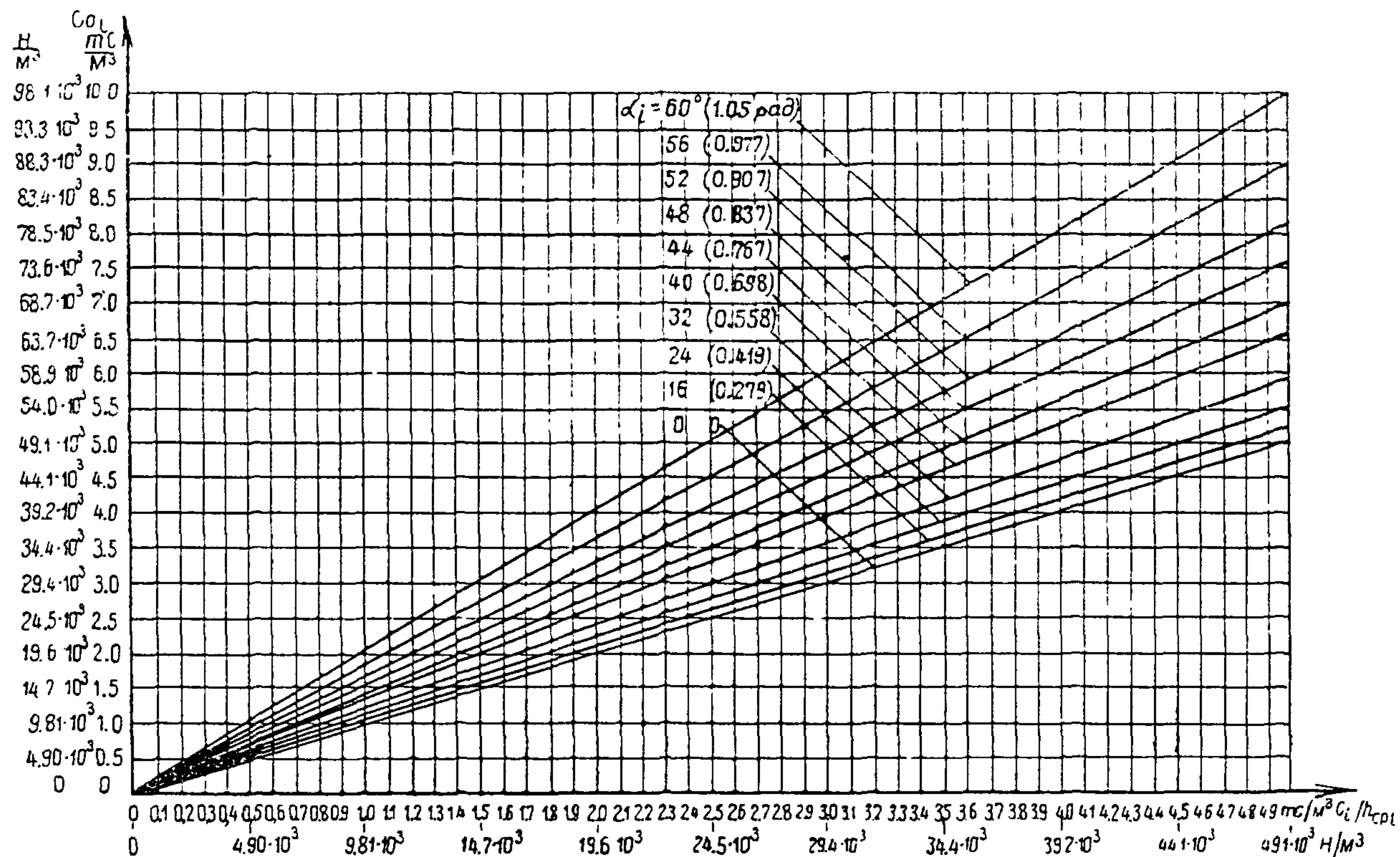
Рис. 14. Графики зависимости c_{oi} = \frac{c_i}{h_{cp, i} \cos \alpha_i}
