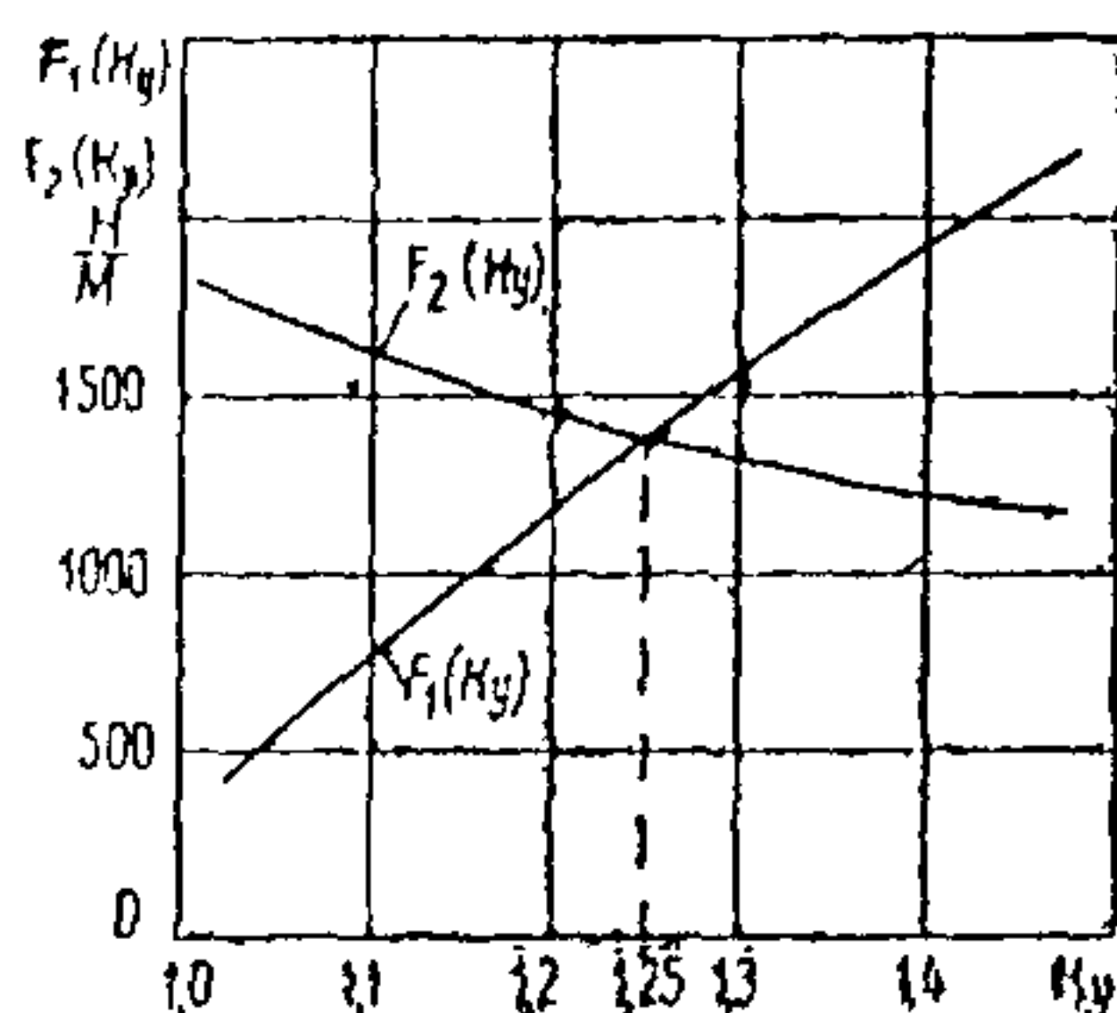
Рис. 7. Определение K_y методом Р. Р. Чугаева
