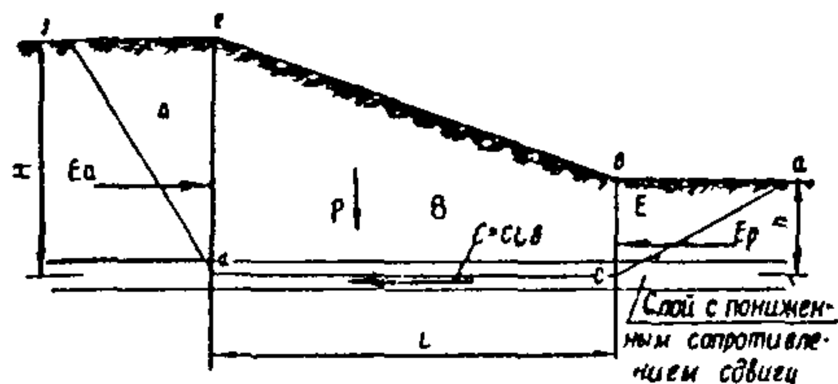
Рис. 17. Метод блока и призм (расчетная схема)
