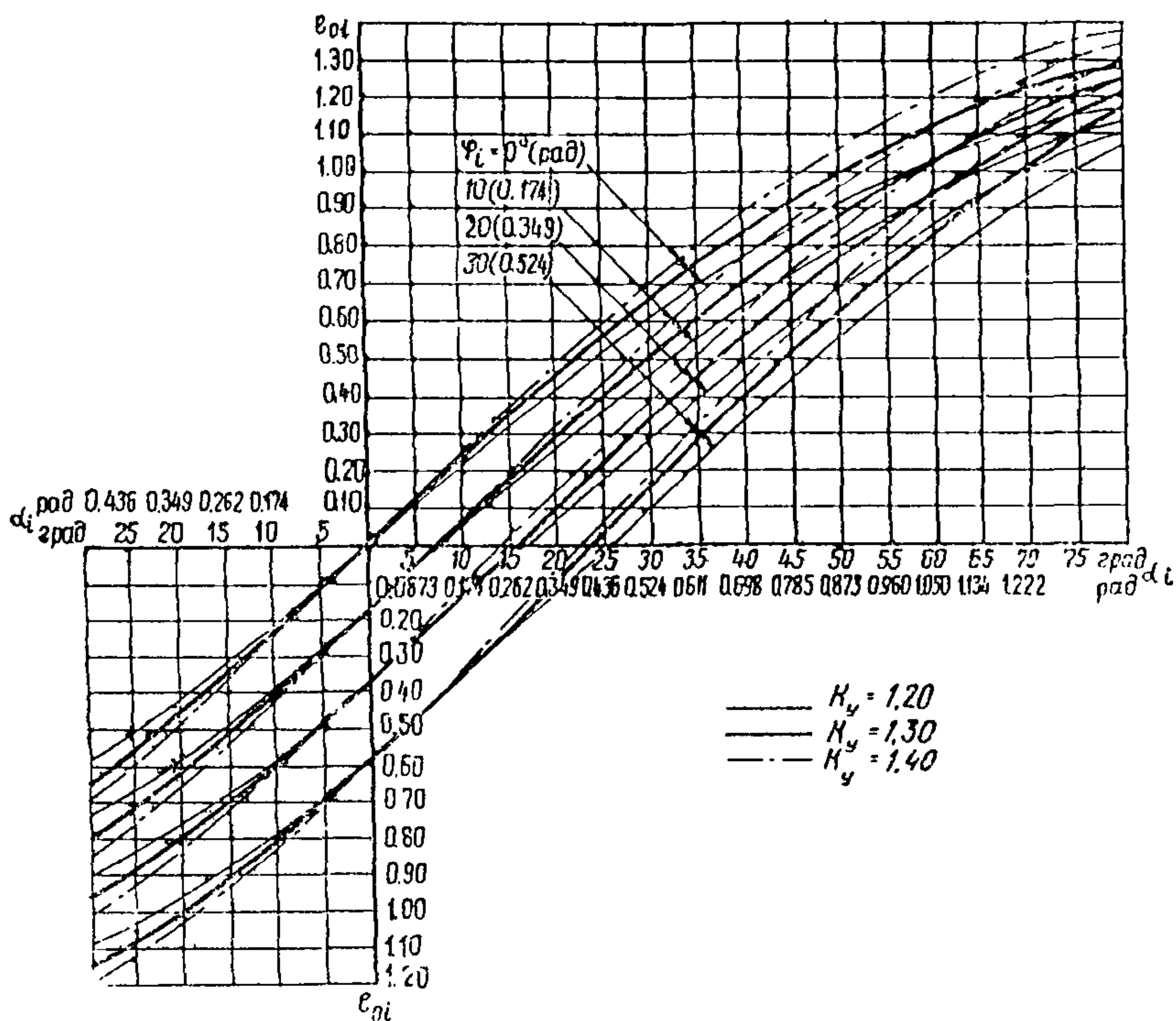
Рис. 13. Графики зависимости e_{oi} = K_y^3 \sin \alpha_i - \cos \alpha_i \tan \varphi_i
