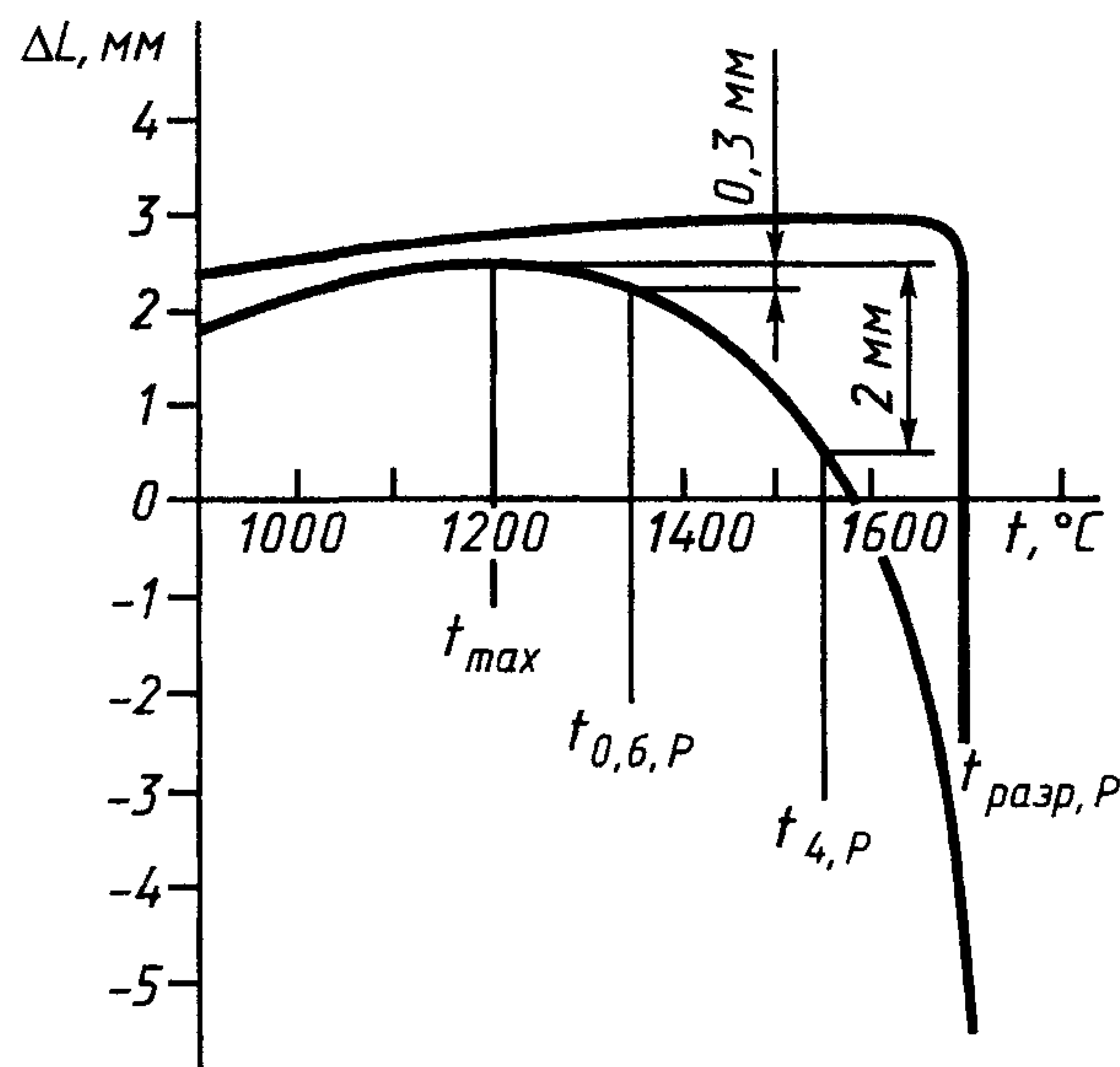
Рисунок 1 — Диаграмма «температура — деформация»
