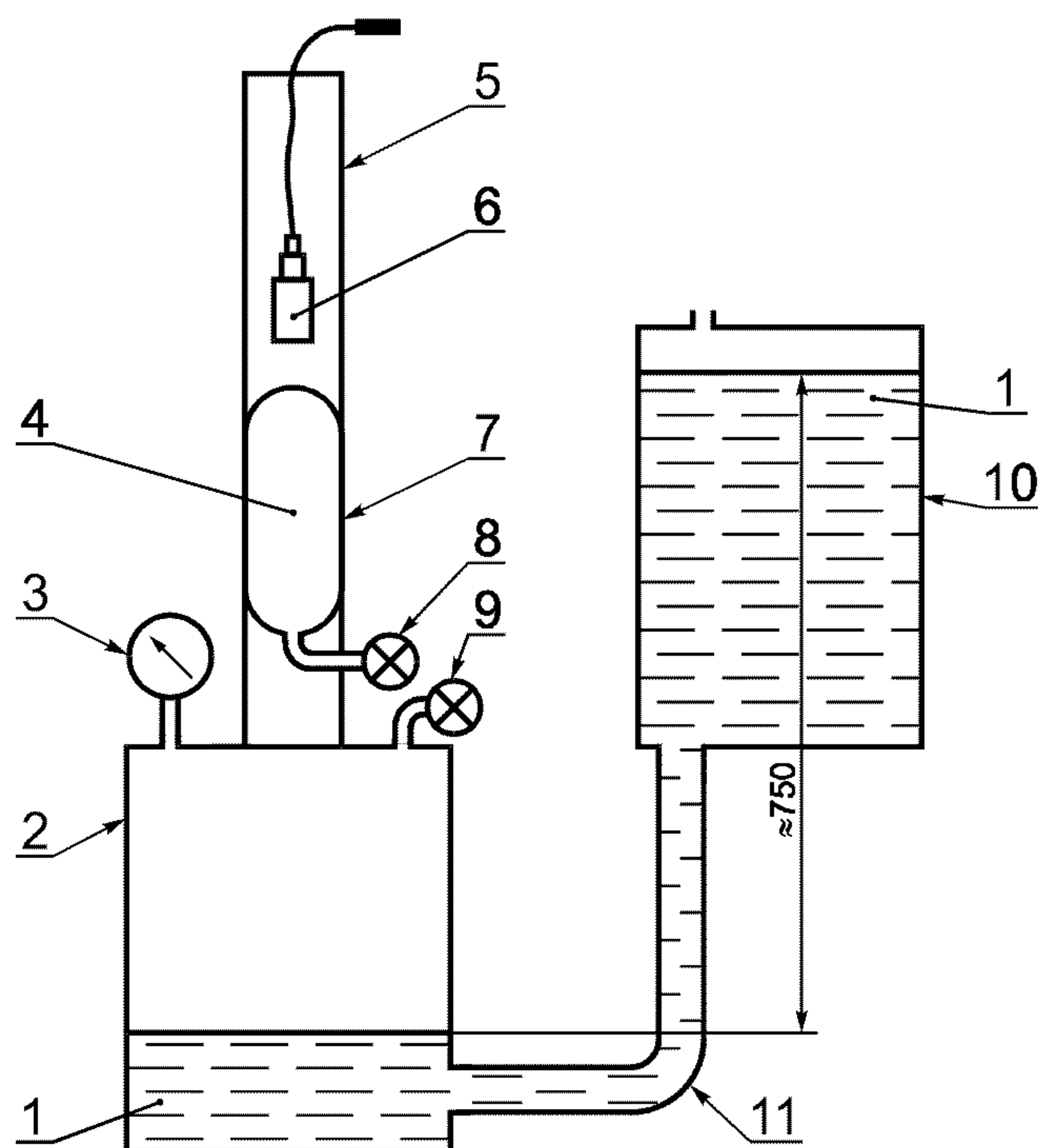
Рисунок В.6 — Схема установки, обеспечивающей скачкообразный переход из чистого воздуха в газозвушную смесь
