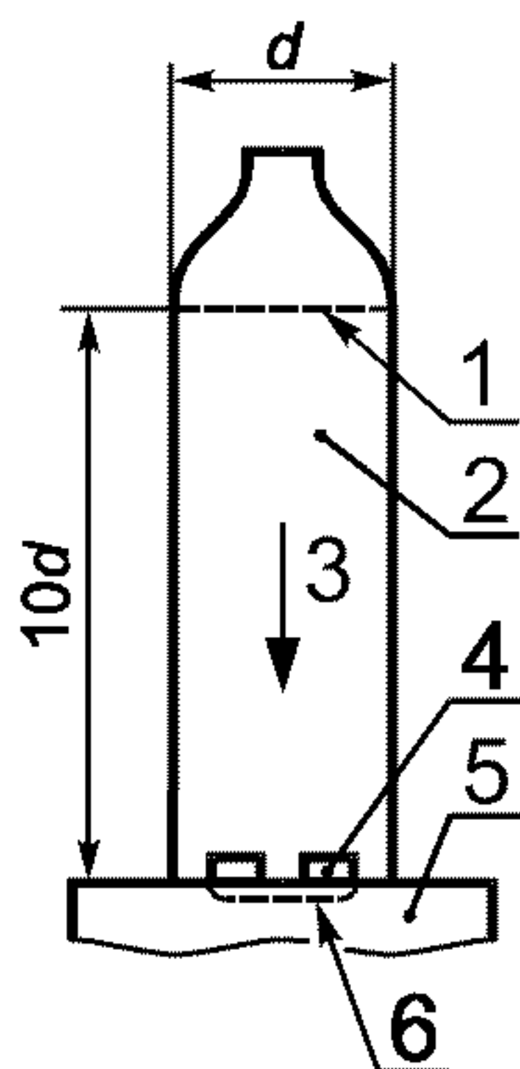
Рисунок В.4 — Схема, показывающая аппликатор и входное отверстие прибора (датчика) во время подачи ПГС или чистого воздуха (см. В.2.2)
