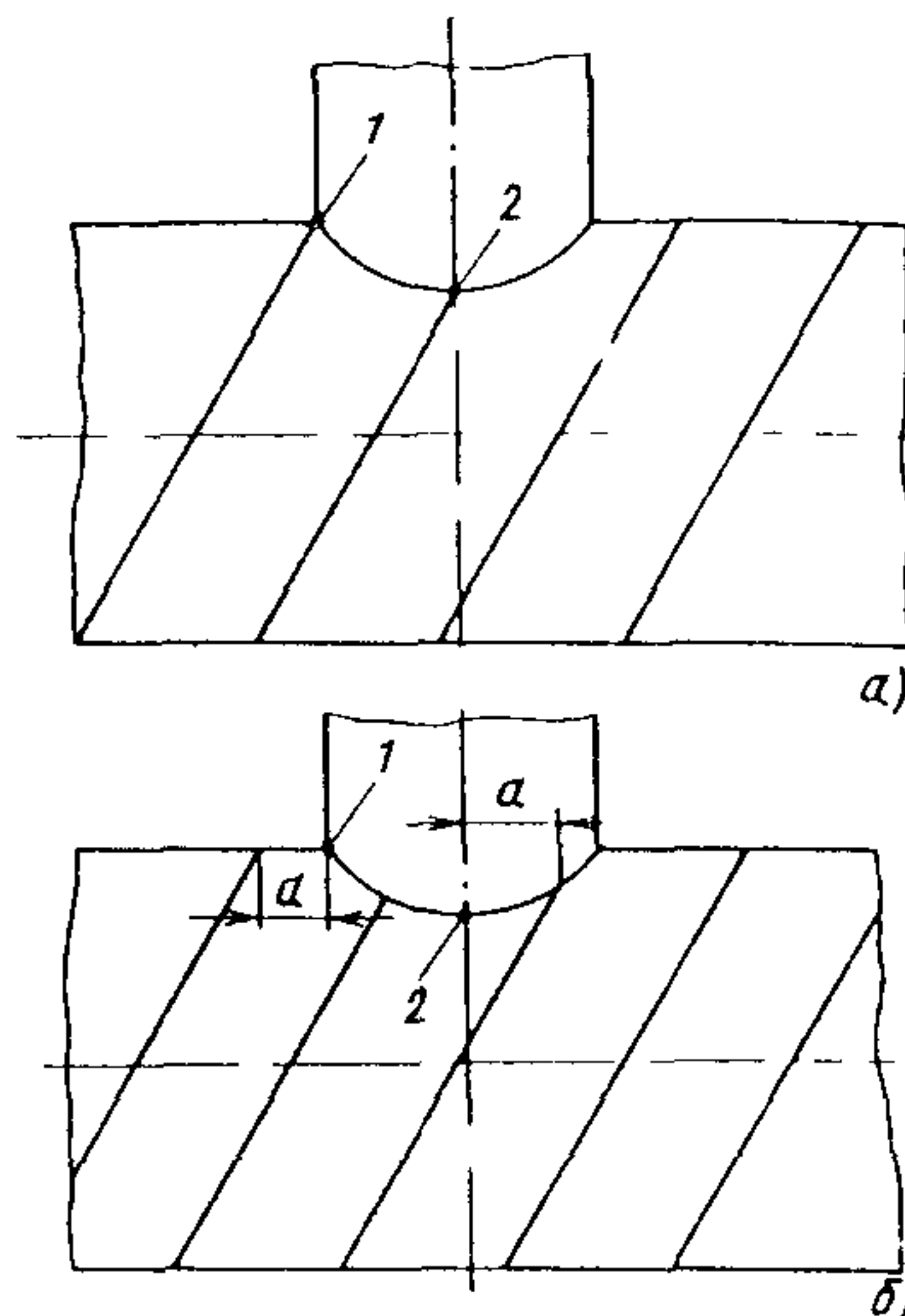
Рис. 17. Вварка штуцеров в трубопроводы со спиральными швами:
