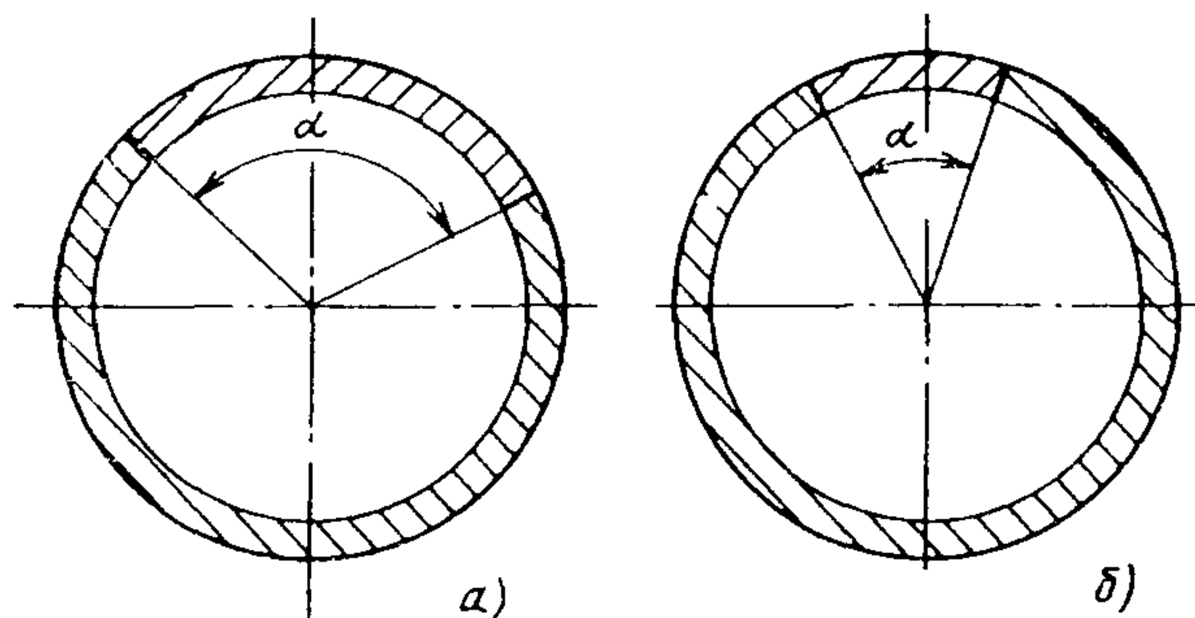
Рис. 7. Труба, изготовленная из двух секторов:
