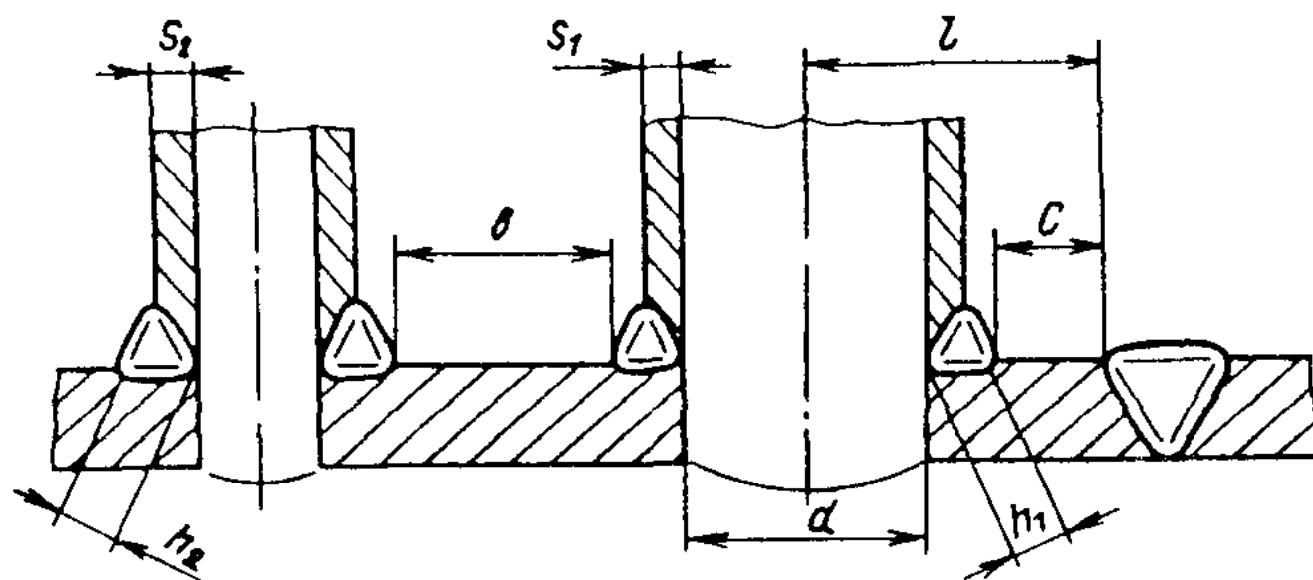
Рис. 13. Расположение сварных швов приварки патрубков.
