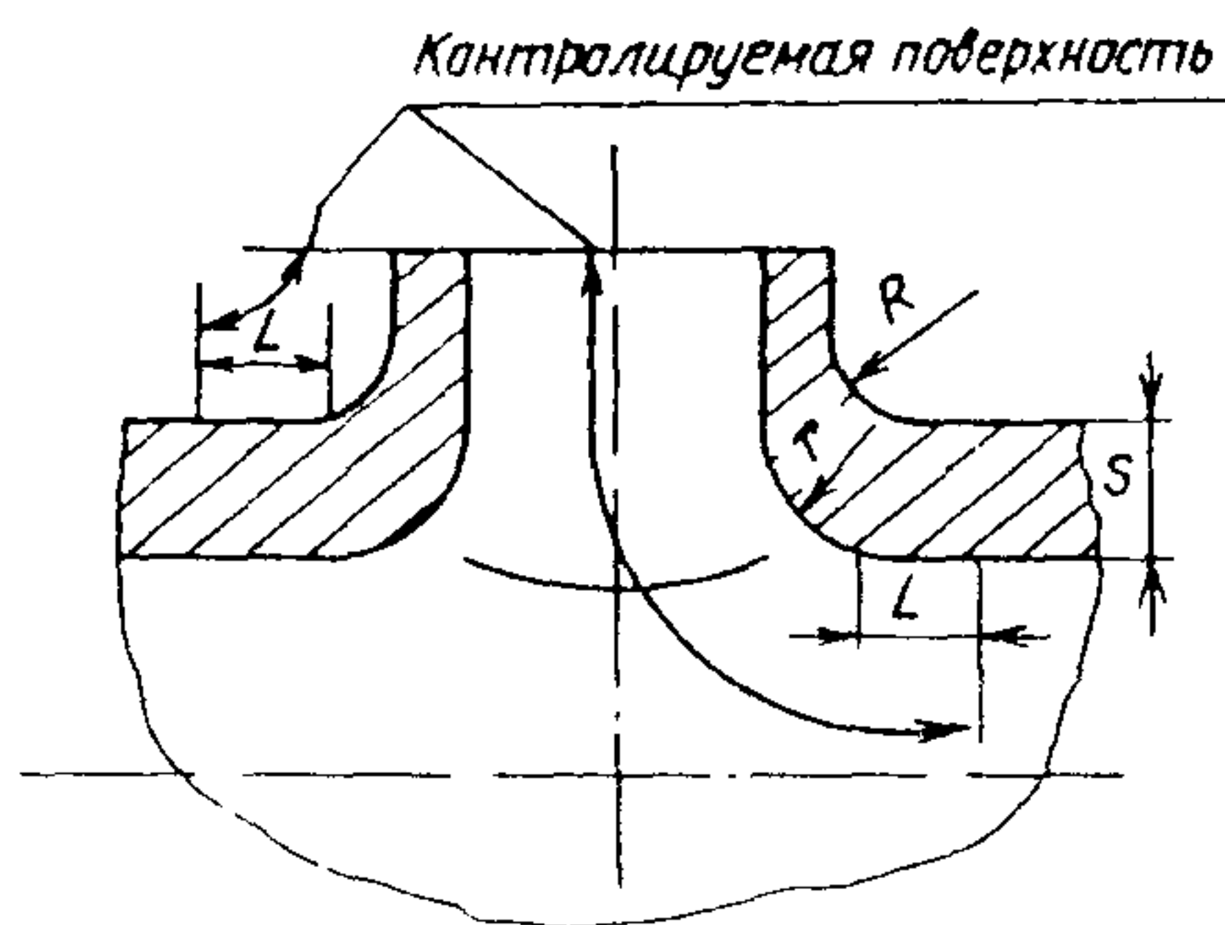
Рис. 18. Схема высаженной горловины ( L = 30 мм)
