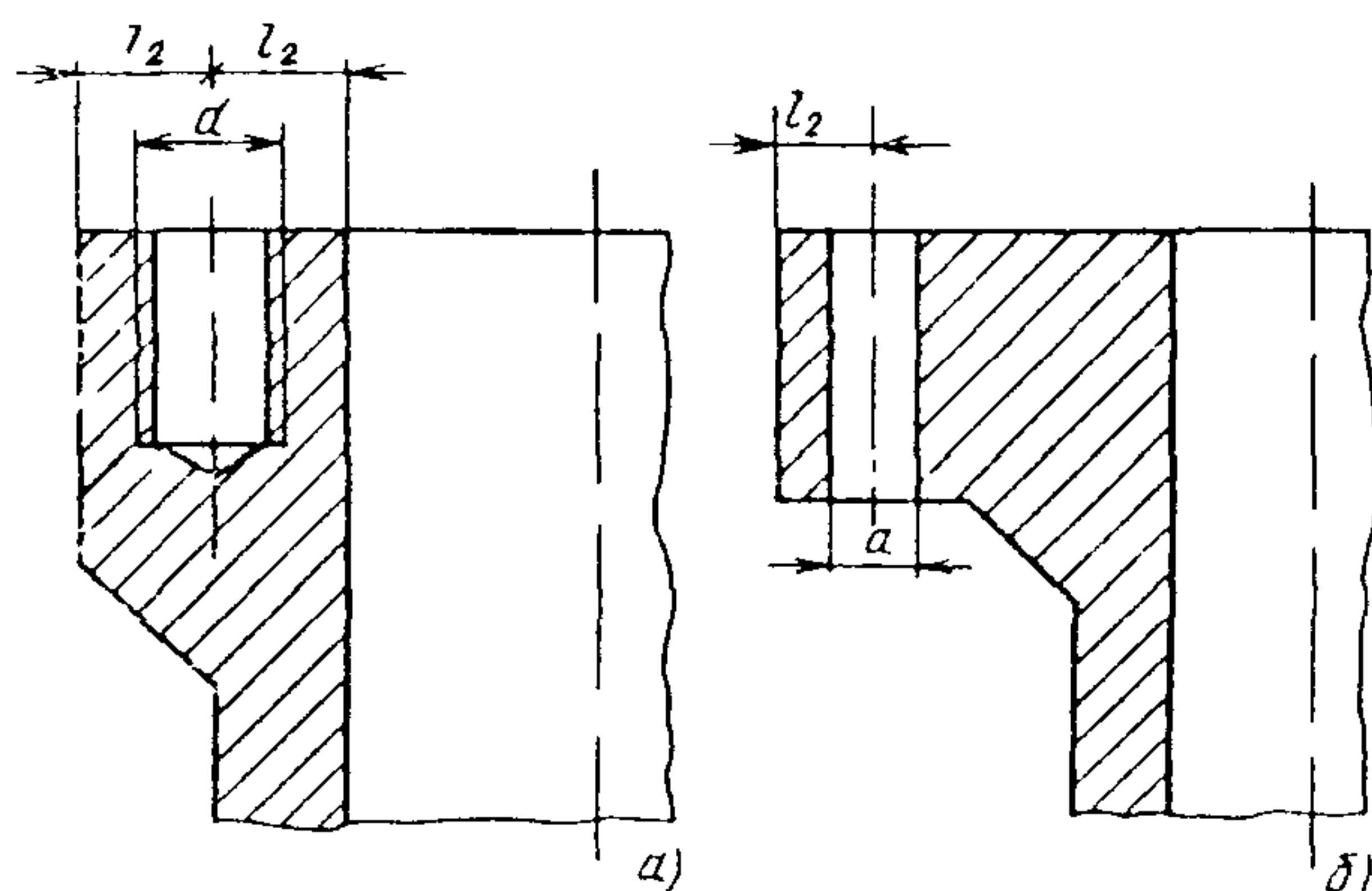
Рис. 5 Расположение отверстий под шпильки (а) и болты (б) ( l_2 \geq 0,85d )
