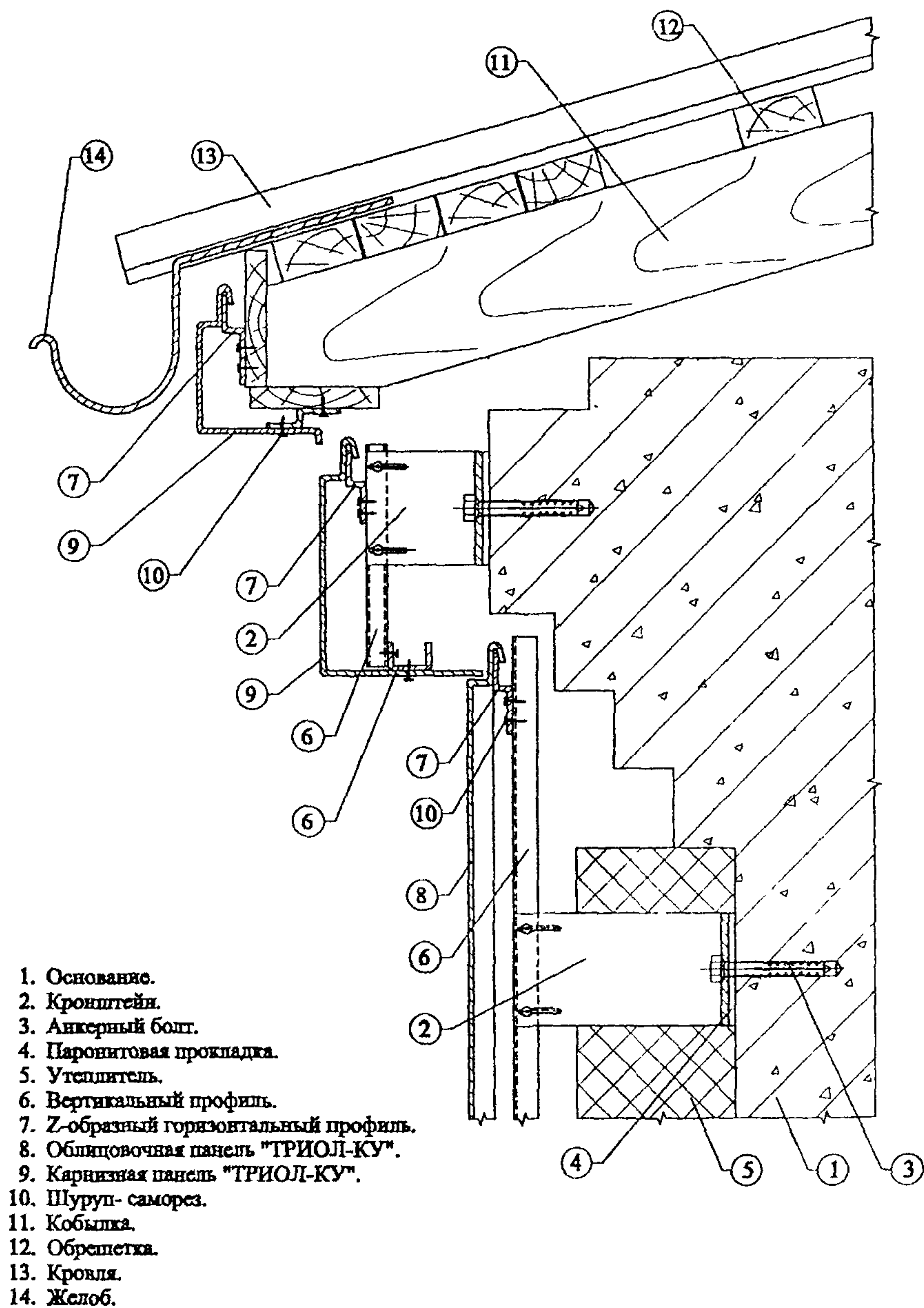
Рис. 3.19 Фасадная система "ТРИОЛ-КУ" у карниза.
