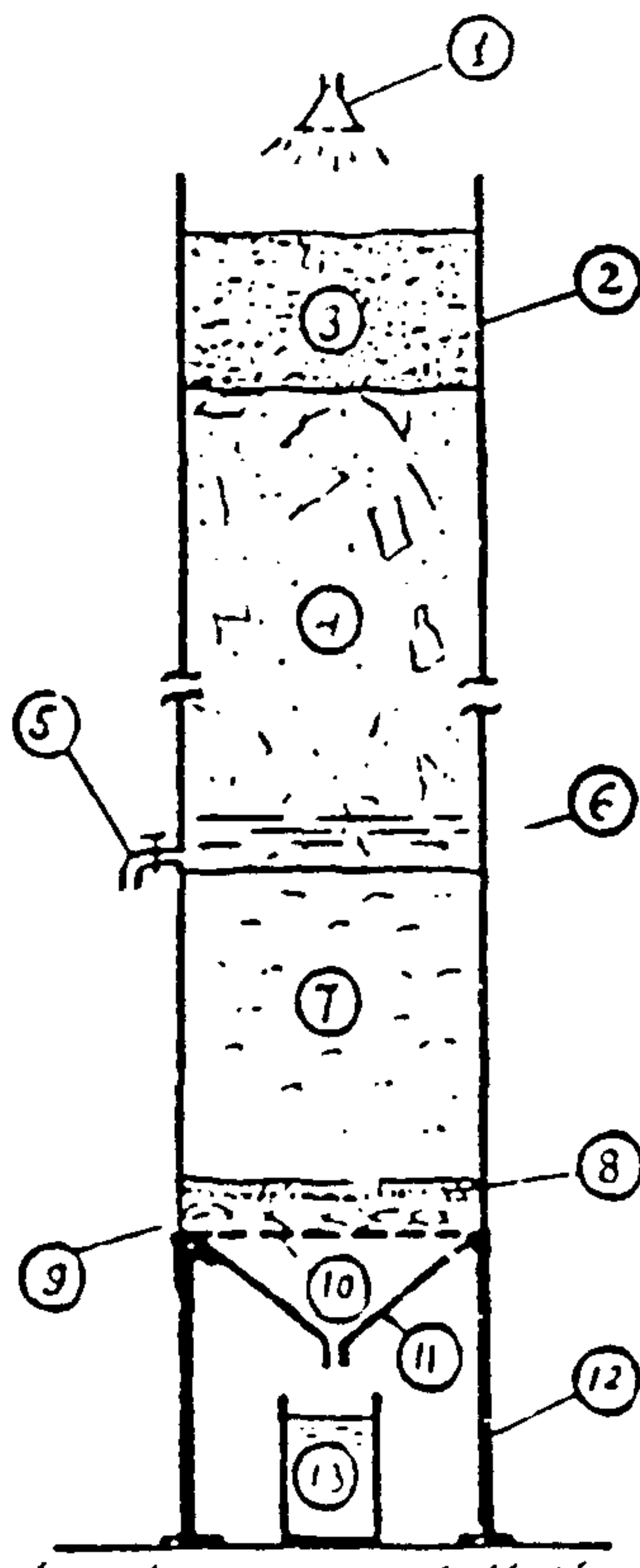
Схема модели полигона твердых бытовых отходов:
