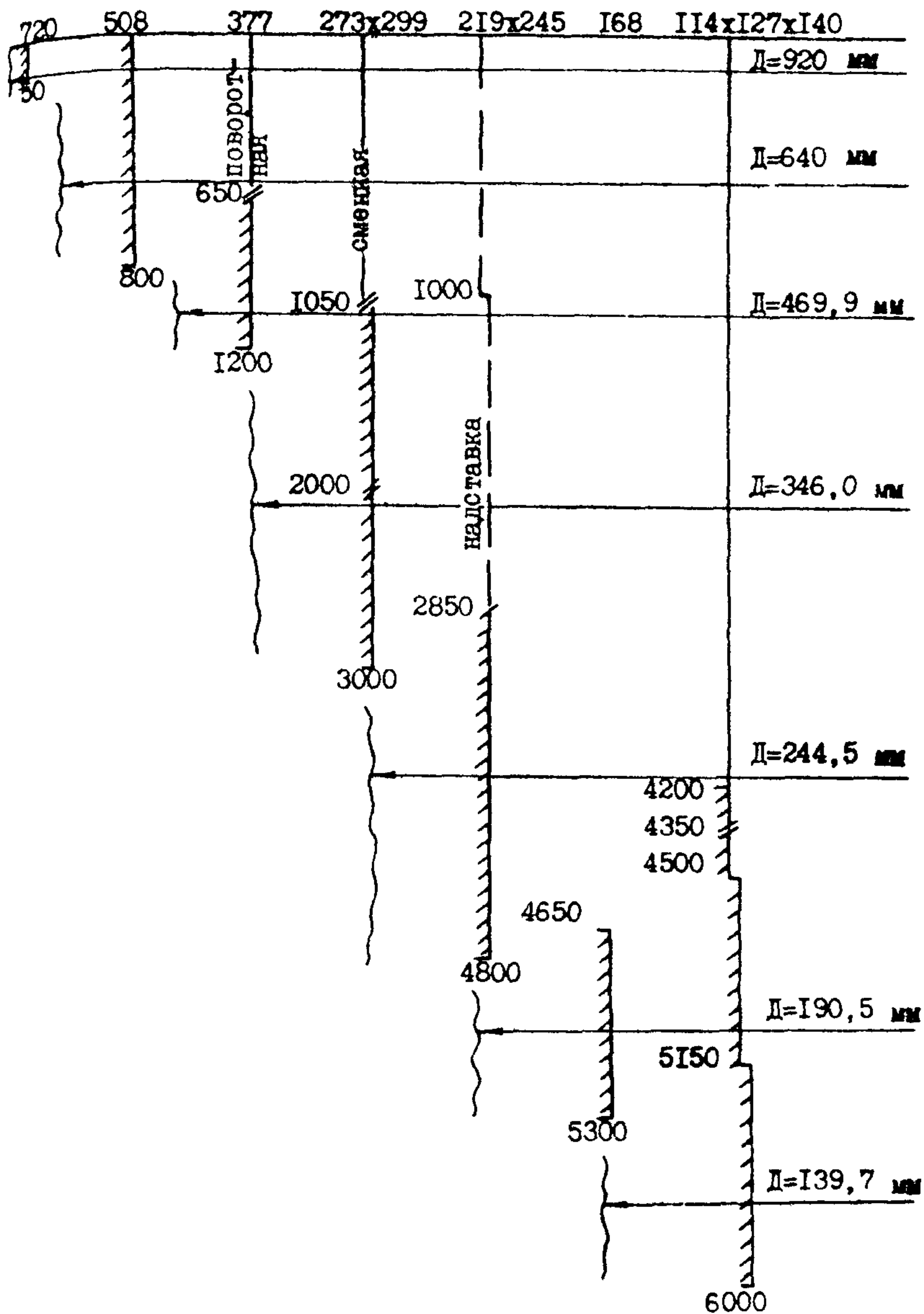
Рис.1. Конструкция скважины (к примеру заполнения табл. 5.2 и 5.3).
