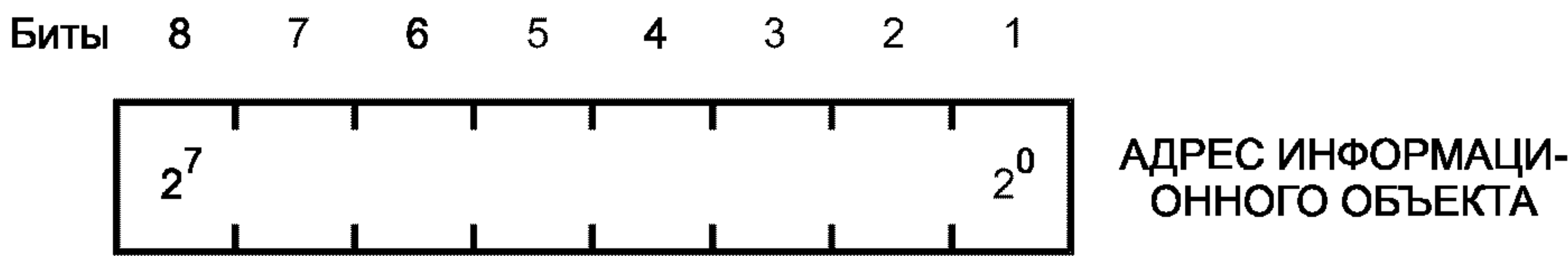
Рисунок 9 — АДРЕС ИНФОРМАЦИОННОГО ОБЪЕКТА (один байт)
