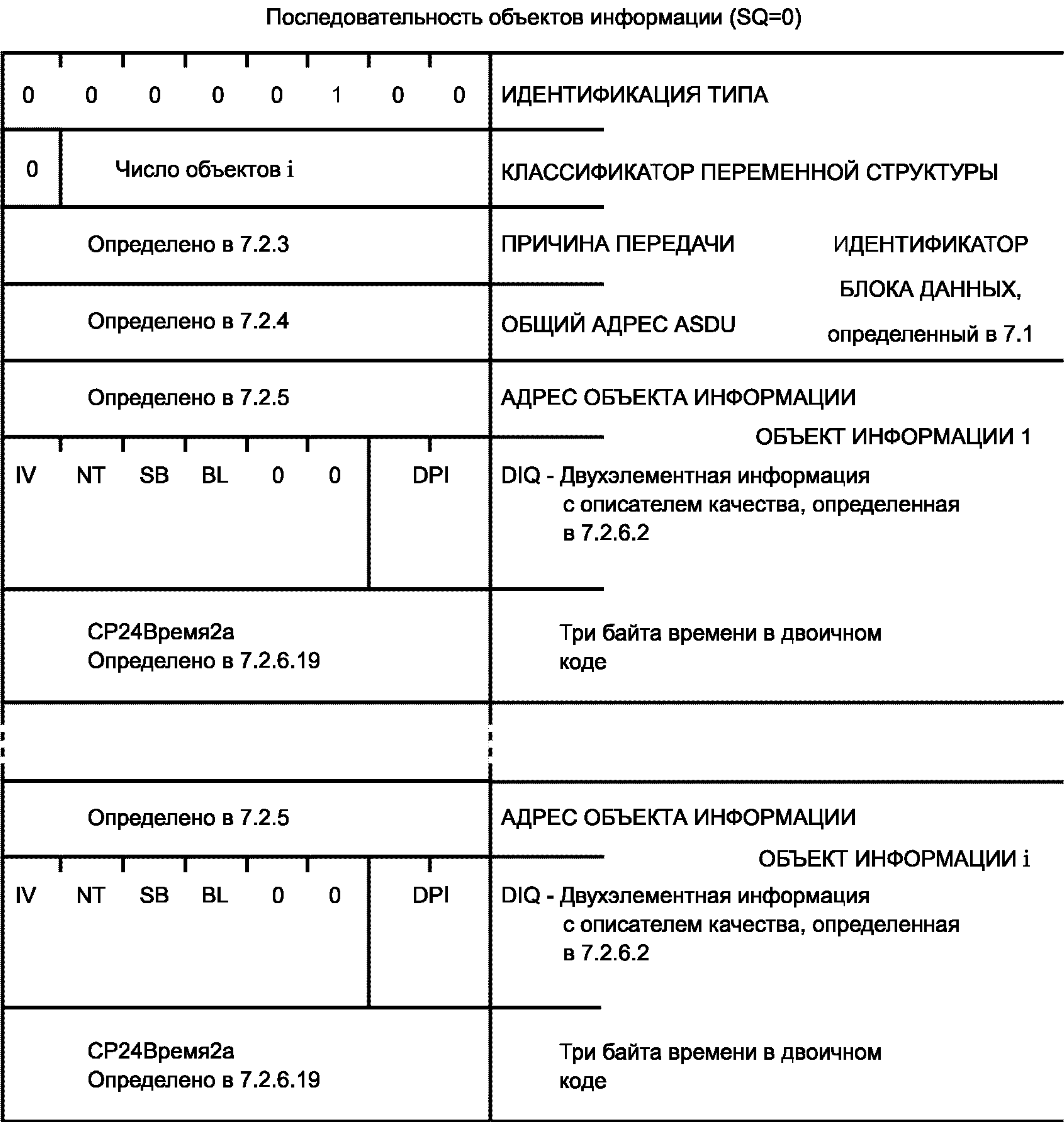
Рисунок 17 — ASDU. M_DP_TA_1. Двухэлементная информация с меткой времени
