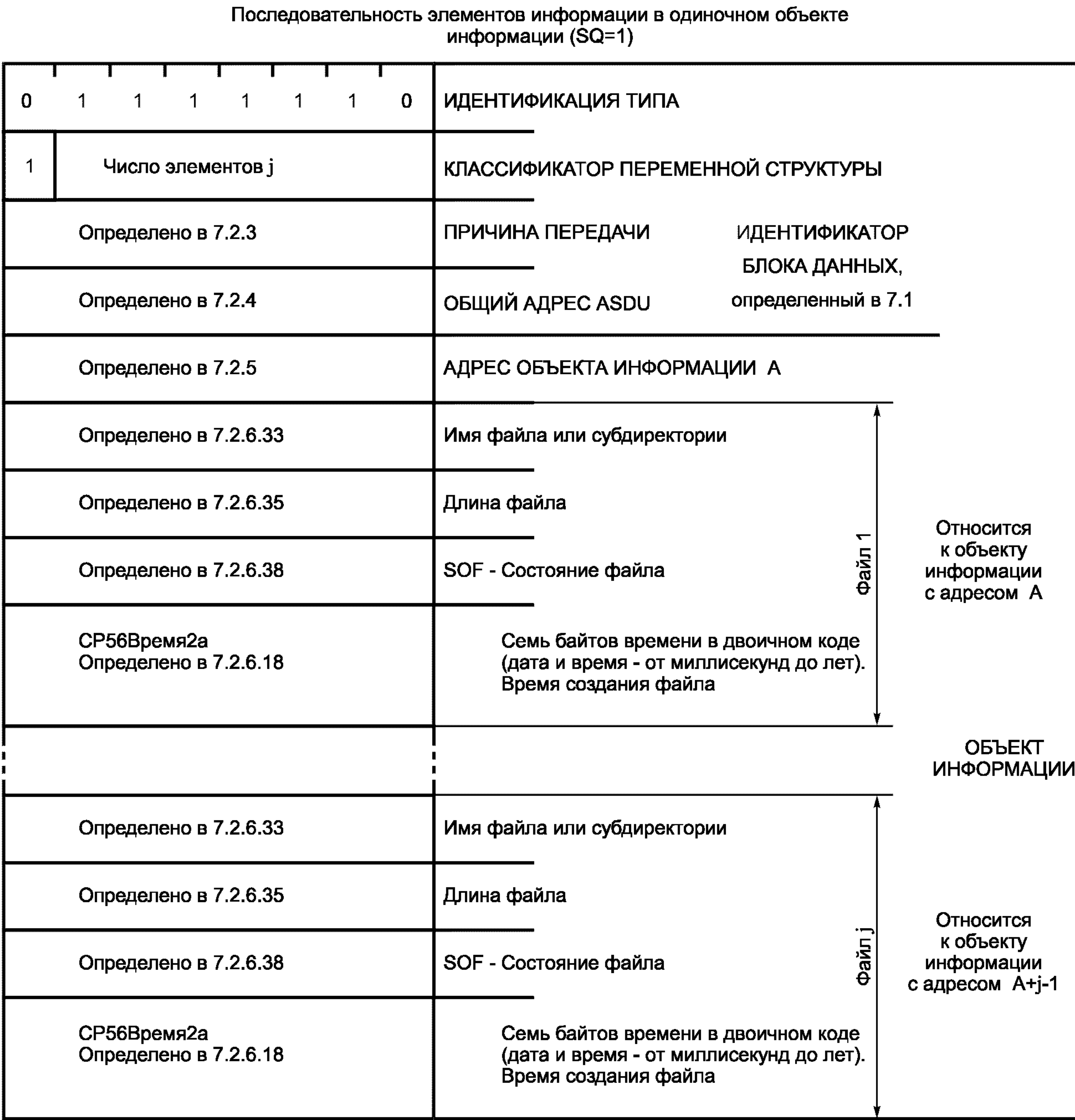
Рисунок 63 — ASDU. F_DR_TA_1. Директория
