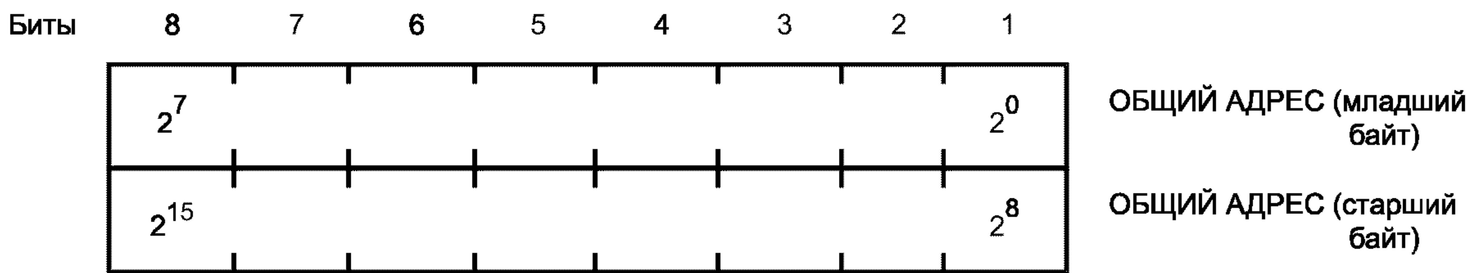
Рисунок 8 — ОБЩИЙ АДРЕС ASDU (два байта)
