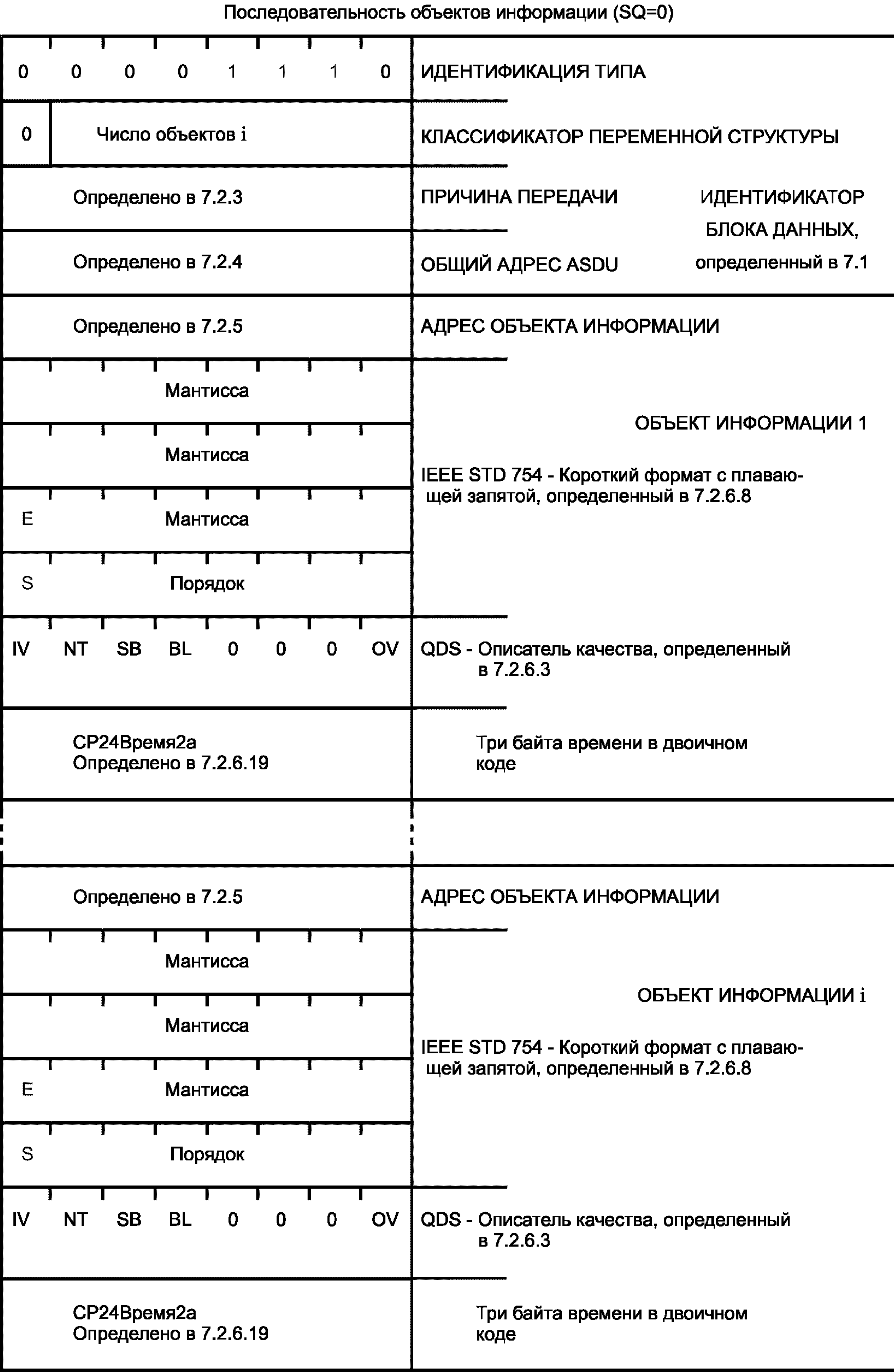
Рисунок 29 — ASDU. M_ME_TC_1. Значение измеряемой величины, короткий формат с плавающей запятой с меткой времени
