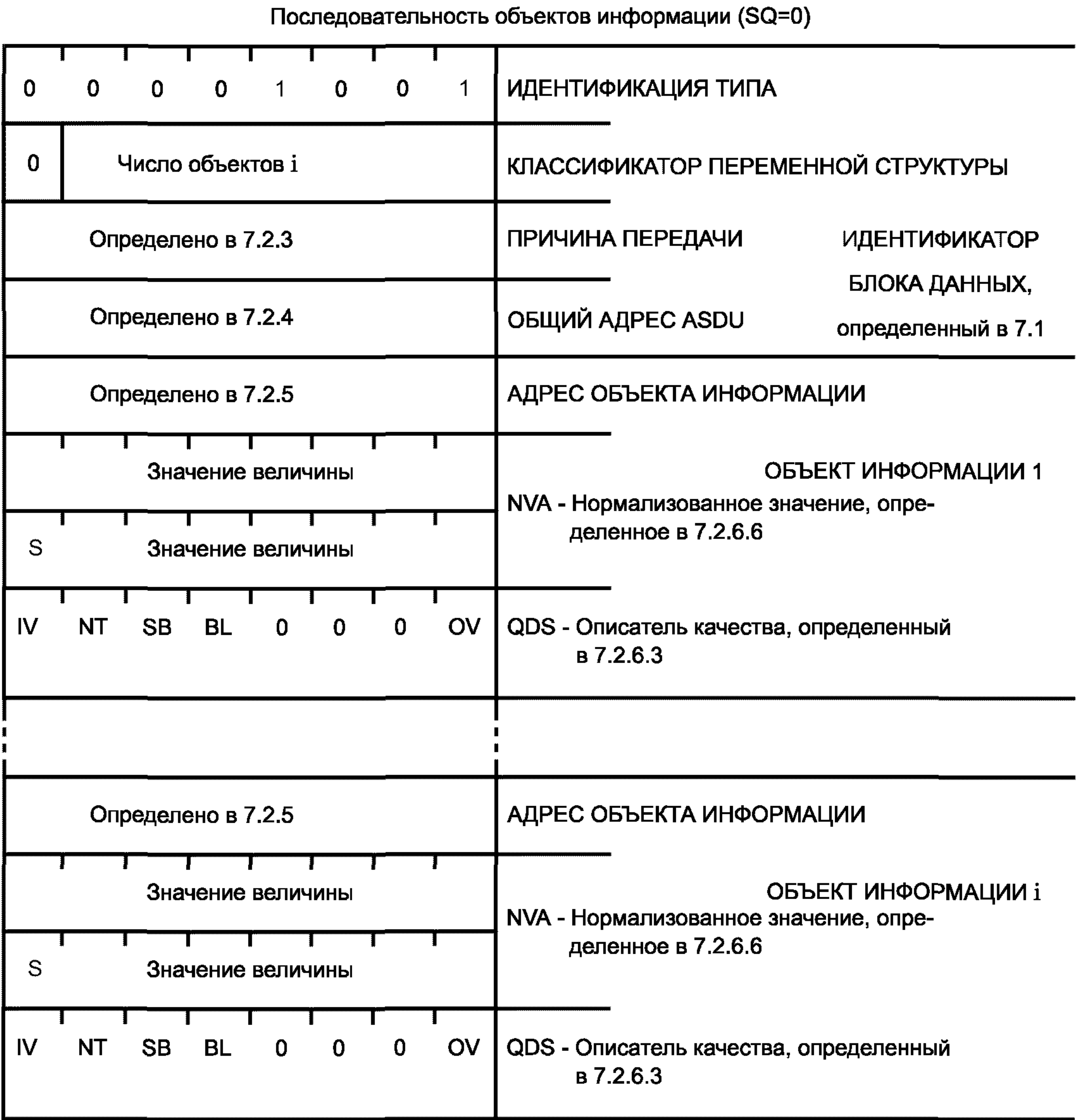
Рисунок 22 — ASDU. M_ME_NA_1. Значение измеряемой величины, нормализованное значение
