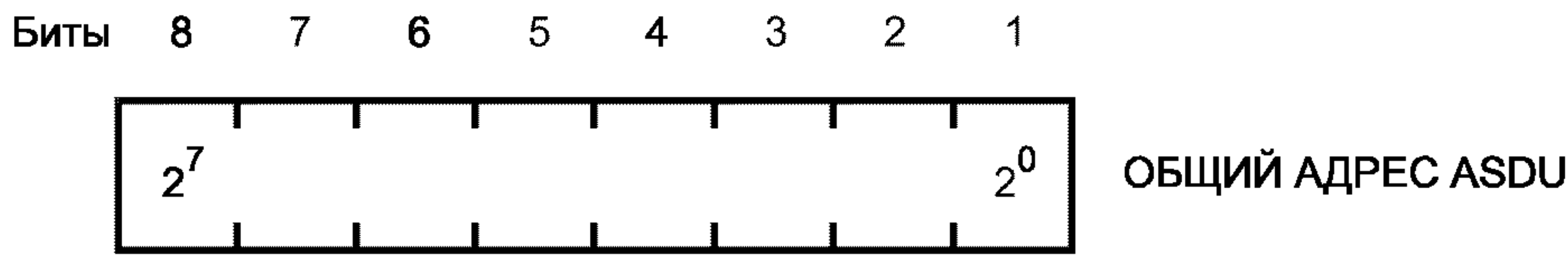
Рисунок 7 — ОБЩИЙ АДРЕС ASDU (один байт)
