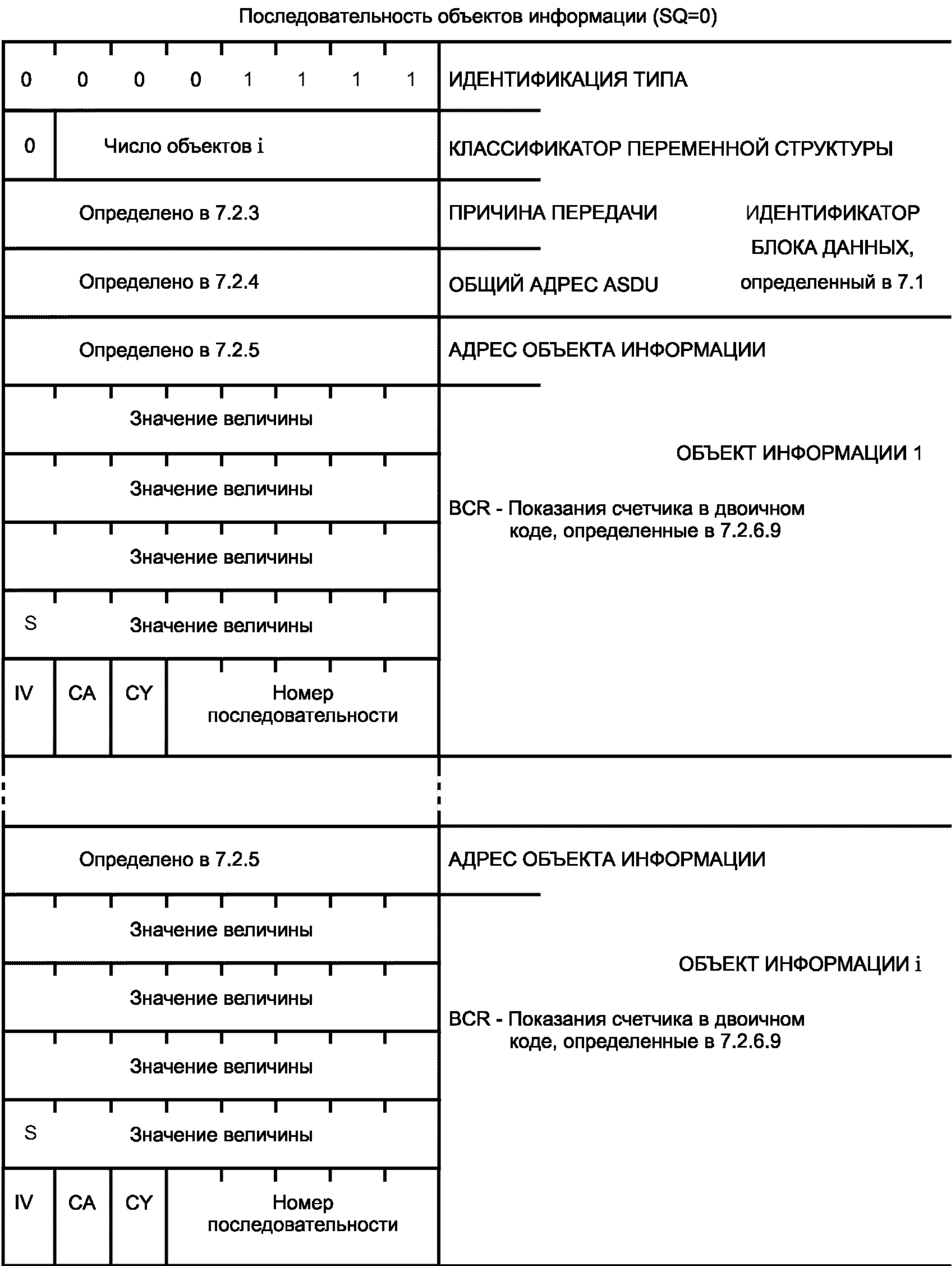
Рисунок 30 — ASDU. M_IT_NA_1. Интегральные суммы
