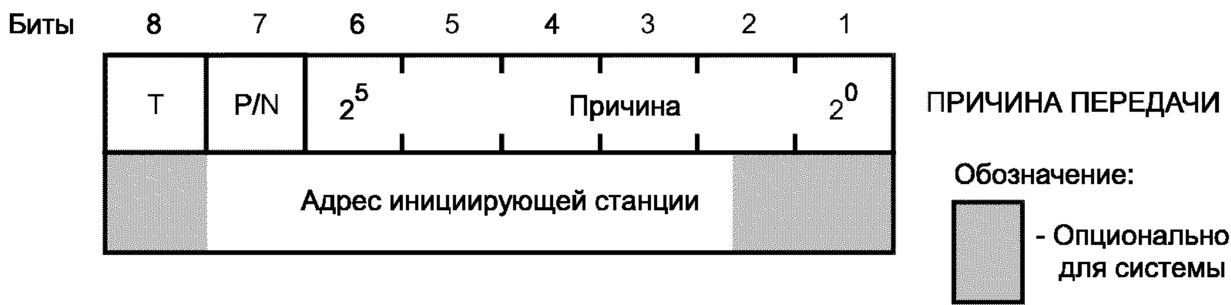
Рисунок 6 — Поле ПРИЧИНЫ ПЕРЕДАЧИ
