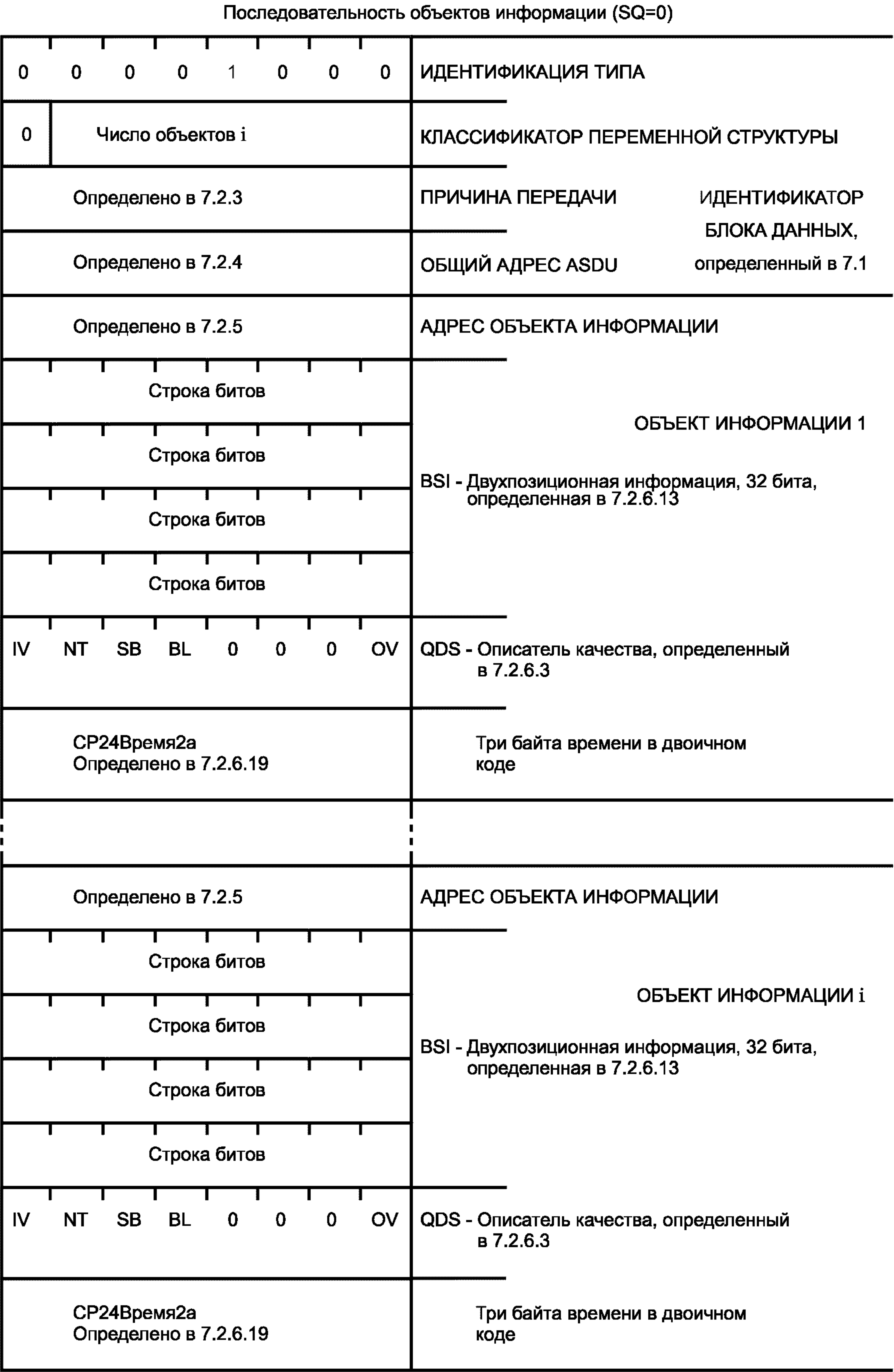
Рисунок 21 — ASDU. M_BO_TA_1. Строка из 32 битов с меткой времени
