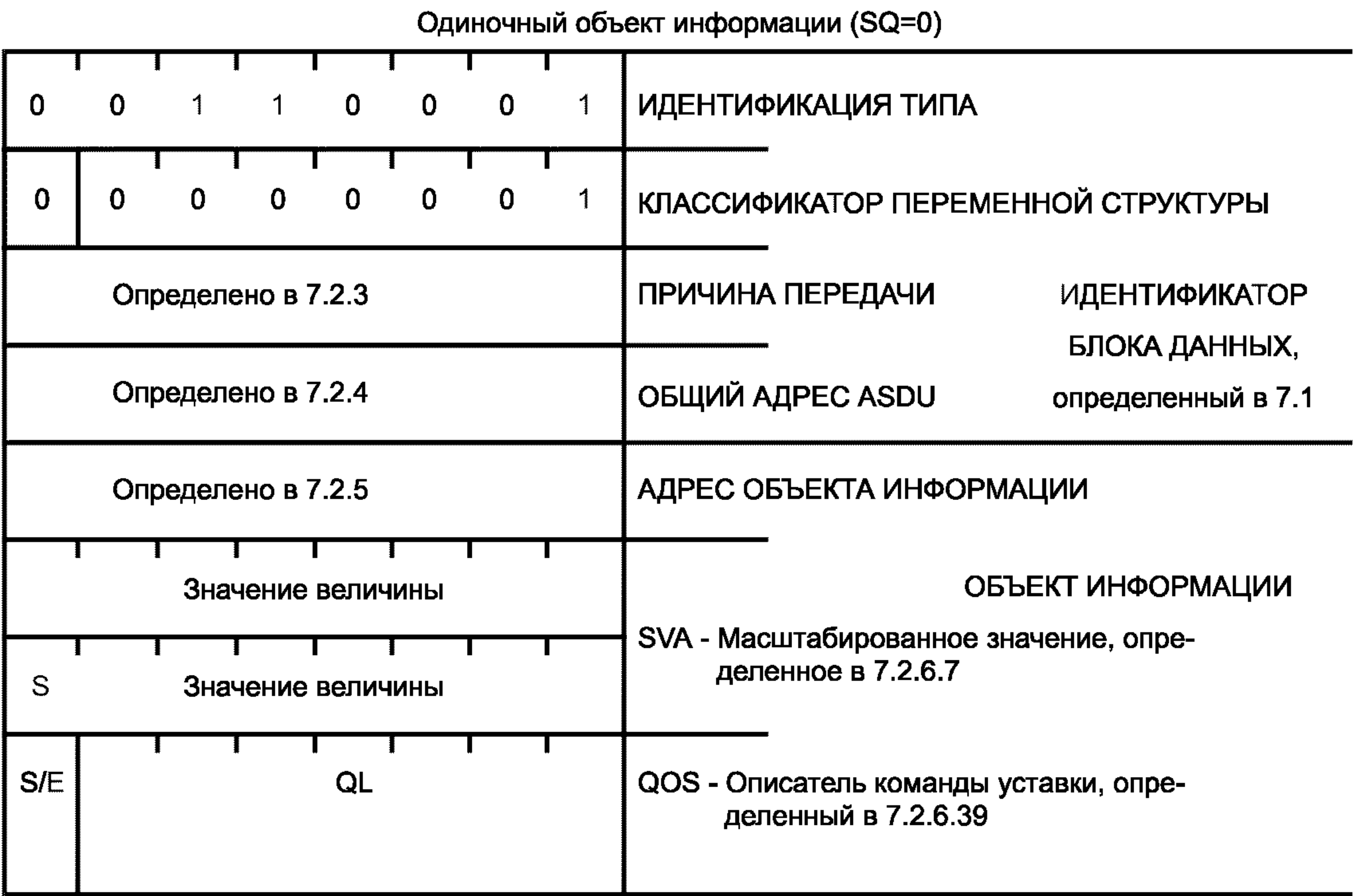
Рисунок 42 — ASDU. C_SE_NB_1. Команда уставки, масштабированное значение
