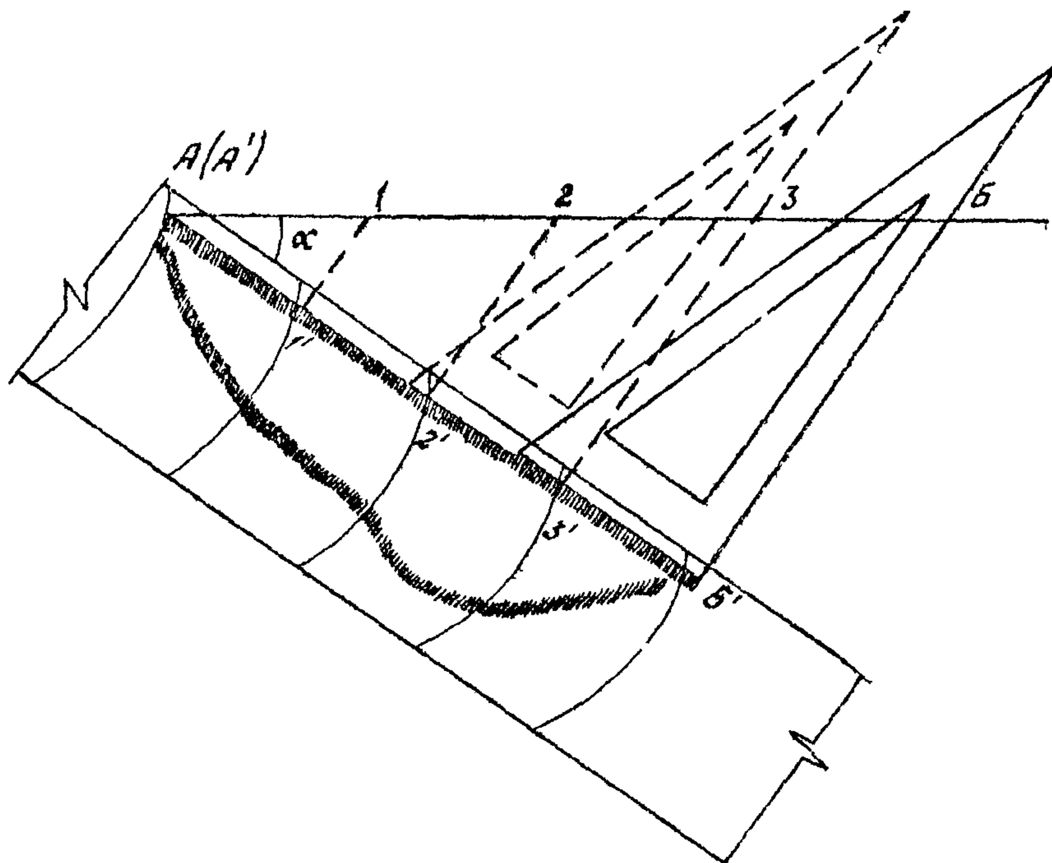
Рис. 8. Перенос отметок на план способом треугольника
