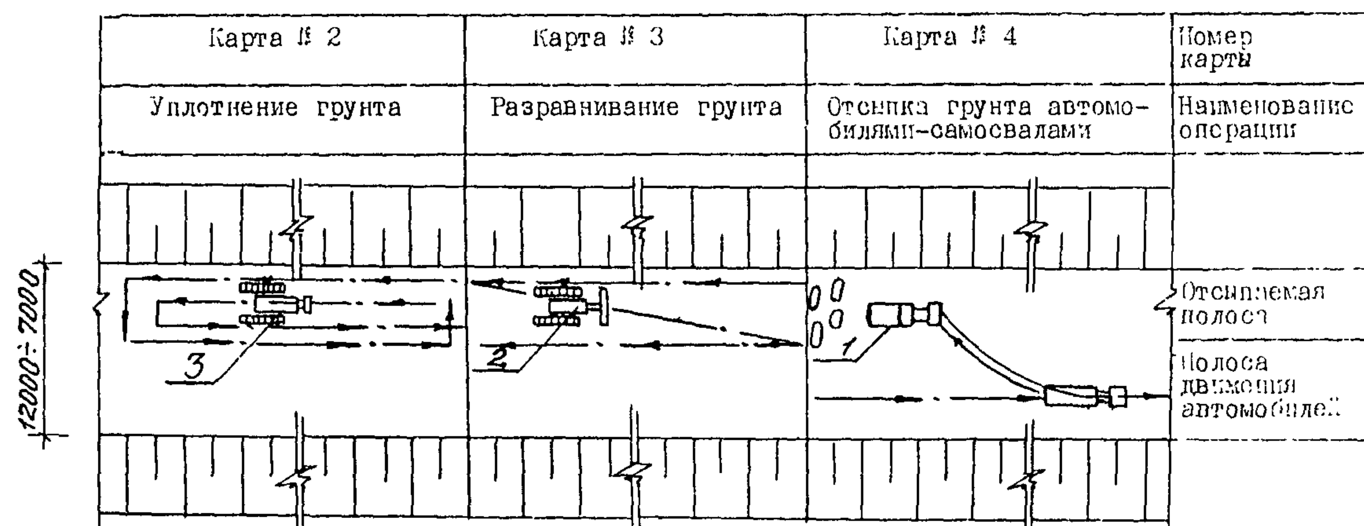
СХЕМА ОТСЫПКИ ВЕРХНЕЙ ЧАСТИ ДАМБЫ
