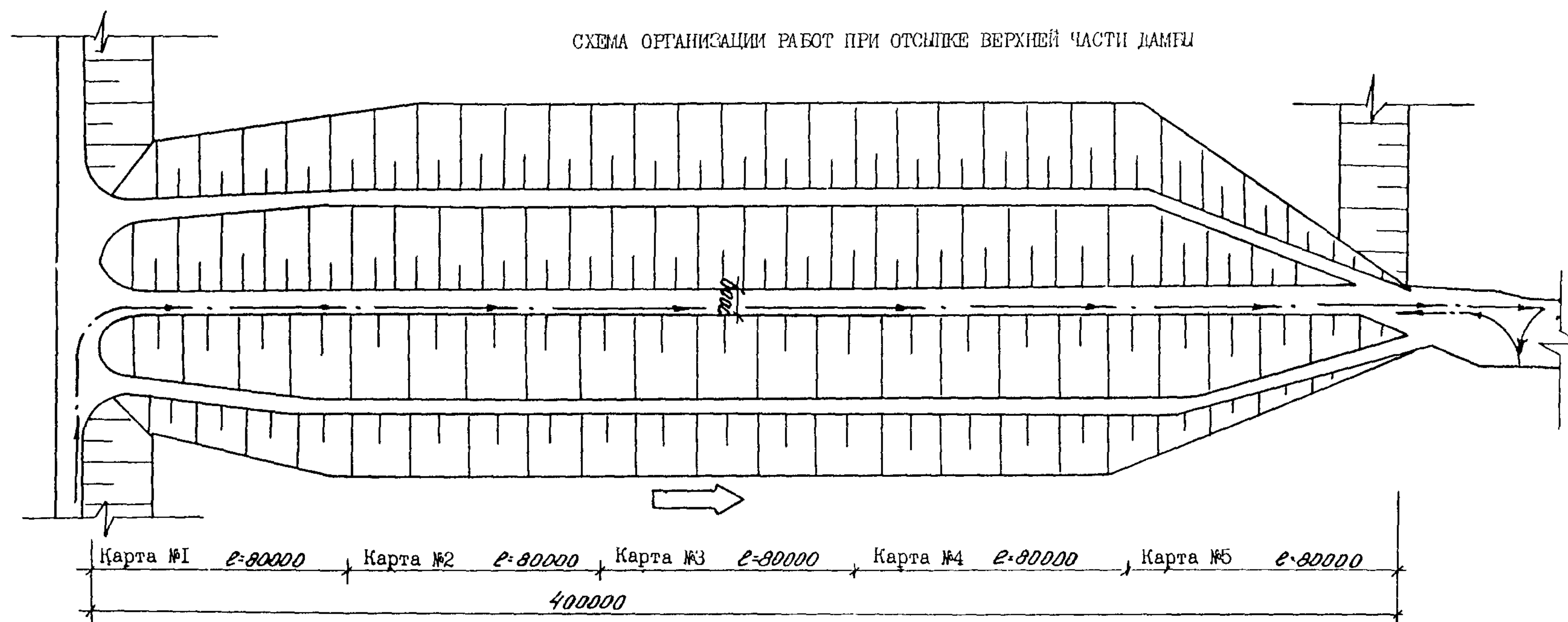
СХЕМА ОТСЫПКИ ВЕРХНЕЙ ЧАСТИ ДАМБЫ
