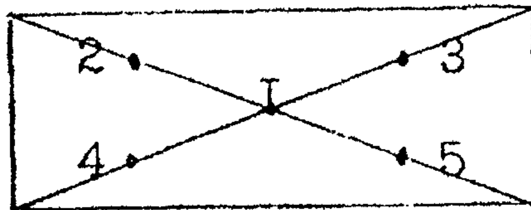
Схема отбора пробы в длинном помещении
