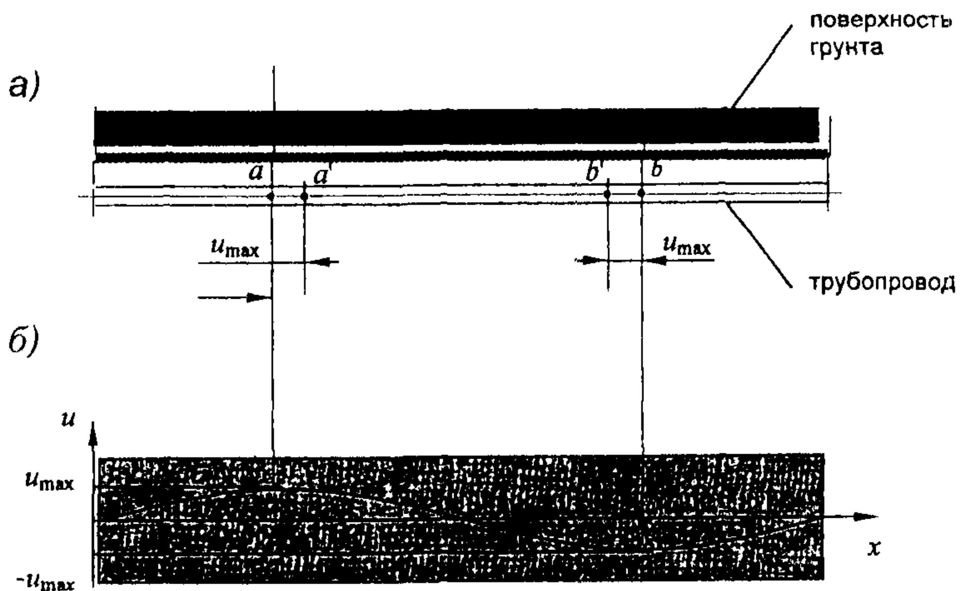
Рис. П.6.1. Деформации линейно-протяженной конструкции при прохождении продольной сейсмической волны:
