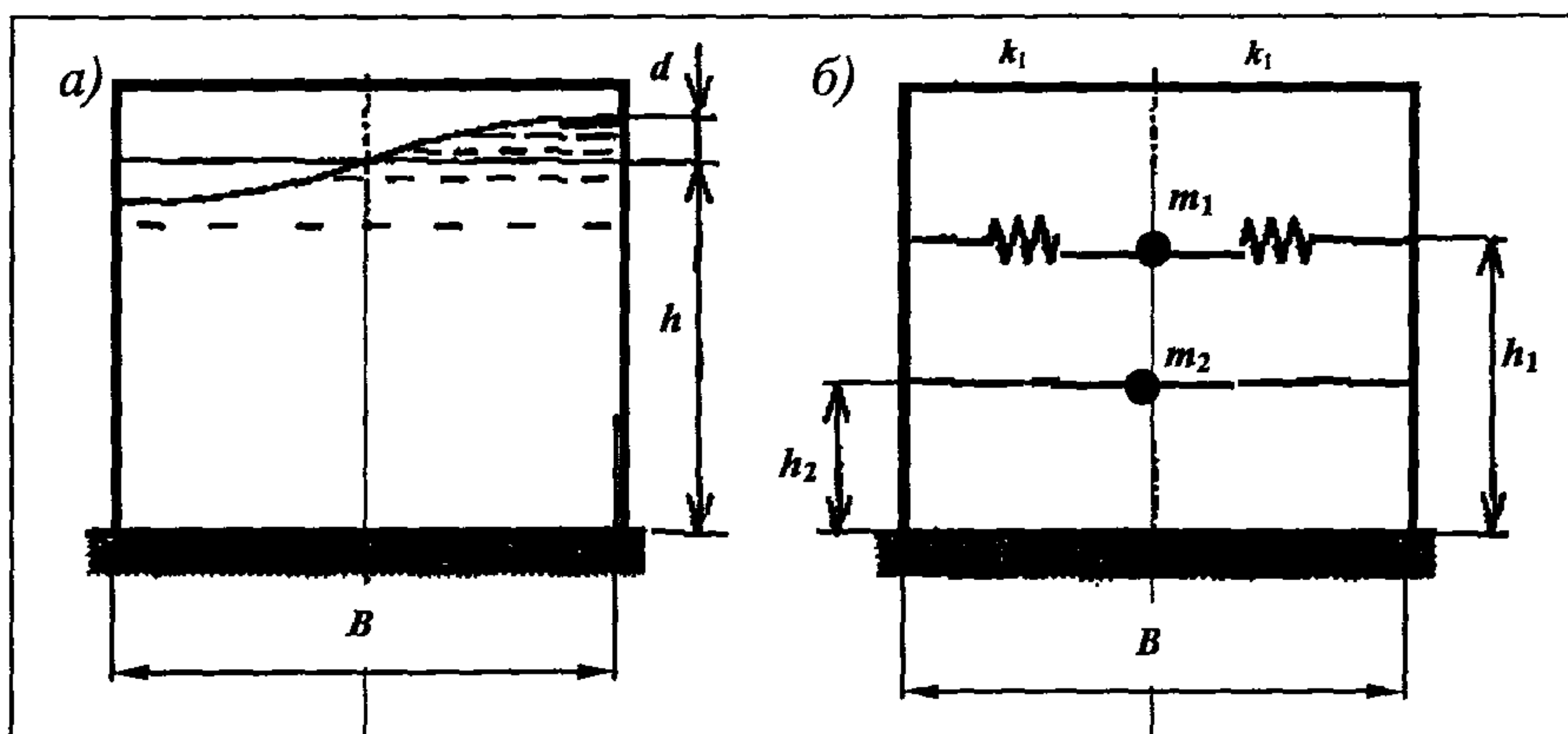
Рис.П.5.1. Моделирование резервуара с жидкостью: а - колебание жидкости в резервуаре; б - расчетная схема резервуара с жидкостью h – уровень жидкости в резервуаре; d – высота волны; m_1 – кинематическая масса; m_2 – инерционная масса; h_1, h_2 – привязки кинематической и инерционной масс
