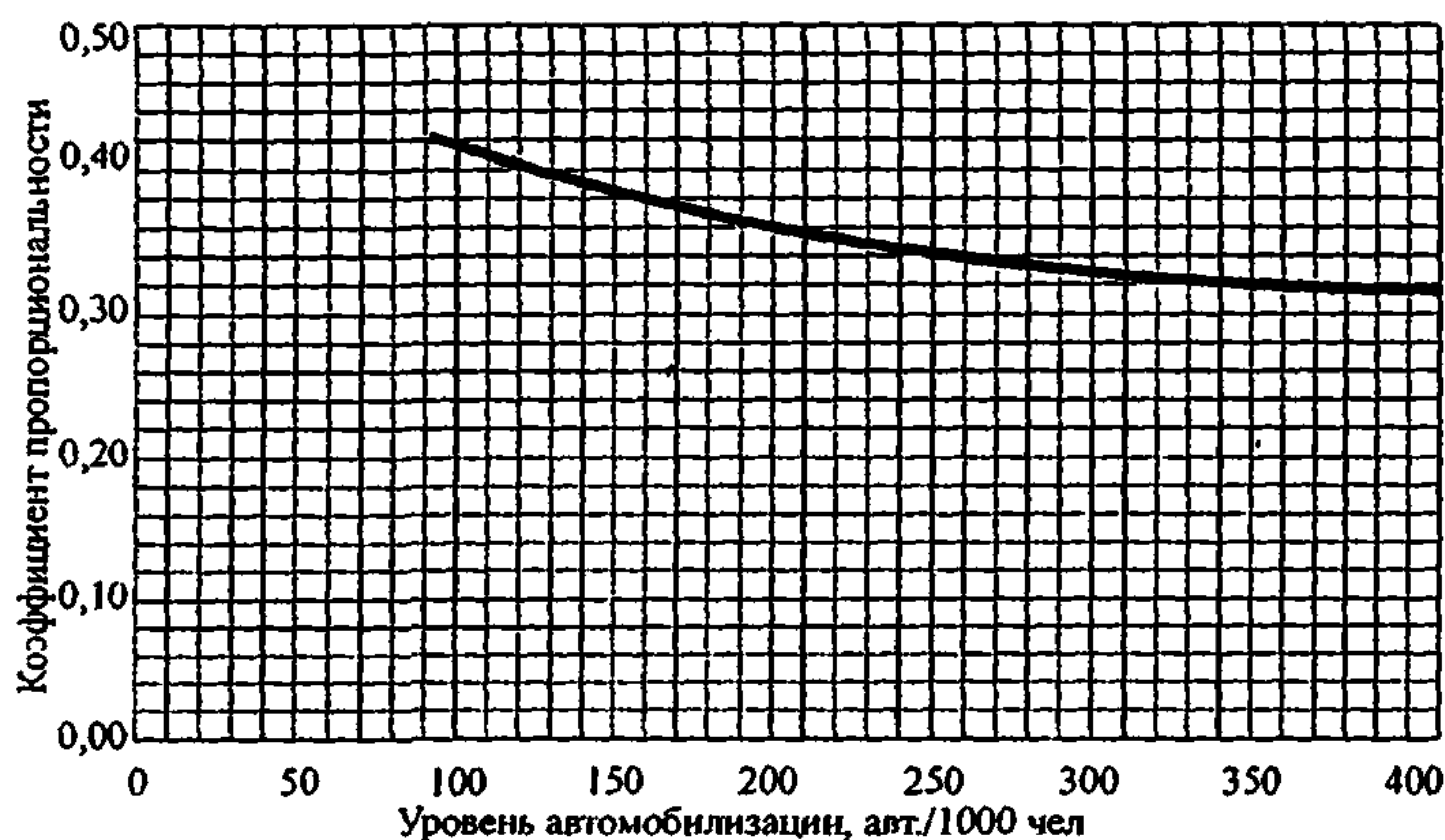
Рис. 2.1. Зависимость коэффициента пропорциональности к_t(a) от уровня автомобилизации для расчета трудовых корреспонденций
