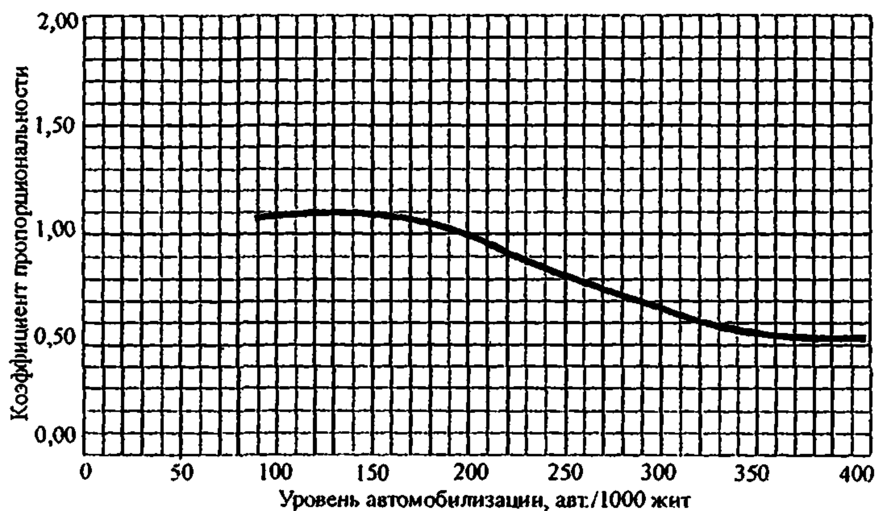
Рис. 2.2. Зависимость коэффициента пропорциональности для деловых корреспонденций к_d(a)
