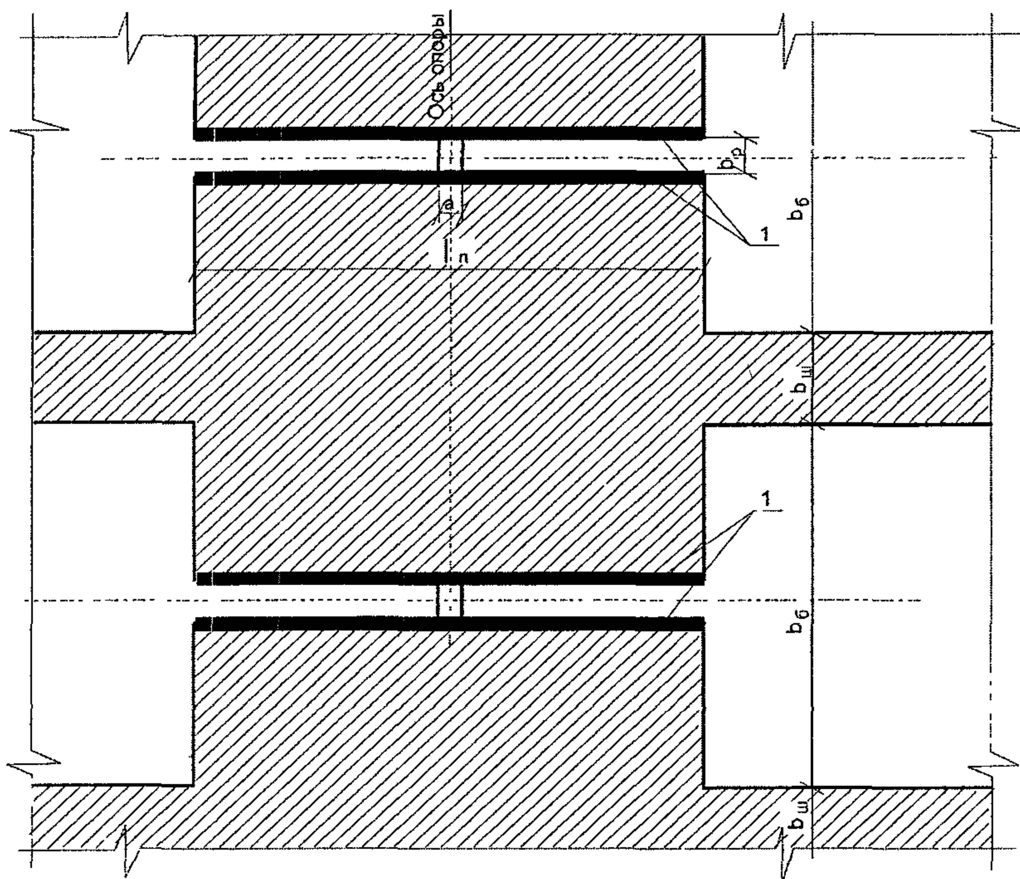
Рис. 3. (по а.с.№ 992645). Схема объединения пролетных строений по части ширины плиты проезжей части с отделением соединительной плиты от ребер в вертикальной плоскости:
