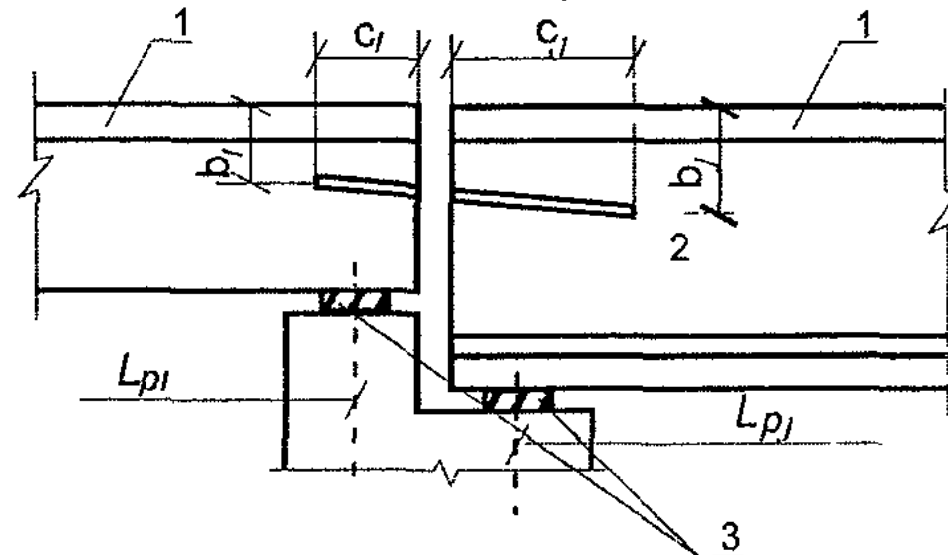
Рис. 13. Объединение пролетных строений тягами в надопорных зонах:
