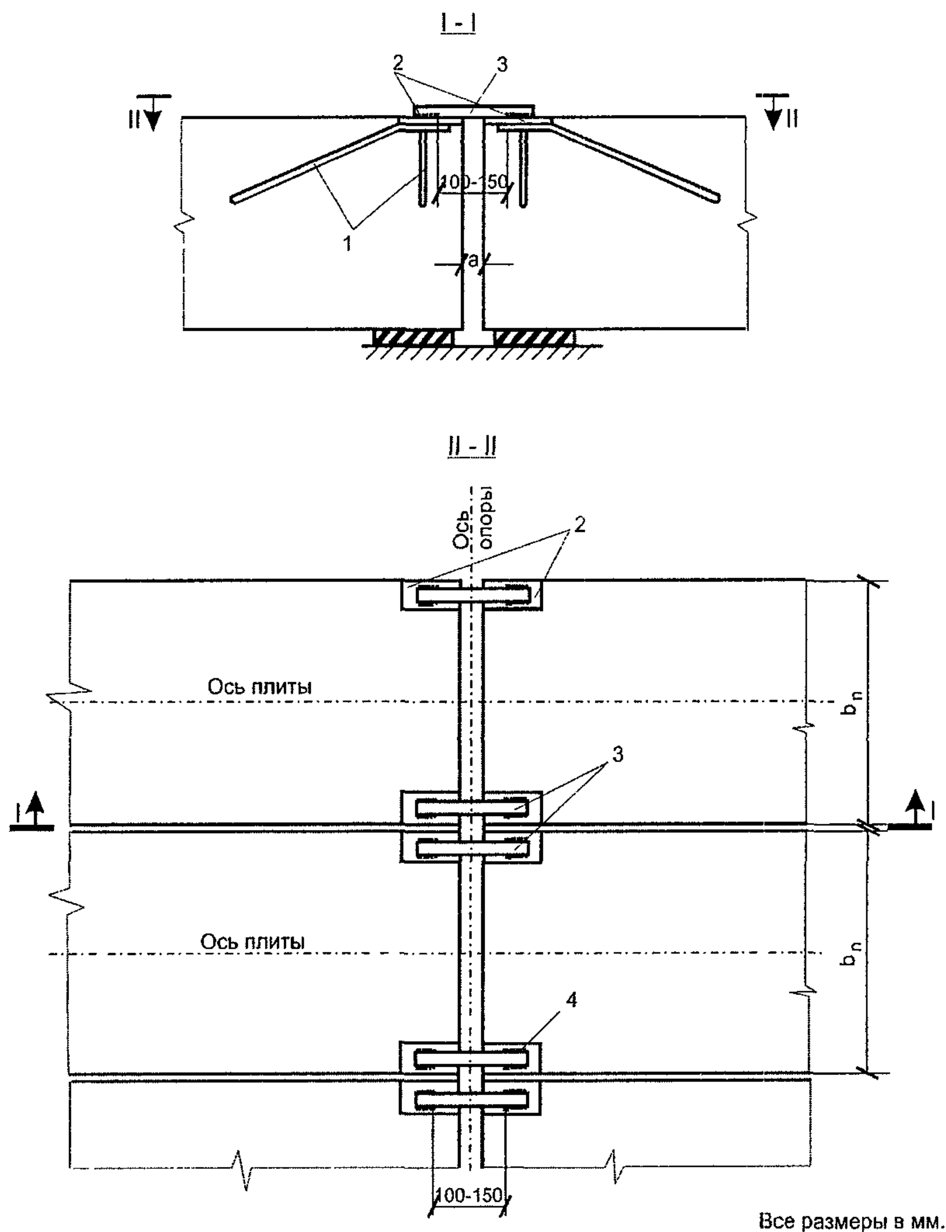
Рис. 5. Схема объединения пролетных строений по стыковым накладкам:
