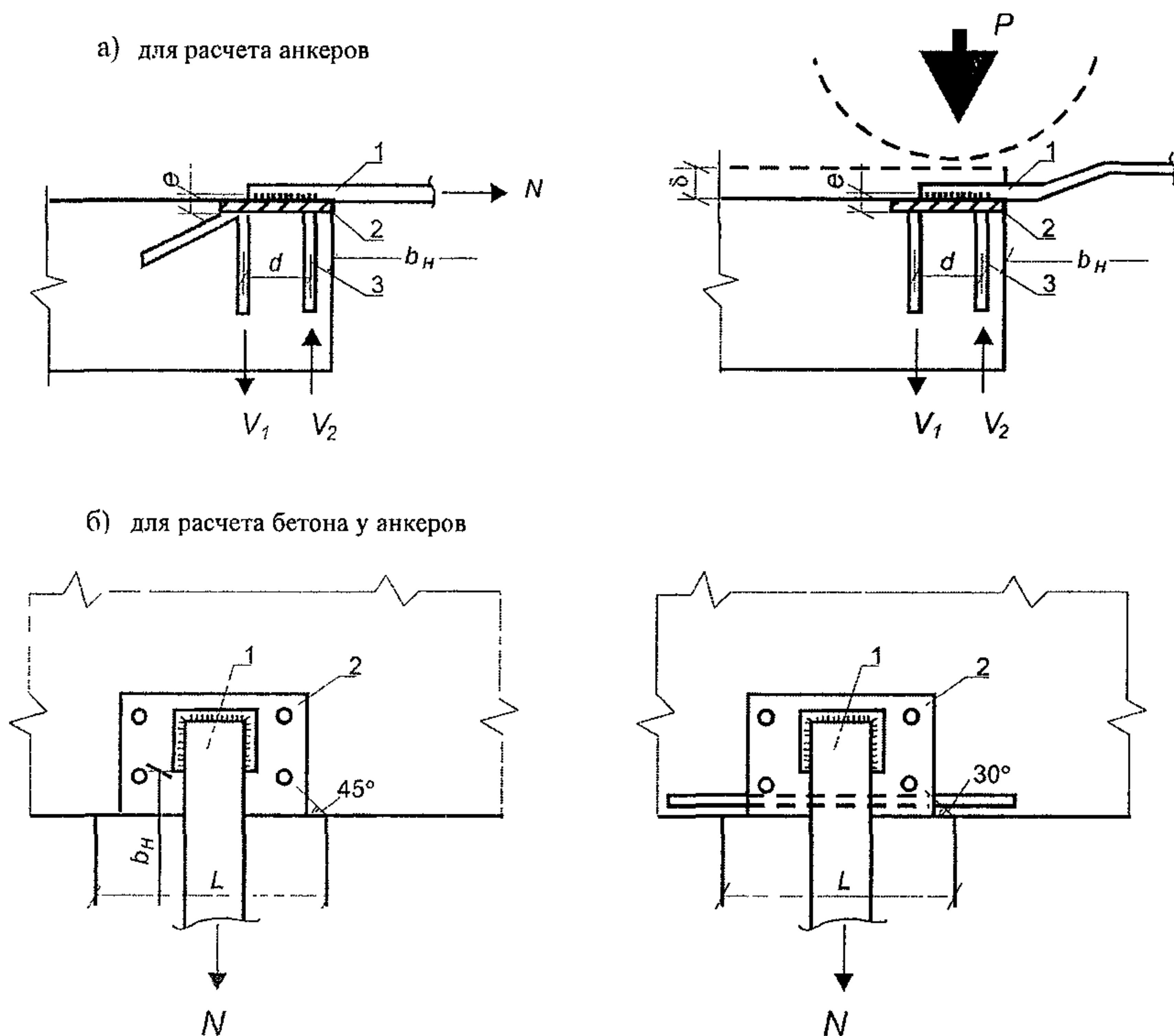
Рис. 21. Схемы к расчету закладных деталей: 1 – стыковая накладка; 2 – закладная деталь; 3 – анкер
