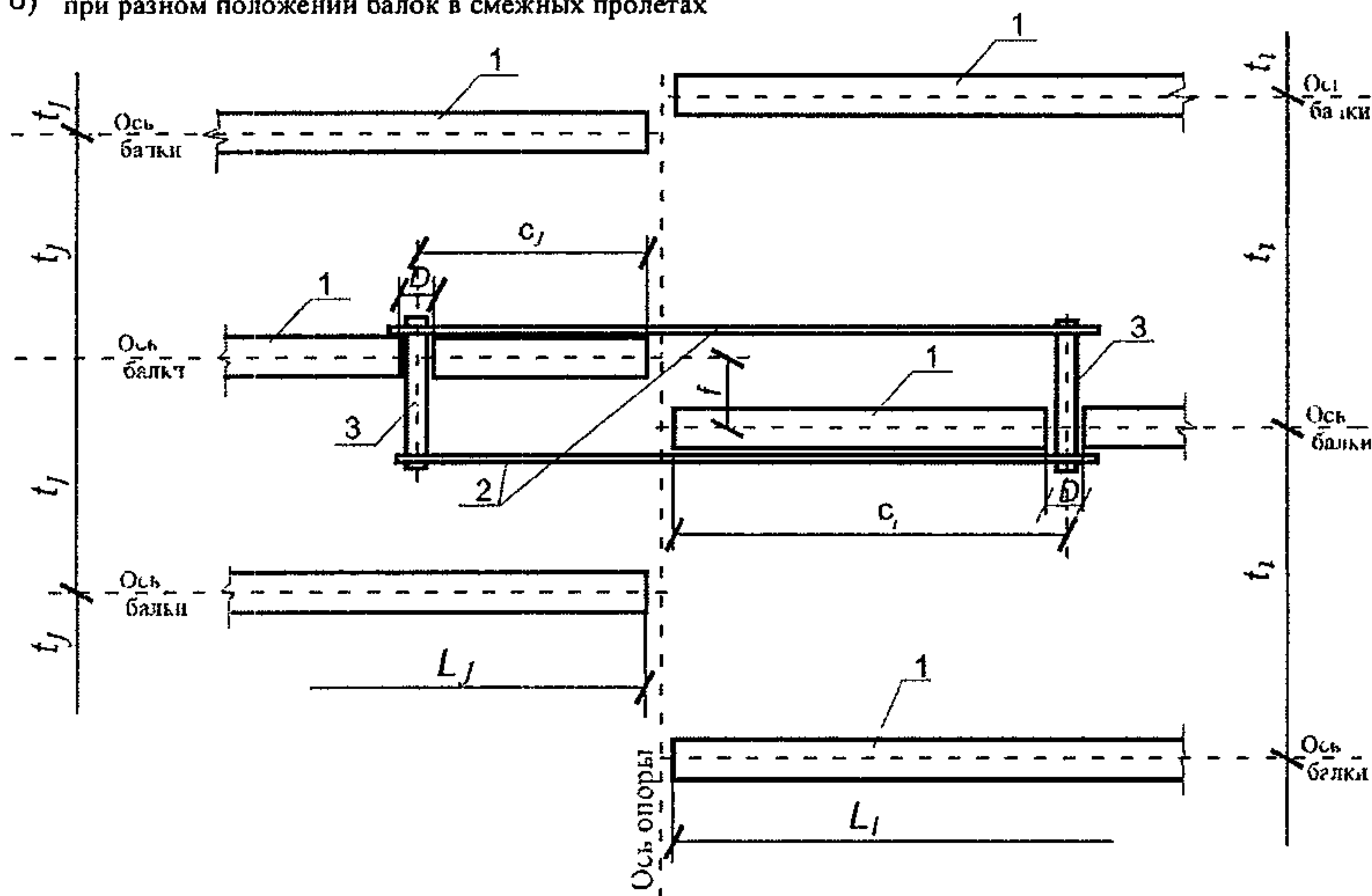
Рис. 14. Объединение пролетных строений тягами (план; плита балок не показана):
