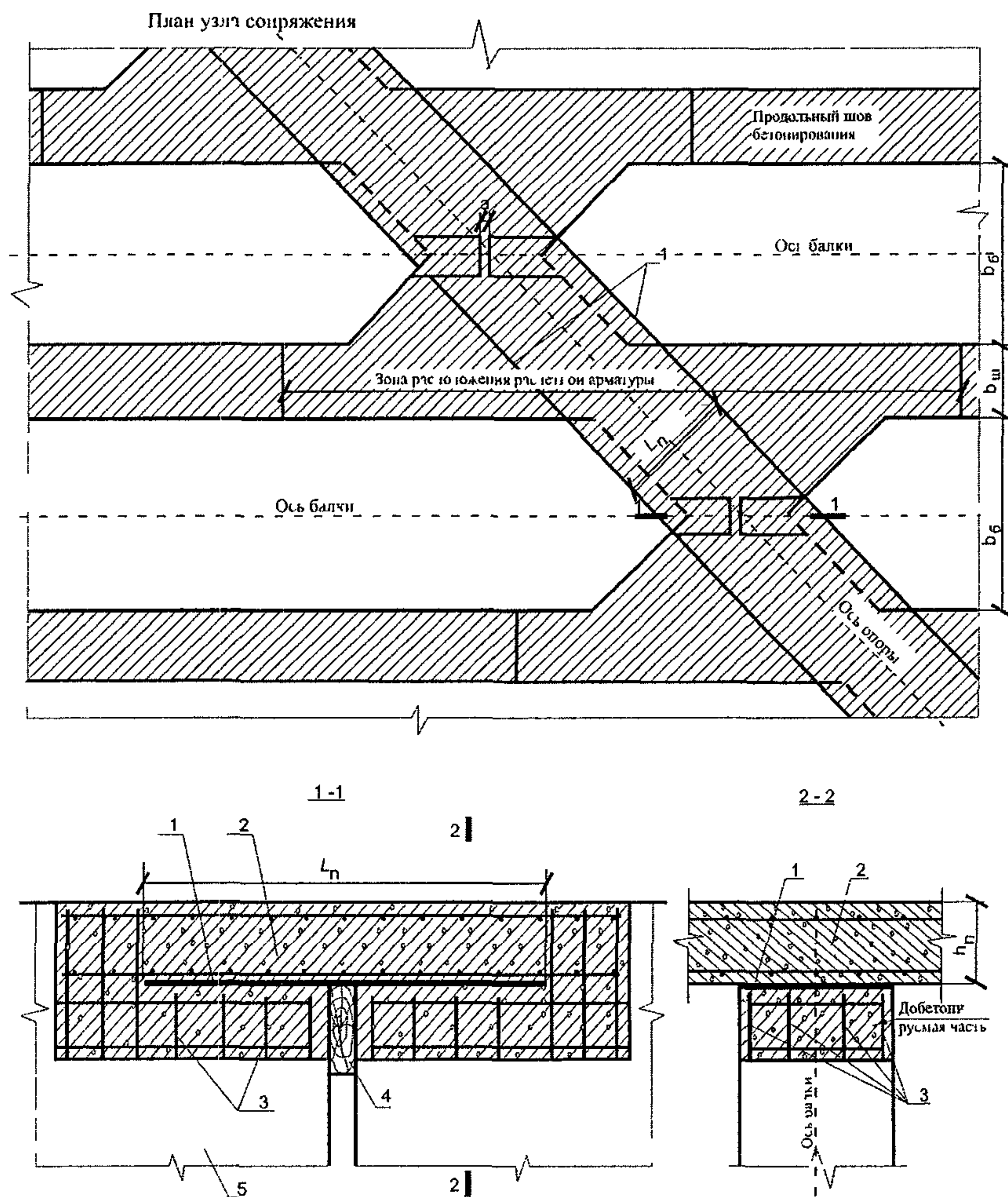
Рис. 10. Объединение пролетных строений по плите проезжей части при использовании типовых косых балок: 1 – прокладка из изопласта; 2 – соединительная плита; 3 – выпуски из ребра балок (обрезать в уровне низа прокладки); 4 – брус-опалубка; 5 – балка; а – расстояние между торцами смежных пролетных строений; b_b – ширина балки; b_{ш} – ширина стыка между балками; L_n – длина соединительной плиты; h_n – толщина соединительной плиты
