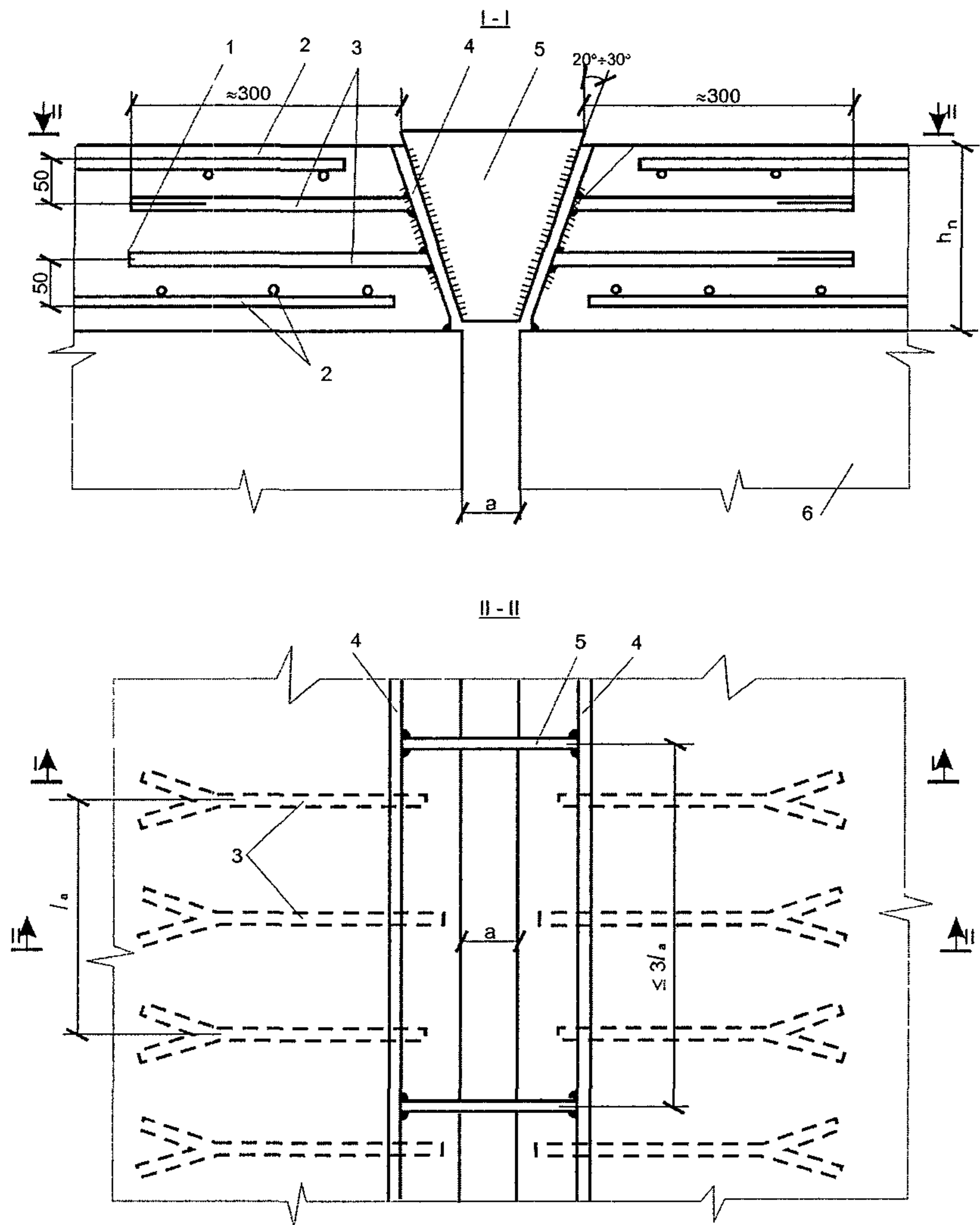
Рис. 6. Схема объединения пролетных строений с помощью шпонок: 1 – плита проезжей части h_n ; 2 – арматура плиты; 3 – анкера закладной детали; 4 – закладная деталь; 5 – соединительная трапецевидная пластина; 6 – ребро балки; l_a – шаг анкеров (устанавливают в шахматном порядке по высоте); a – расстояние между торцами смежных пролетных строений (размеры в мм)
