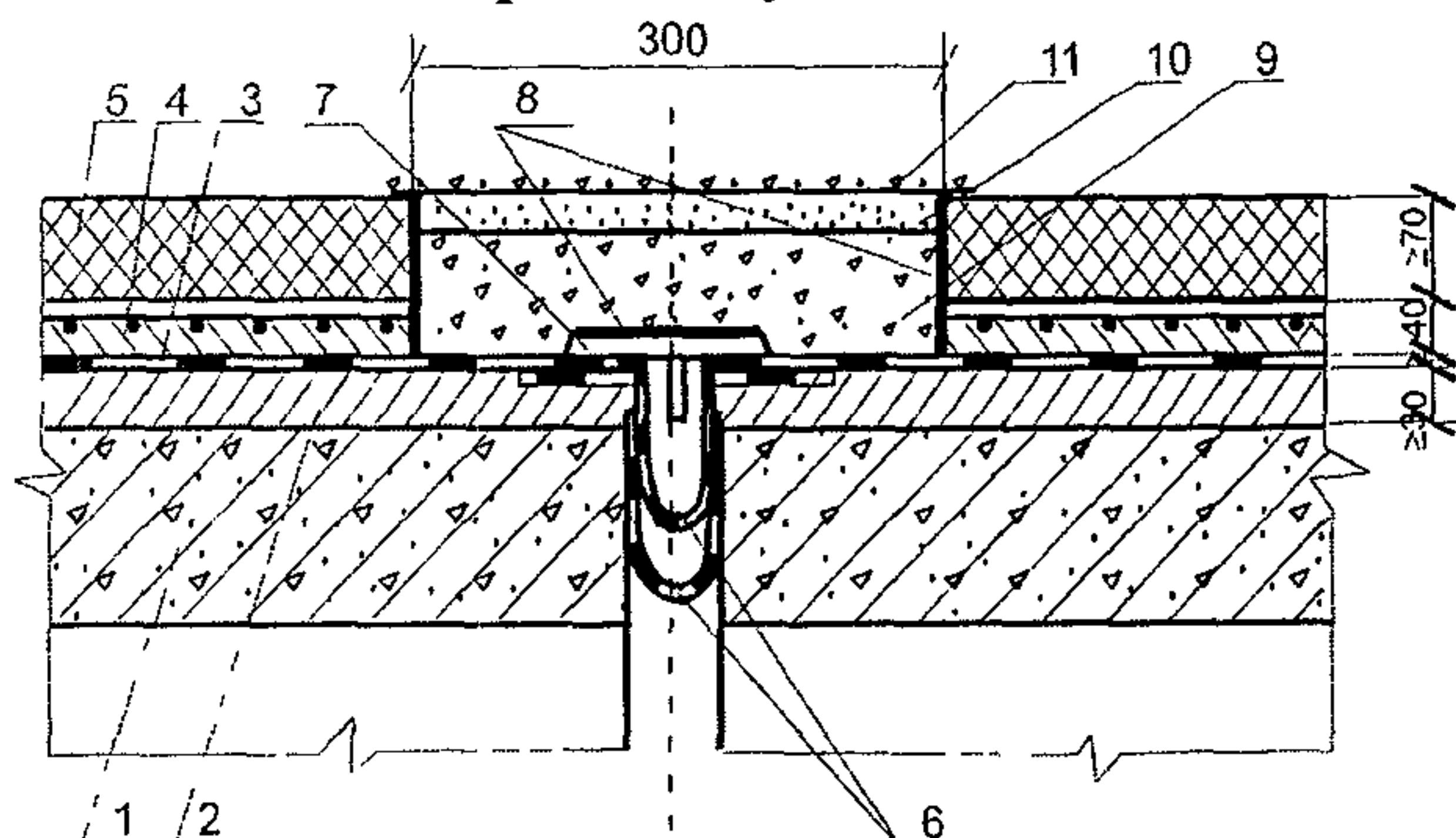
Рис. 23. Конструкция деформационного шва над узлом шарнирного сопряжения с заполнением мастикой: 1 – пролетное строение; 2 – выравнивающий слой (может отсутствовать); 3 – гидроизоляция; 4 – защитный слой; 5 – двухслойное асфальтобетонное покрытие; 6 – компенсатор; 7 – заполнение жгутами пороизола; 8 – полимерно-битумная мастика
