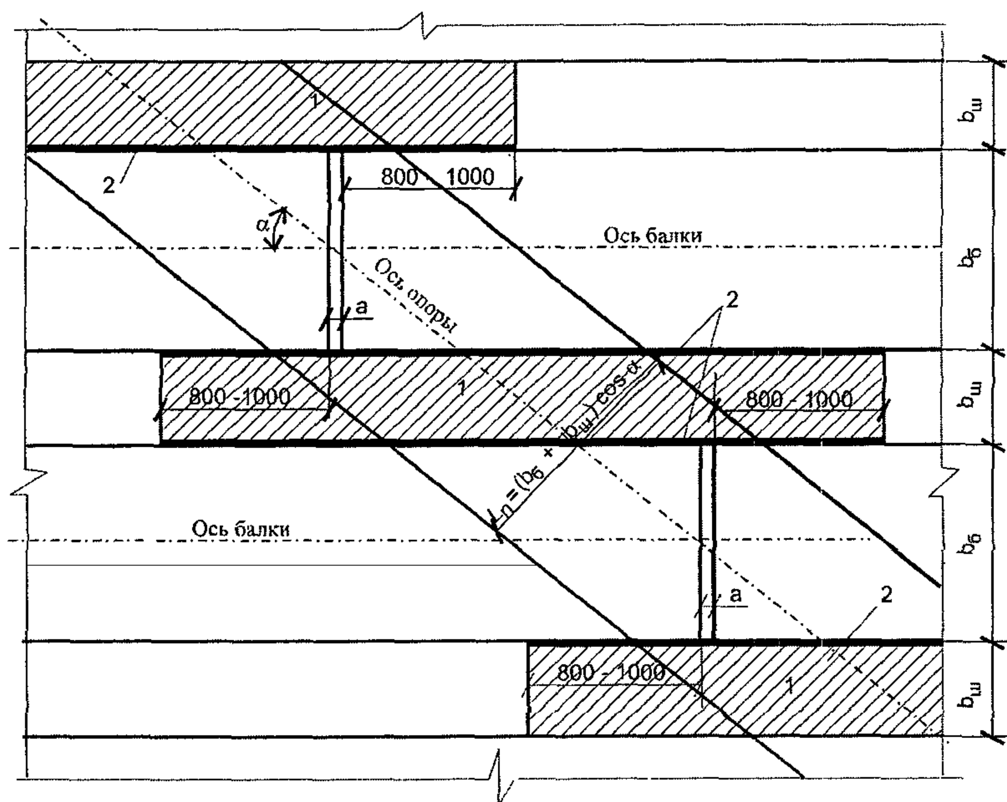
Рис. 11. Схема объединения косых пролетных строений по продольным бетонируемым стыкам:
