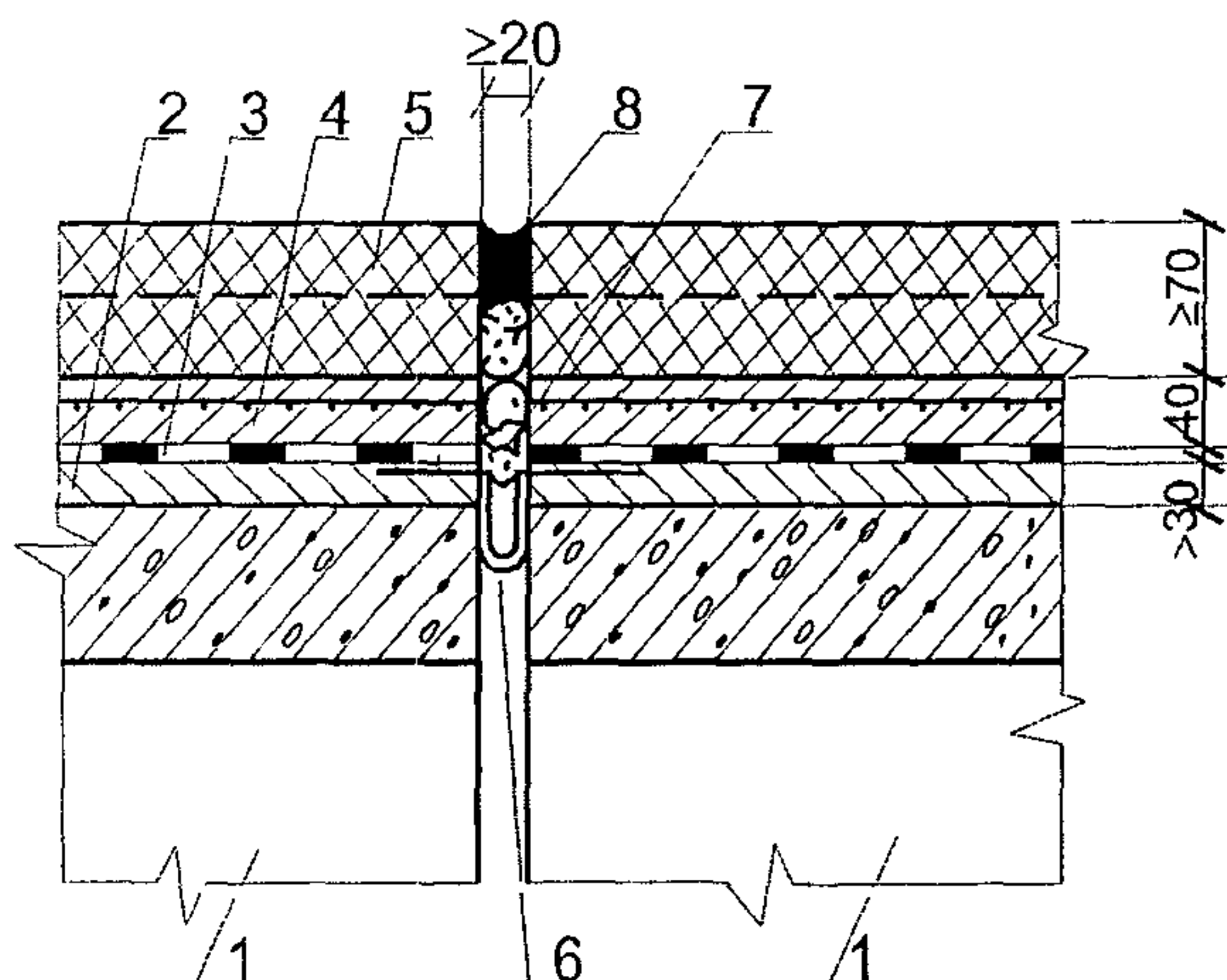
Рис. 23. Конструкция деформационного шва над узлом шарнирного сопряжения с заполнением мастикой: 1 – пролетное строение; 2 – выравнивающий слой (может отсутствовать); 3 – гидроизоляция; 4 – защитный слой; 5 – двухслойное асфальтобетонное покрытие; 6 – компенсатор; 7 – заполнение жгутами пороизола; 8 – полимерно-битумная мастика
