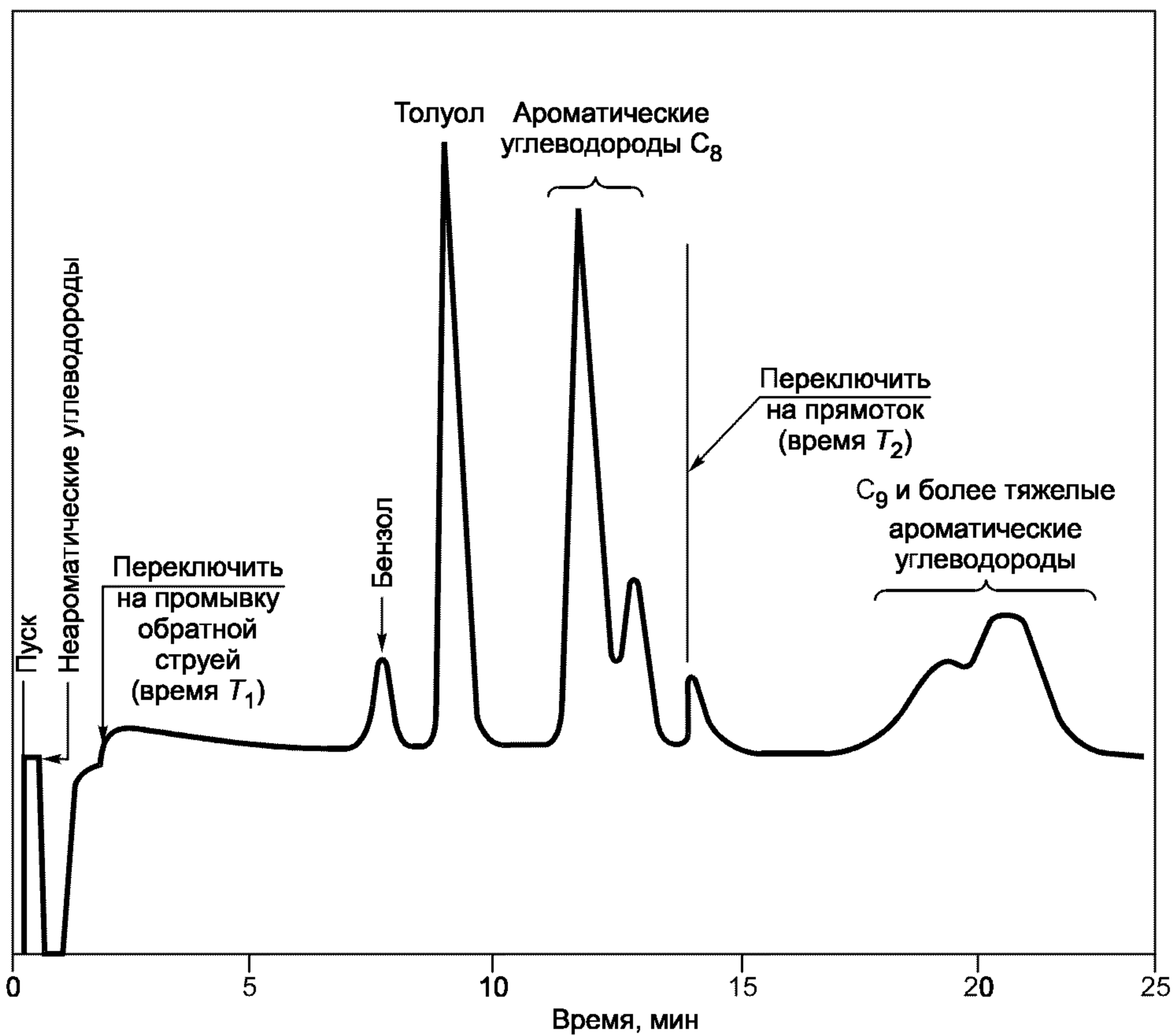
Рисунок 4 — Хроматограмма бензина
