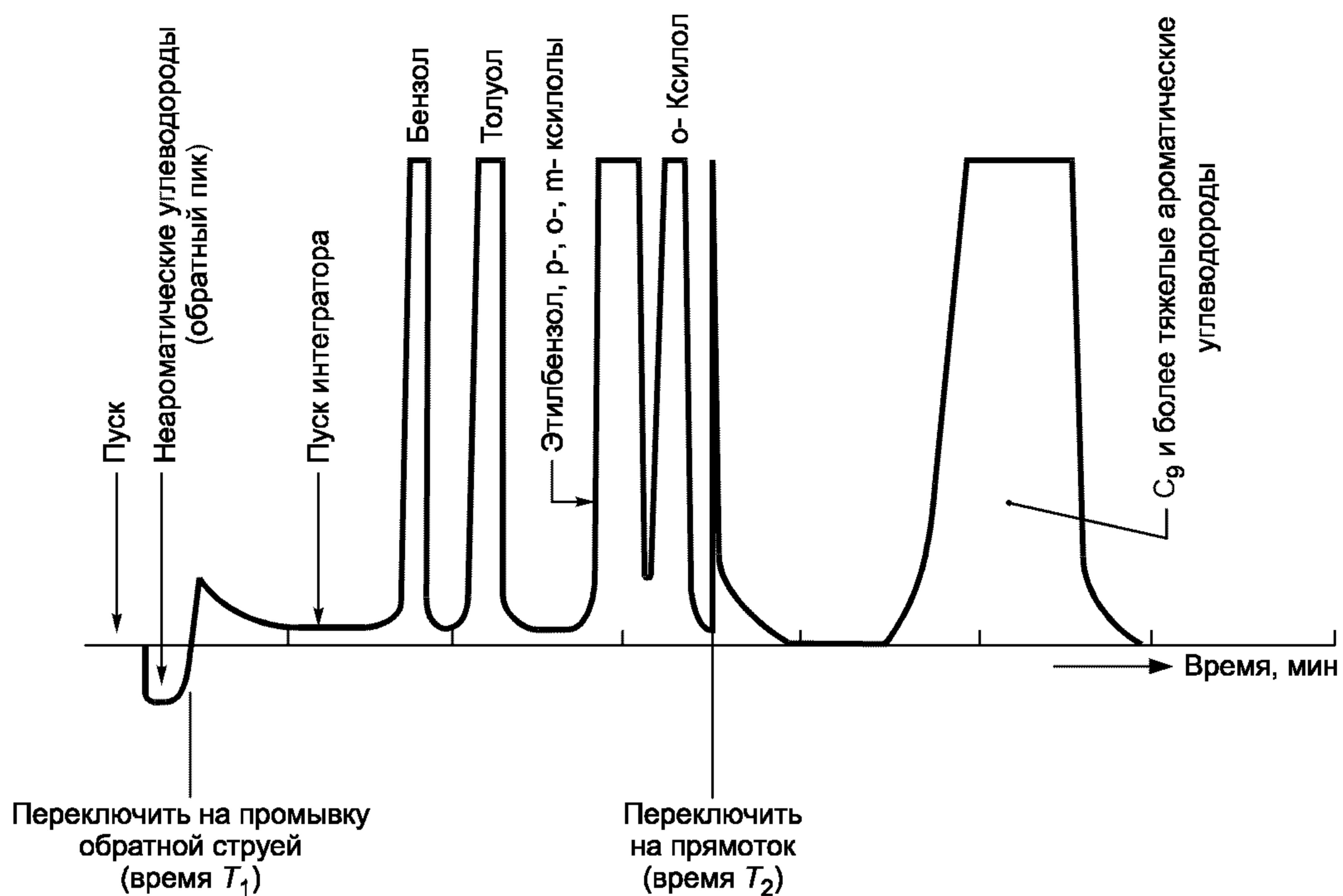
Рисунок 3 — Хроматограмма, показывающая позиции включения клапана
