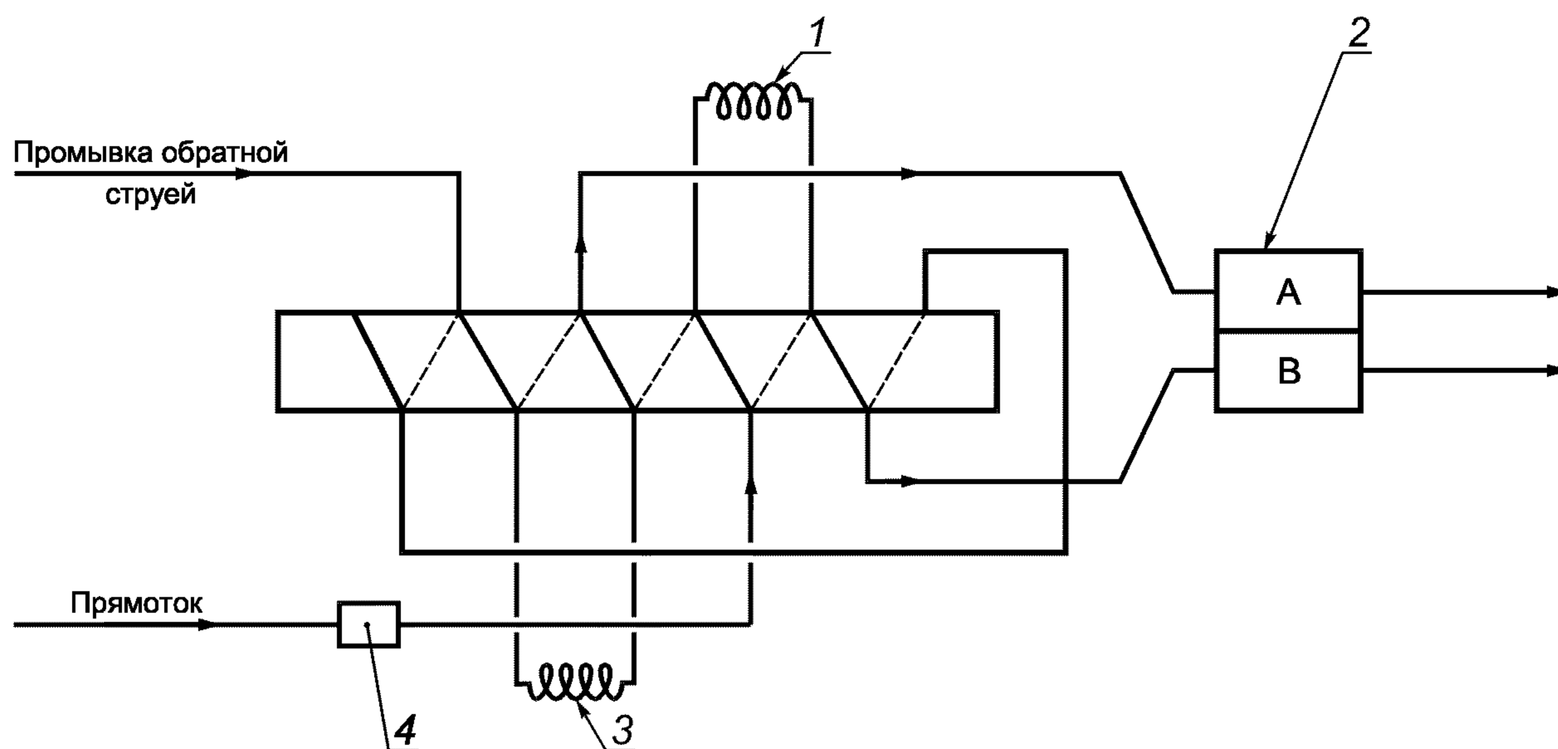
1 — колонка А; 2 — детектор; 3 — колонка В; 4 — система ввода
