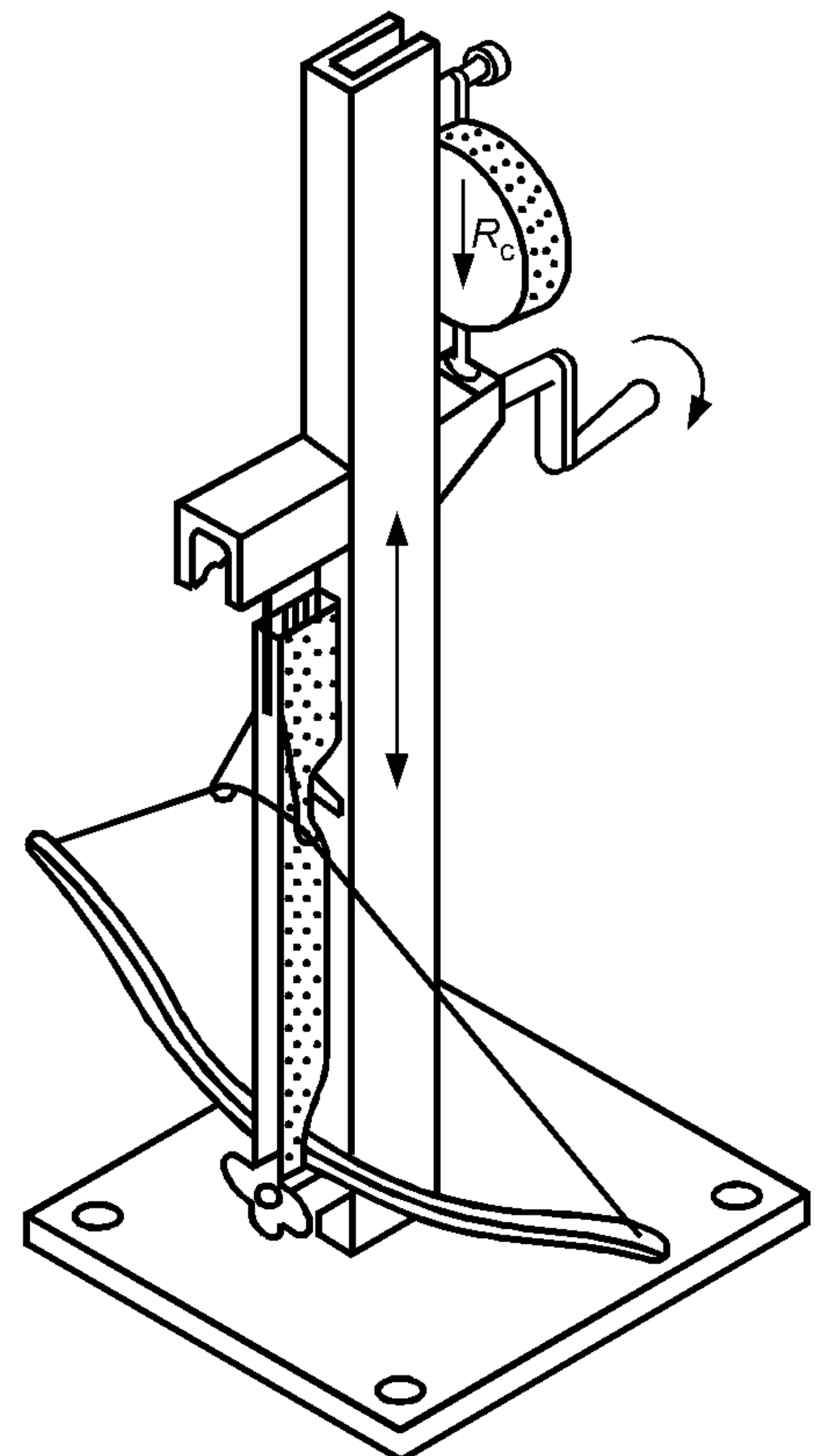
Рисунок 2 — Схема измерения силы дуг (дуги) арбалета
