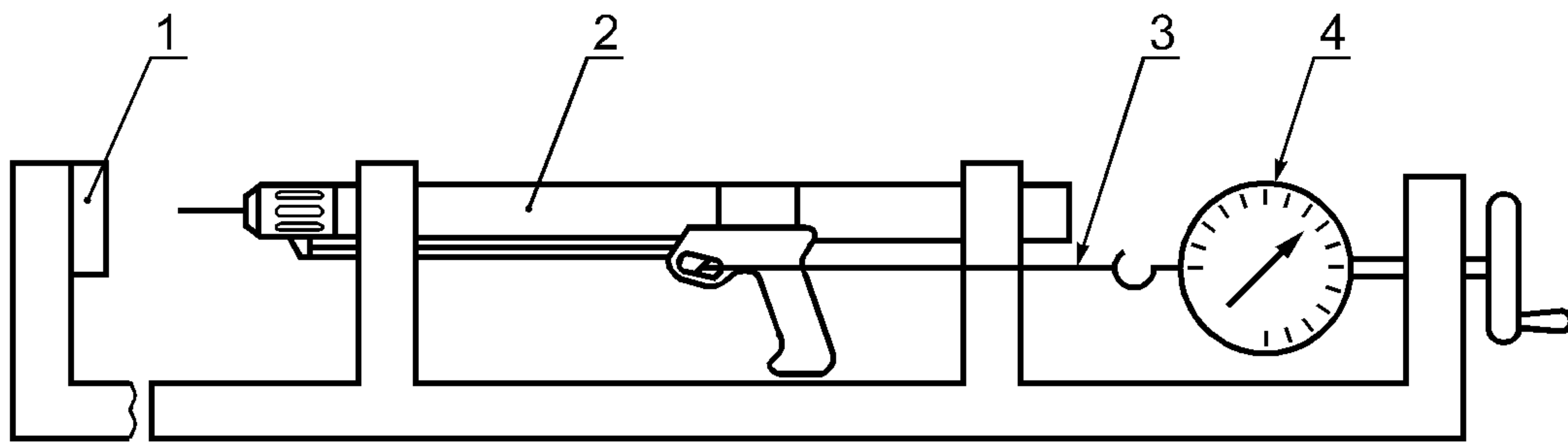
1 — приспособление, 2 — арбалет, 3 — трос, 4 — динамометр
