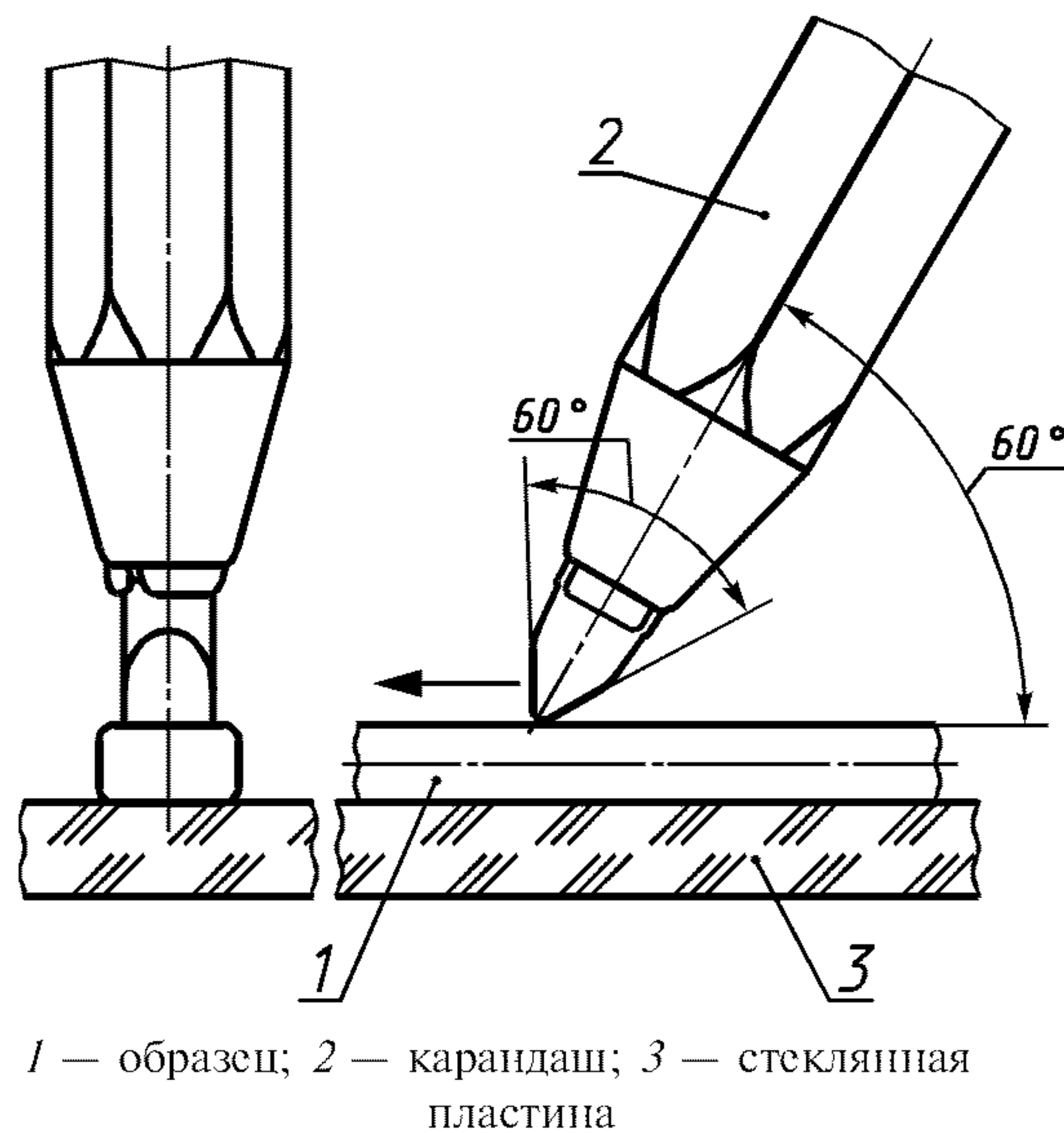
Рисунок 1 — Испытание на стойкость к воздействию растворителей
