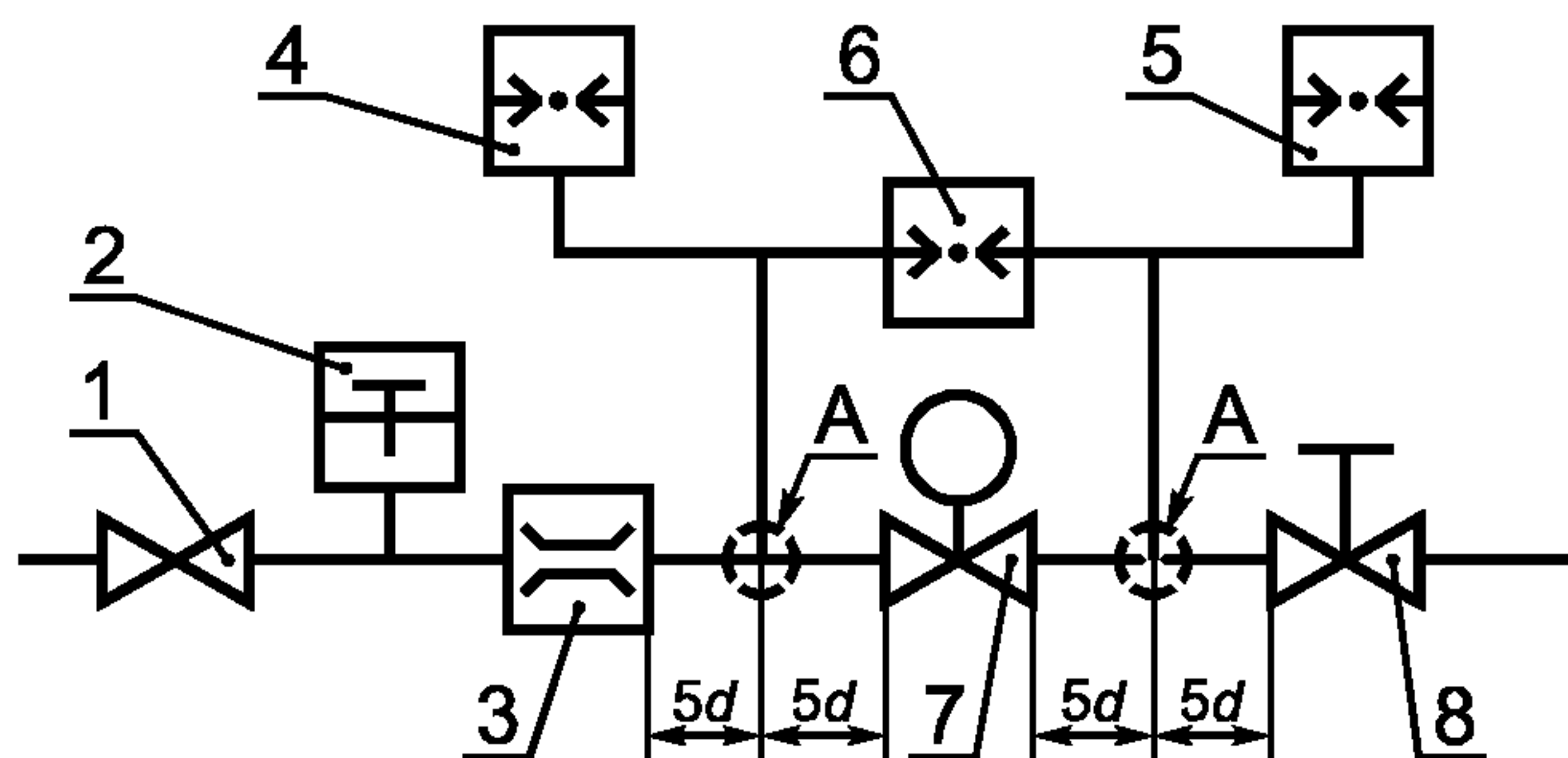
A — деталь; d — внешний диаметр; 1 — настраиваемый регулятор входного давления; 2 — термометр; 3 — расходомер; 4 — прибор для измерения давления на входе; 5 — прибор для измерения давления на выходе; 6 — прибор для измерения перепада давления; 7 — испытуемый клапан; 8 — ручной регулирующий кран
