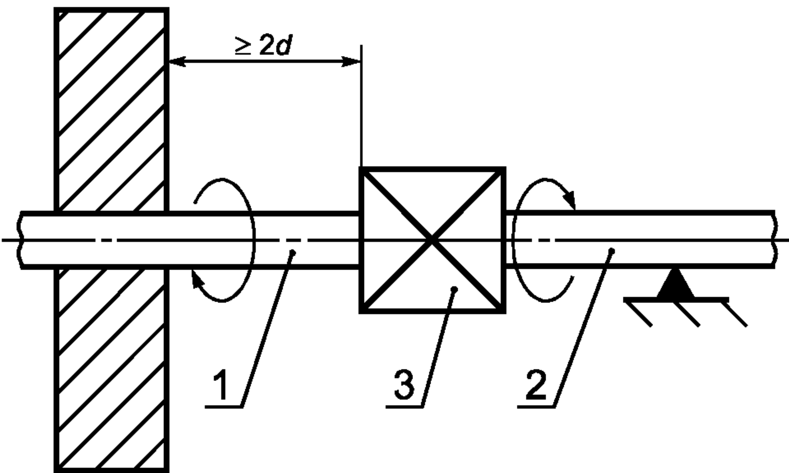
d — внешний диаметр трубы; 1 — первая труба; 2 — вторая труба; 3 — испытываемый клапан
