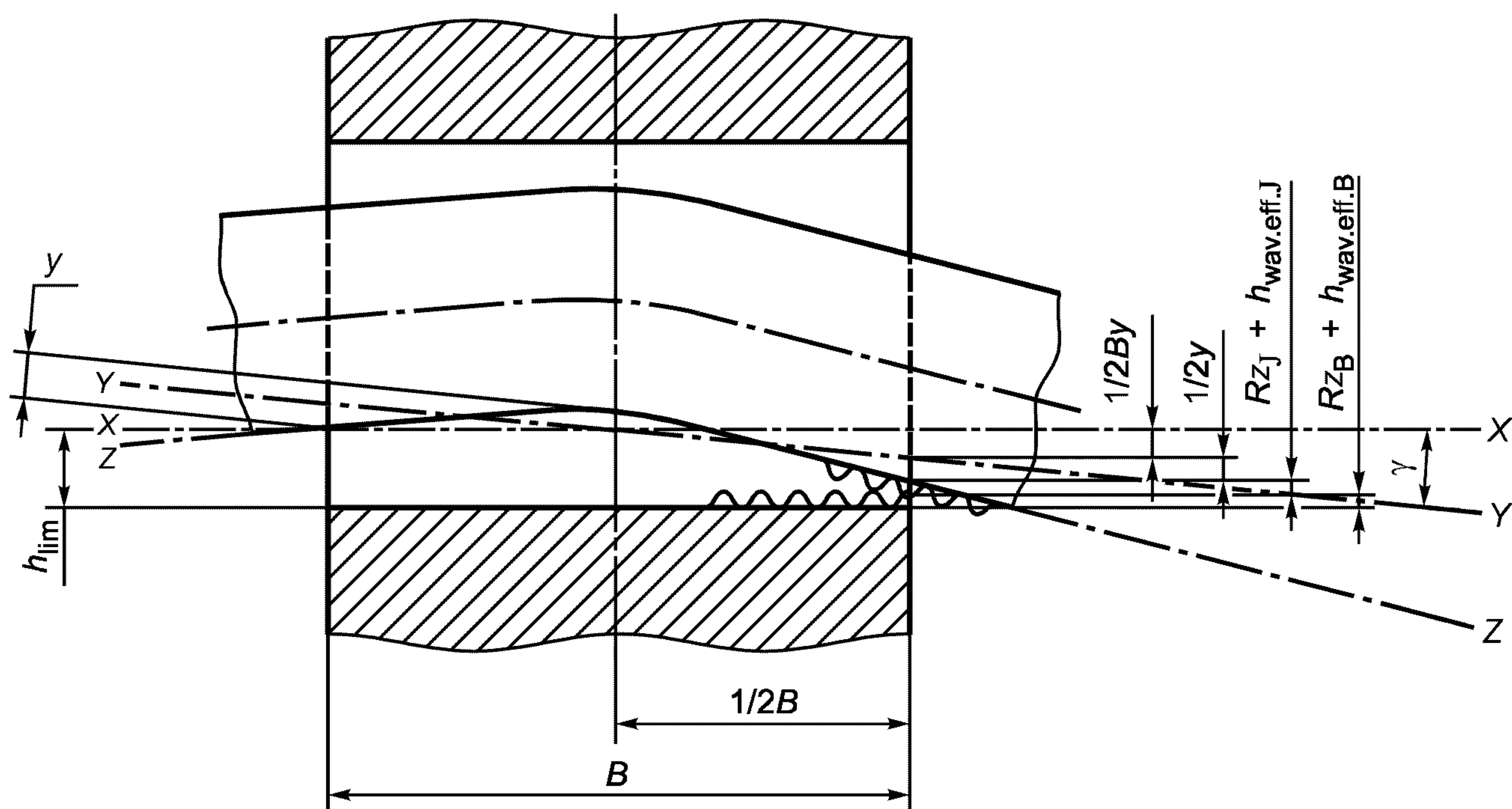
Рисунок 1 — Минимальная допустимая толщина смазочного слоя, когда не допускается процесс приработки
