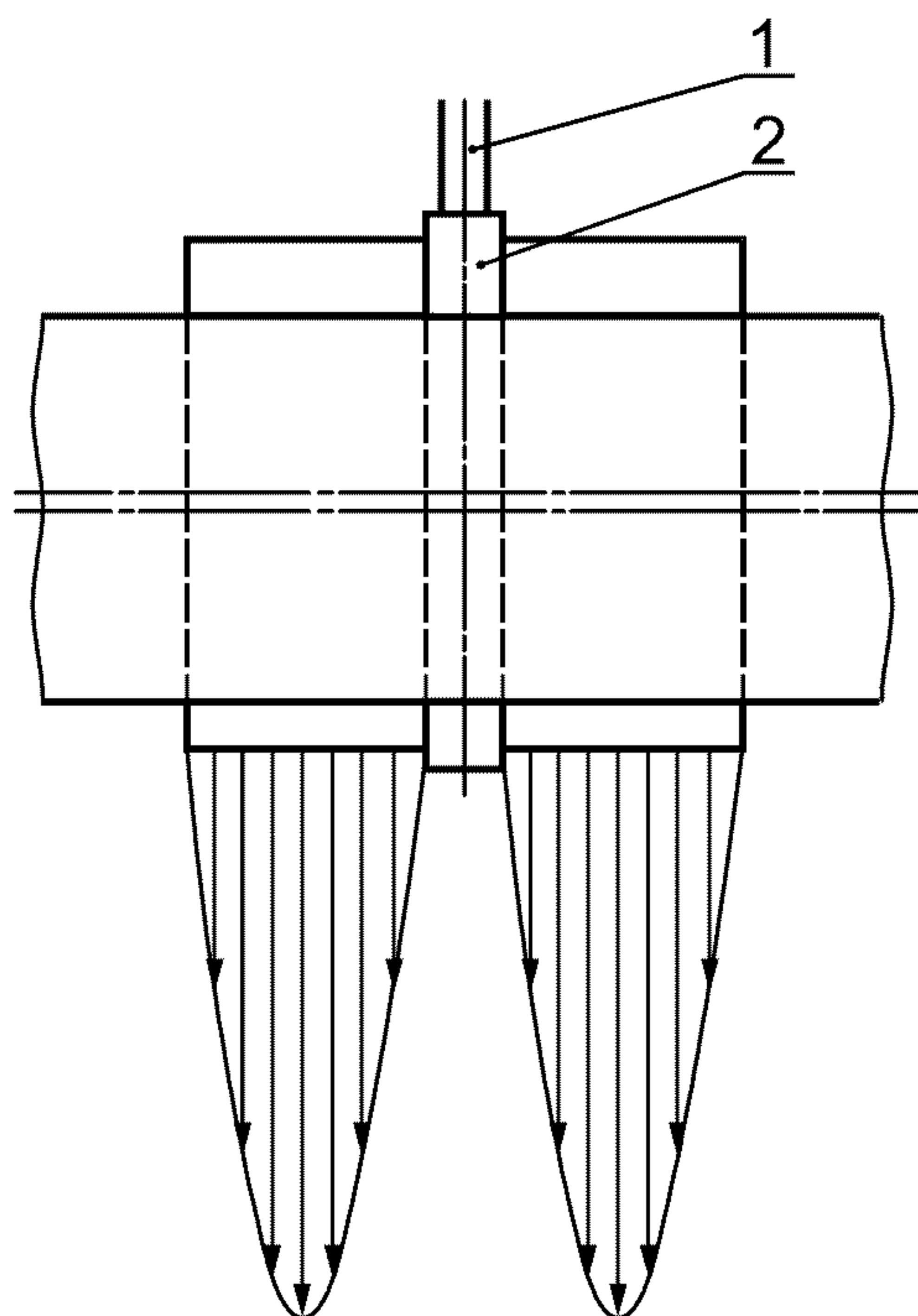
1 — смазочное отверстие; 2 — смазочная канавка
