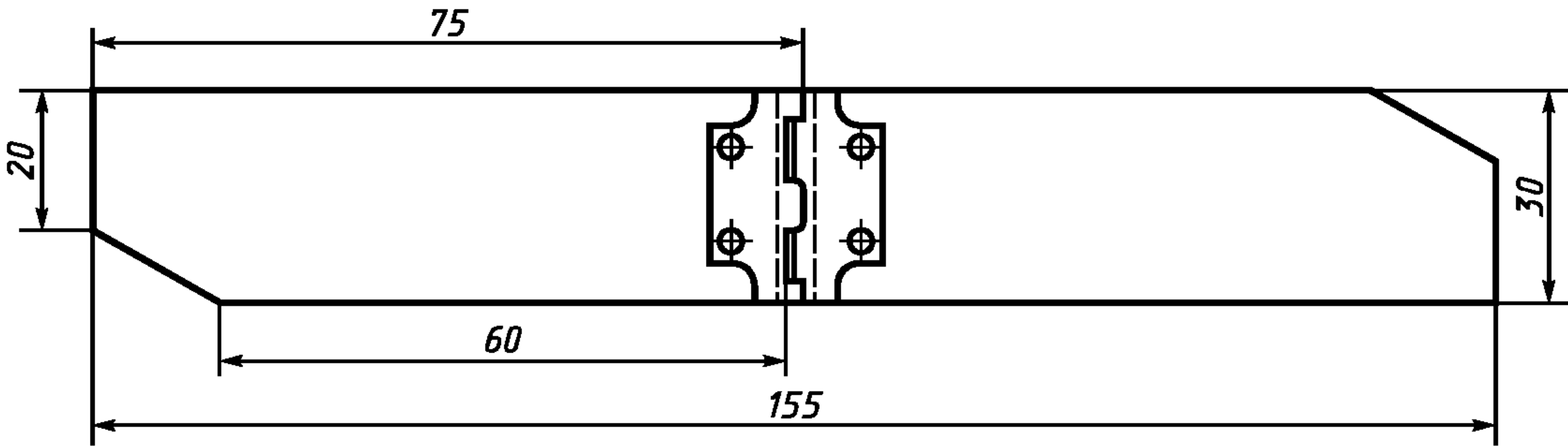
Рисунок Г.1 — Давильная пластина
