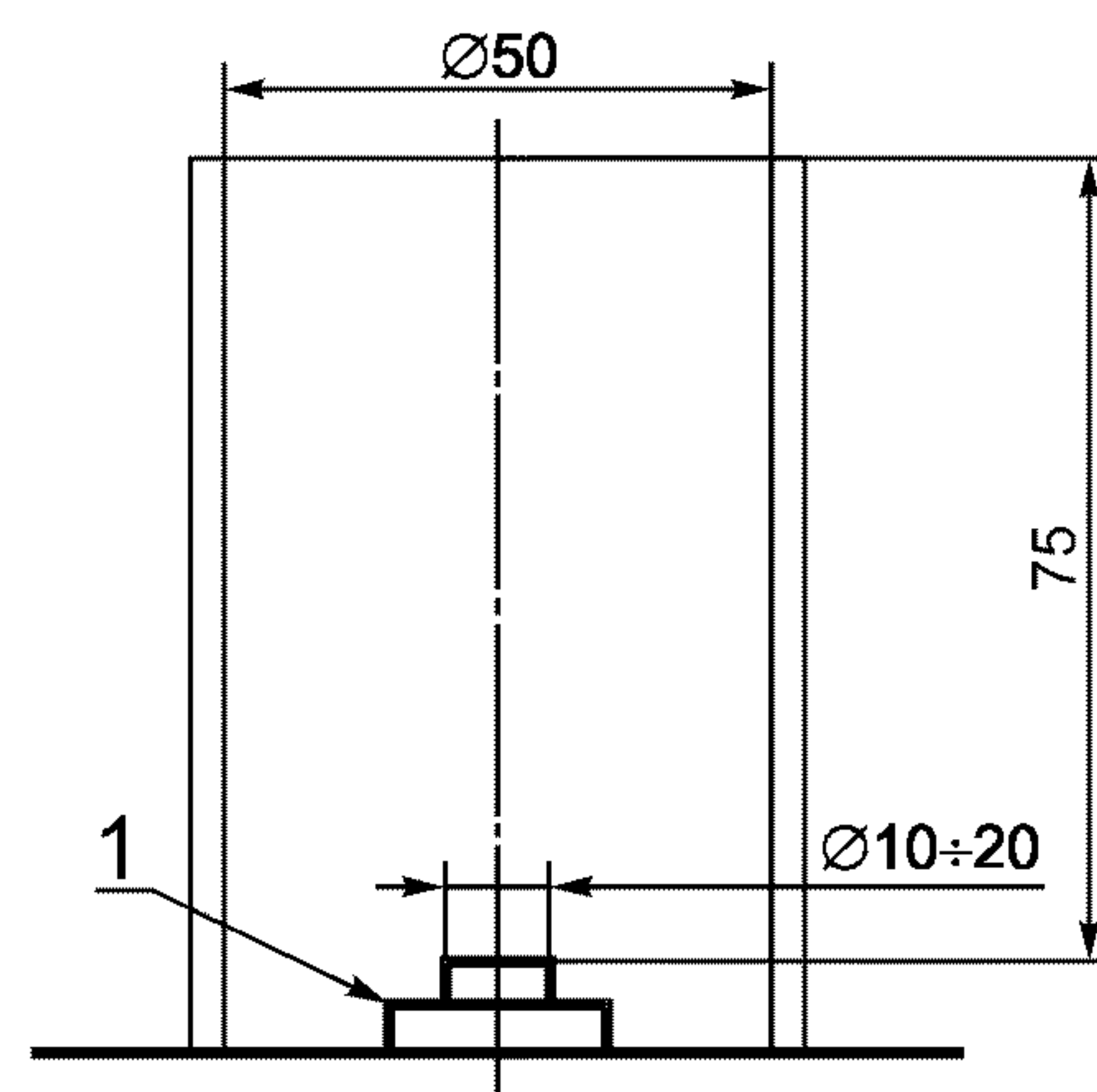
1 — головка фотометра
