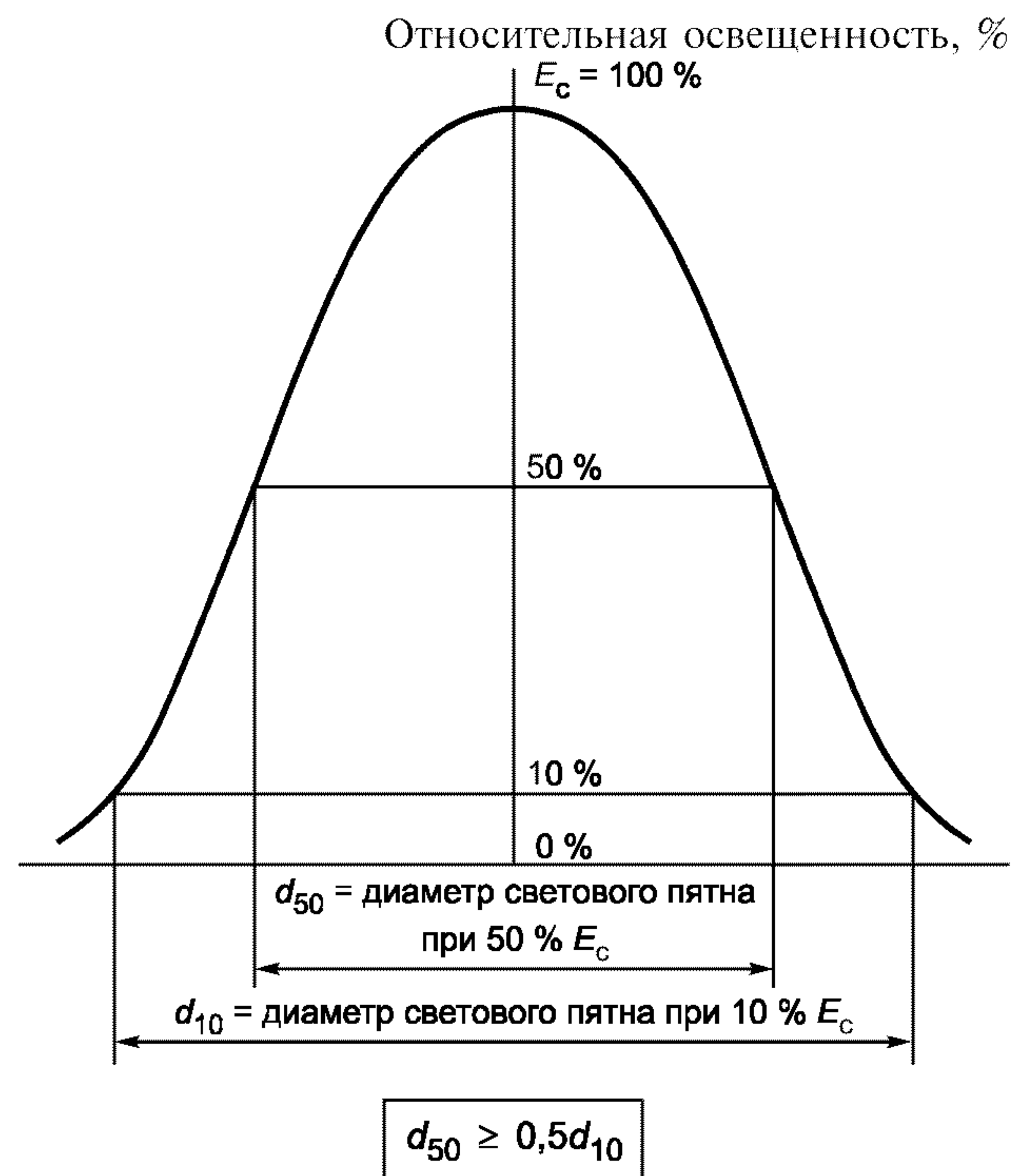
Рисунок 104 — Распределение света
