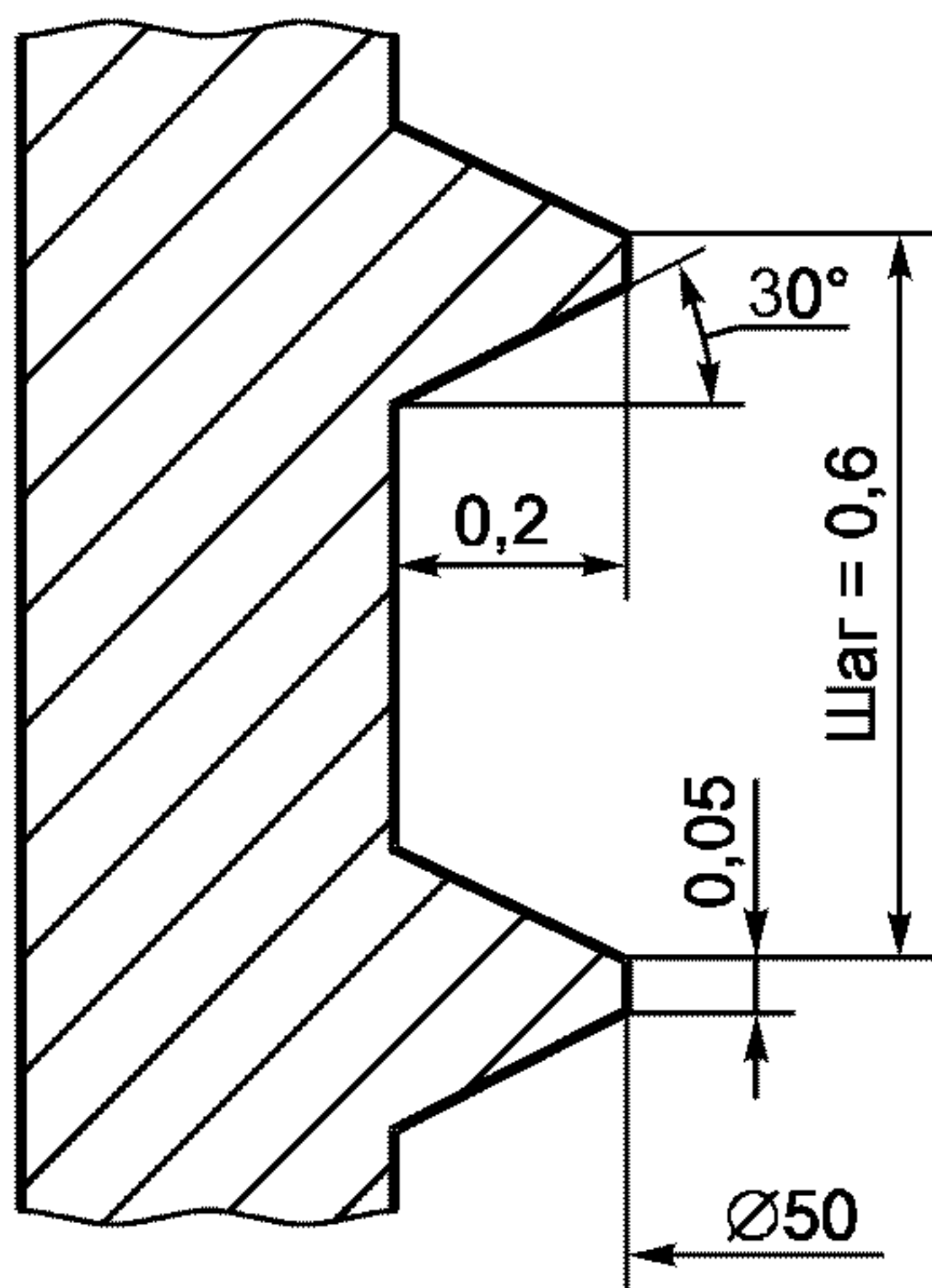
Рисунок 111 — Деталь внутренней поверхности трубки (пример)
