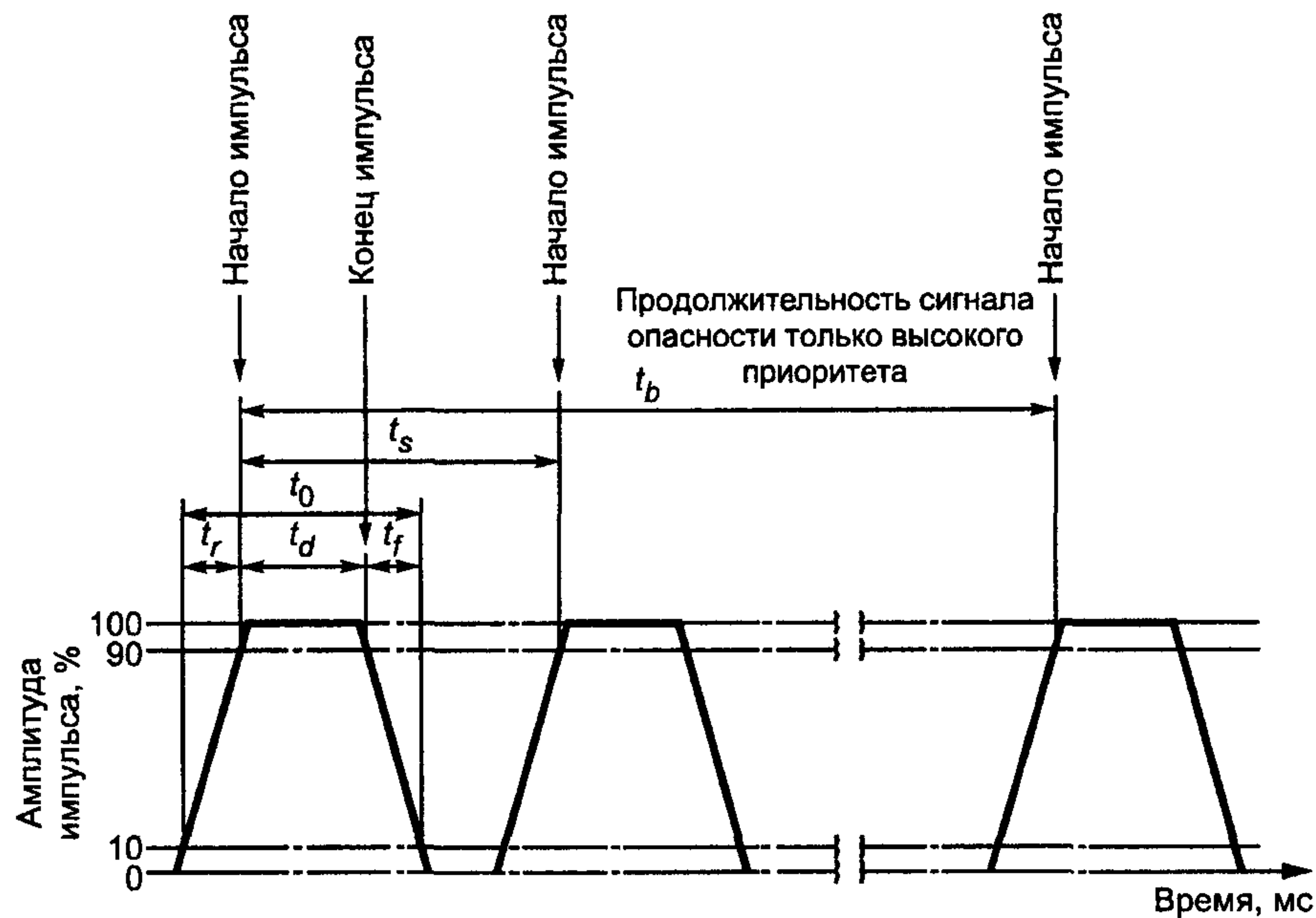
Рисунок 1 — Временные характеристики звуковых сигналов
