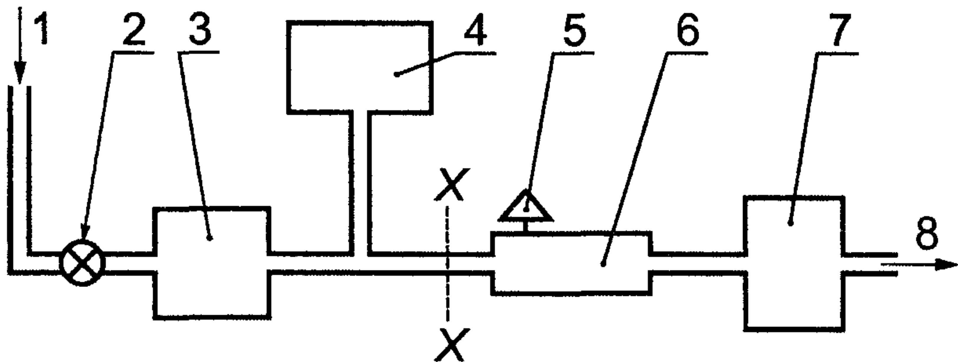
1 — подача воздуха; 2 — клапан контроля потока; 3 — устройство регулирования потока; 4 — устройство измерения давления; 5 — устройство сброса давления; 6 — передающие и принимающие системы СВГС с устройством сброса давления; 7 — система вывода или эквивалентное испытательное устройство; 8 — выход; X—X — вход в СВГС
