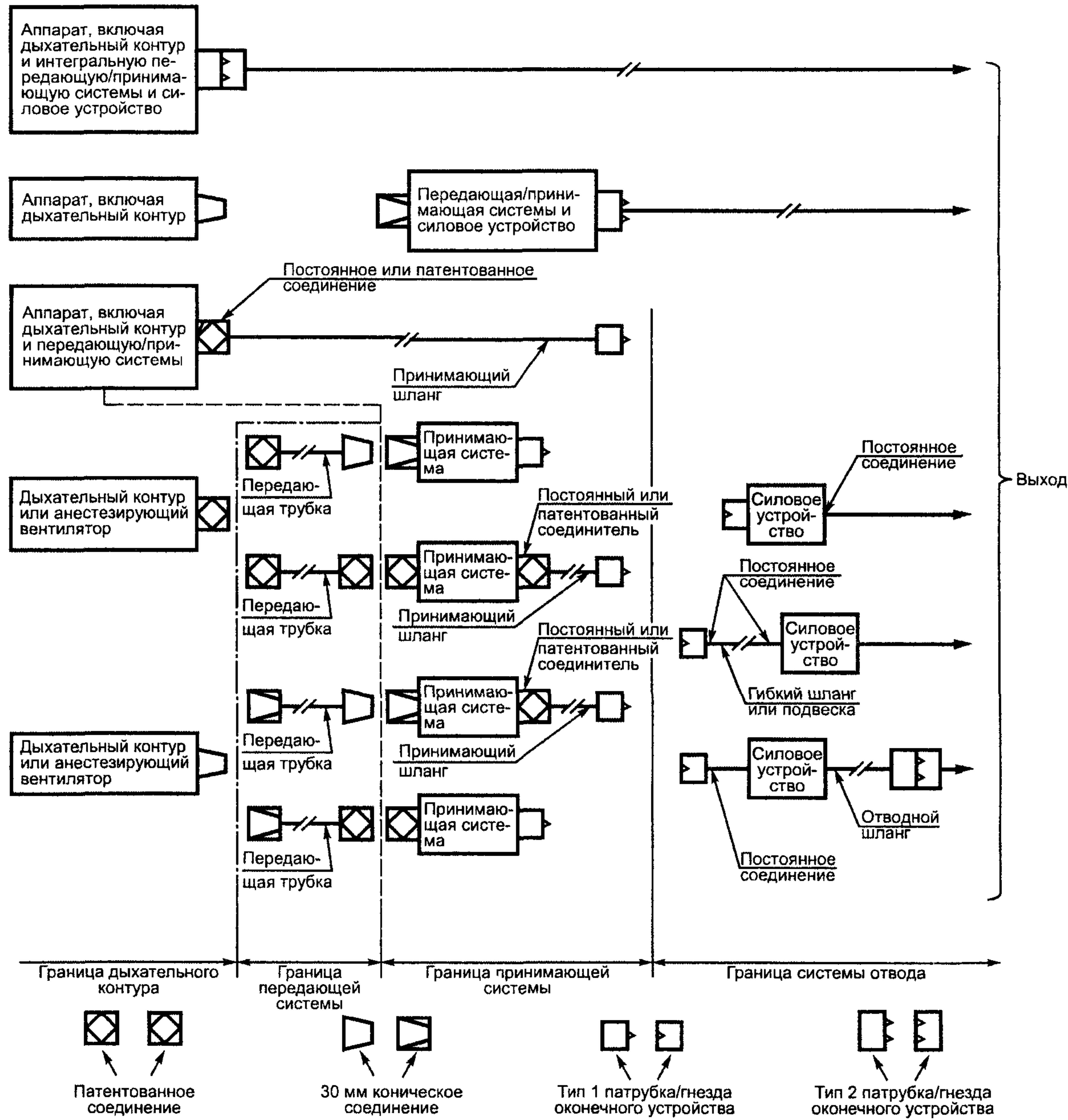
Рисунок 1 — Схема типичных соединений СВГС
