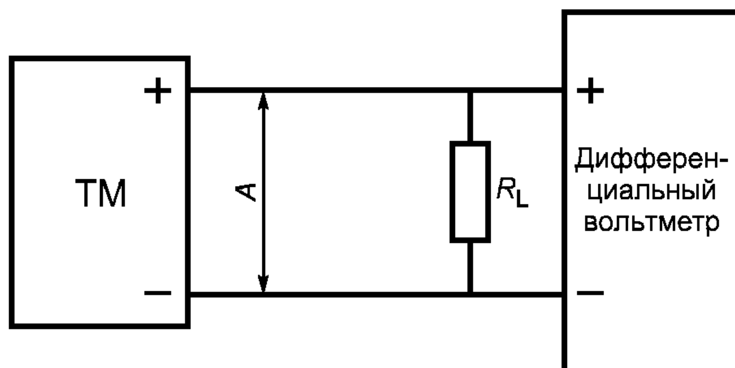
Рисунок 5 — Схема измерения выходного шума ТМ
