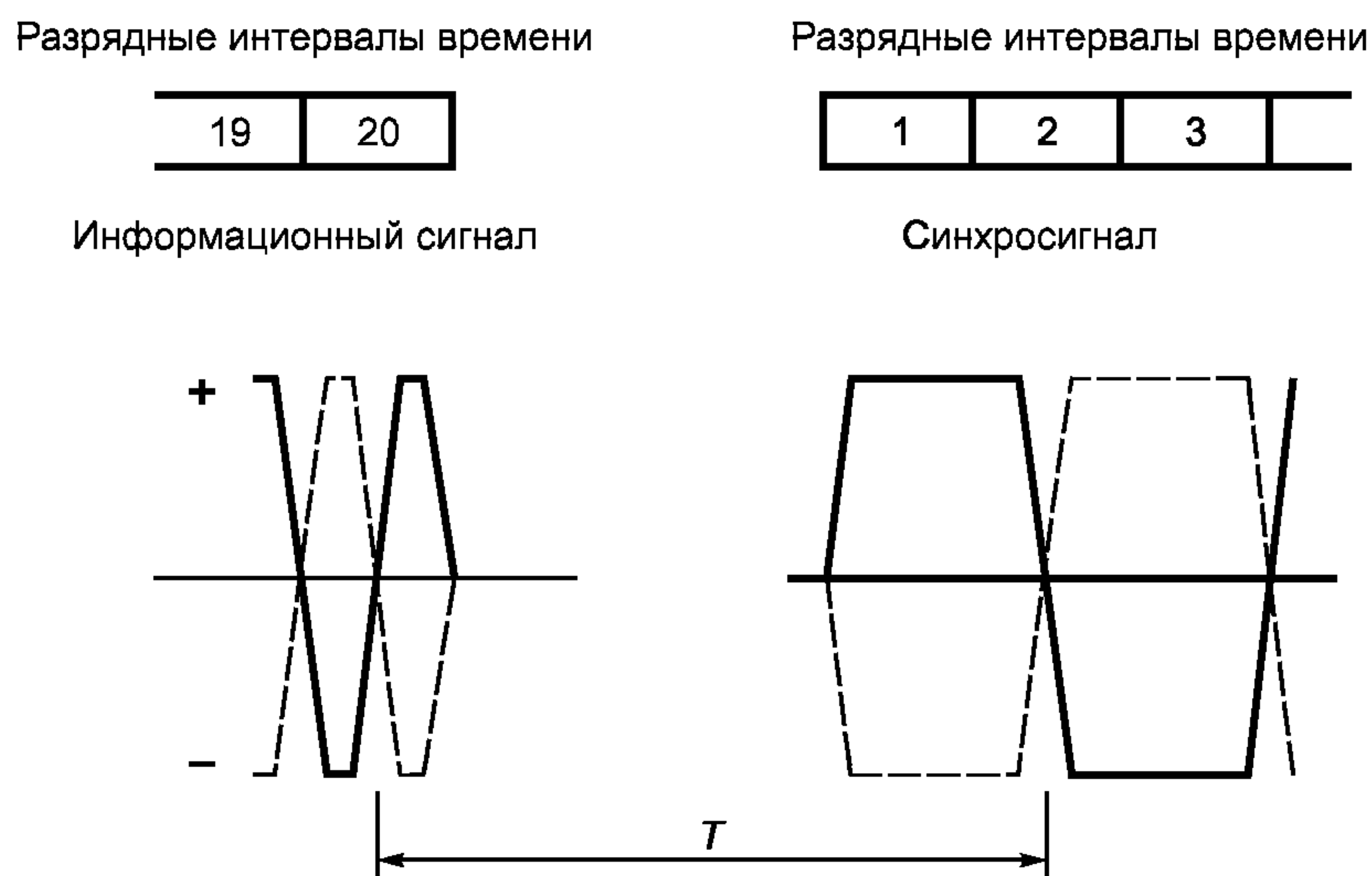
Рисунок 6 — Измерение временных пауз при передаче информации
