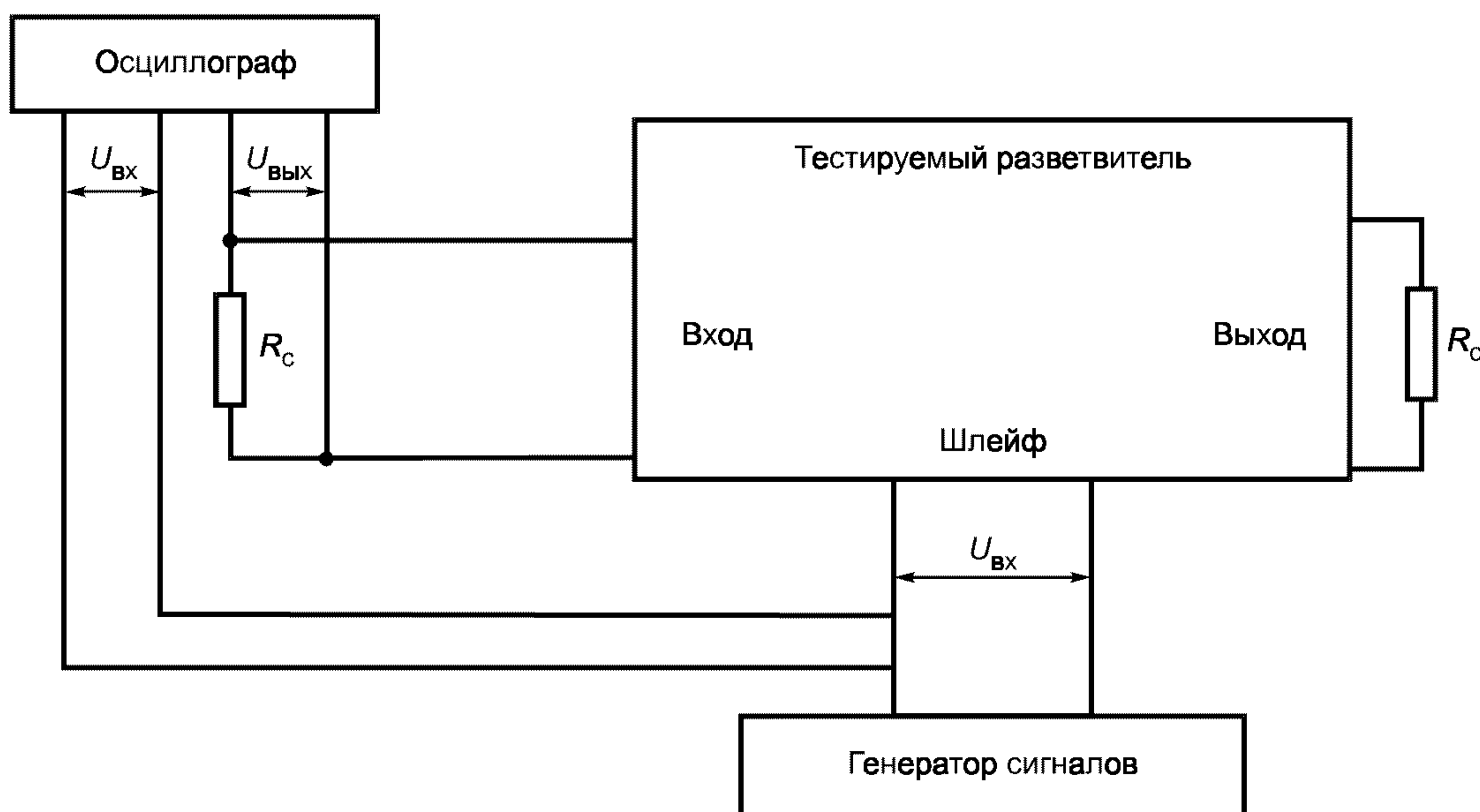
Рисунок 7 — Схема передачи сигнала от шлейфа к шине
