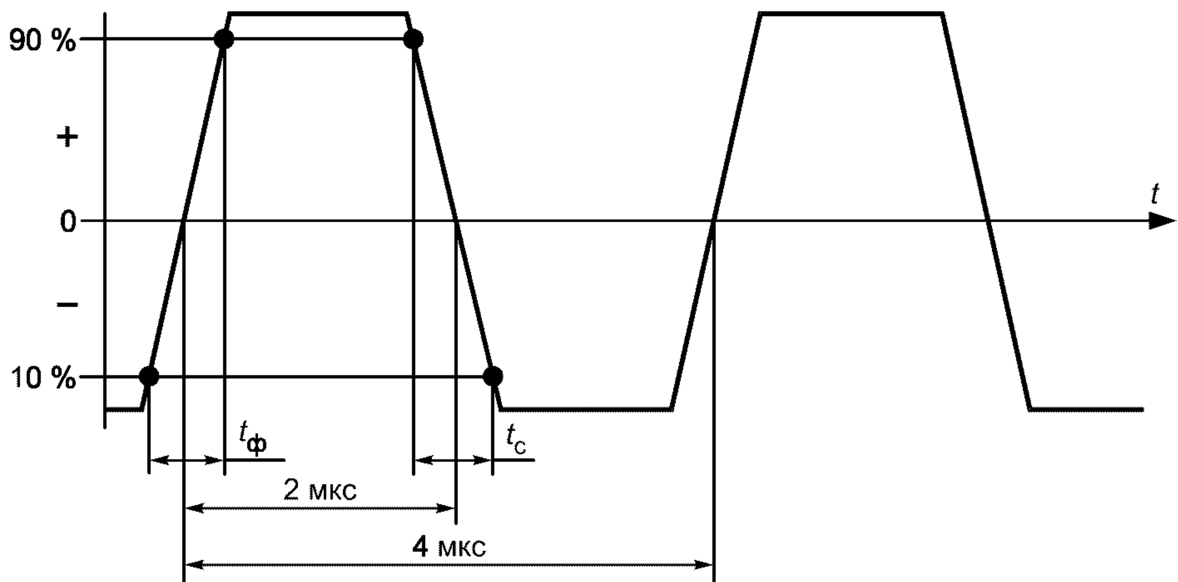
Рисунок 4 — Форма и параметры входного сигнала
