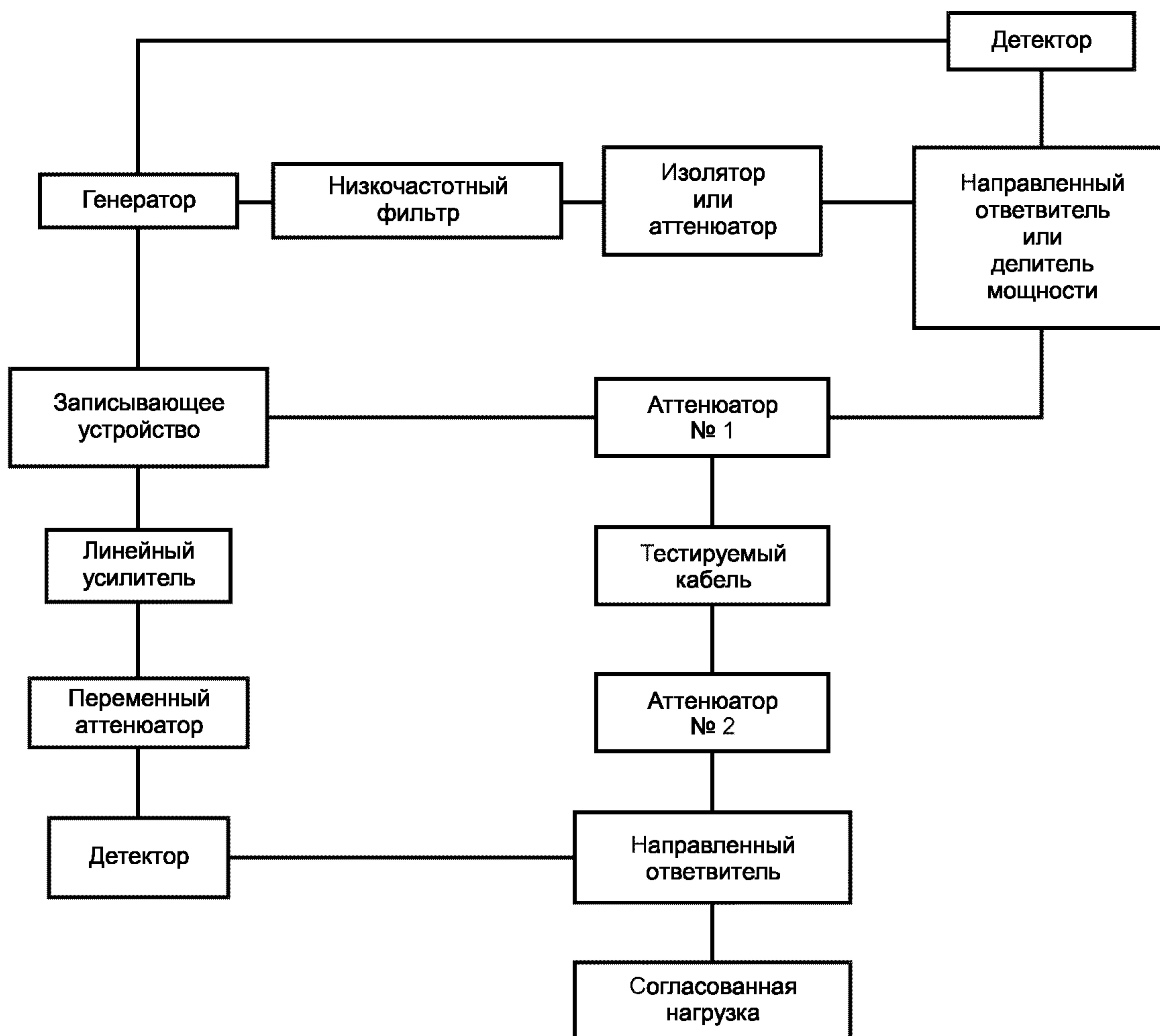
Рисунок 9 — Схема тестирования затухания в кабеле
