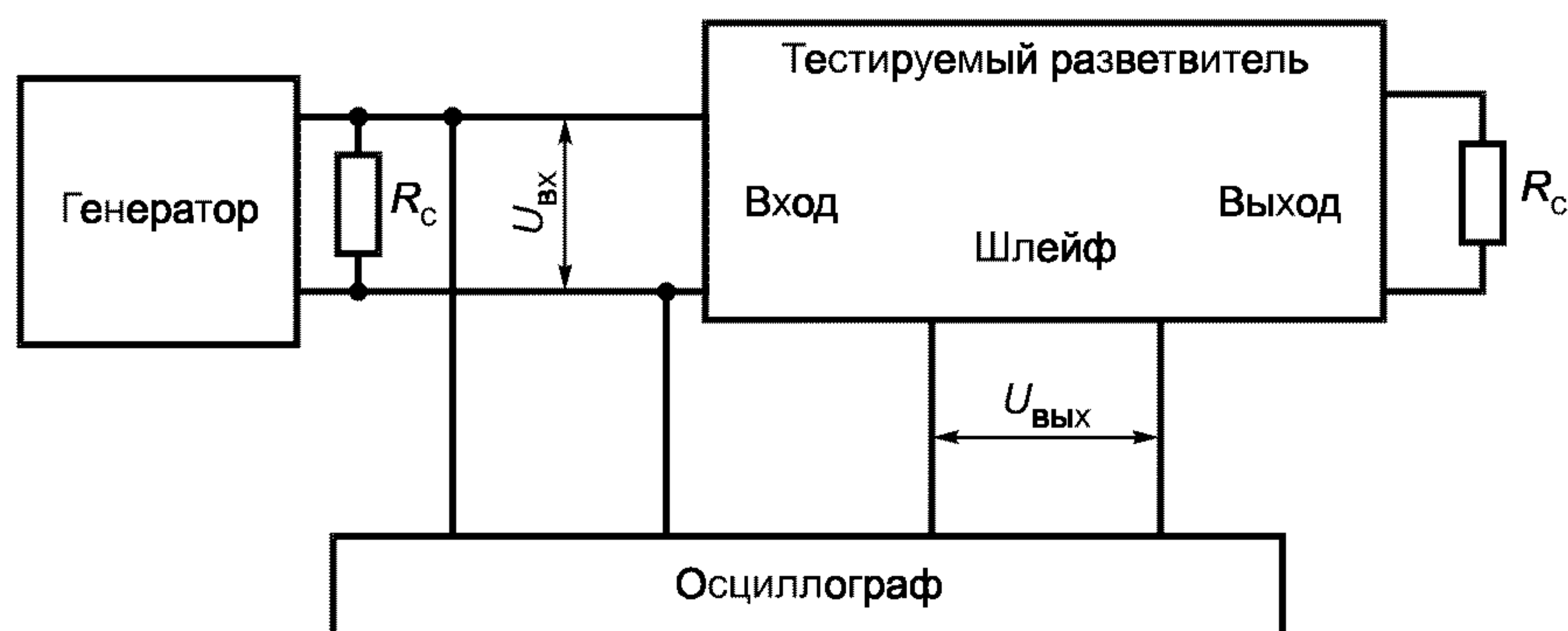
Рисунок 8 — Схема передачи сигнала от шины к шлейфу
