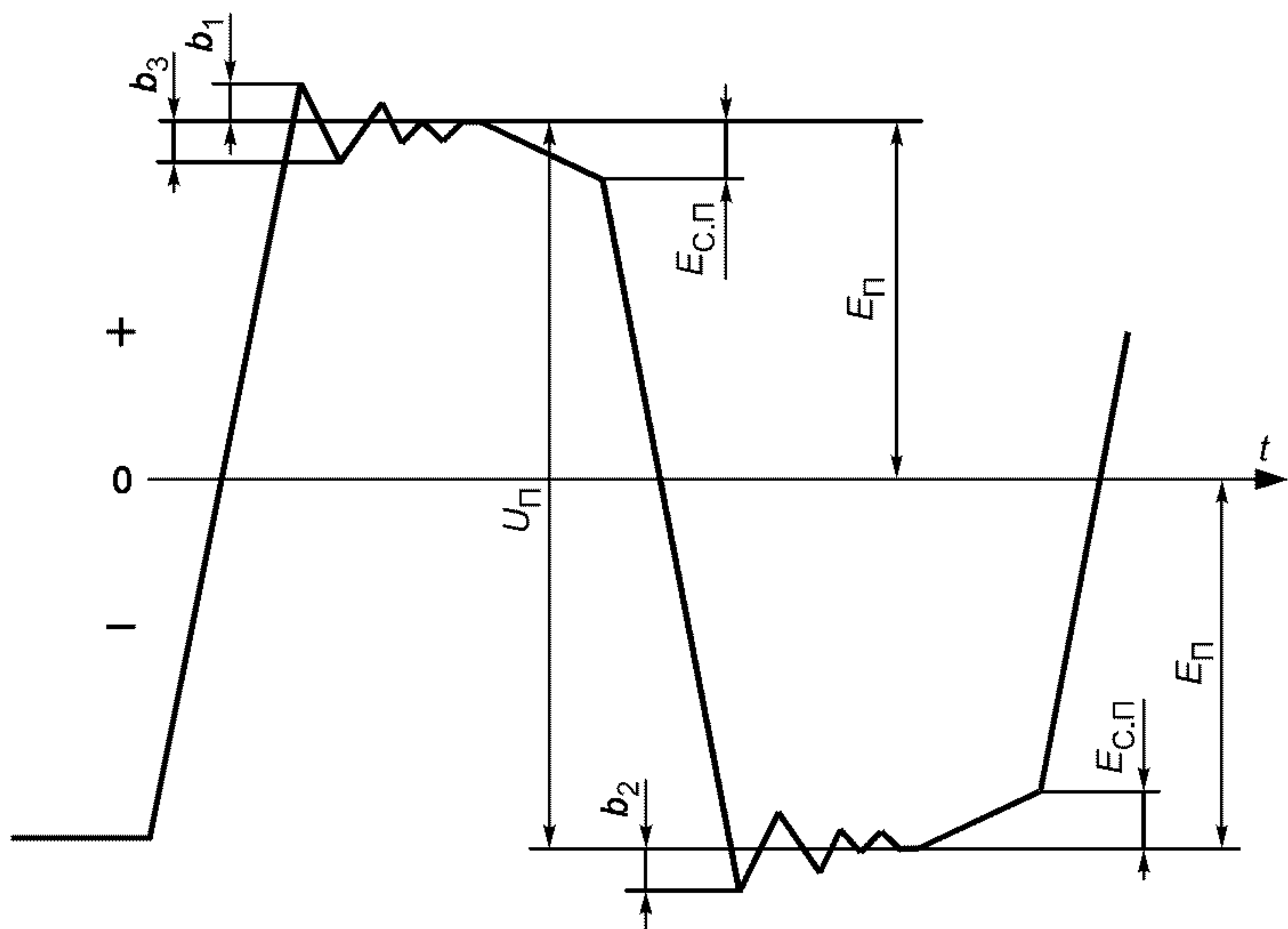
Рисунок 4 — Форма и параметры входного сигнала
