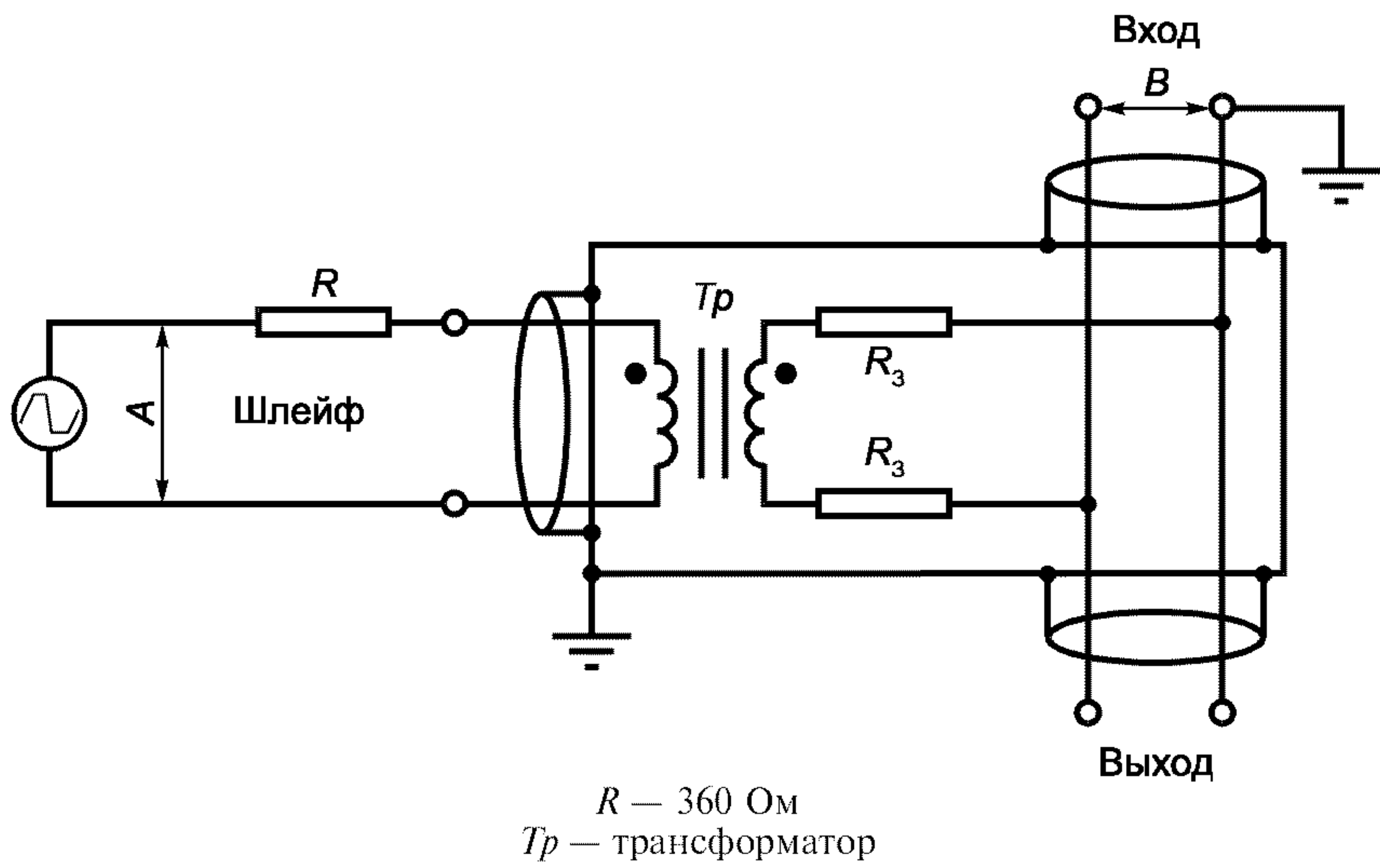
Рисунок 3 — Схема измерения выходного сигнала
