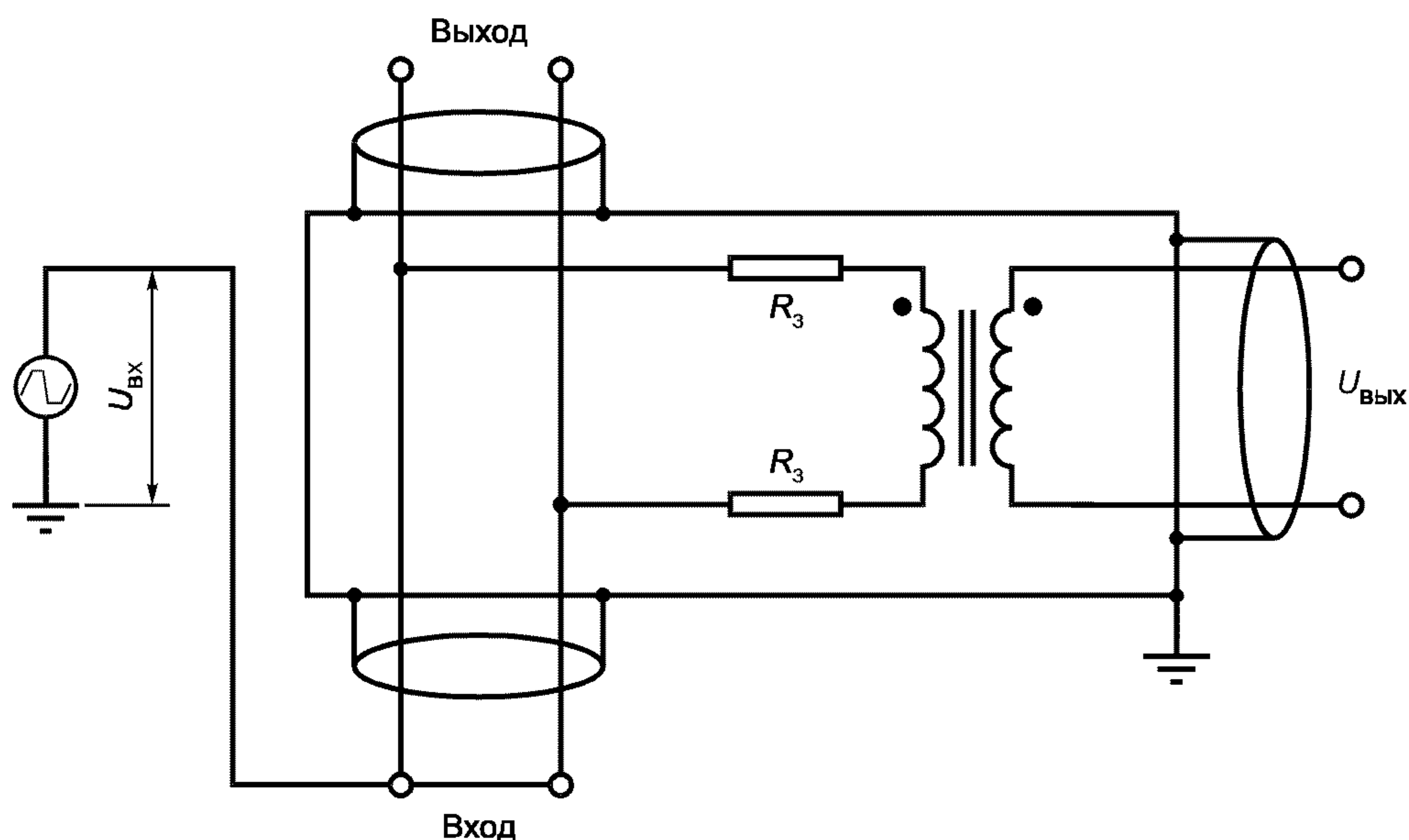
Рисунок 6 — Схема тестирования ослабления синфазного сигнала
