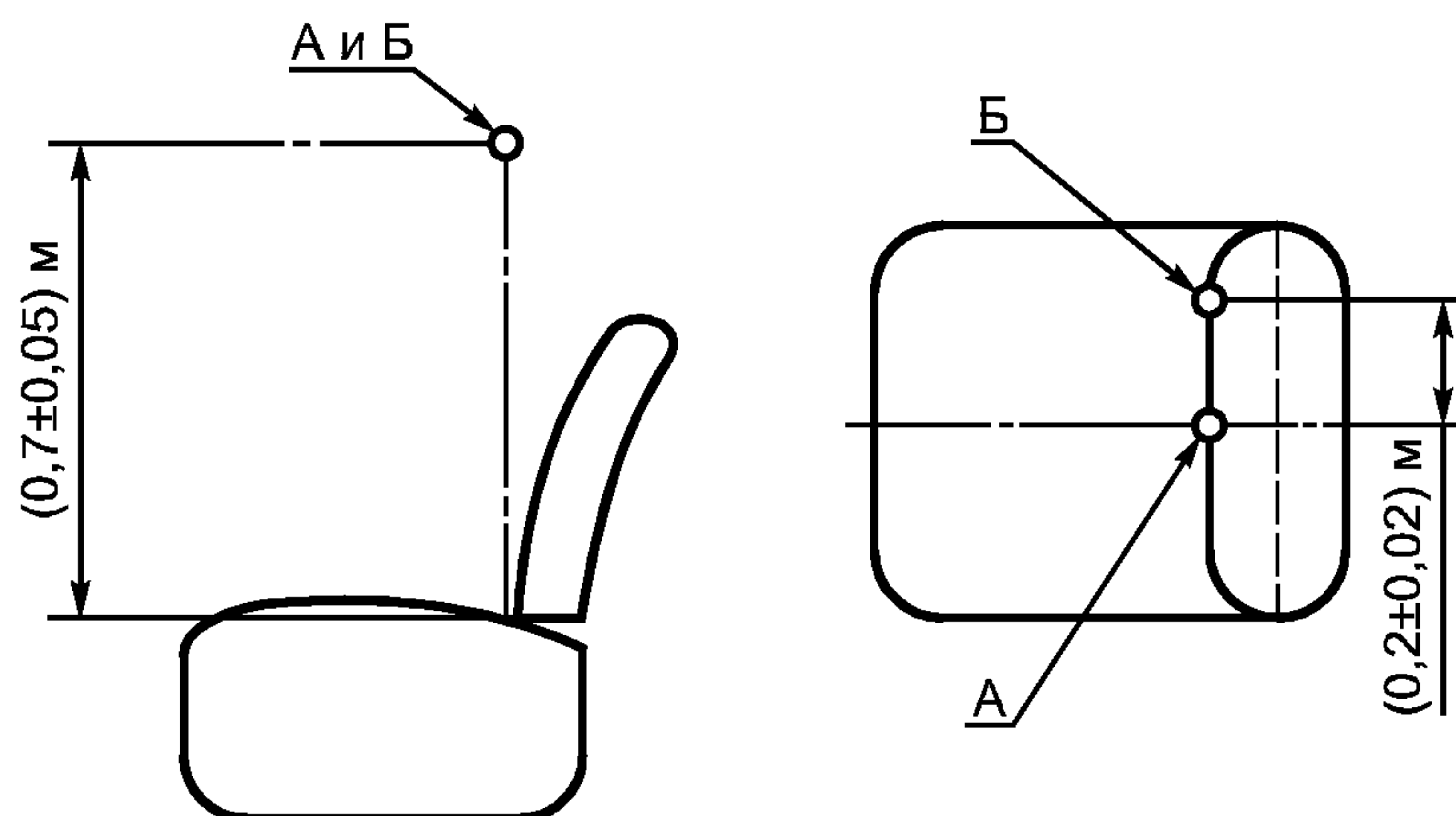
Рисунок 1 — Положение микрофона относительно сиденья
