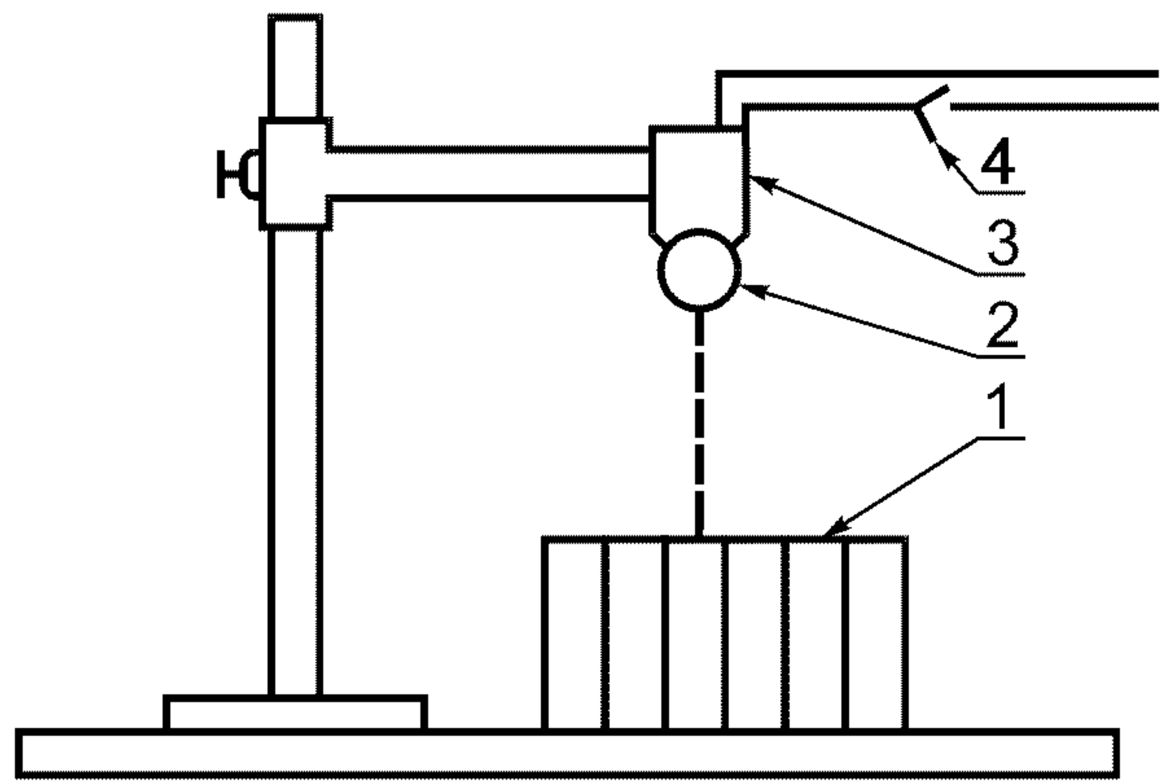
1 — моноблок; 2 — шар; 3 — электромагнит; 4 — реле
