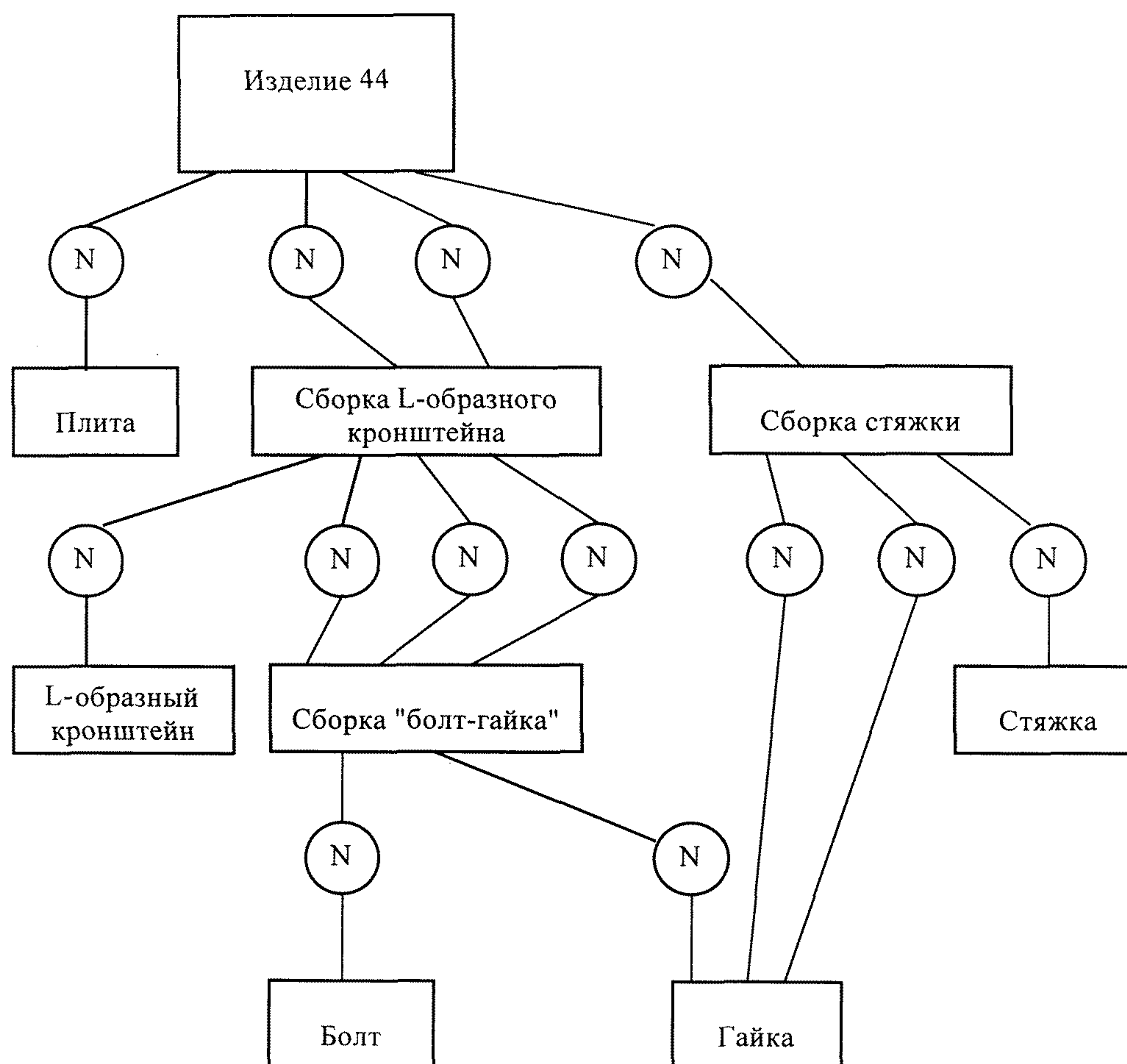
Рисунок Е.6 — Структура данных СП для изделия 44
