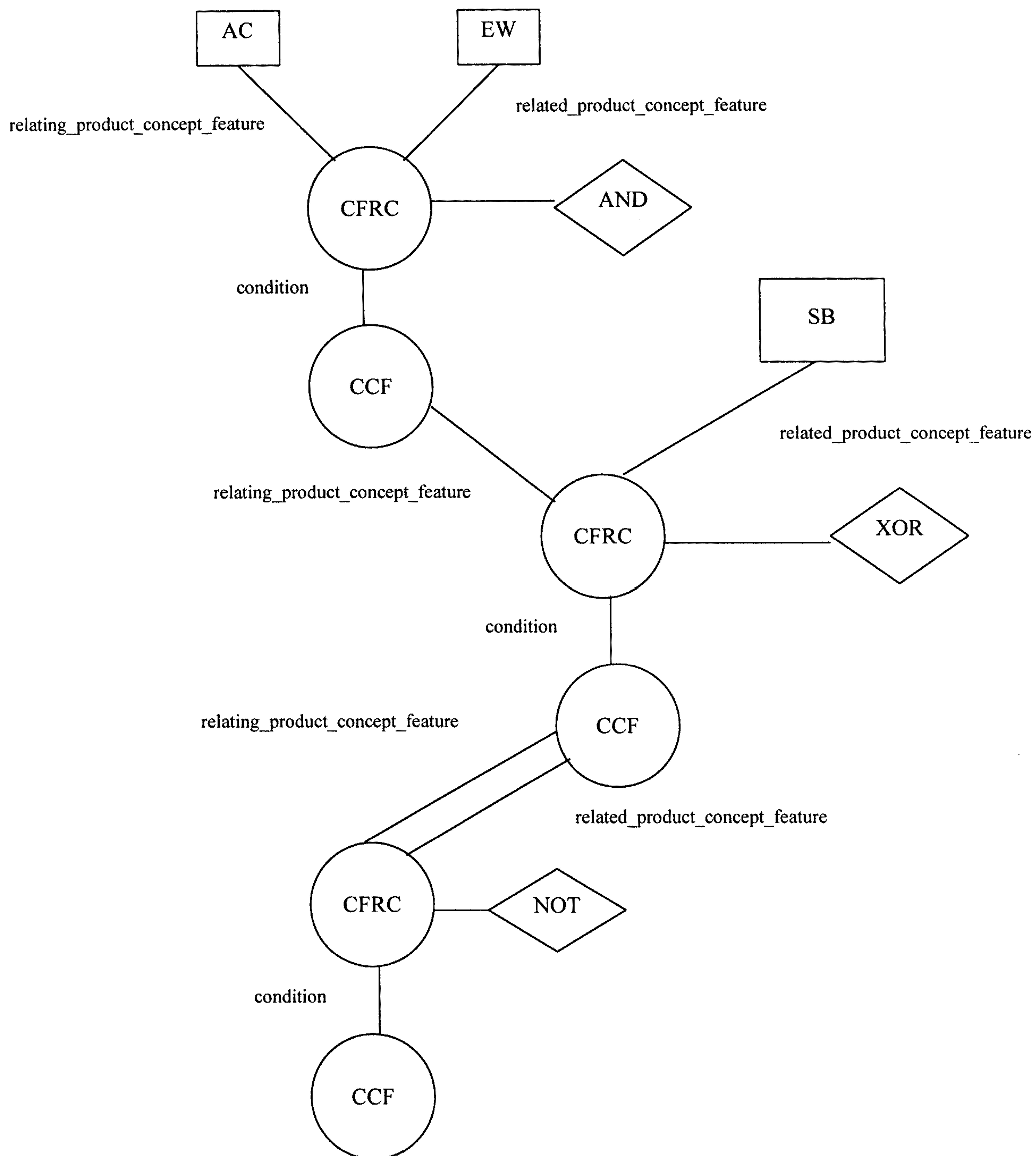
Рисунок E.12 — Альтернативные двоичные операторы для conditional_concept_feature
