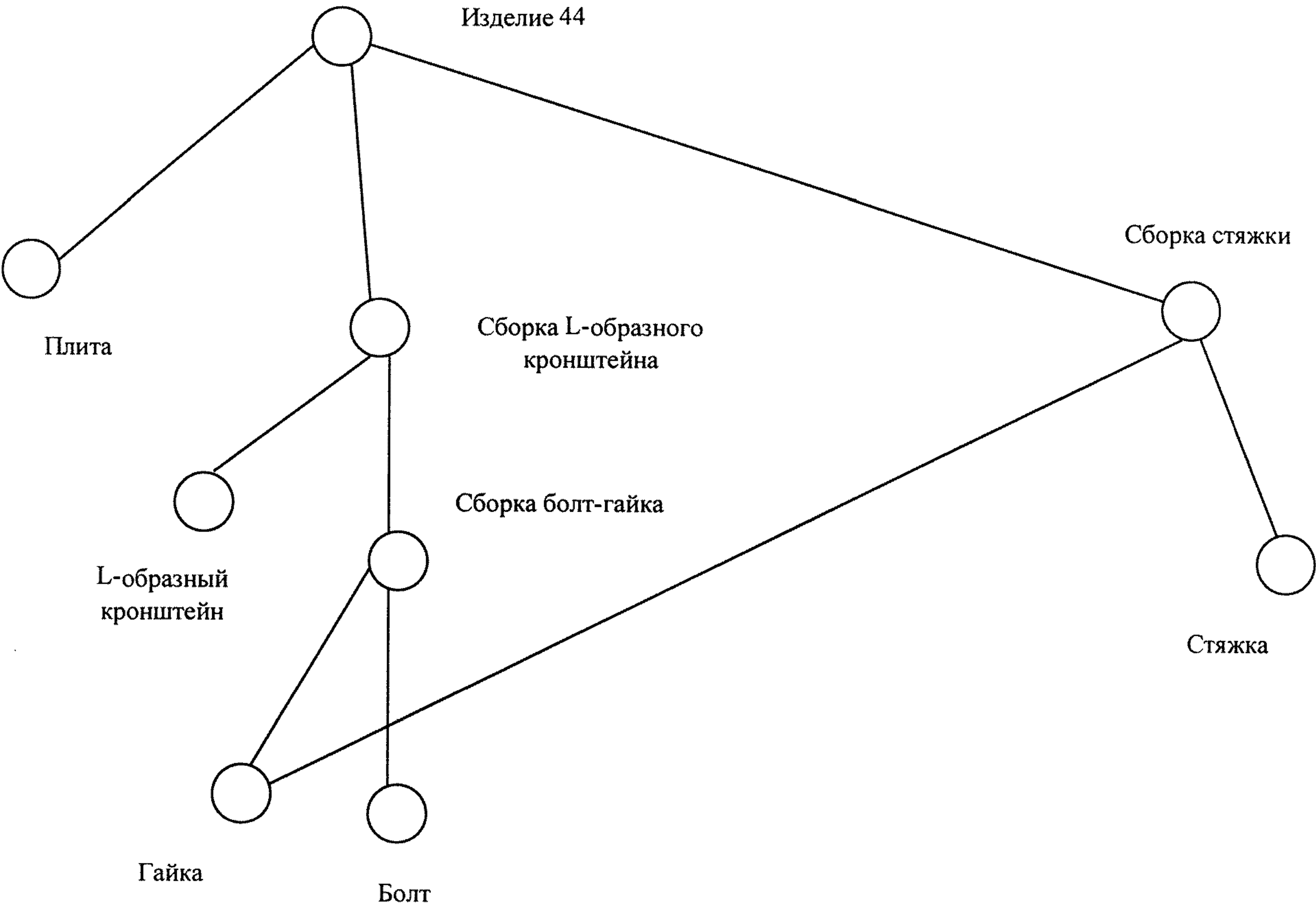
Рисунок Е.3 — Структура данных СП для изделия 44
