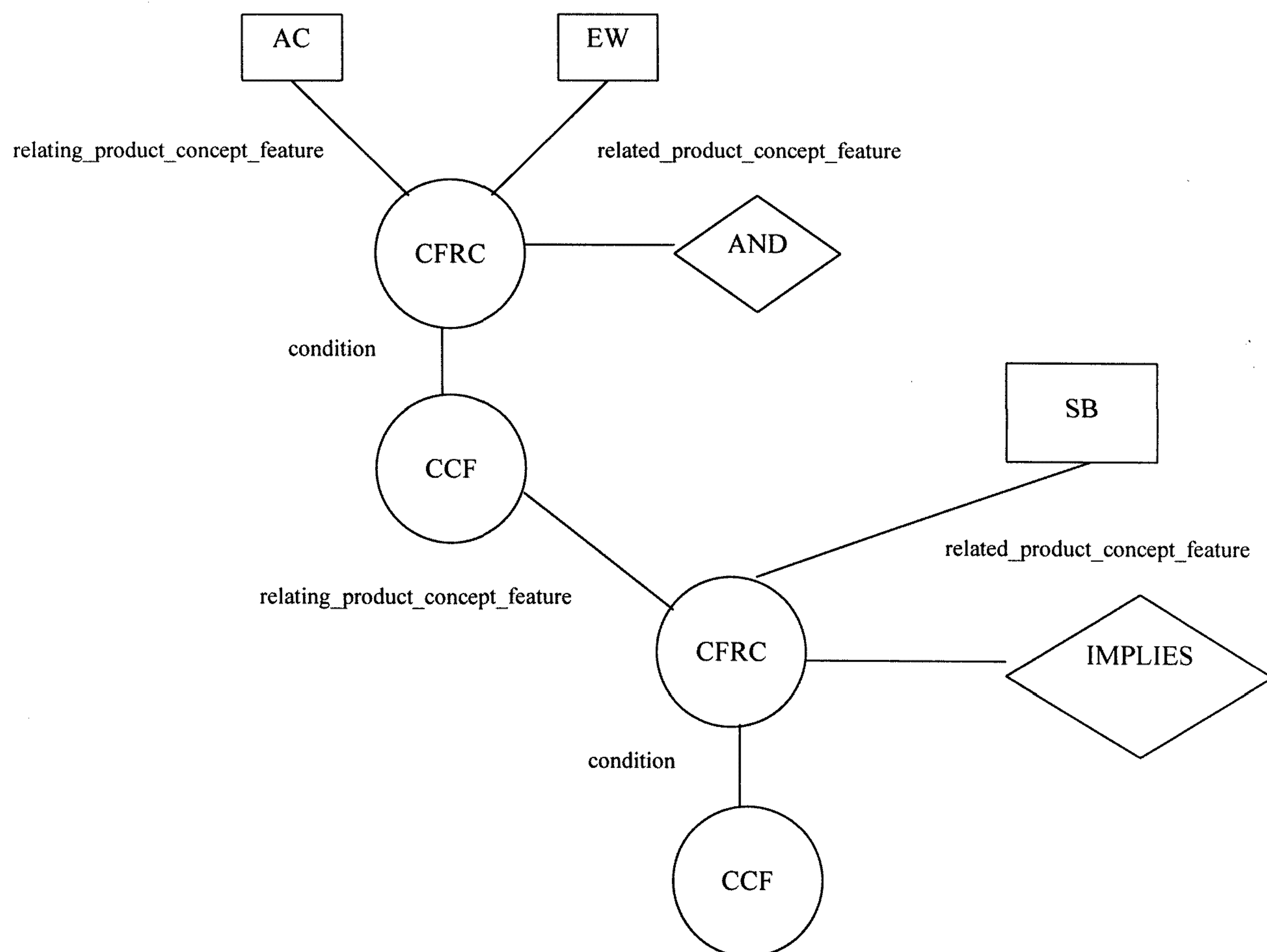
Рисунок Е.14 — Определенные операторы для conditional_concept_feature
