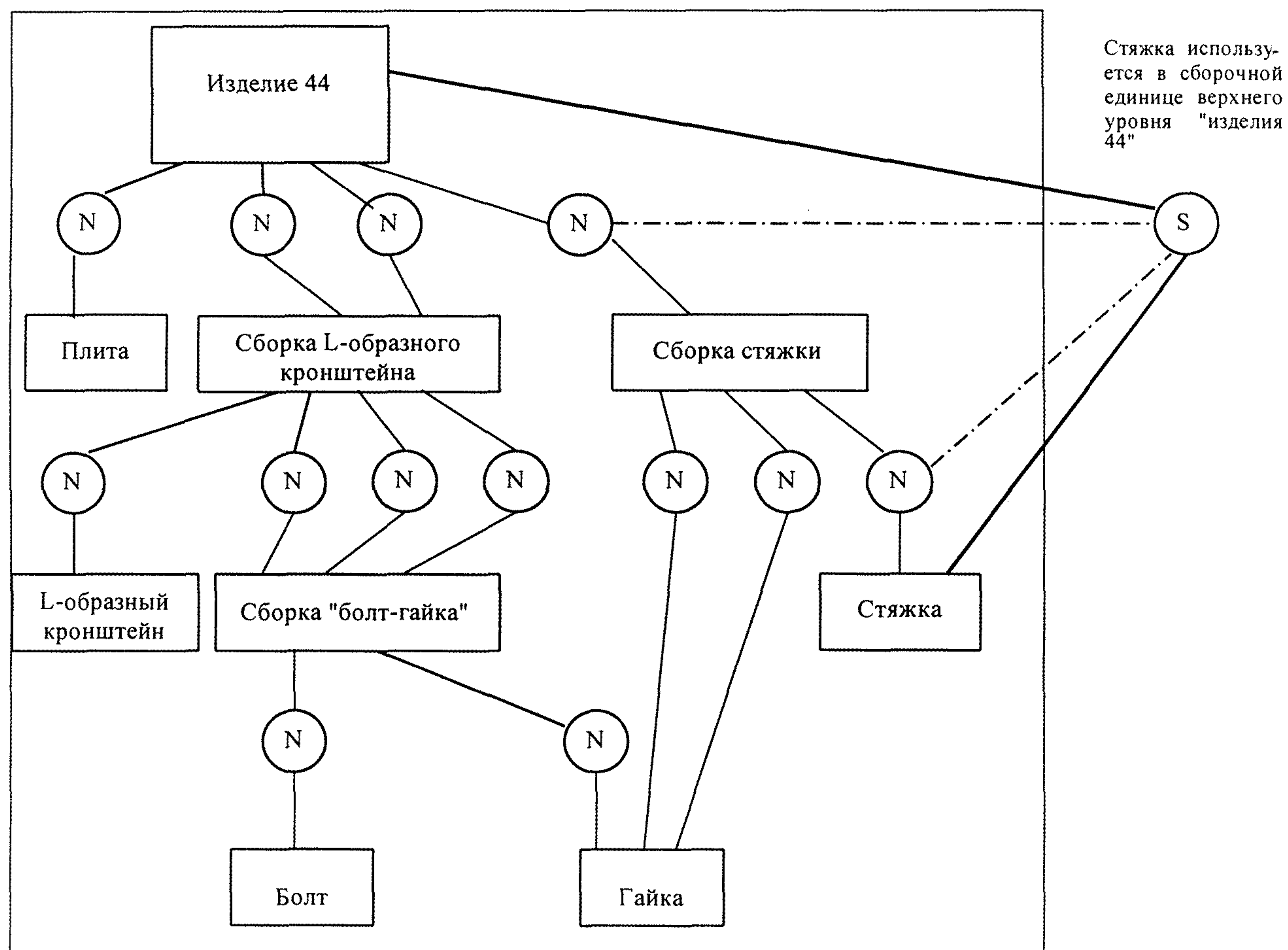
Рисунок E.8 — Элементарное применение в сборке верхнего уровня
