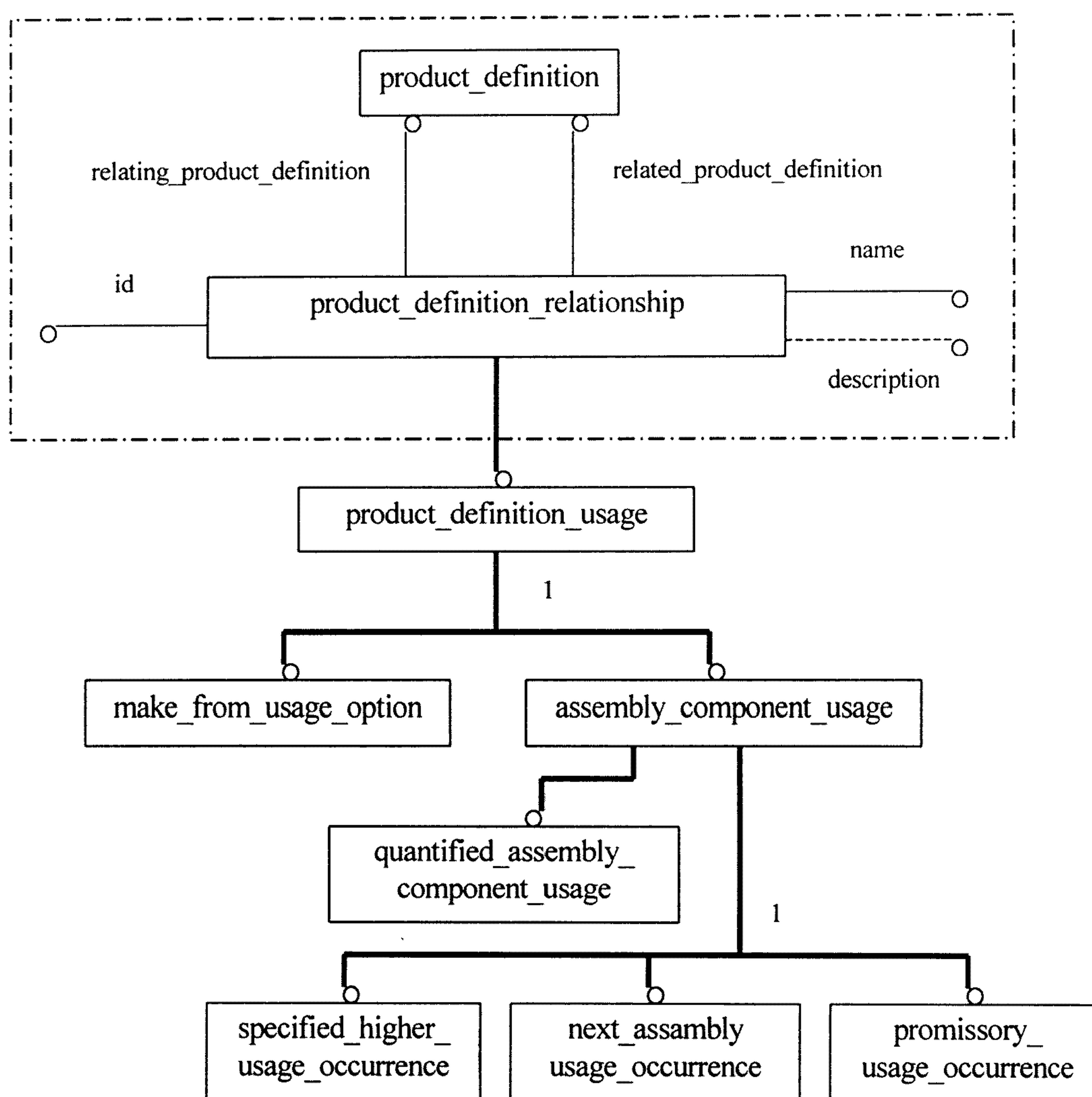
Рисунок 2 — Взаимосвязь объектов структуры изделия по ИСО 10303-41
