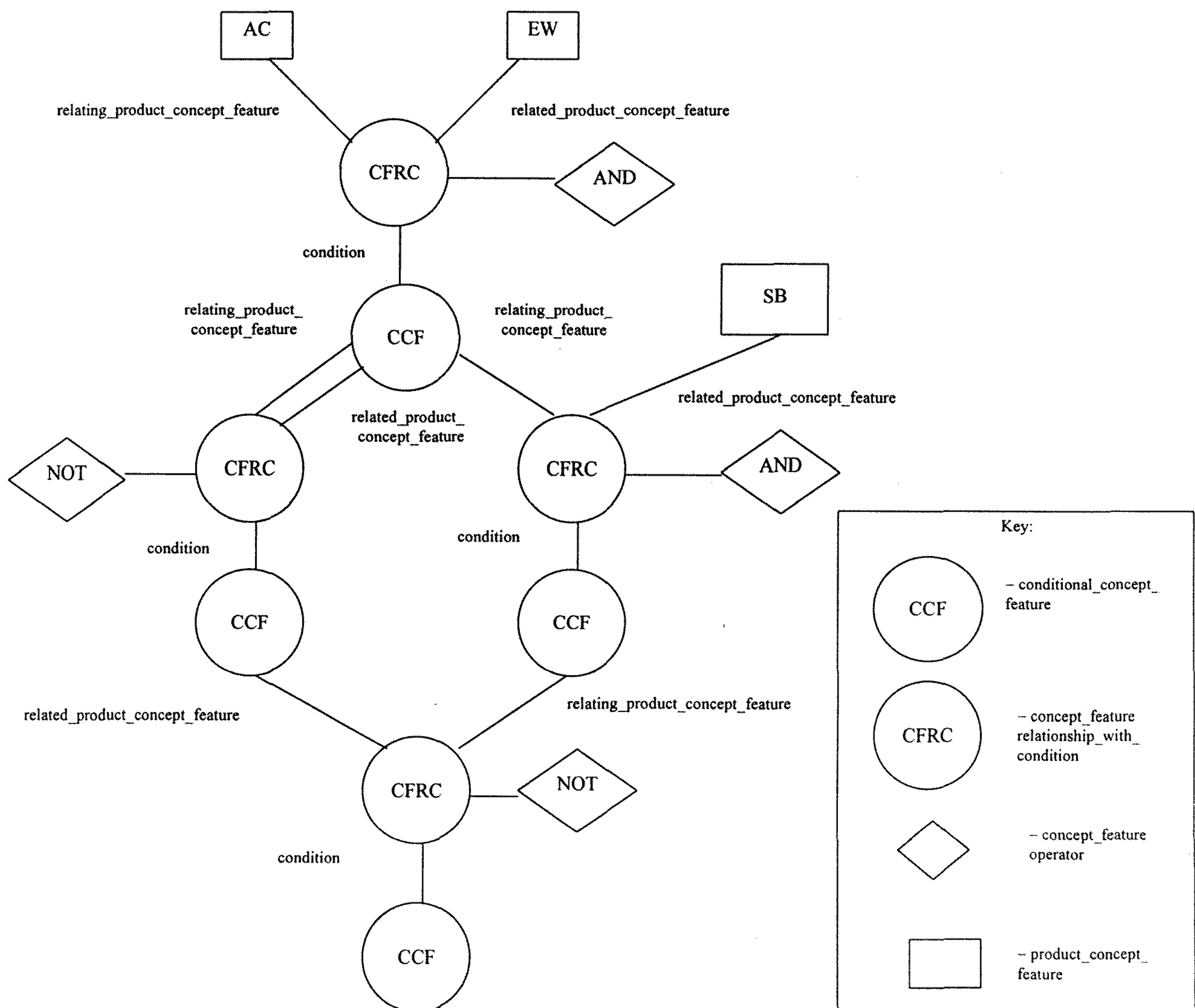
Рисунок E.13 — Двоичные операторы для conditional_concept_feature
