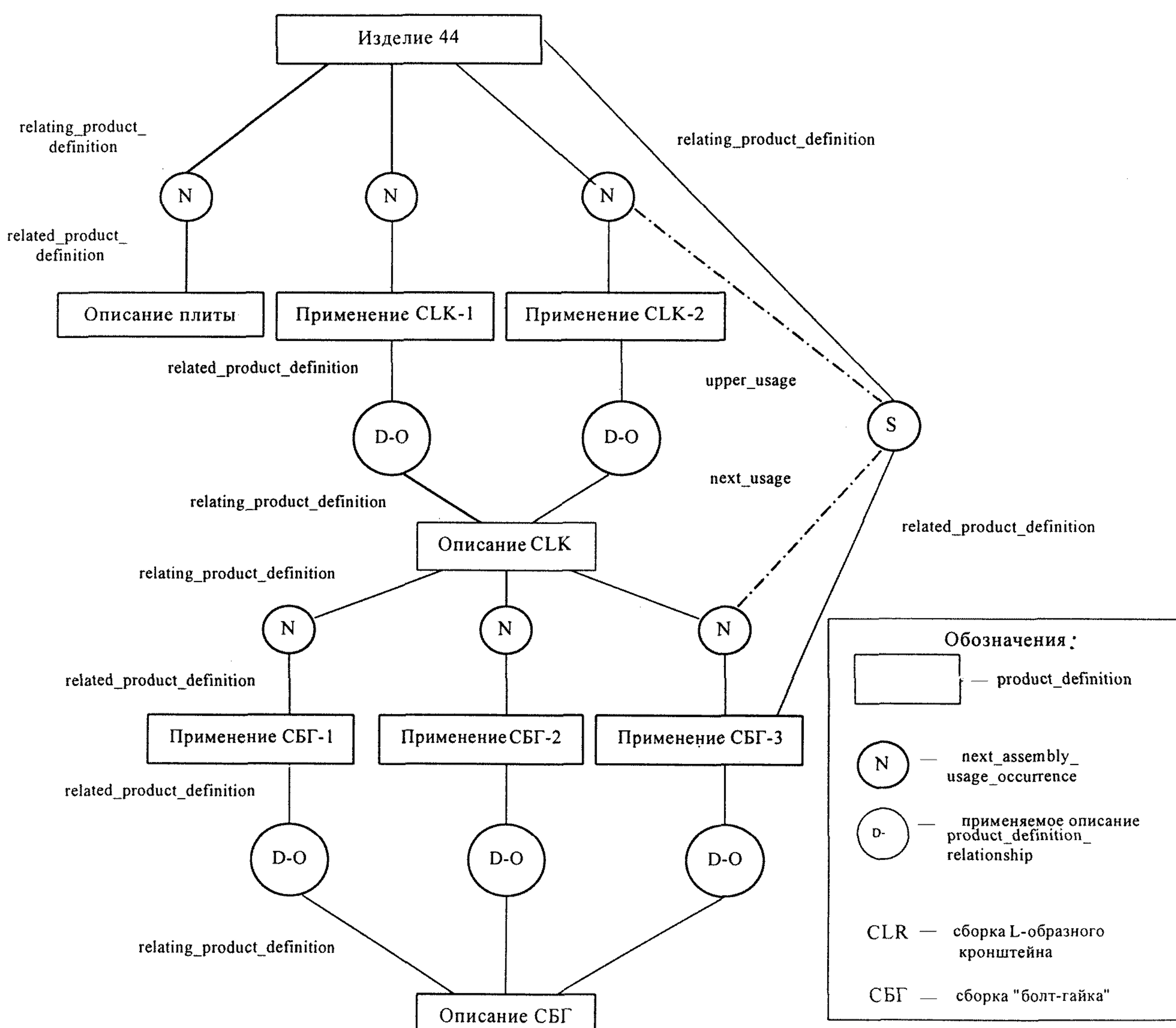
Рисунок Е.11 — Смешанная структура изделия 44
