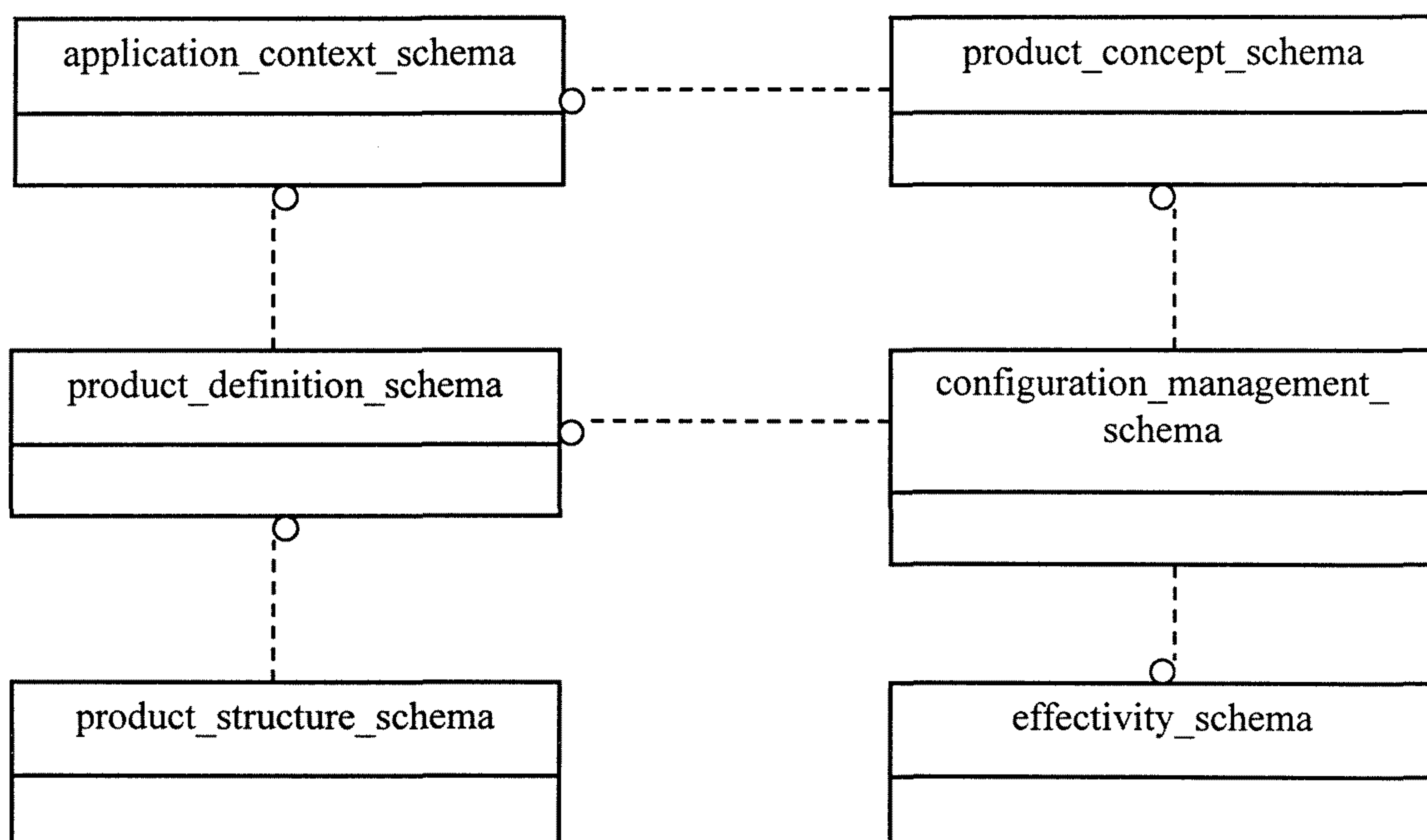
Рисунок 1 — Отношения схем интегрированных ресурсов
